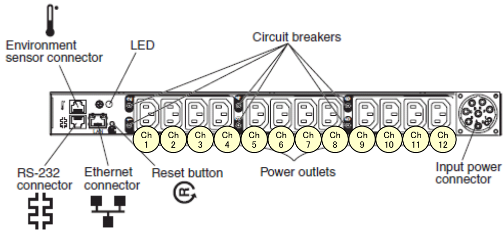
図 1-1 iPDU 各部の名称
