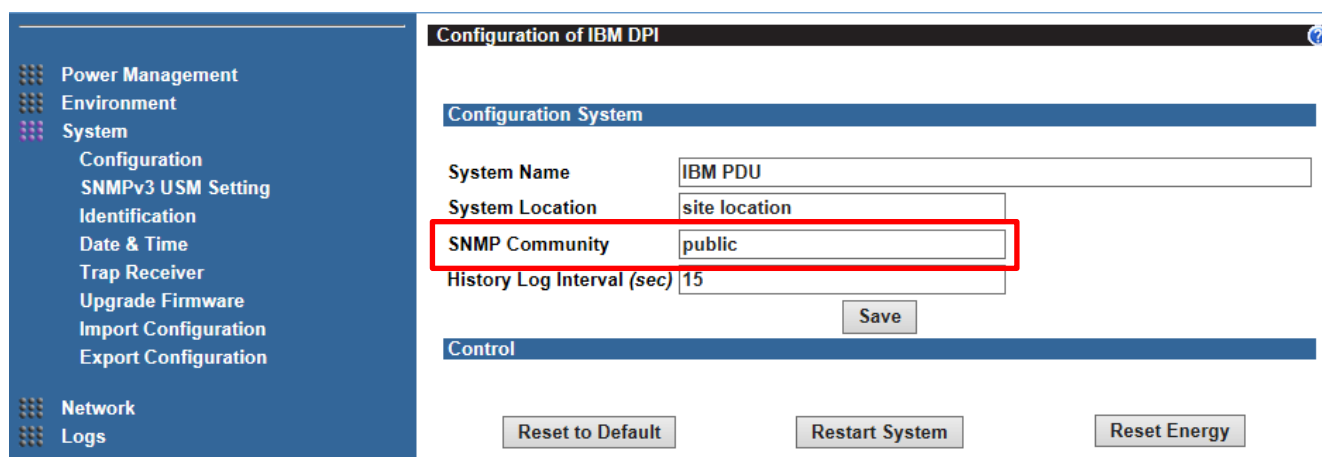
図 4-2 Configurationメニュー
