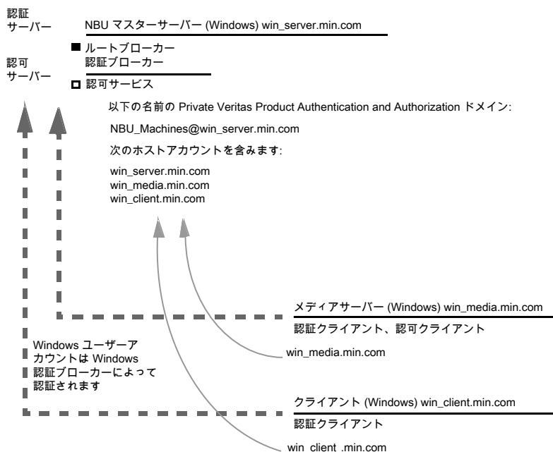
図 14-1 Windows システムだけが存在する構成の例
