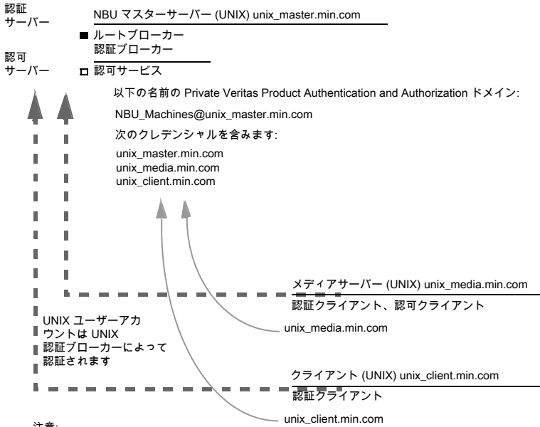
図 14-3 UNIX システムだけが存在する構成の例
