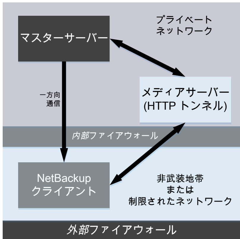
図 15-2 DMZ 設定での NetBackup クライアントとプライマリサーバーの通信
