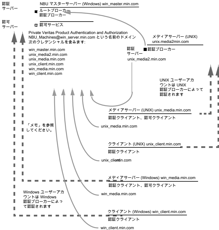
図 14-6 Windows プライマリサーバーが存在する複合構成の例
