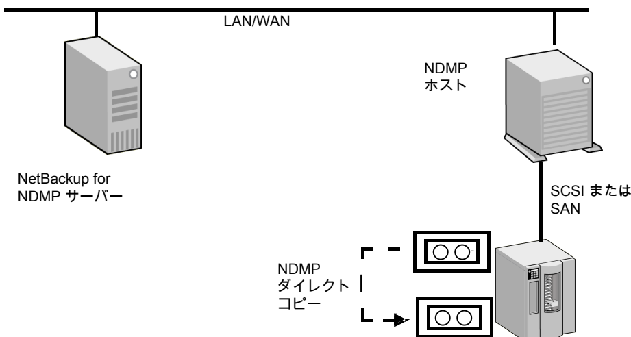
図 13-3 NDMP ホストにアクセス可能なテープドライブ間の NDMP ダイレクトコピー
