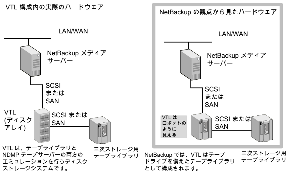
図 13-1 VTL を使用した NDMP ダイレクトコピーの概要
