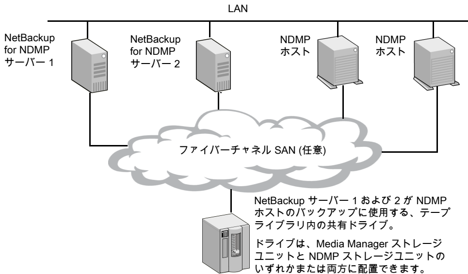
図 16-1 Shared Storage Option を使用した NDMP バックアップ
