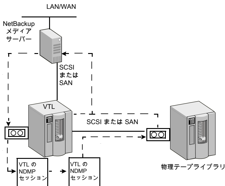
図 13-2 VTL を使用した NDMP ダイレクトコピーのデータの流れおよび制御
