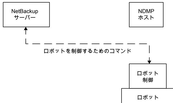
図 9-7 NetBackup サーバーに接続されたロボット制御
