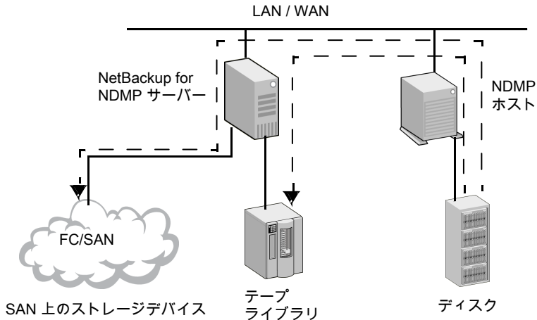
図 9-4 Media Manager デバイスへの NDMP バックアップ (リモート NDMP)
