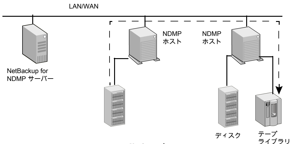
図 9-3 NDMP 3-Way バックアップとリストア
