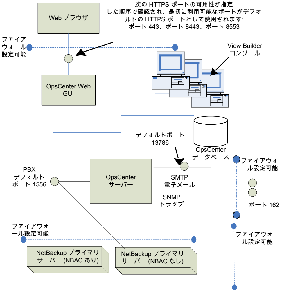
図 3-1 OpsCenter の主要なコンポーネントと通信方法
