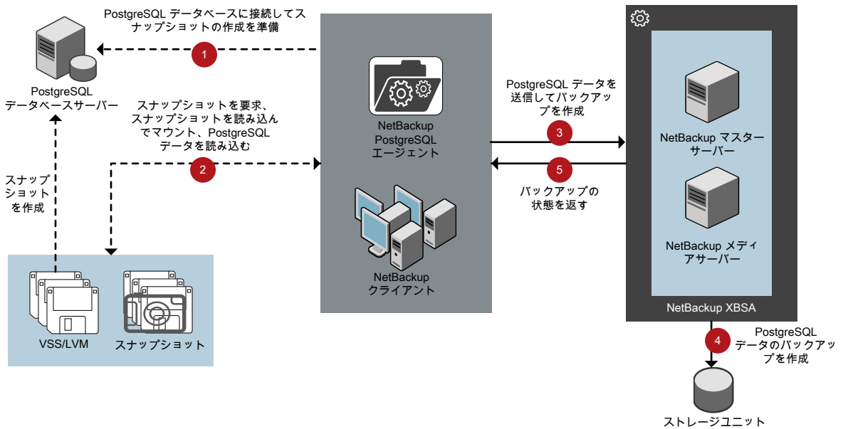
図 4-1 NetBackup for PostgreSQL のバックアップのワークフロー
