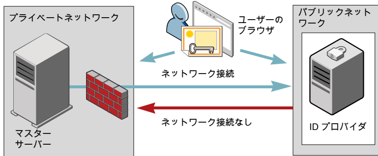
図 12-2 NAT 構成の例: プライベートネットワークのマスターサーバー
