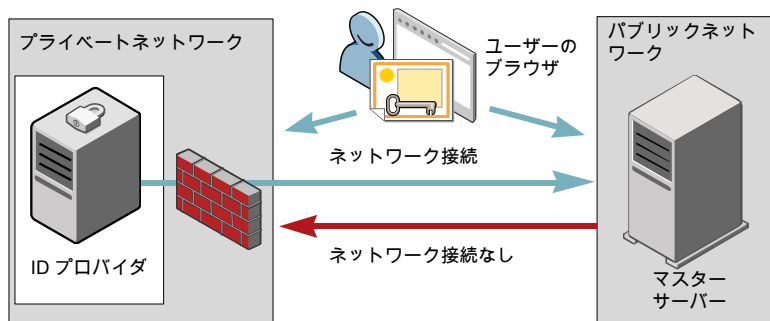
図 12-1 NAT 構成の例: プライベートネットワークの ID プロバイダ
