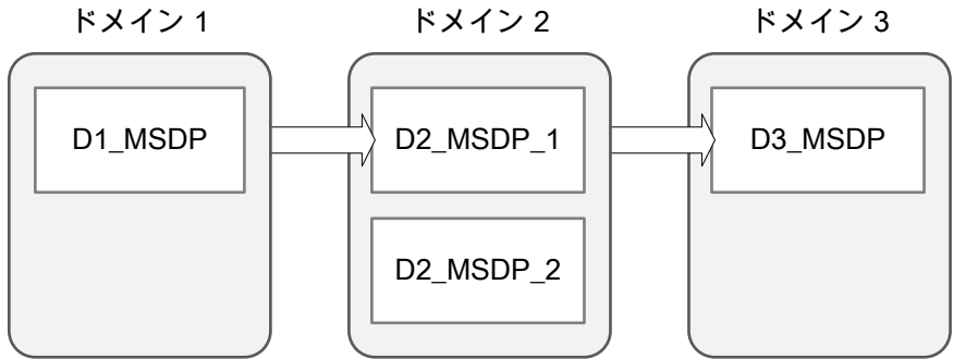
図 28-13 ストレージライフサイクルポリシーのトポロジの例
