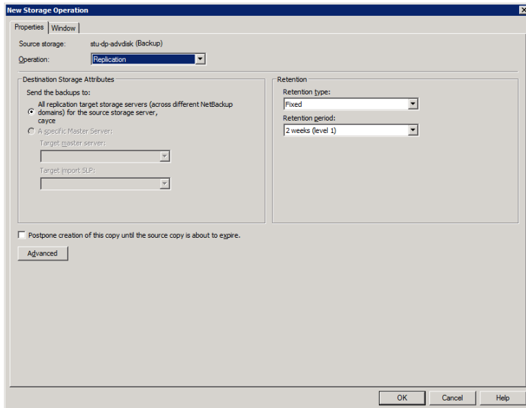
図 16-11 バックアップ操作に続くレプリケーション操作
