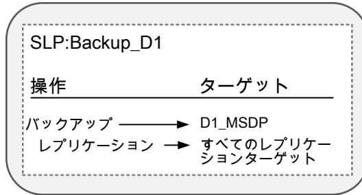
図 28-11 ストレージライフサイクルポリシーのトポロジーの例
