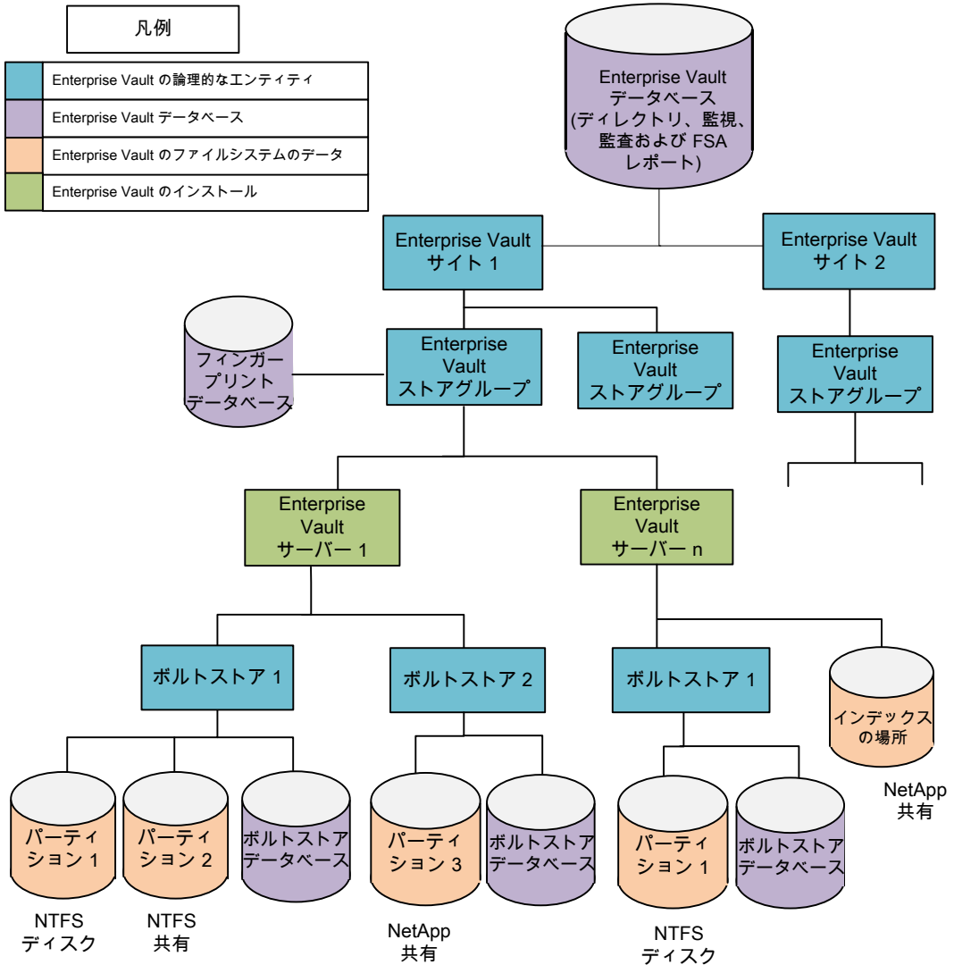
図 1-1 Enterprise Vault 10.0 以降の階層
