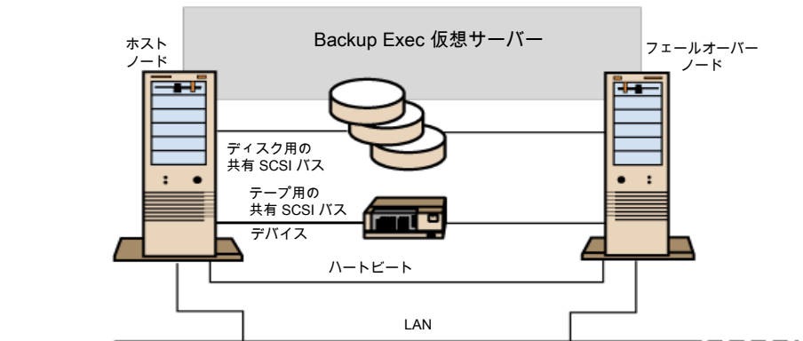
図 18-2 共有 SCSI バス上のテープデバイスを使用する 2 ノードクラスタ
