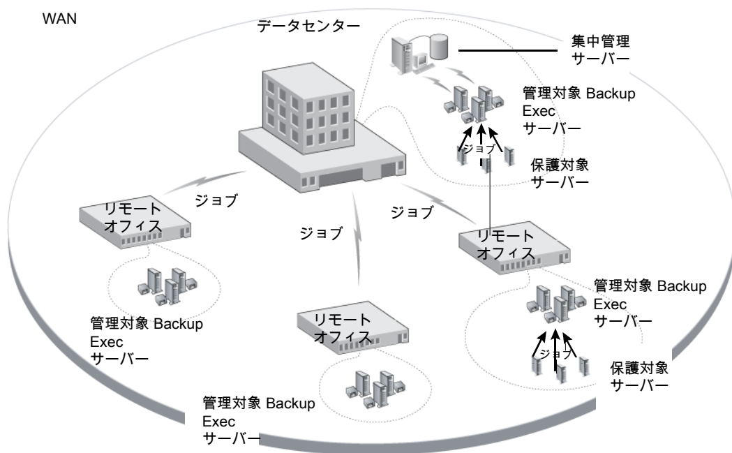
図 L-2 CASO 構成の Backup Exec 環境: WAN
