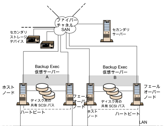
図 17-4 Central Admin Server Option を使用したファイバーチャネル SAN 上の 2 つの 2 ノードクラスタ
