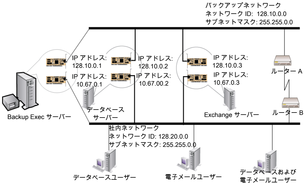
図 14-1 バックアップネットワークの例
