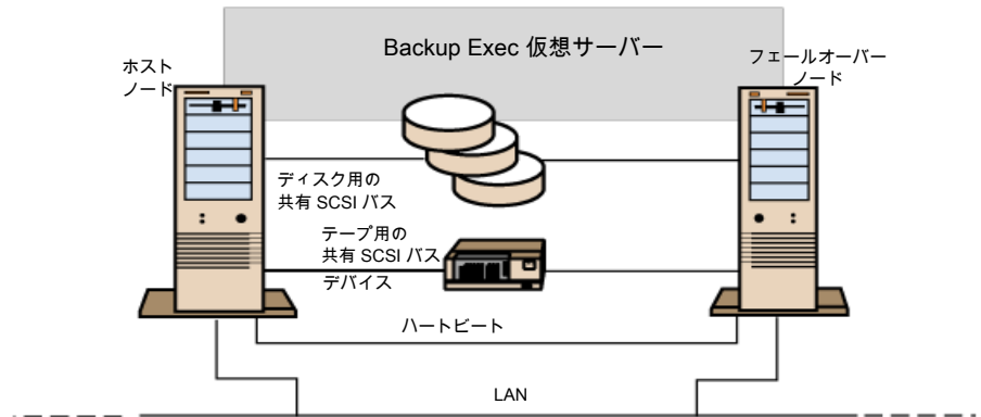
図 17-2 共有 SCSI バス上のテープデバイスを使用する 2 ノードクラスタ
