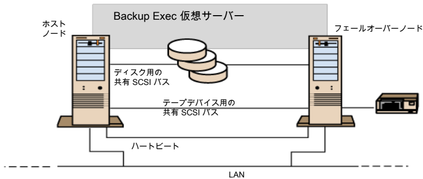
図 17-3 バス端に接続したテープデバイスを使用するクラスターの例
