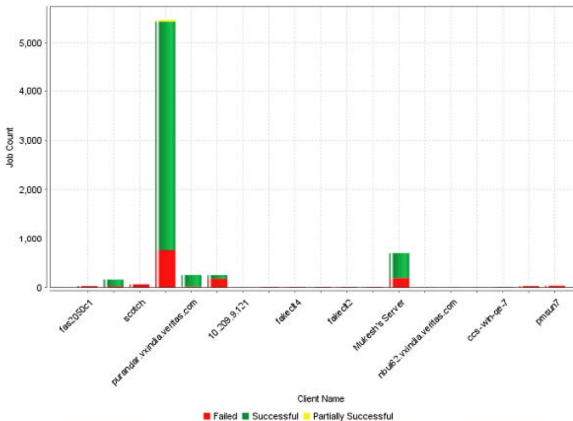
図 2-62 [クライアントごとのジョブの成功率 (Job Success by Client)] レポート
