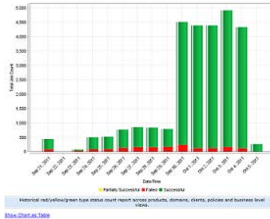
図 2-44 [ジョブ状態 (Job Status)] ([履歴 (Historical)]) レポート
