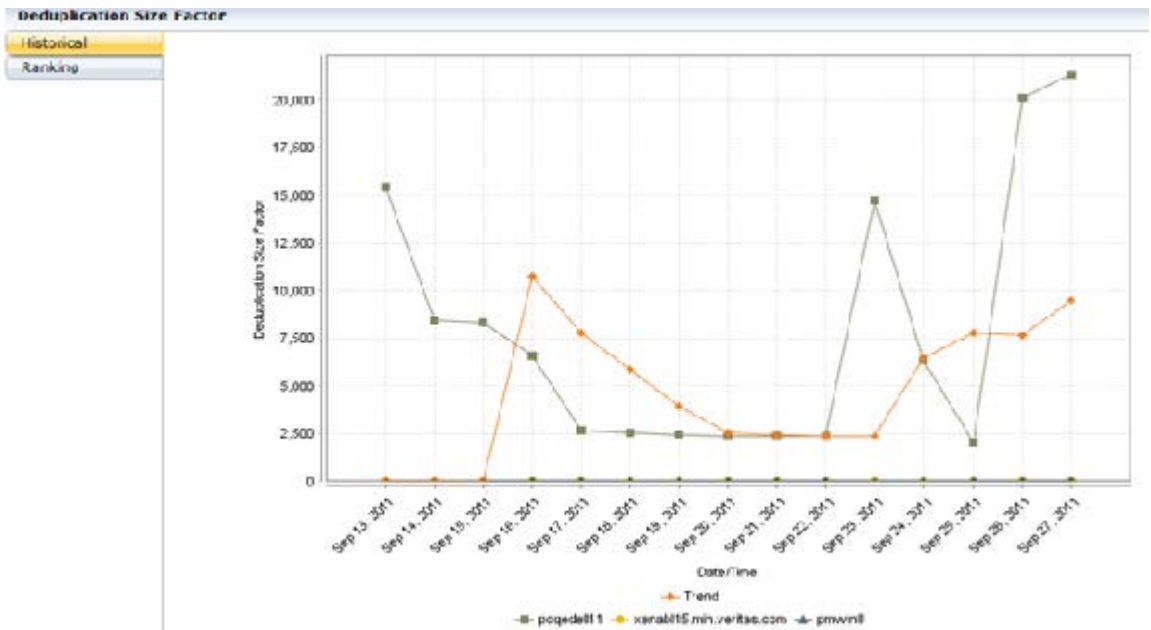
図 2-1 [サイズの重複排除の係数 (Deduplication Size Factor)]レポート ([履歴 (Historical)])
