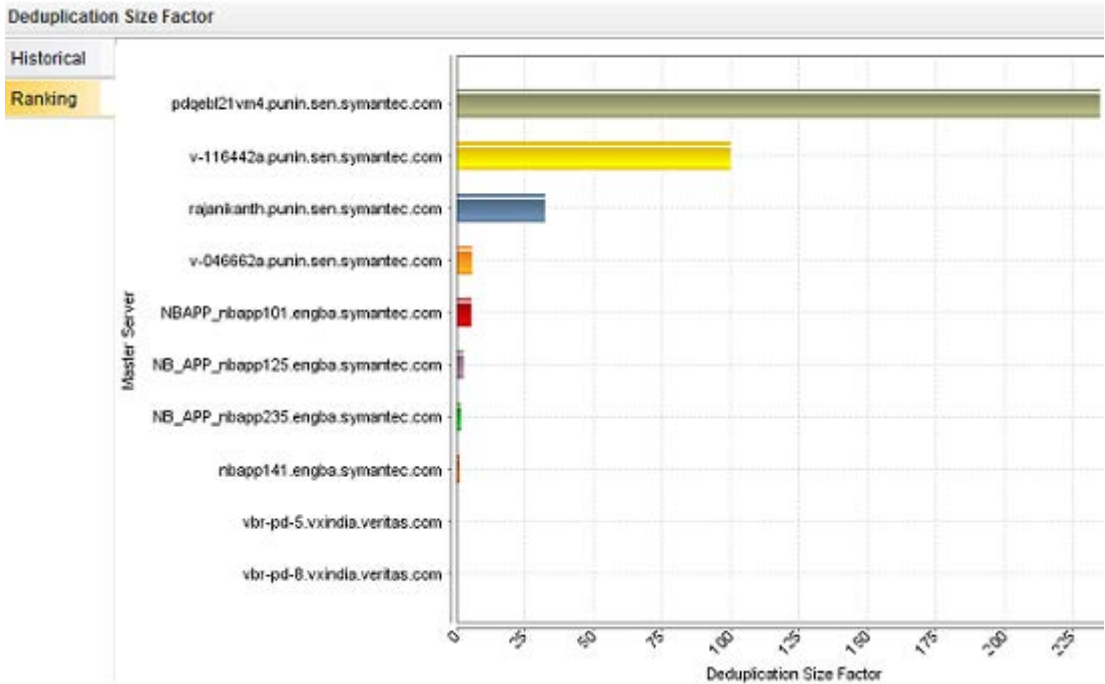
図 2-2 [サイズの重複排除の係数 (Deduplication Size Factor)] レポート ([ランキング (Ranking)])
