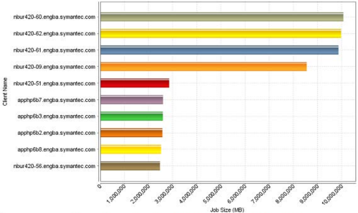
図 2-15 [ジョブのサイズ (Job Size)]レポート ([ランキング (Ranking)])
