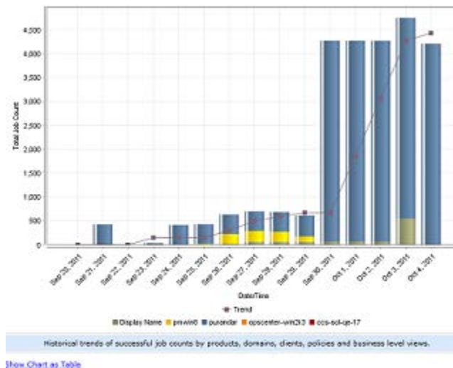
図 2-38 [成功したジョブ数 (Successful Job Count)] レポート
