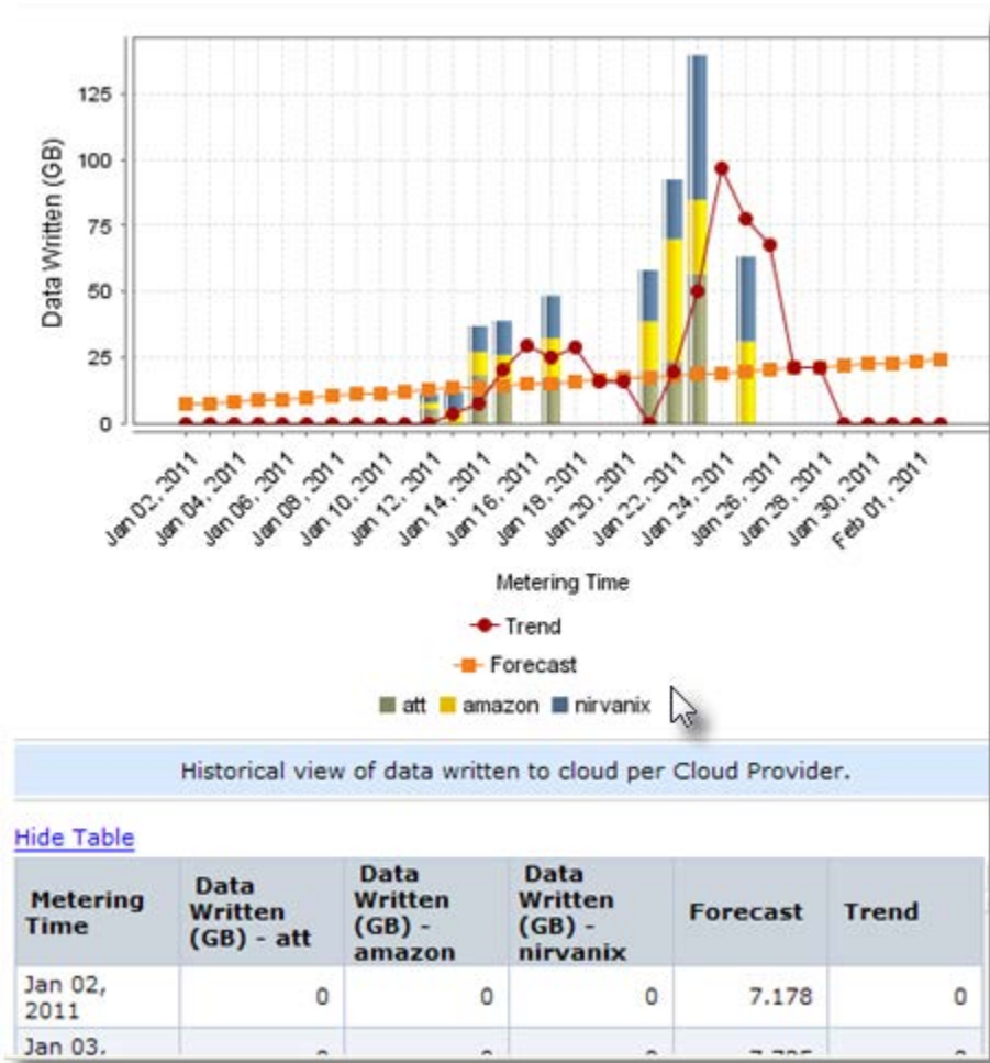
図 2-67 [クラウドの計測 (Cloud Metering)]レポート
