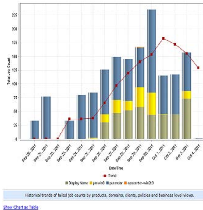
図 2-36 [失敗したジョブ数 (Failed Job Count)]レポート
