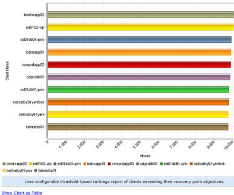
図 2-58 [Recovery Point Objective (RPO)]レポート
