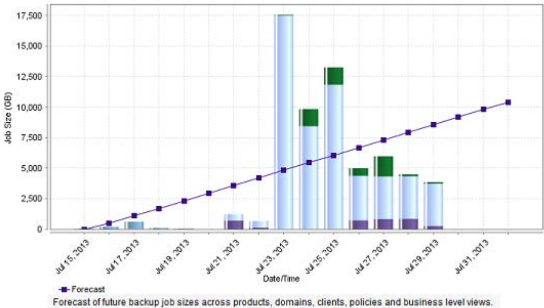
図 2-30 [ジョブのサイズ - 予測 (Job Size - Forecast)]レポート ([履歴 (Historical)])
