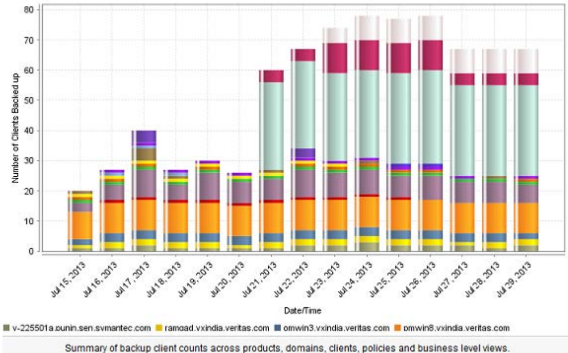
図 2-18 [クライアント数 (Client Count)]レポート ([履歴 (Historical)])
