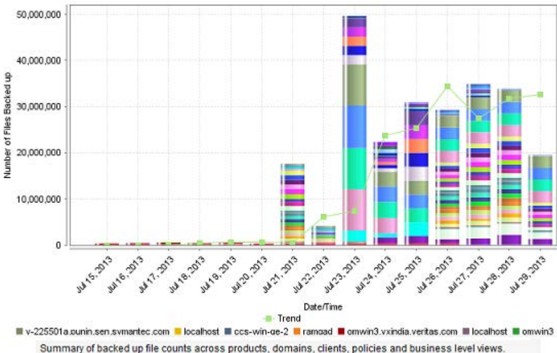
図 2-24 [ファイル数 (File Count)] レポート ([履歴 (Historical)])
