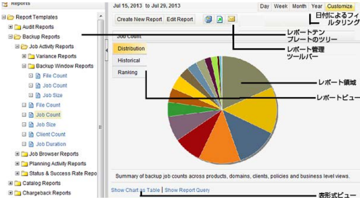
図 1-1 レポートテンプレート
