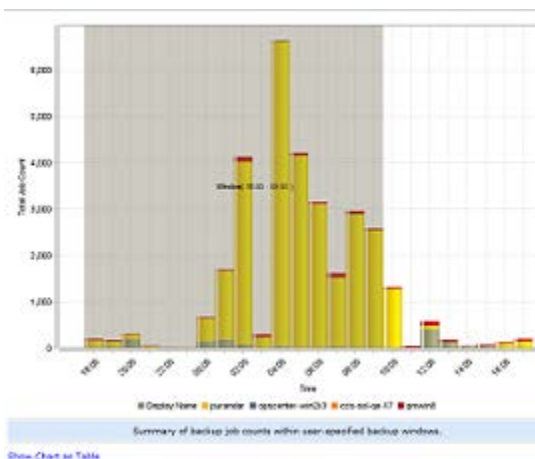
図 2-9 [ジョブ数 (Job Count)]レポート
