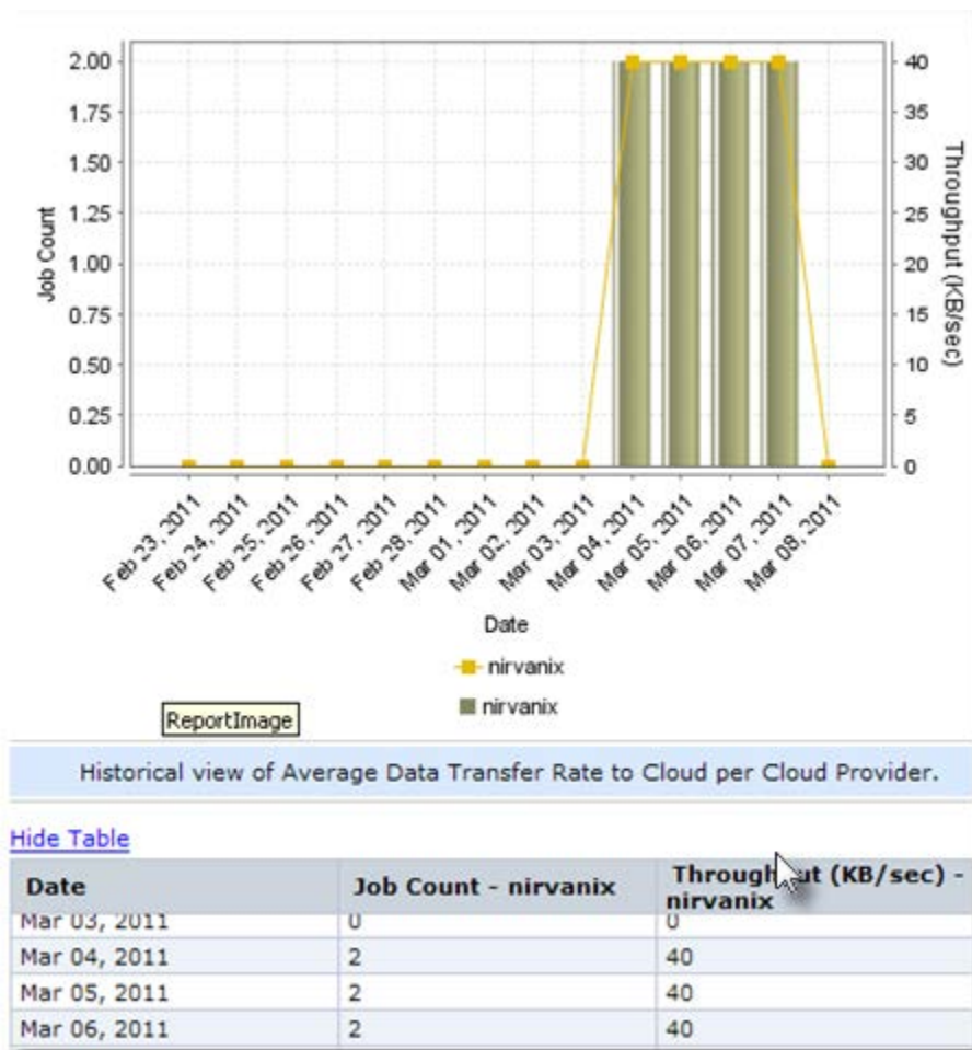
図 2-68 [平均データ転送率 (Average Data Transfer Rate)] レポート
