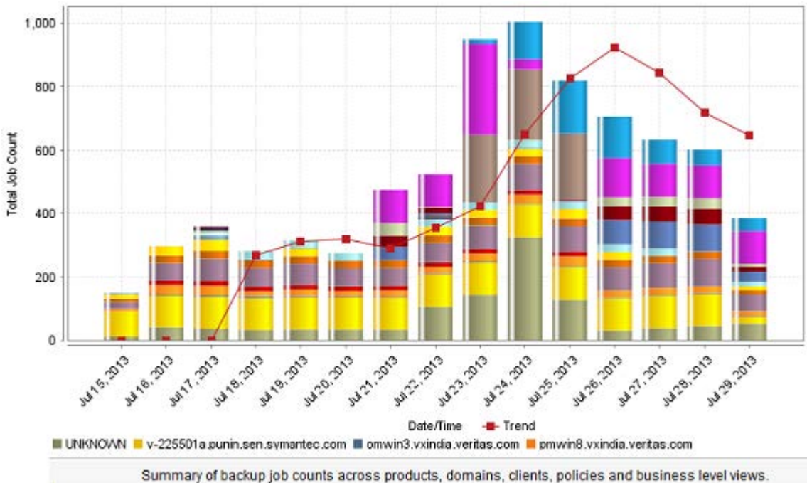
図 2-10 [ジョブ数 (Job Count)]レポート ([履歴 (Historical)])
