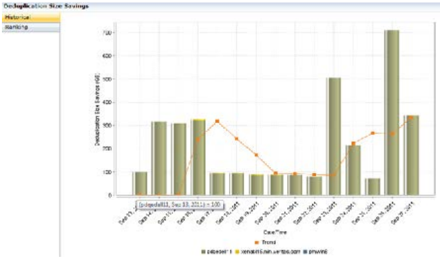
図 2-4 [サイズの重複排除による削減 (Deduplication Size Savings)]レポート ([履歴 (Historical)])
