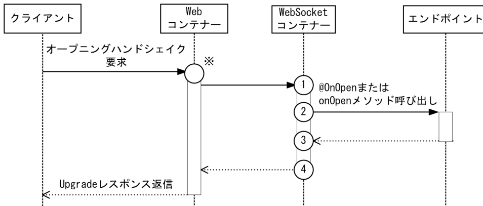
図 10-32 WebSocket のトレース取得ポイント（オープニングハンドシェイク要求受信時）
