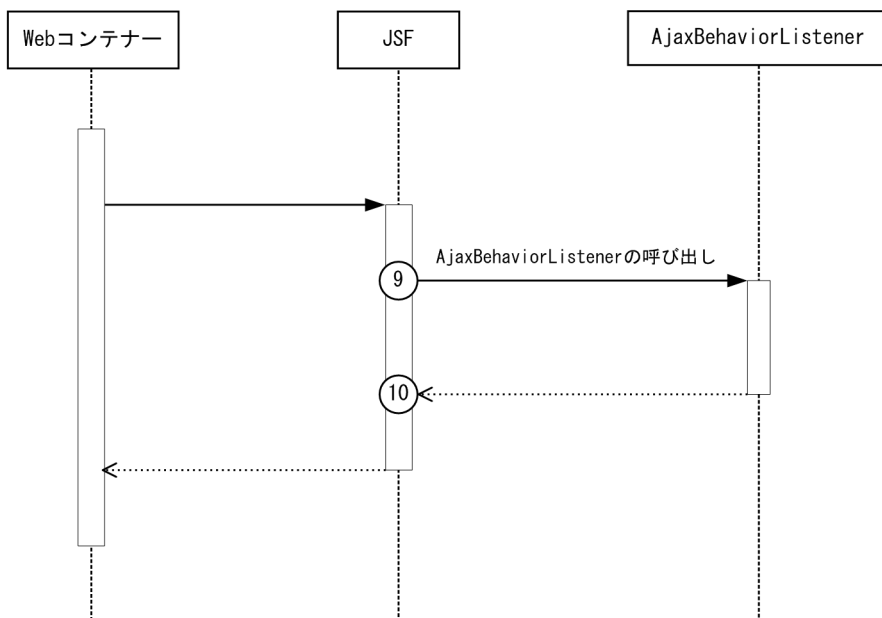
図 10-16 JSF のトレース取得ポイント (AjaxBehaviorListener が呼び出される場合)
