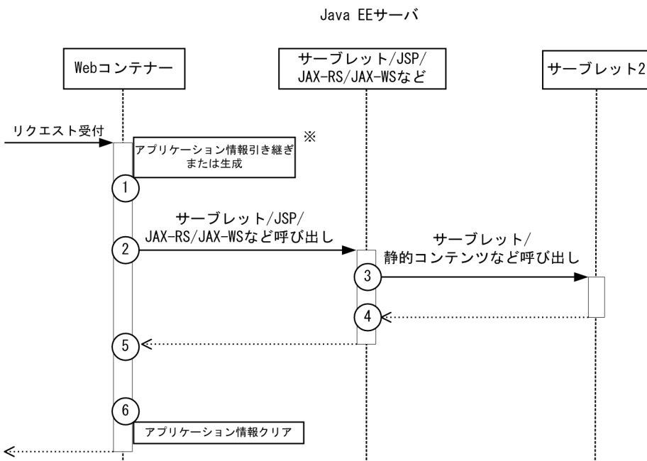
図 10-1 Web コンテナのトレース取得ポイント（同期処理の場合）
