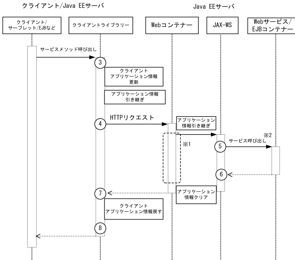
図 10-25 JAX-WS のトレース取得ポイント (request-response オペレーション (同期) の場合)
