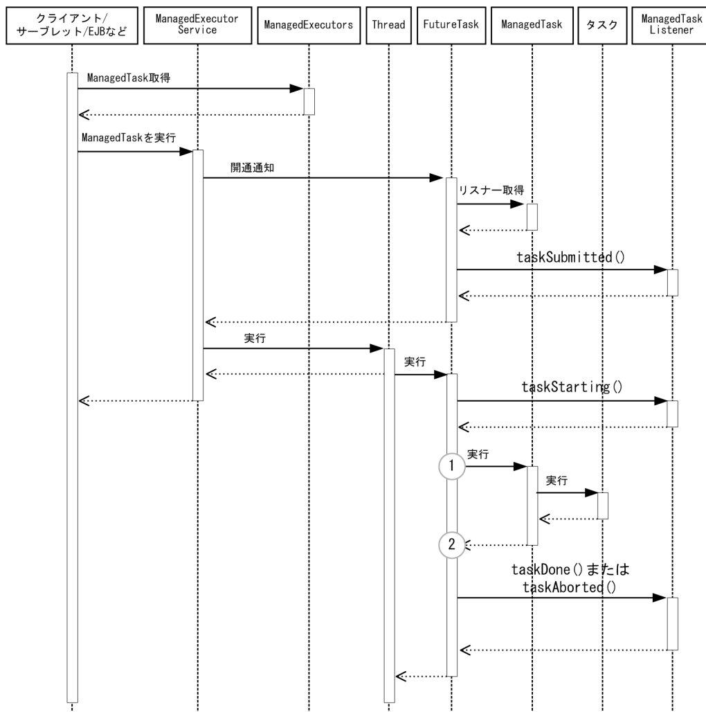
図 10-30 Concurrency Utilities のトレース取得ポイント（Java EE の ExecutorService 上で ManagedTask を実行した場合）
