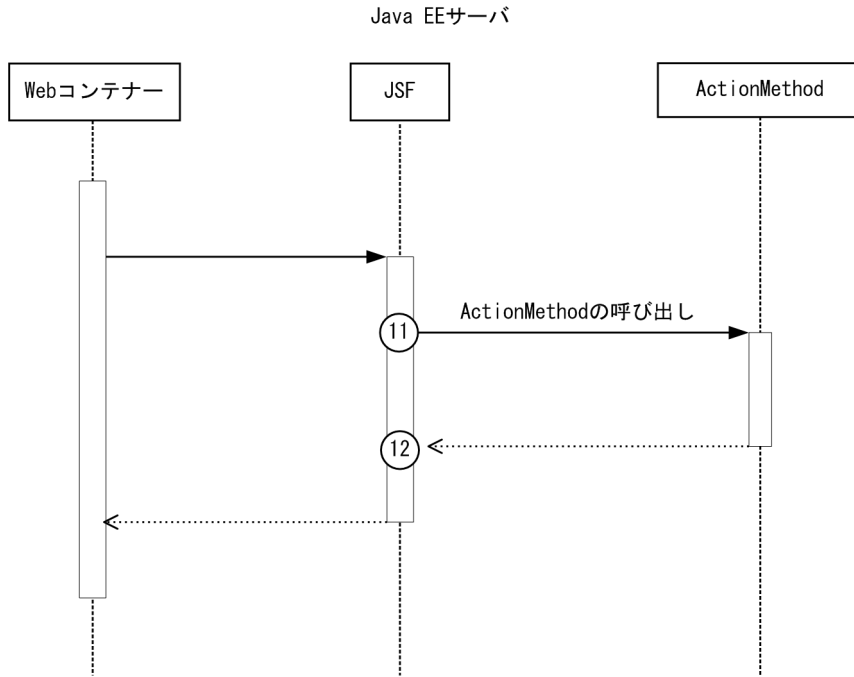
図 10-17 JSF のトレース取得ポイント (ActionMethod が呼び出される場合)
