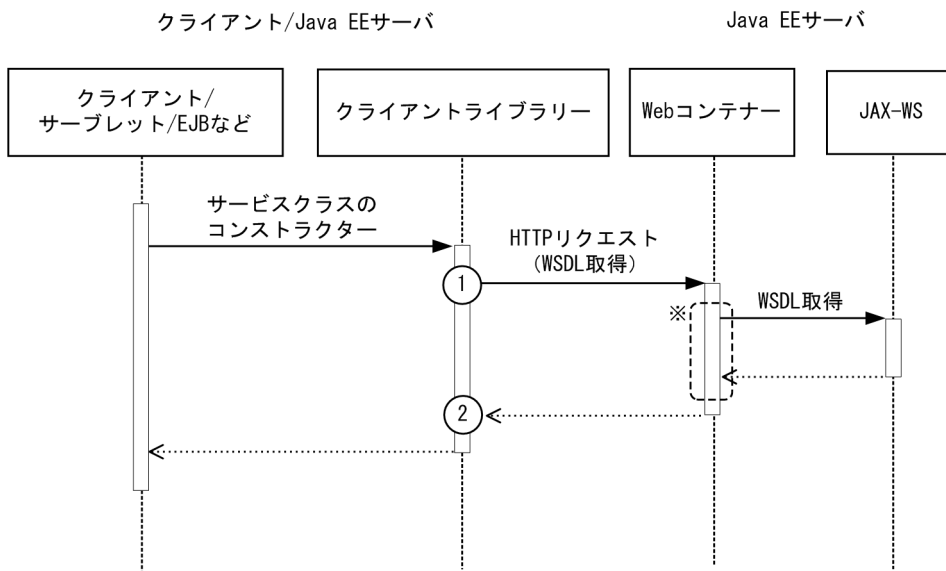
図 10-23 JAX-WS のトレース取得ポイント（リモート WSDL 取得の場合）
