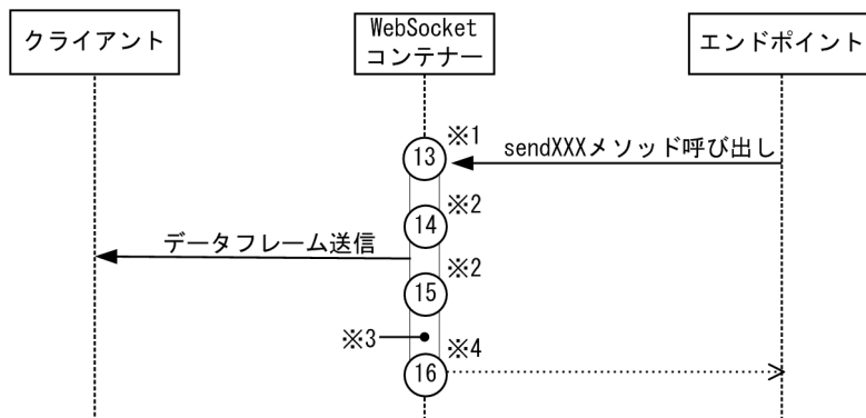
図 10-35 WebSocket のトレース取得ポイント（データ送信時）
