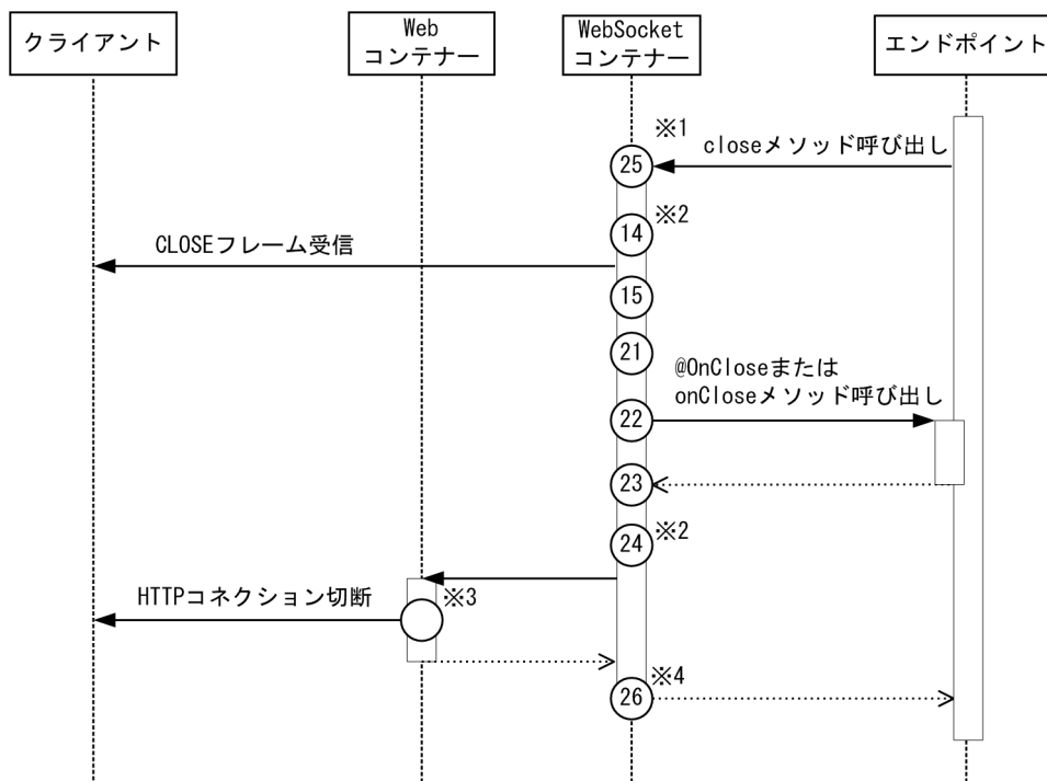
図 10-40 WebSocket のトレース取得ポイント（クロー징ハンドシェイク要求送信時）
