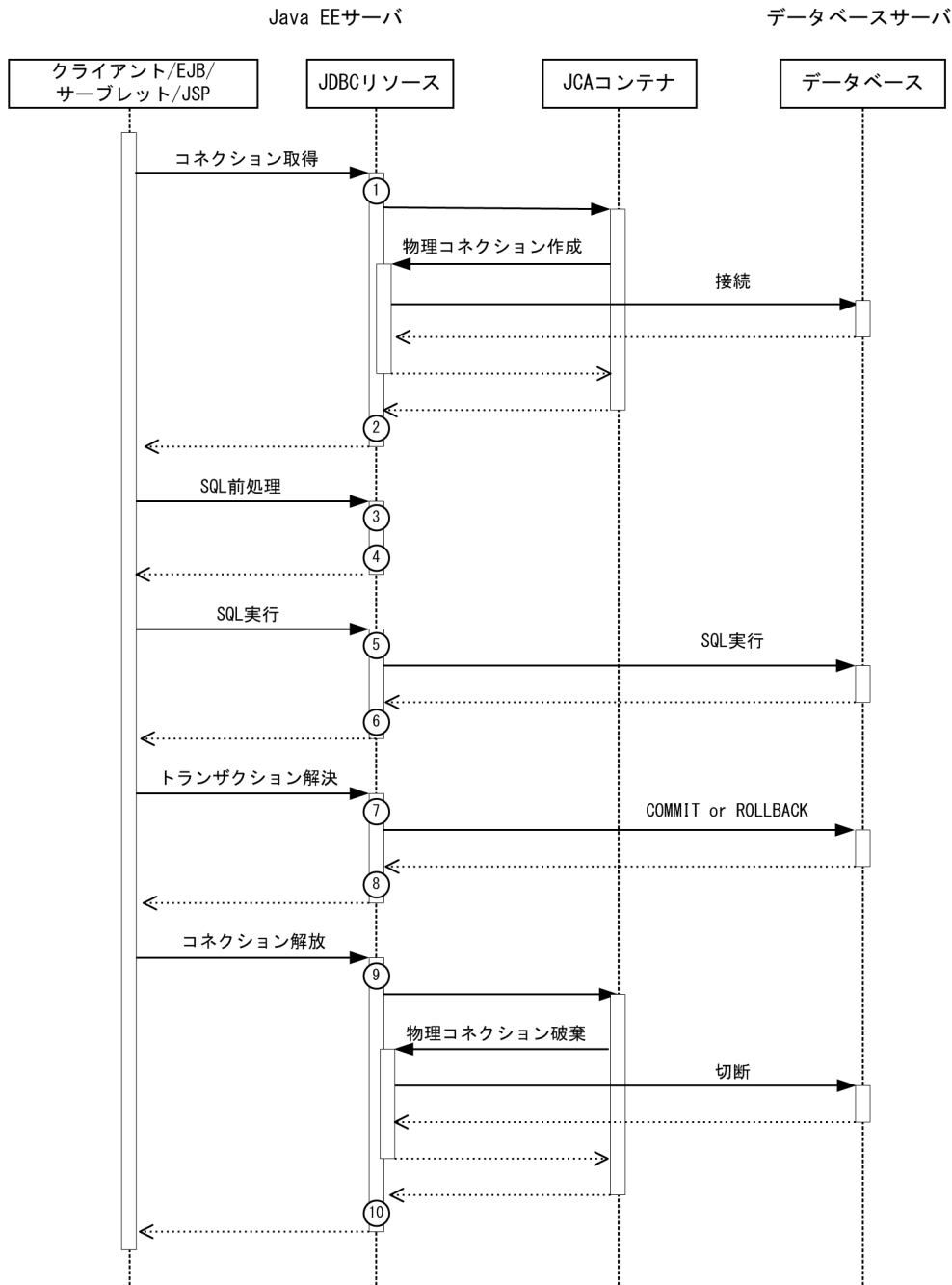
図 10-11 JDBC のトレース取得ポイント
