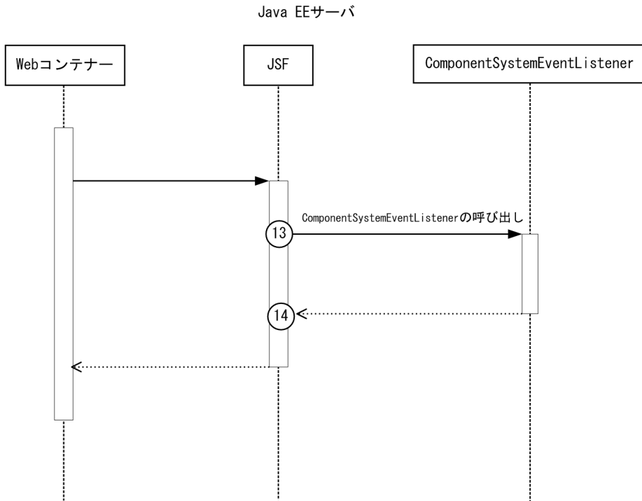
図 10-18 JSF のトレース取得ポイント（ComponentSystemEventListener が呼び出される場合）
