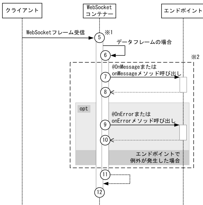
図 10-33 WebSocket のトレース取得ポイント（メッセージ（データフレーム）受信時）
