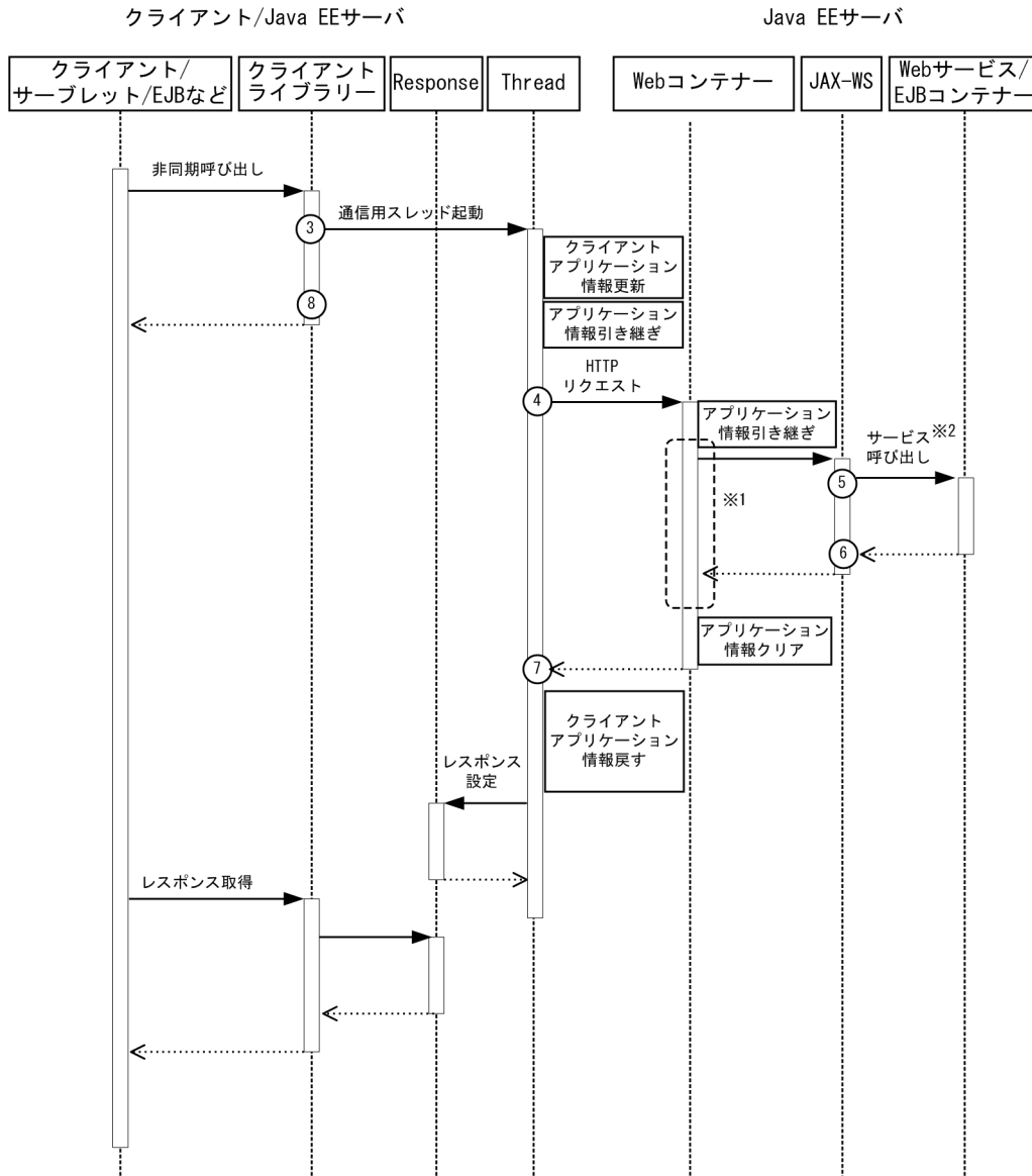
図 10-27 JAX-WS のトレース取得ポイント (request-response オペレーション (非同期) の場合)
