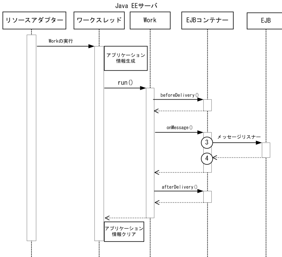
図 10-4 Message Driven Bean のトレース取得ポイント
