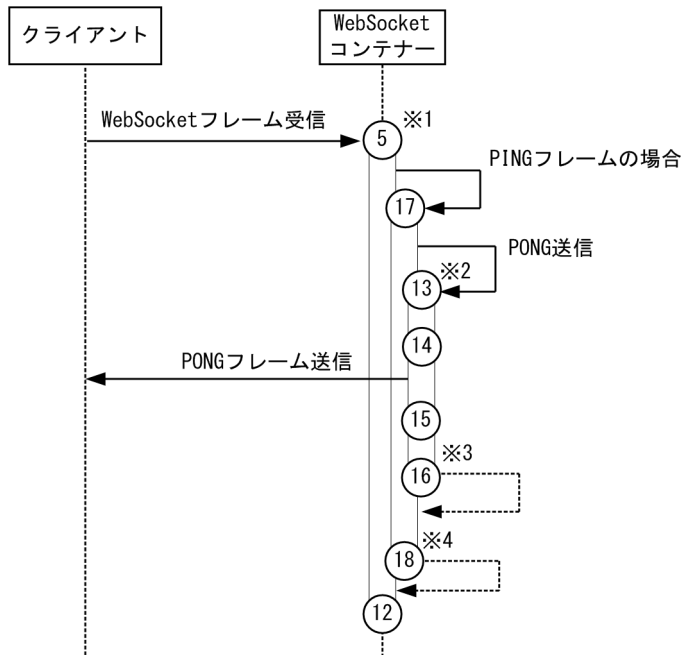
図 10-36 WebSocket のトレース取得ポイント (PING 受信時)
