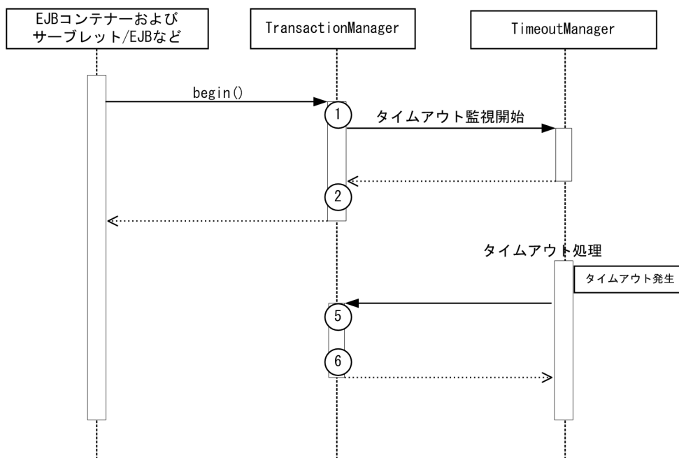
図 10-10 JTA のトレース取得ポイント（トランザクションがタイムアウトする場合）
