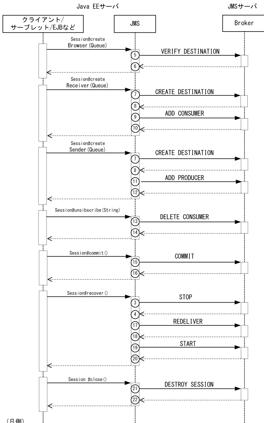
図 10-20 JMS のトレース取得ポイント (Session オブジェクト操作の場合)
