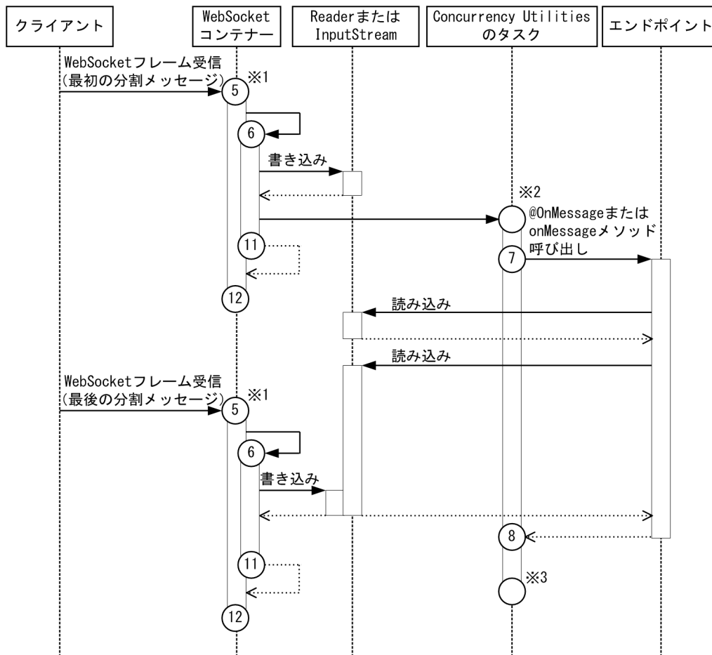
図 10-34 WebSocket のトレース取得ポイント (Reader または InputStream 型の引数を持つメッセージハンドラによる分割メッセージ受信時)
