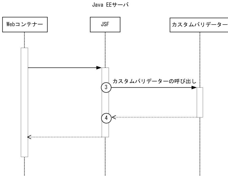
図 10-13 JSF のトレース取得ポイント（カスタムバリデーターが呼び出される場合）
