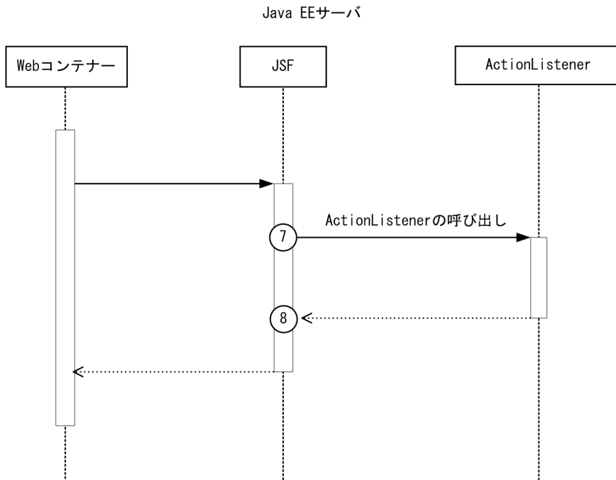
図 10-15 JSF のトレース取得ポイント (ActionListener が呼び出される場合)
