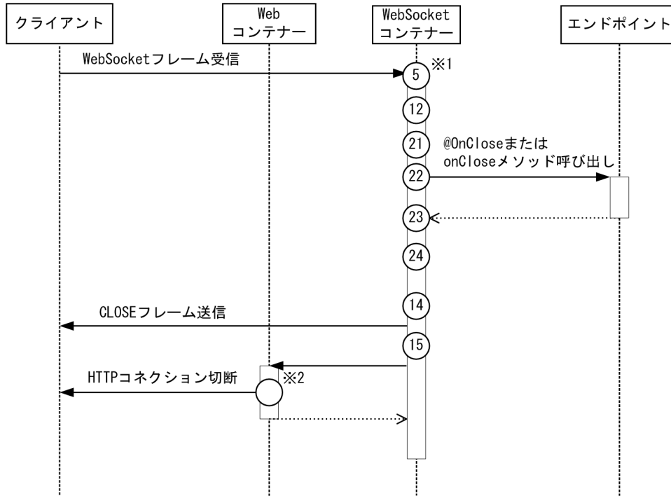
図 10-39 WebSocket のトレース取得ポイント（クローリングハンドシェイク要求受信時（ペイロードデータなし））
