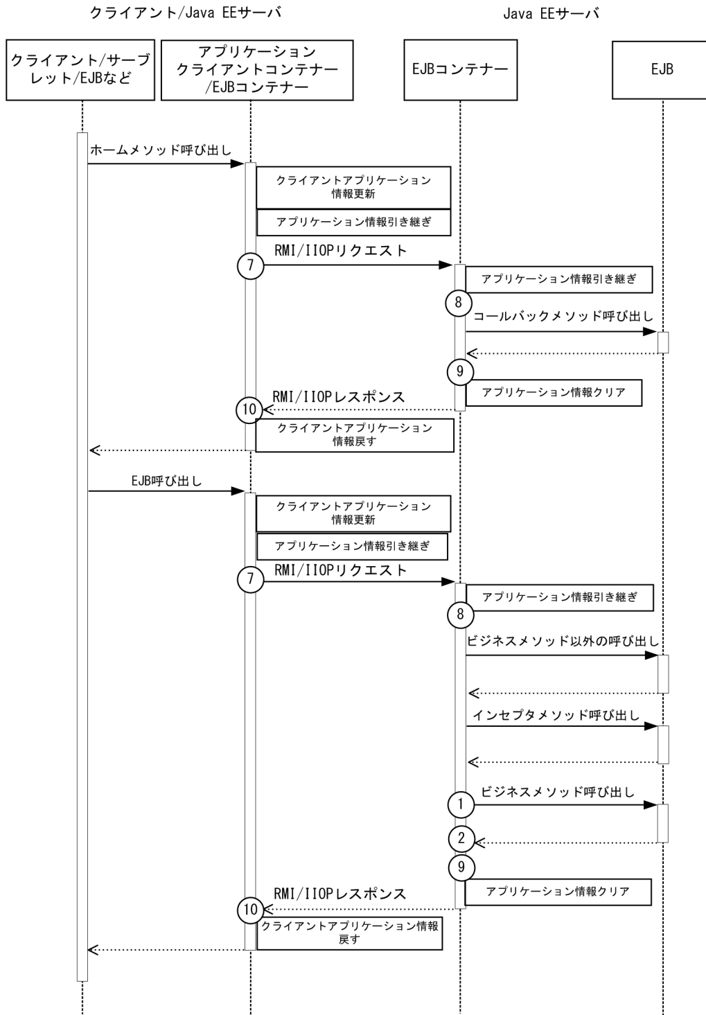
図 10-6 Session Bean および Entity Bean (リモート呼び出し) のトレース取得ポイント
