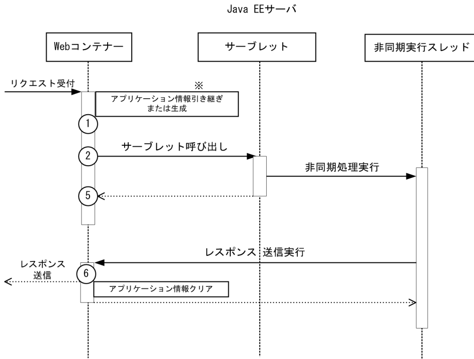
図 10-2 Web コンテナの取得ポイント（非同期処理の場合）
