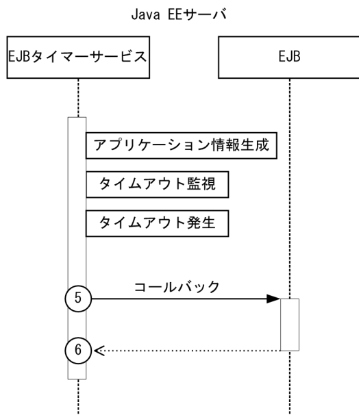
図 10-5 Timer Service のトレース取得ポイント
