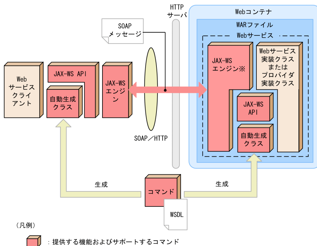
図 1-1 SOAP Web サービスの構成（POJO の Web サービス）
