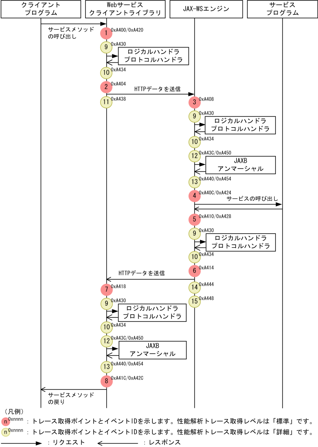
図 39-8 POJO の Web サービス呼び出し時のトレース取得ポイント（request-response オペレーション）
