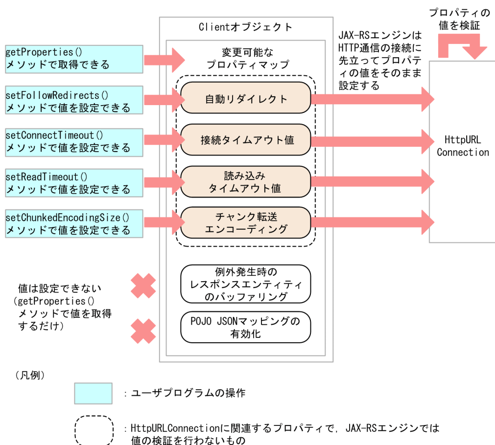
図 11-3 変更可能なプロパティマップの構造
