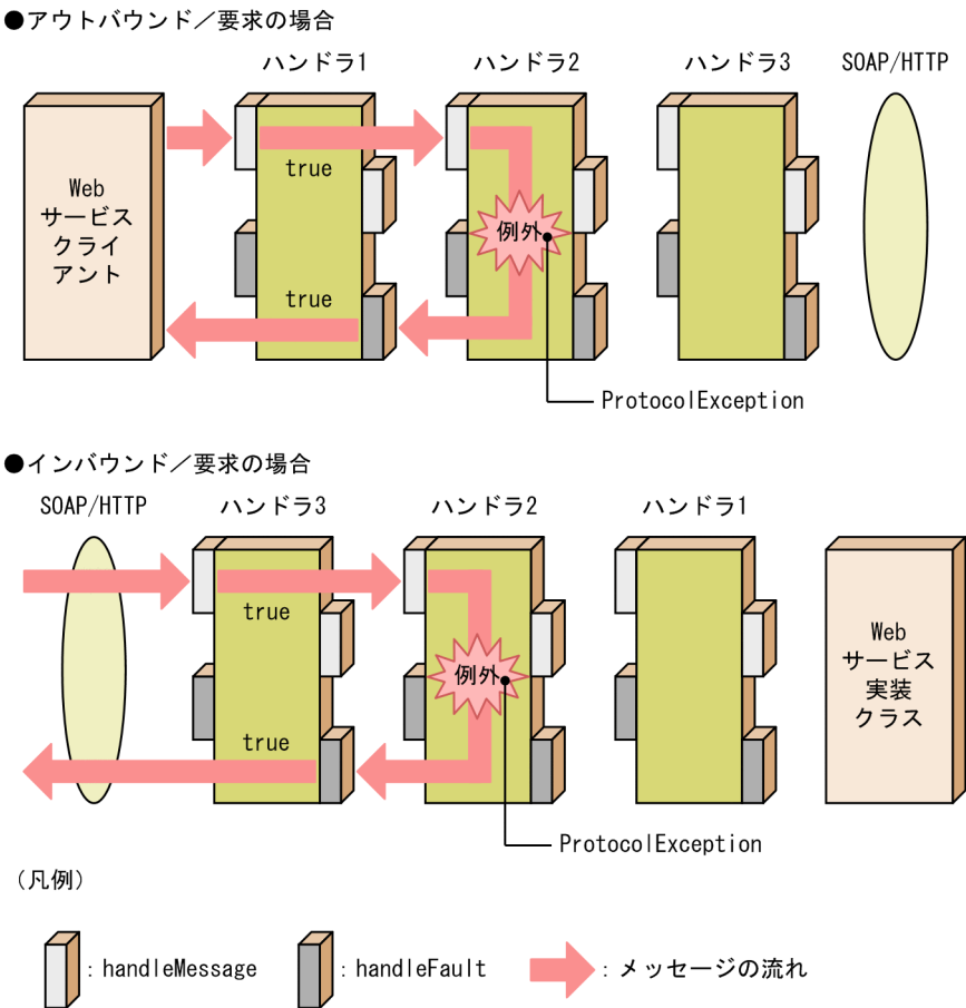
図 36-8 handleMessage で ProtocolException をスローする場合の処理 (要求)
