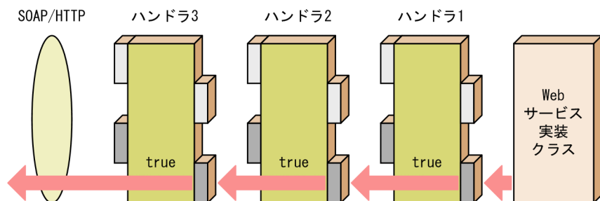
図 36-12 handleFault で true を返す場合の処理（応答）
