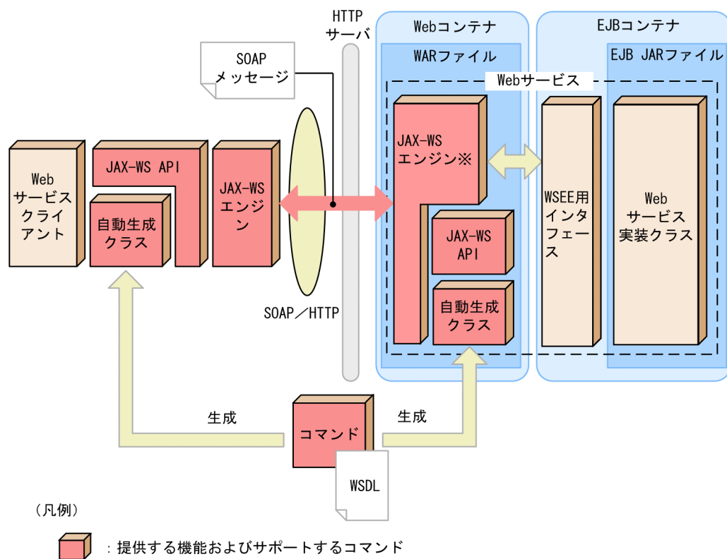
図 1-2 SOAP Web サービスの構成 (EJB の Web サービス)
