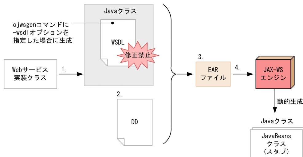
図 2-4 SEI を起点とした Web サービスの開発の流れ (hwsген コマンドを使用する場合)
