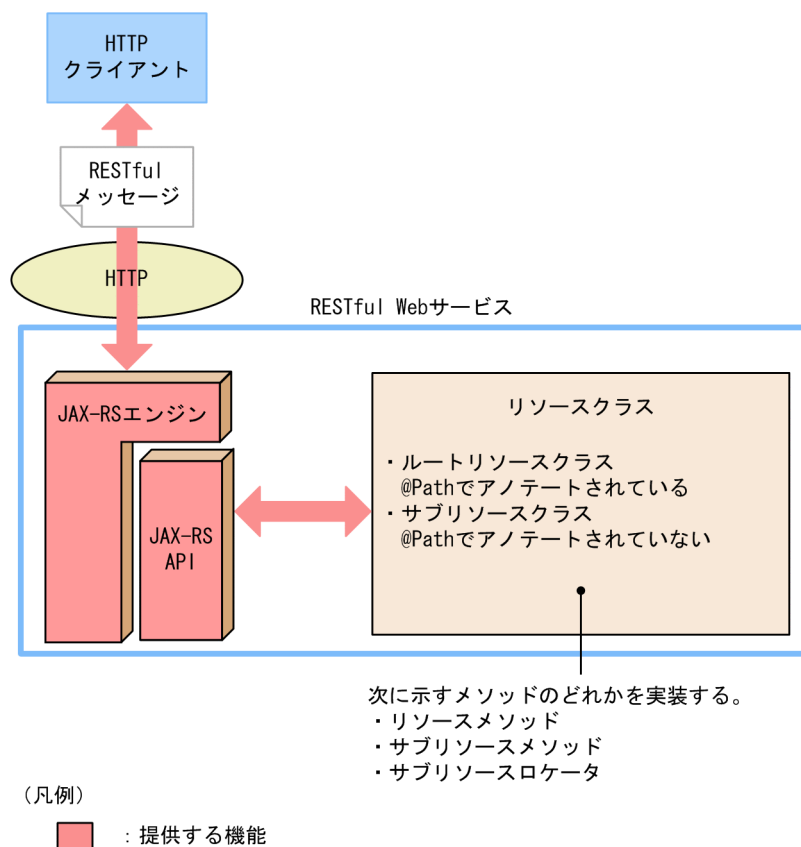
図 1-7 RESTful Web サービス (Web リソース)
