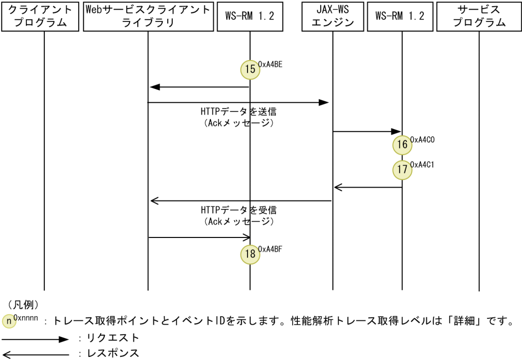
図 39-13 Ack メッセージのトレース取得ポイント
