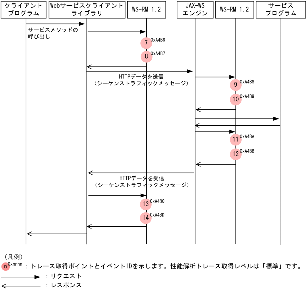
図 39-12 シーケンストラフィックメッセージのトレース取得ポイント
