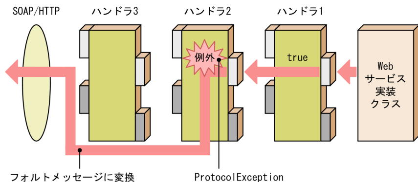
図 36-9 handleMessage で ProtocolException をスローする場合の処理（応答）
