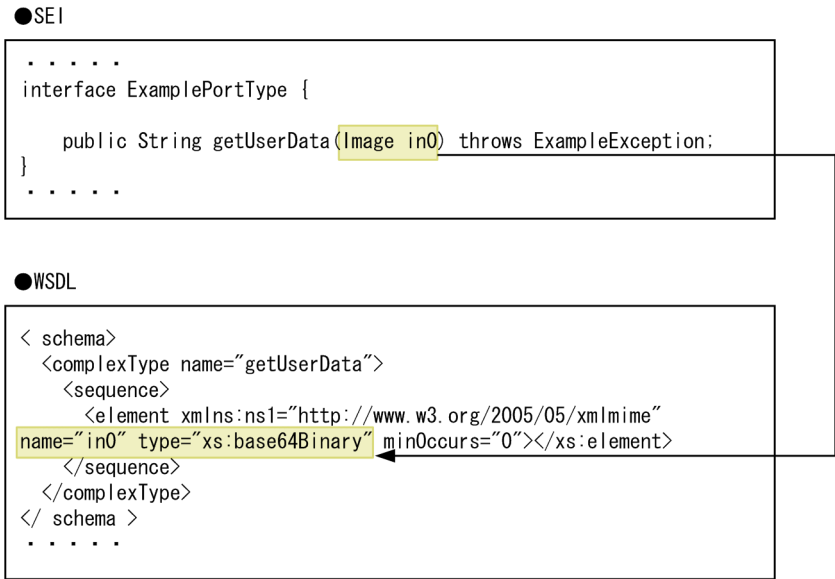
図 16-20 javax.xml.bind.annotation.XmlMimeType アノテーションを使用しない例
