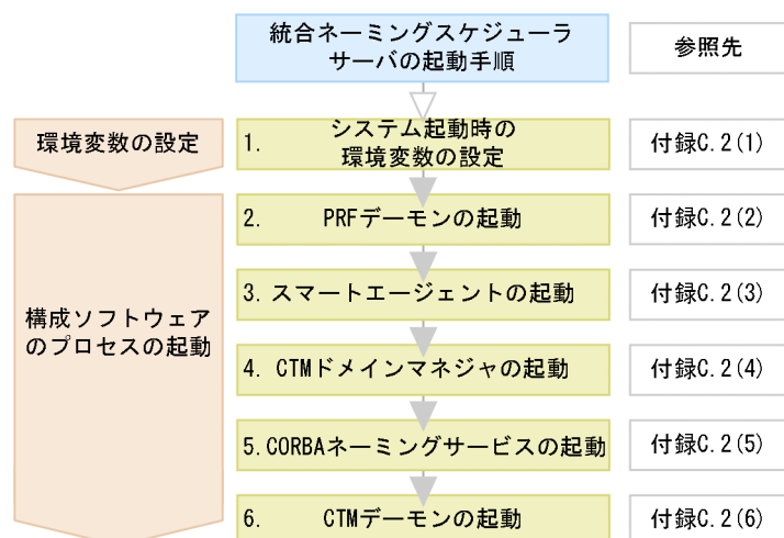
図 C-2 統合ネーミングスケジューラサーバの起動の流れ (Windows の場合)
