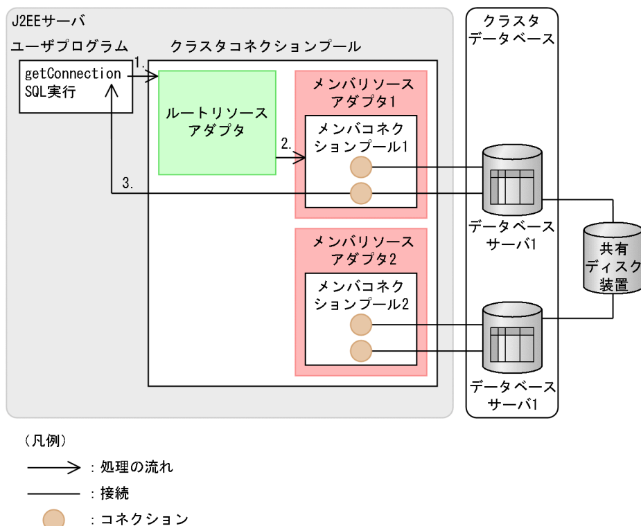
図 19-3 コネクション取得時の処理の流れ
