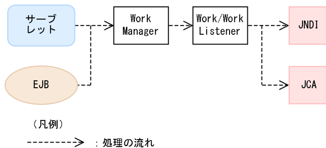
図 20-2 WorkManager を使用した非同期スレッド処理の流れ
