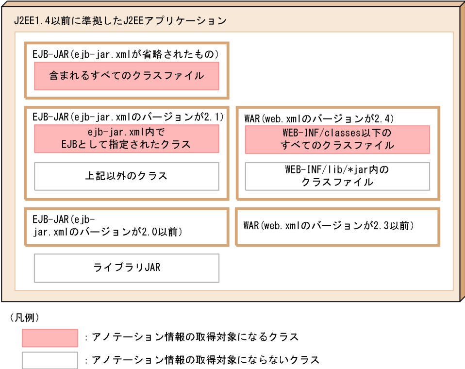
図 18-1 アノテーション情報を読み込むためにロードするクラス
