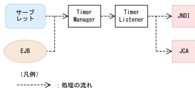
図 20-1 TimerManager を使用した非同期タイマ処理の流れ
