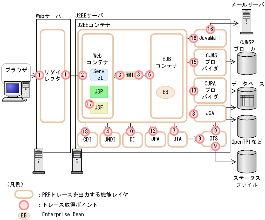
図 14-2 機能レイヤとトレース取得ポイント (Web クライアント構成の場合)
