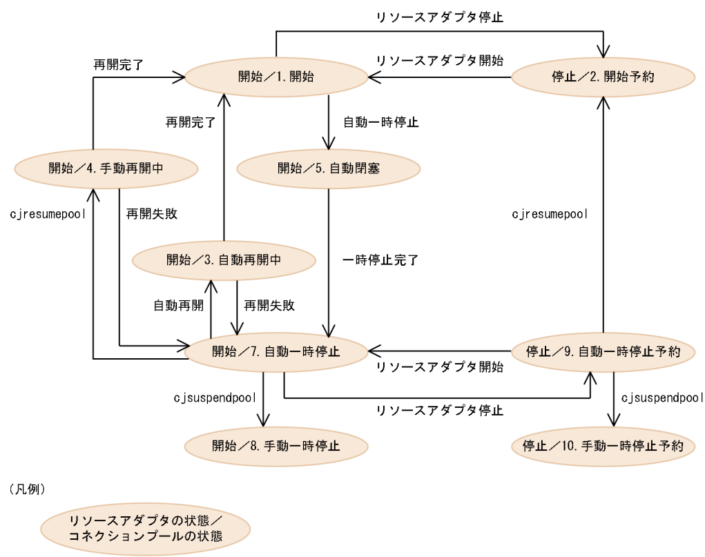
図 19-5 メンバコネクションプールの状態遷移（自動で一時停止が実行される場合）
