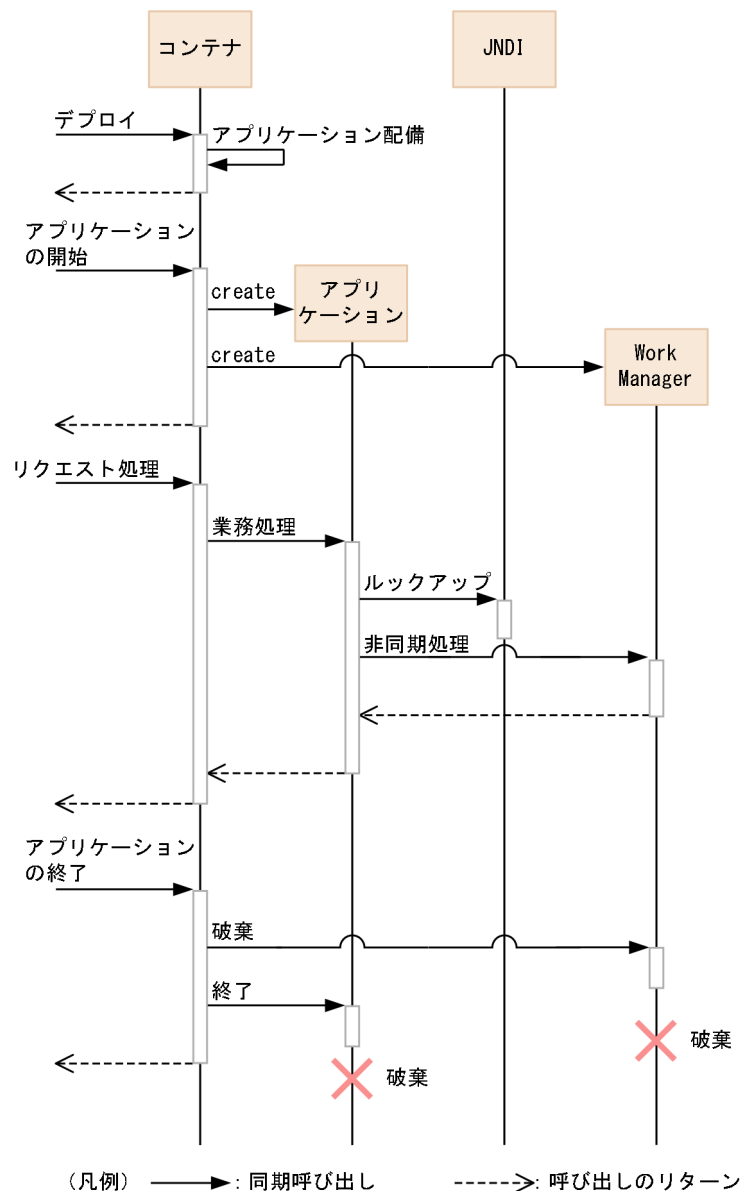
図 20-7 WorkManager のライフサイクル
