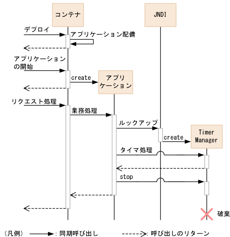
図 20-5 TimerManager のライフサイクル
