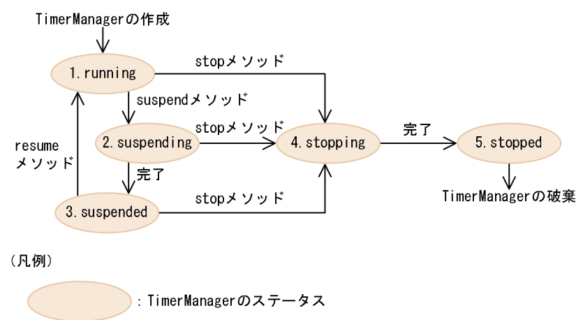
図 20-6 TimerManager のステータス遷移
