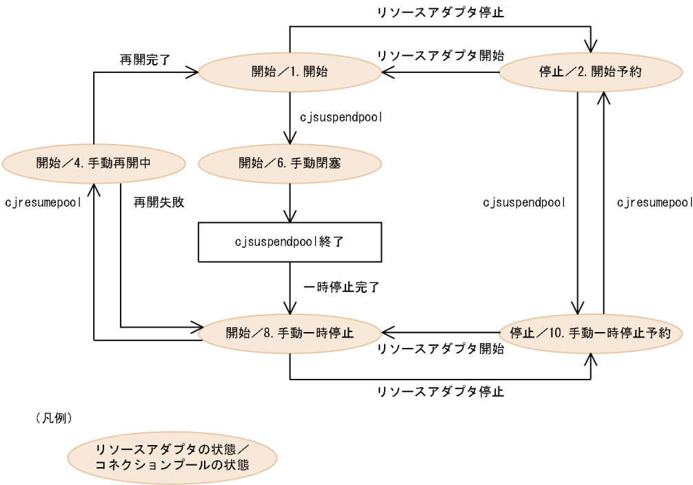
図 19-4 メンバコネクションプールの状態遷移（手動で一時停止を実行する場合）
