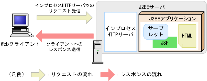
図 6-7 タイムアウトを設定できる通信（インプロセス HTTP サーバを使用する場合）
