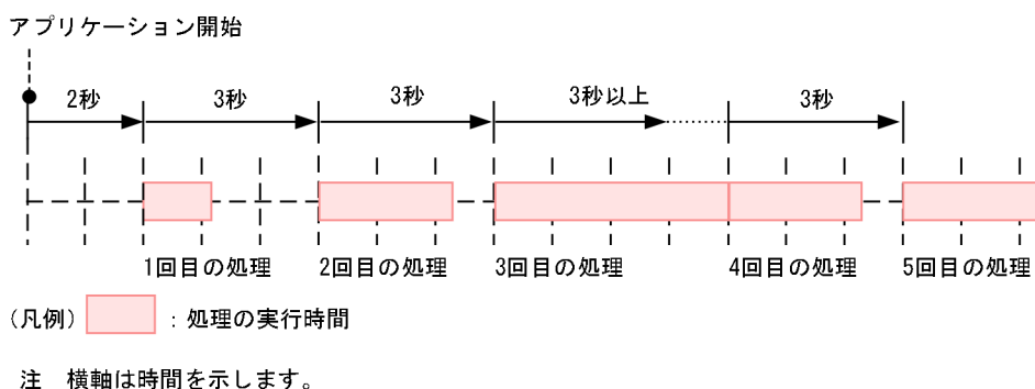
図 20-3 fixed-rate の処理のイメージ
