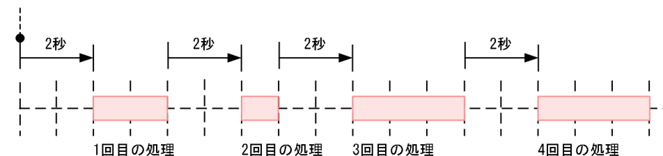
図 20-4 fixed-delay の処理のイメージ
