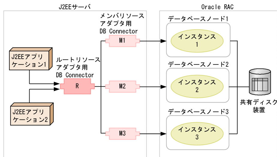
図 19-1 クラスタコネクションプール機能を使用した接続
