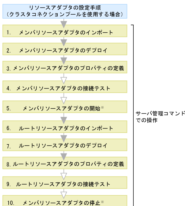
図 19-6 クラスタコネクションプールでのリソースアダプタの設定の流れ
