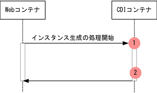
図 14-33 サーブレット・フィルタ・リスナと CDI を組み合わせて利用する場合のトレース取得ポイント
