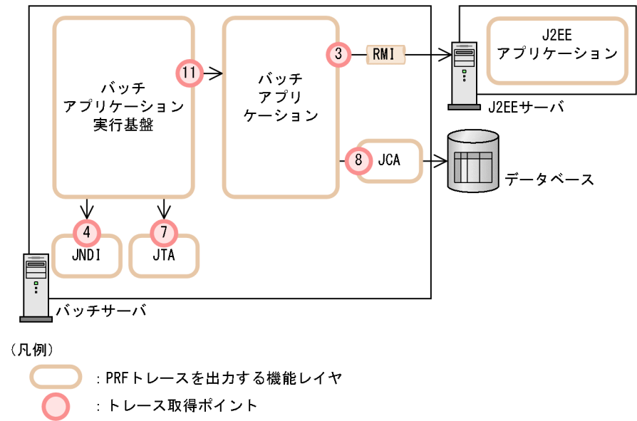
図 14-3 機能レイヤとトレース取得ポイント (バッチアプリケーションを実行するシステムの場合)
