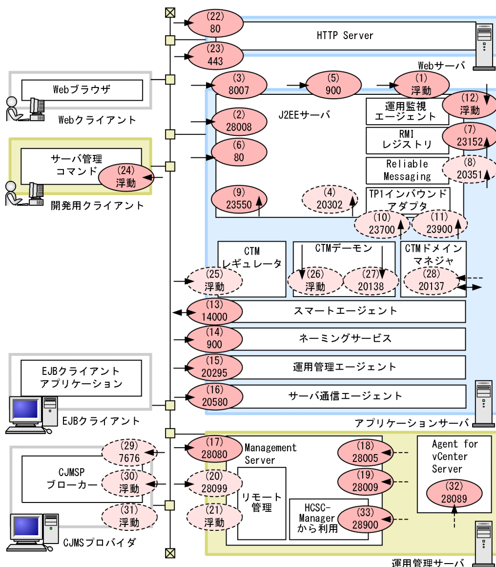
図 16-5 アプリケーションサーバが使用する TCP/UDP のポート番号
