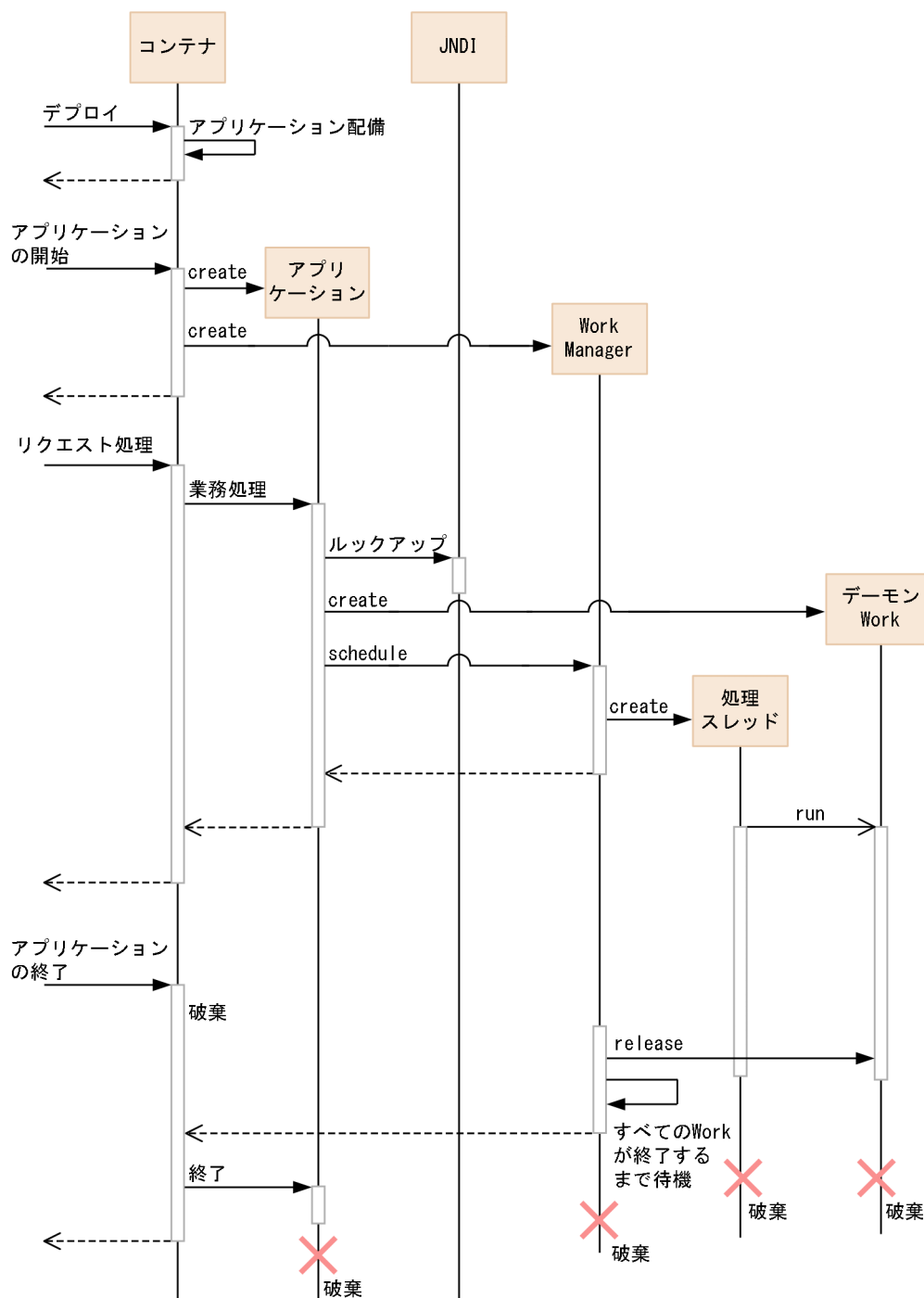
図 20-8 デーモン Work のライフサイクル
