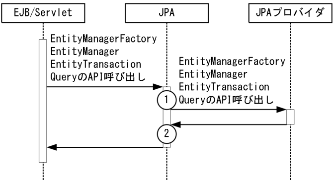
図 14-16 アプリケーション管理の永続化コンテキストを利用した場合のトレース取得ポイント
