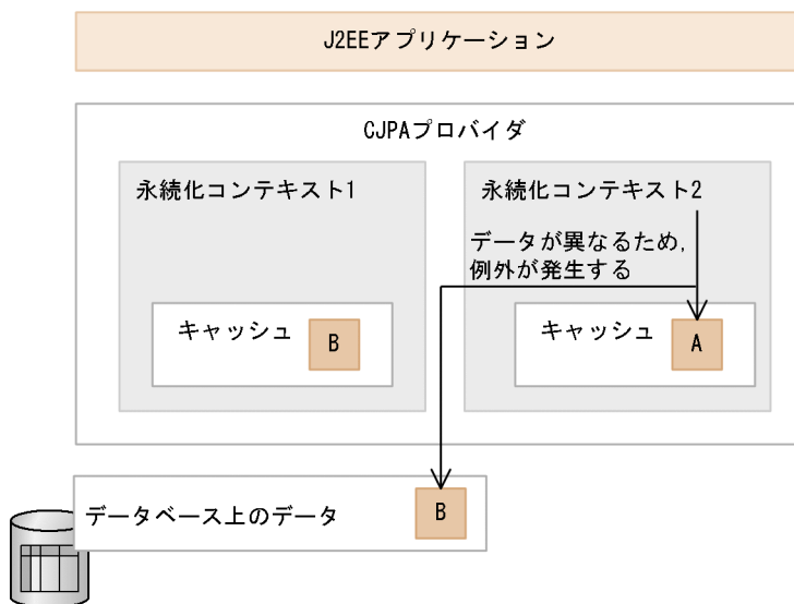
図 8-21 永続化コンテキスト 2 でのデータの変更
