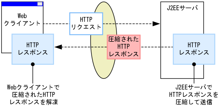
図 9-1 HTTP レスポンス圧縮機能の概要
