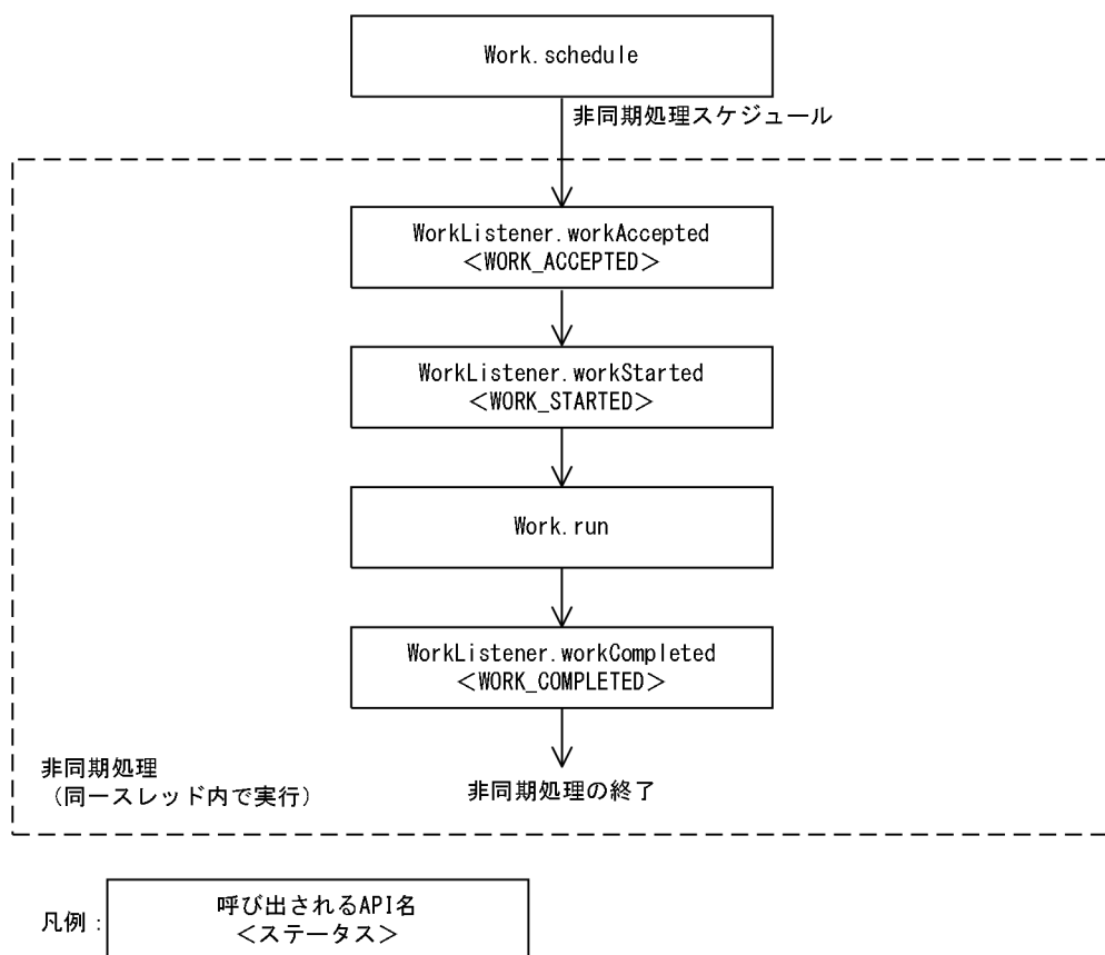
図 20-10 WorkListener インタフェースの API が呼び出される流れとステータスの遷移
