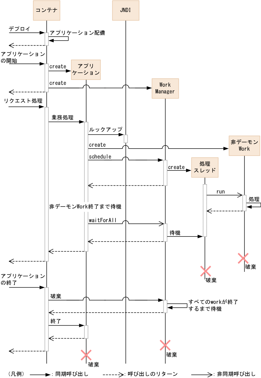
図 20-9 非デーモン Work のライフサイクル
