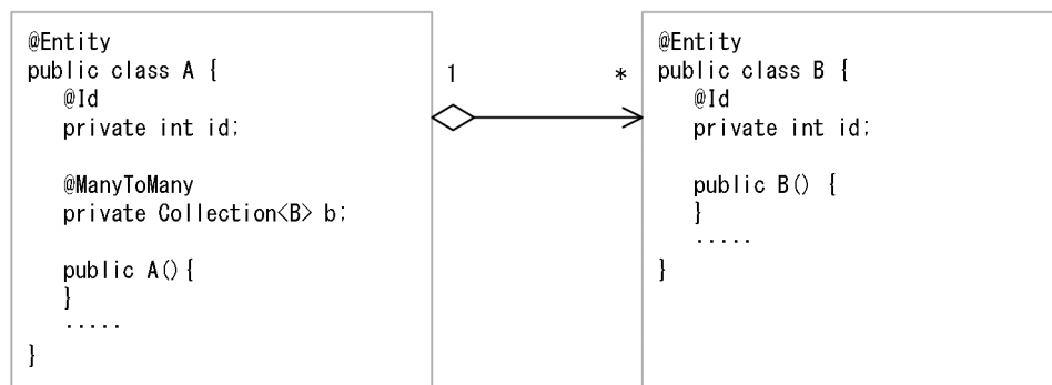
図 8-12 単方向 ManyToMany でのデフォルトマッピング
