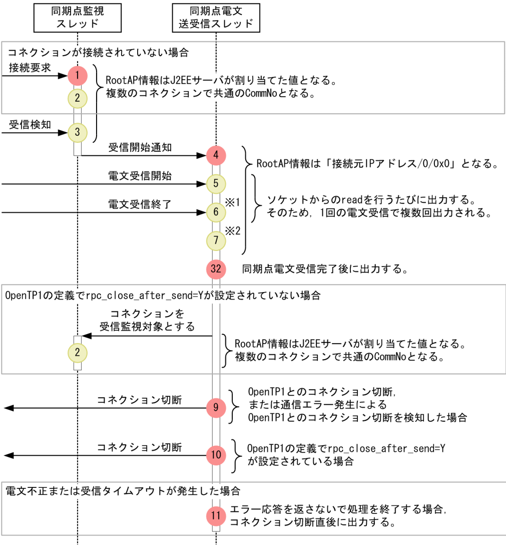
図 8-77 同期点処理の A 部分のトレース取得ポイント
