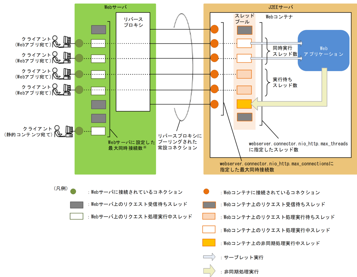
図 12-4 アプリケーションサーバ 11-70 のスレッド数制御の仕組み (Web サーバ連携の場合)
