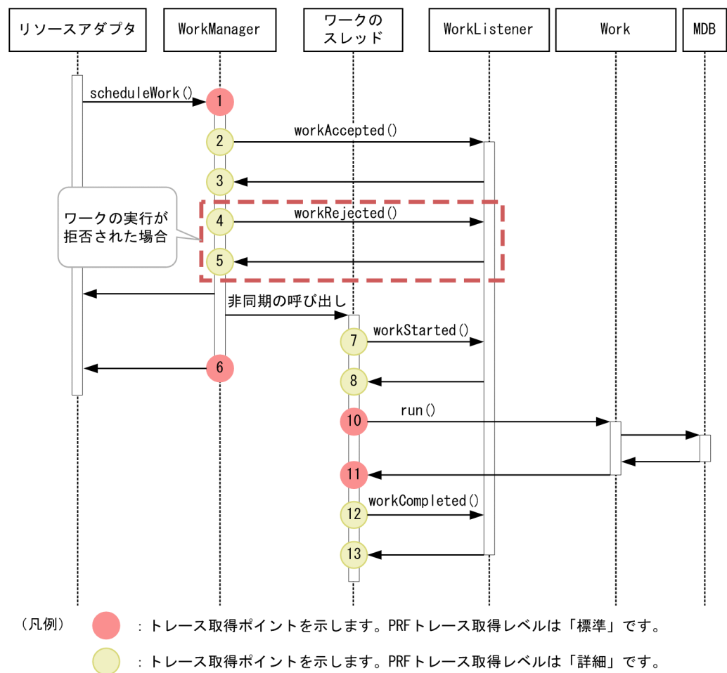
図 8-54 DB Connector, JCA コンテナでのトレース取得ポイントの詳細 (scheduleWork() 呼び出し時)
