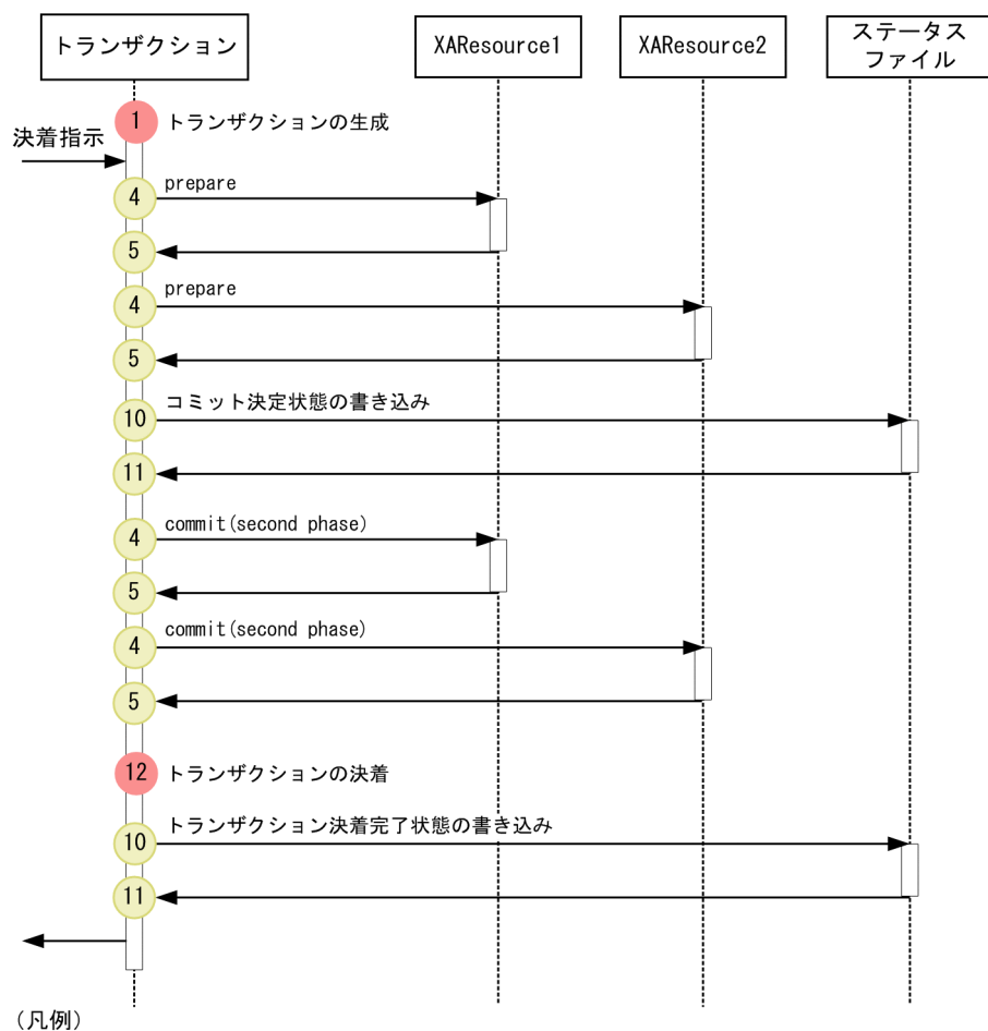
図 8-62 典型的な 2 フェーズコミットモデルでのトレース取得ポイント
