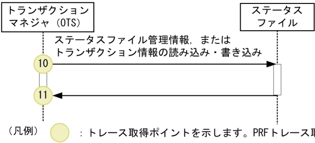
図 8-59 インプロセス OTS 初期化時のステータスファイルへの読み込み・書き込みに関連するトレース取得ポイント
