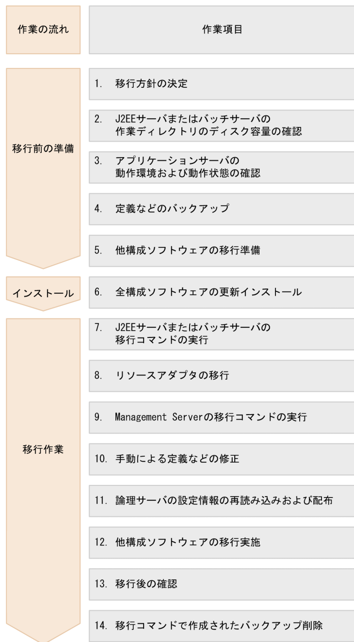
図 10-2 旧バージョンからアプリケーションサーバ 11-70 への移行作業（更新インストールの場合）
