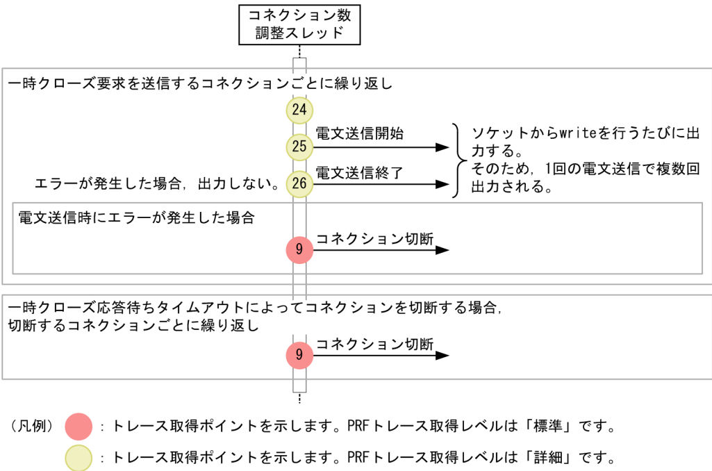
図 8-79 コネクション数調整スレッドのトレース取得ポイント
