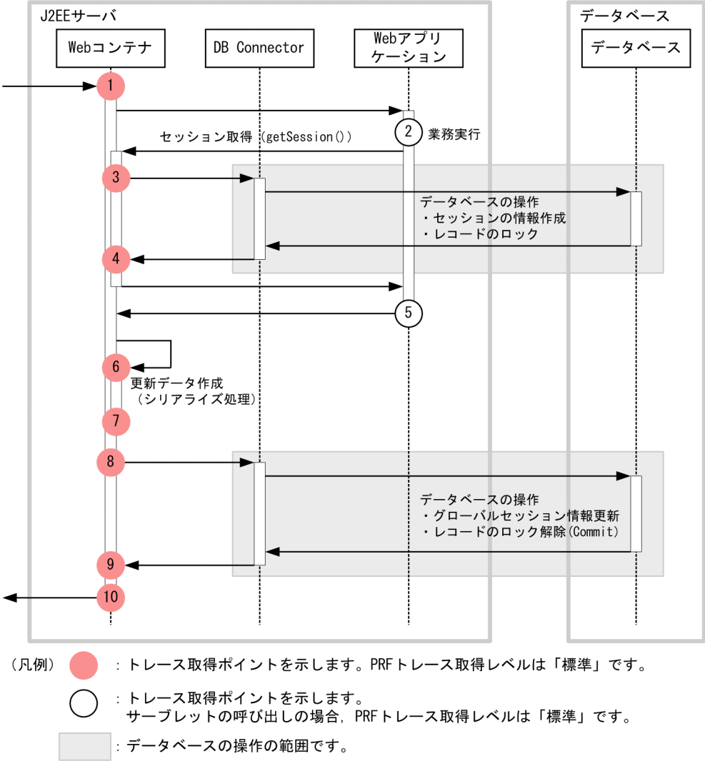
図 8-13 HTTP セッションを作成するリクエスト処理のトレース取得ポイント（データベースセッションフェイルオーバ機能）
