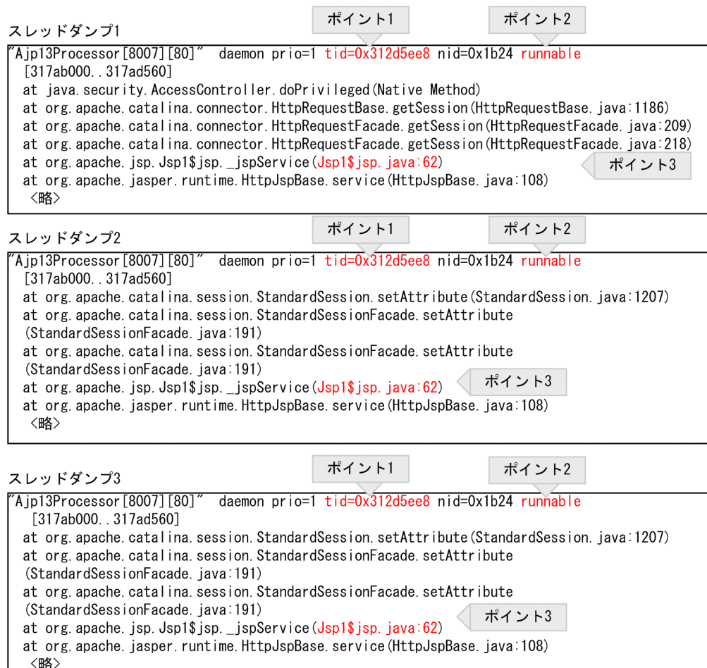
図 6-10 スレッドダンプ（無限ループ）の出力例
