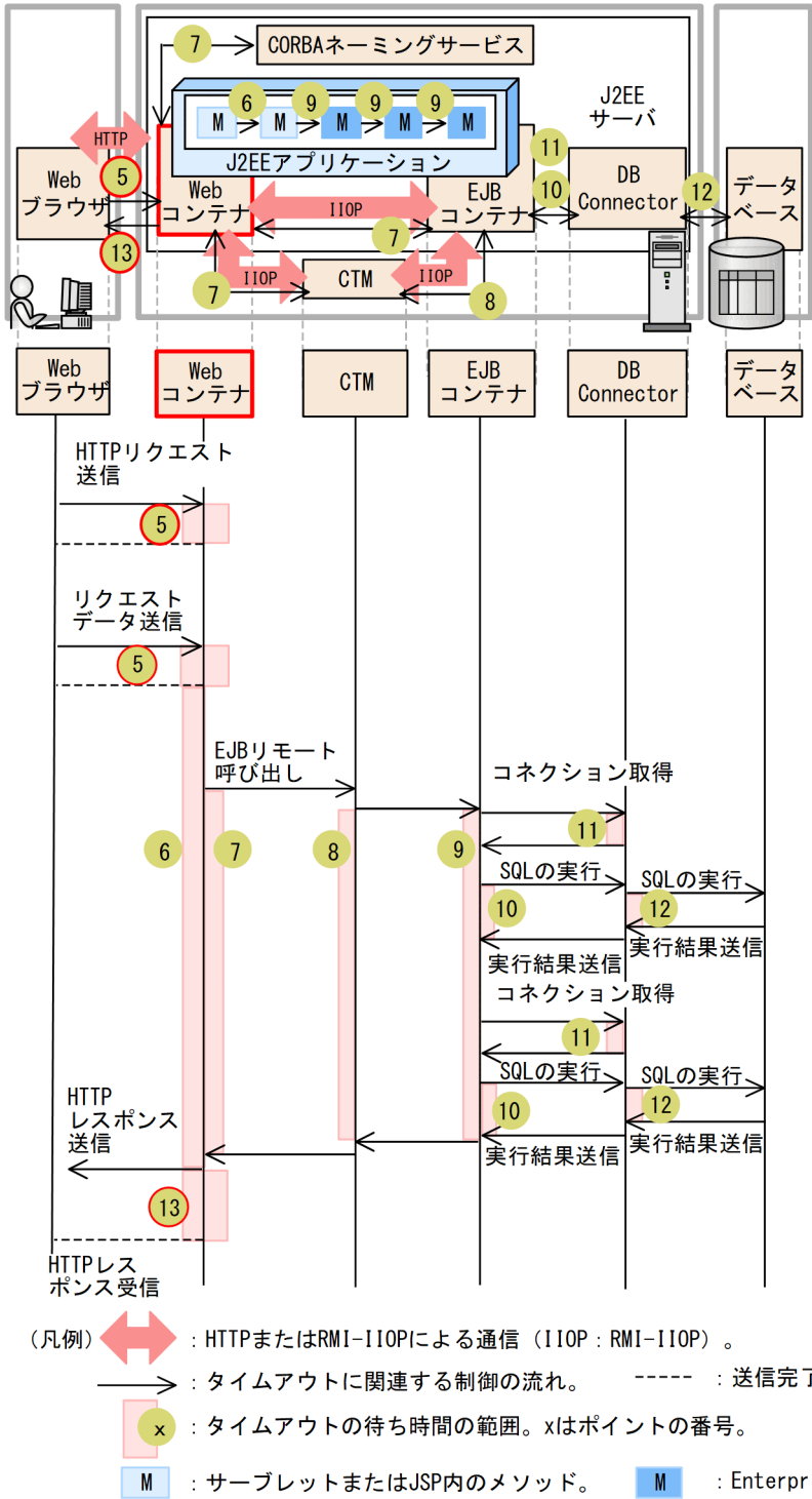
図 12-7 タイムアウトが設定できるポイント（インプロセス HTTP サーバの場合）
