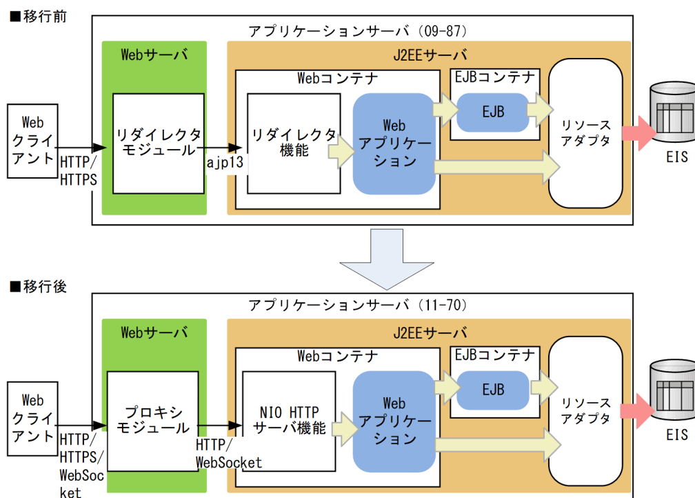
図 12-1 リダイレクタによる Web サーバ連携構成をアプリケーションサーバ 11-70 に移行する場合
