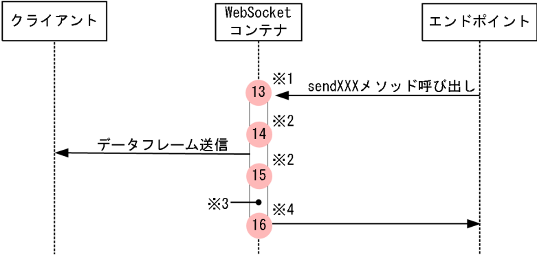
図 8-113 WebSocket のトレース取得ポイント（データ送信時）
