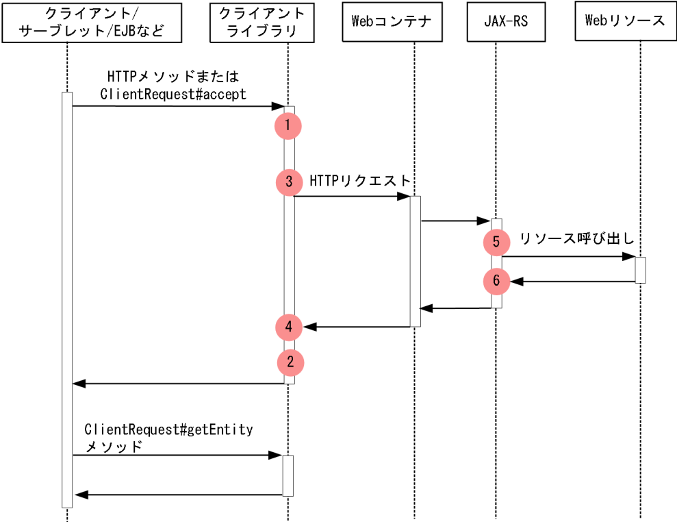
図 8-105 JAX-RS のトレース取得ポイント
