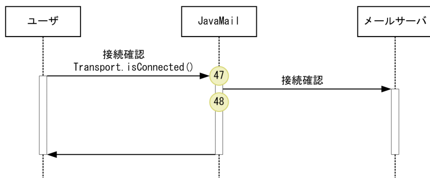
図 8-90 JavaMail のコネクション接続確認時のトレース取得ポイント
