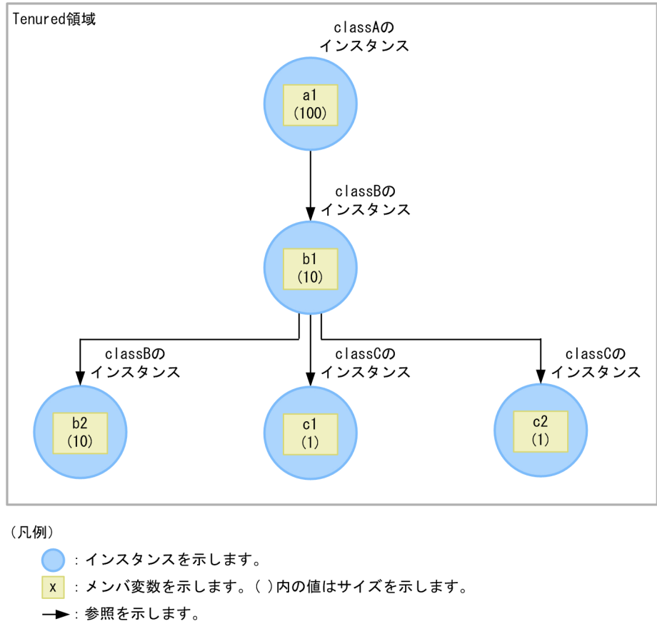
図 9-11 Tenured 領域内の不要なオブジェクトによる参照関係の例
