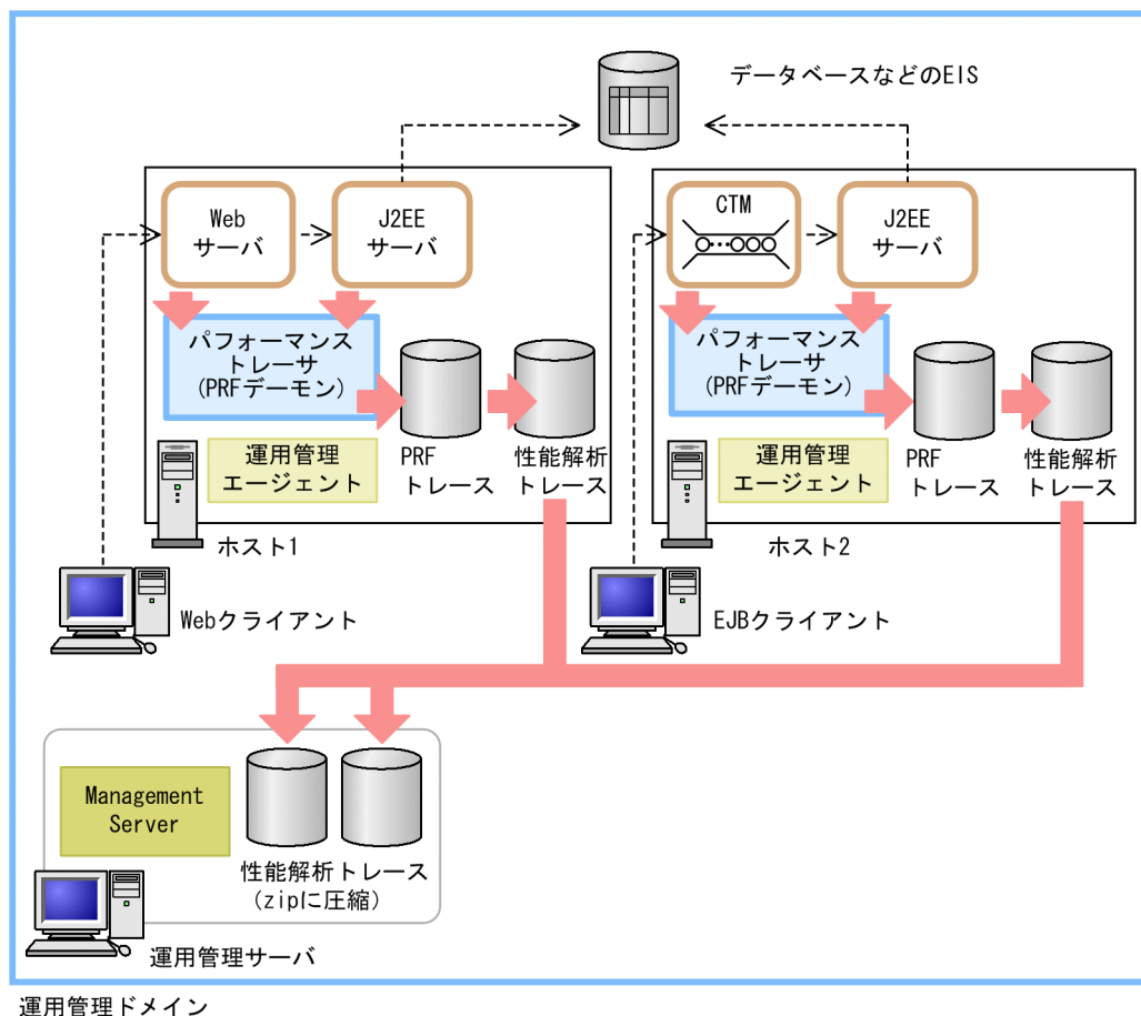
図 7-2 性能解析トレースのトレース情報収集の概要
