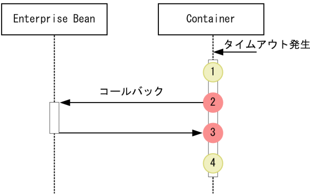
図 8-27 Timer Service のトレース取得ポイント (コールバックの場合)
