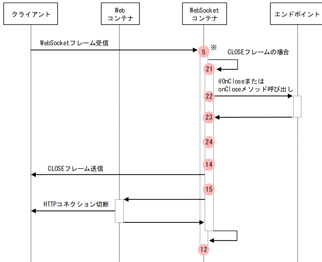
図 8-116 WebSocket のトレース取得ポイント (クロー징ハンドシェイク要求受信時 (ペイロードデータあり))
