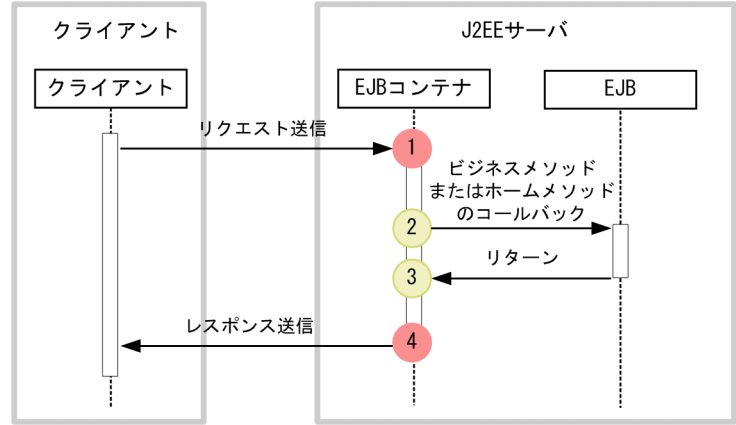
図 8-21 Session Bean, Entity Bean のトレース取得ポイント
