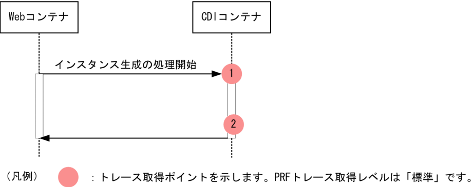
図 8-103 サーブレット・フィルタ・リスナと CDI を組み合わせて利用する場合のトレース取得ポイント
