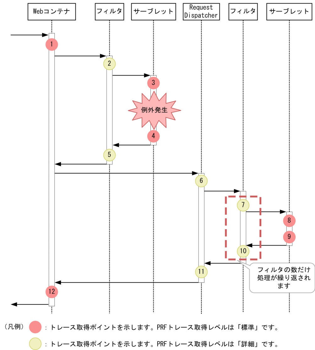
図 8-12 例外が発生した場合の Web コンテナでのトレース取得ポイント
