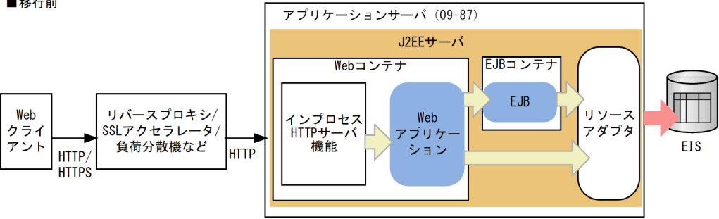
図 12-2 インプロセス HTTP サーバ構成をアプリケーションサーバ 11-70 に移行する場合
