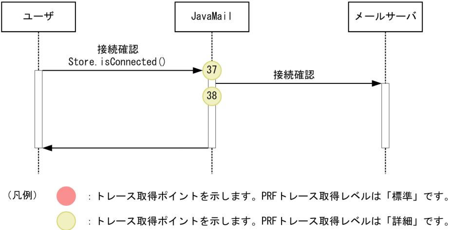
図 8-92 JavaMail のコネクション接続確認時の取得ポイント
