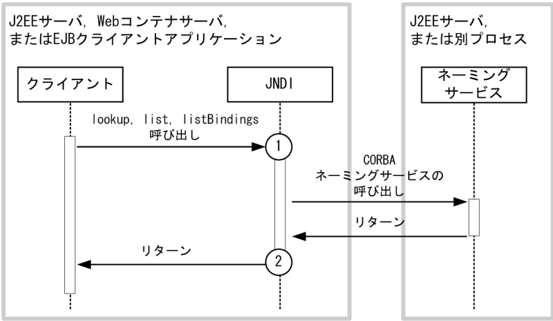
図 8-42 JNDI のトレース取得ポイント
