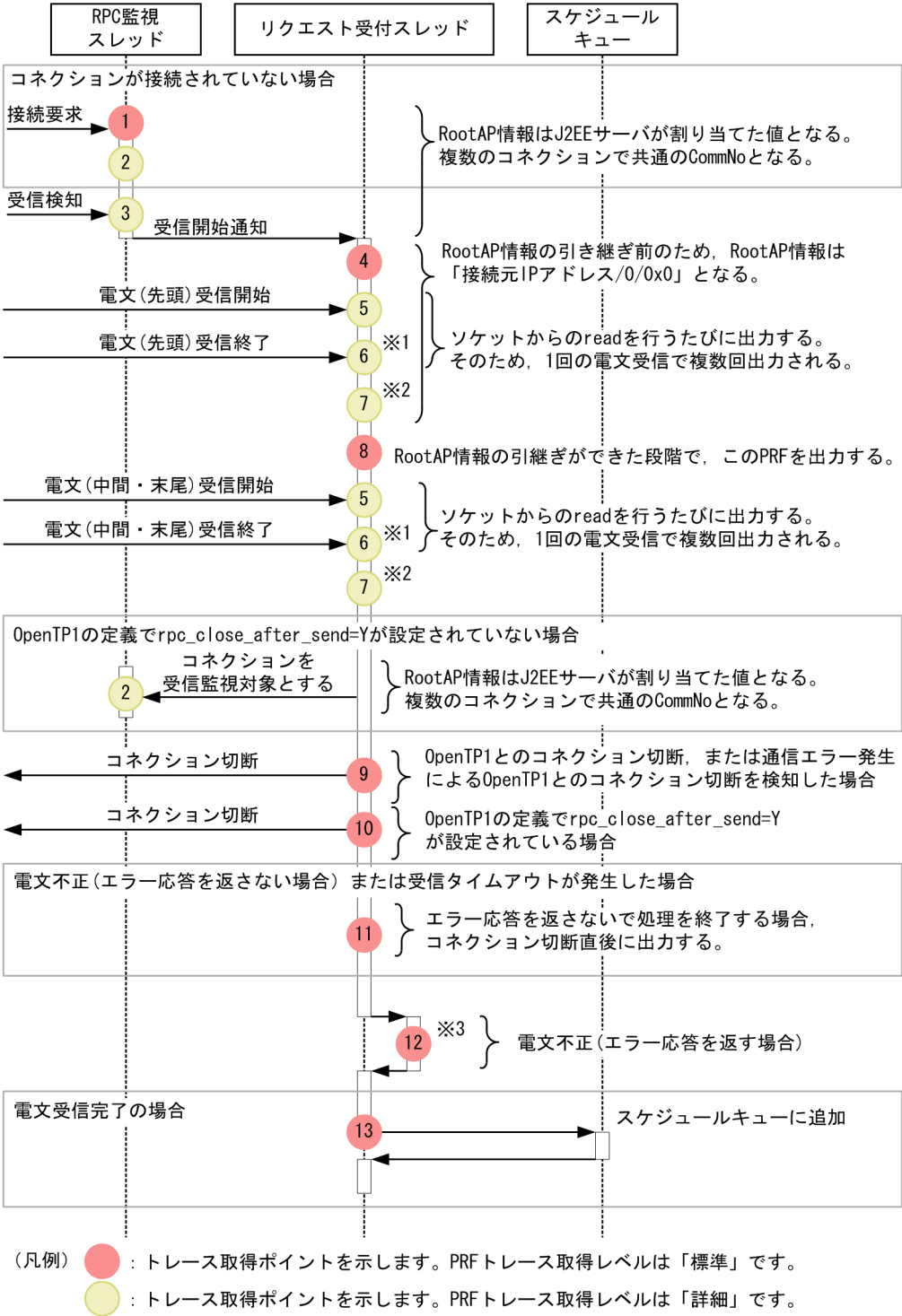
図 8-74 A 部分のトレース取得ポイント
