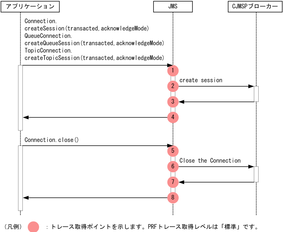
図 8-81 JMS Connection インタフェースのトレース取得ポイント
