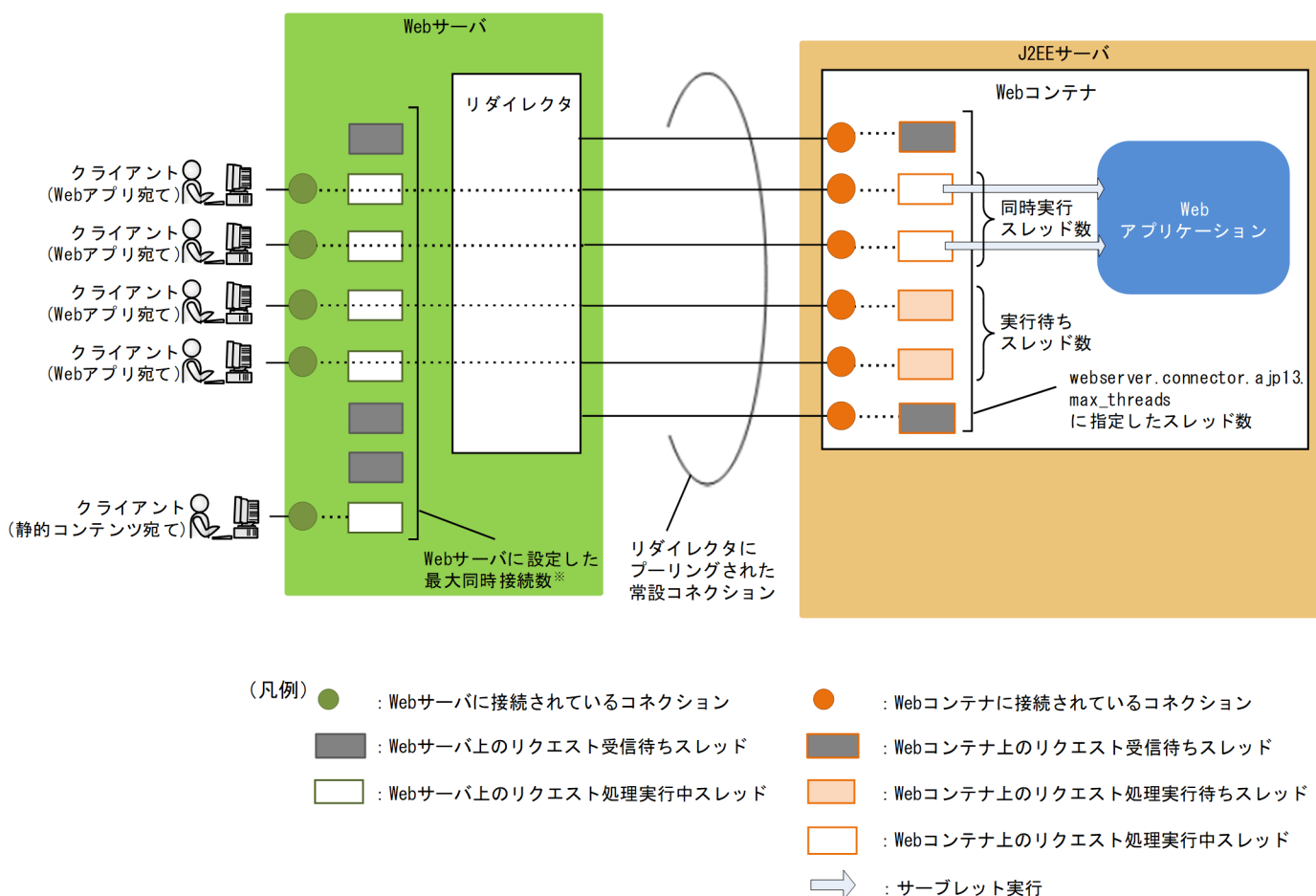
図 12-3 アプリケーションサーバ 09-87 のスレッド数制御の仕組み (Web サーバ連携の場合)
