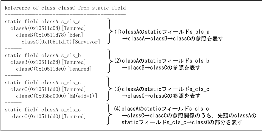
図 9-9 出力結果 (static フィールドを基点とした参照関係情報出力機能)
