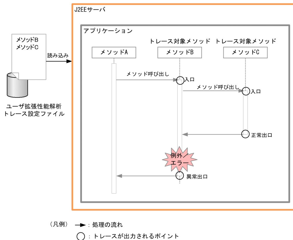
図 7-6 ユーザ拡張性能解析トレースによるトレース出力の概要
