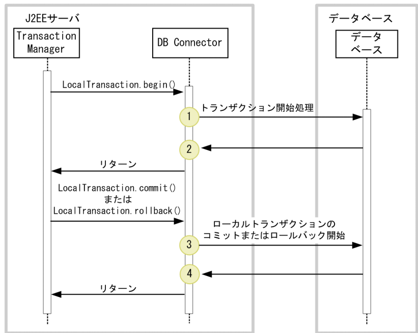
図 8-50 DB Connector, JCA コンテナでのトレース取得ポイントの詳細（ローカルトランザクション関連）
