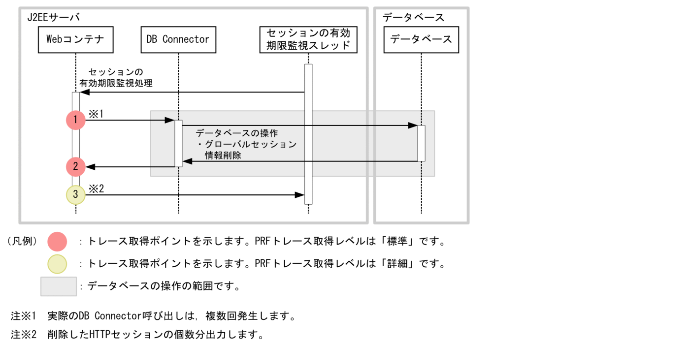
図 8-16 有効期限監視で HTTP セッションを無効化するリクエスト処理のトレース取得ポイント（データベースセッションフェイルオーバー機能）
