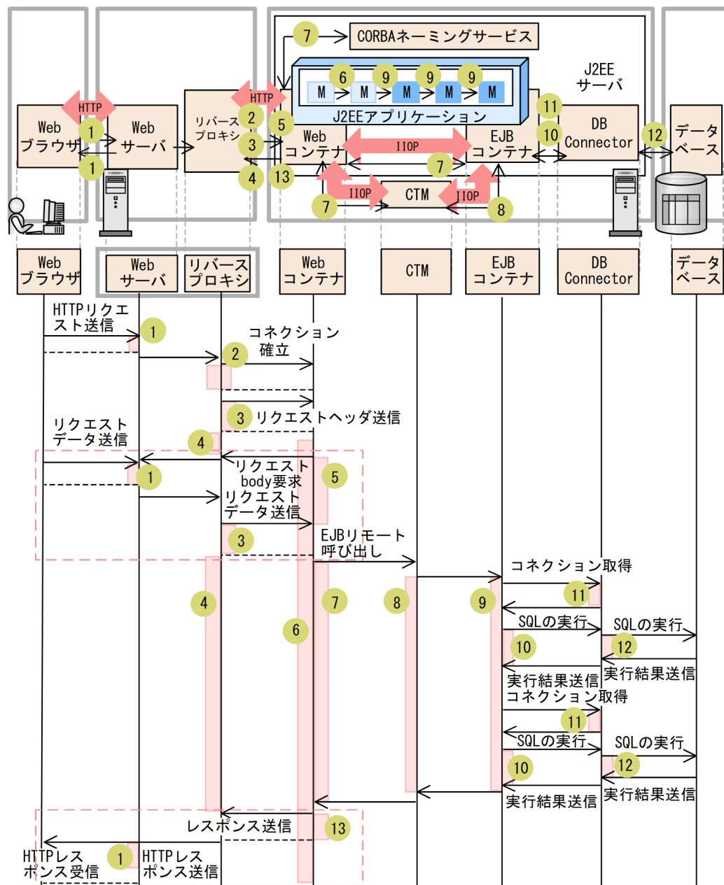
図 12-6 アプリケーションサーバ 11-70 でタイムアウトが設定できるポイント (Web サーバ連携の場合)
