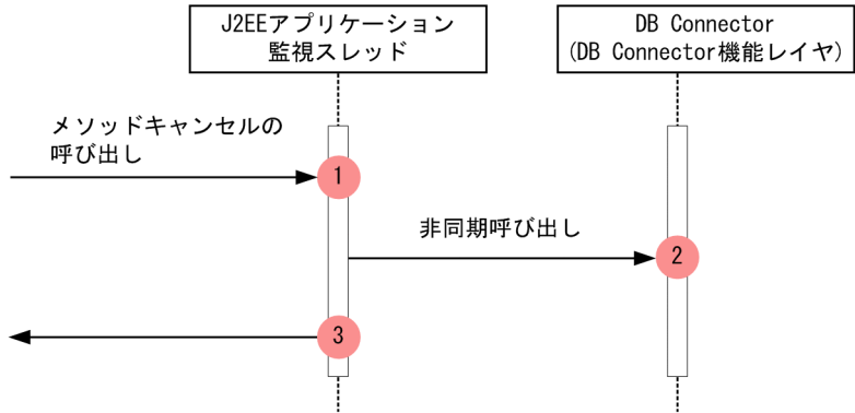
図 8-41 メソッドキャンセルが発生した場合のトレース取得ポイント
