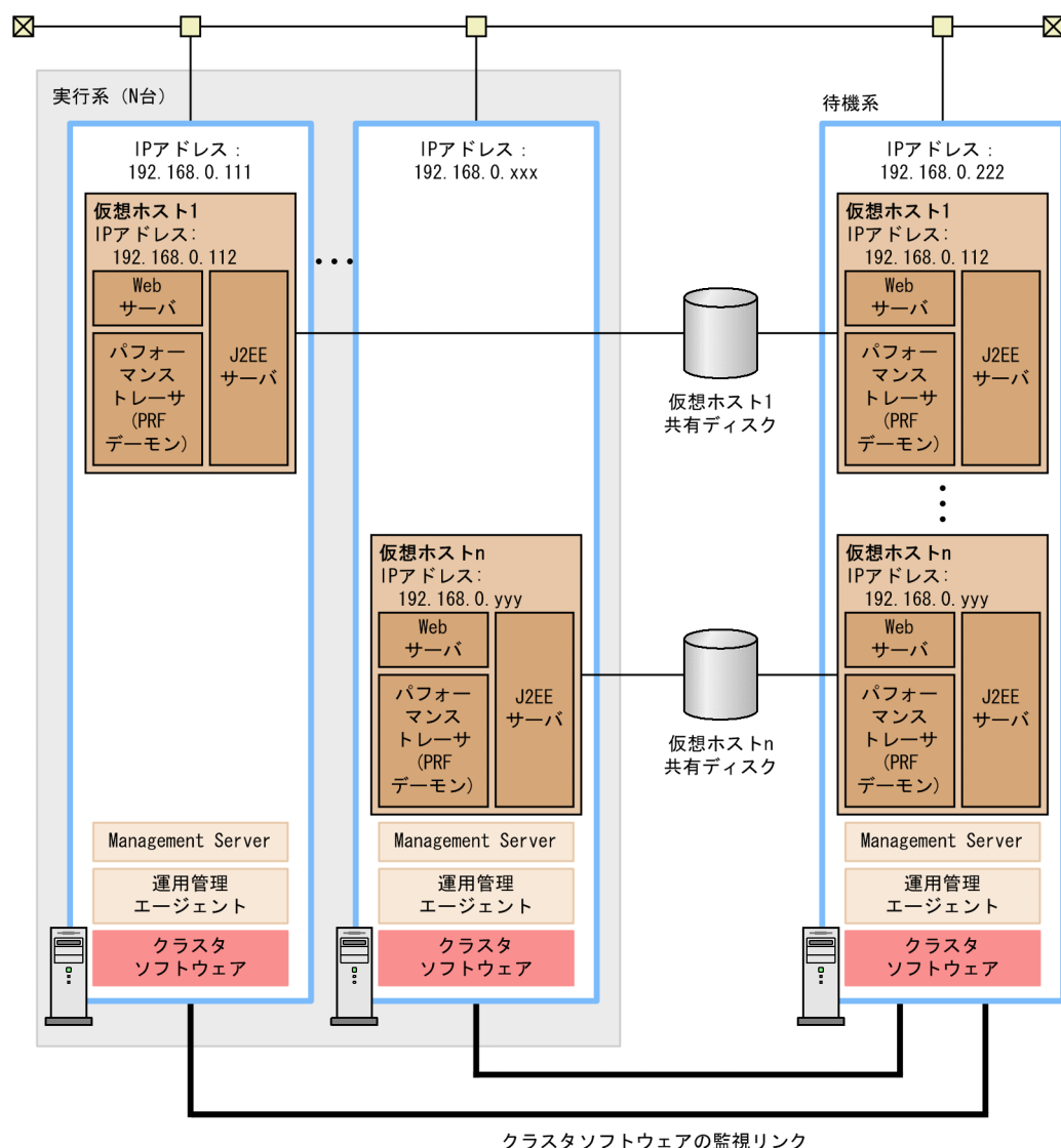
図 16-1 ホスト単位管理モデルを対象にした系切り替えシステムのシステム構成例
