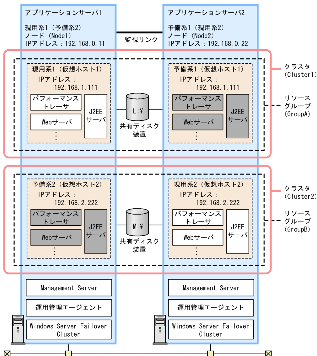
図 18-5 相互系切り替えシステムの構成例 (Windows の場合)
