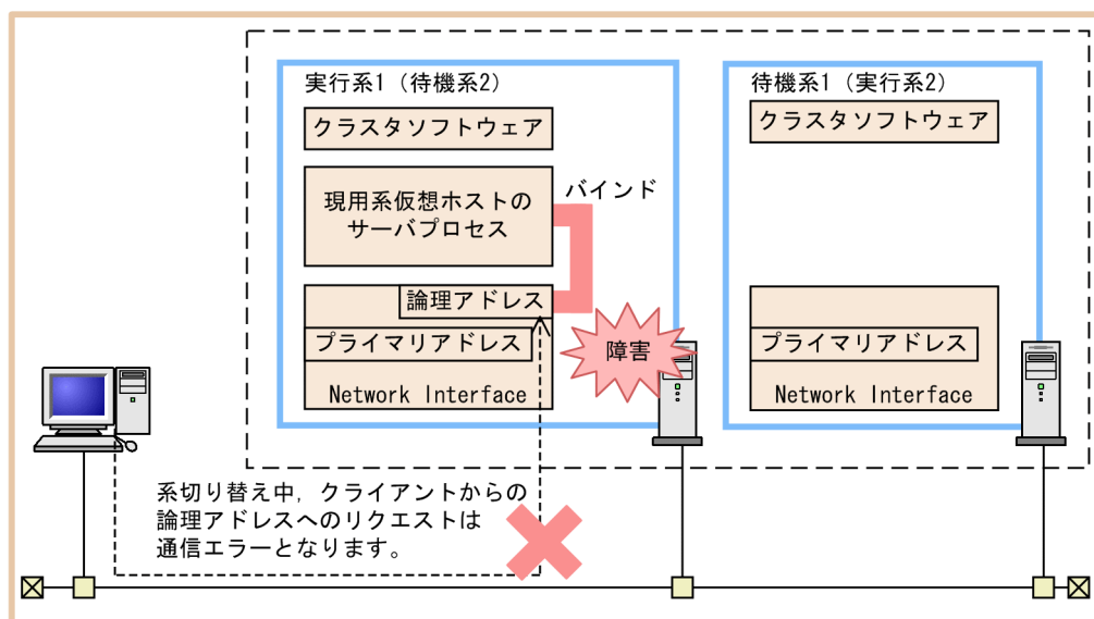
図 18-2 相互系切り替えシステムでの系切り替えの動作
