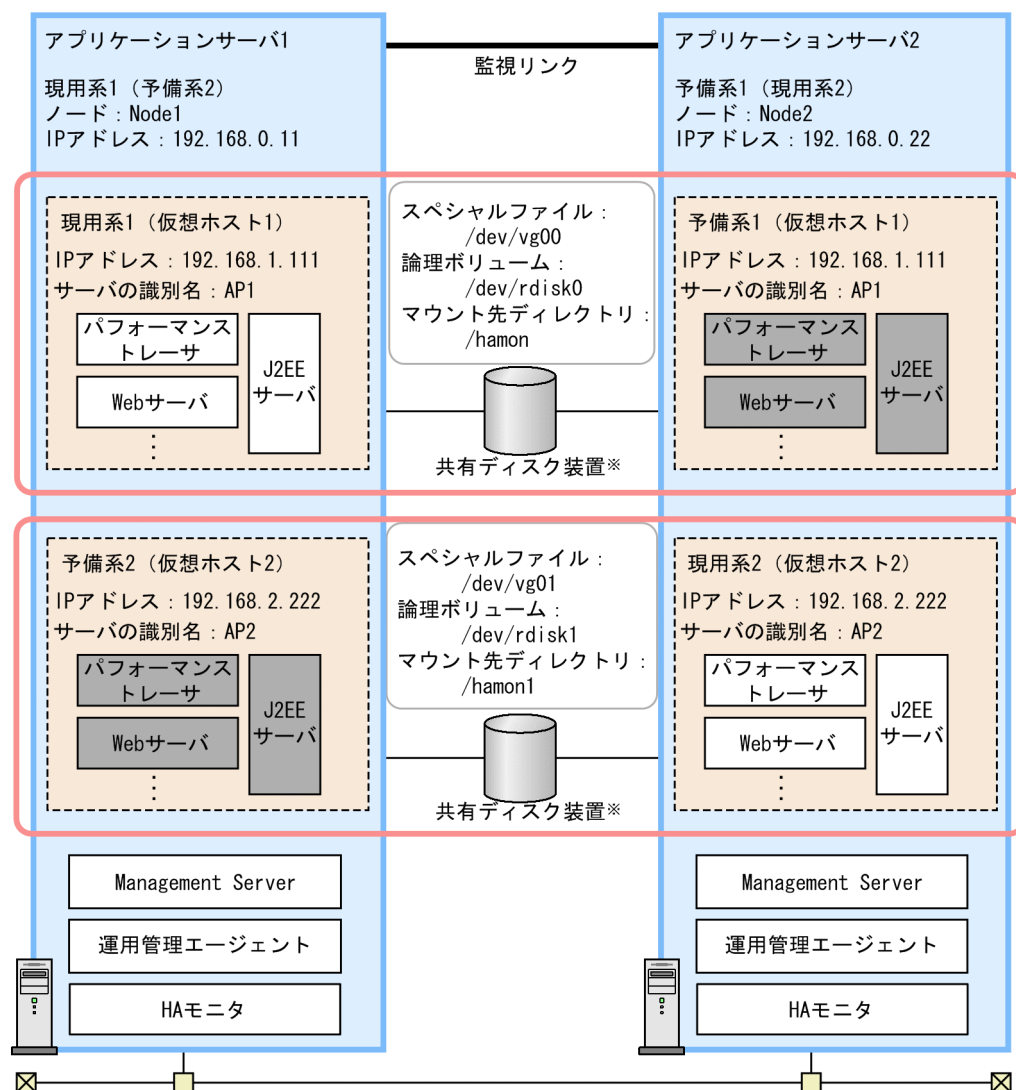
図 18-7 相互系切り替えシステムの構成例 (UNIX の場合)
