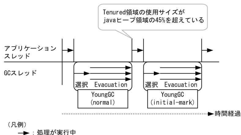
図 7-29 YoungGC の流れ
