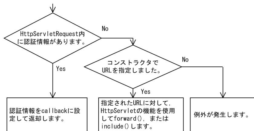
図 15-1 認証情報の読み込み順序
