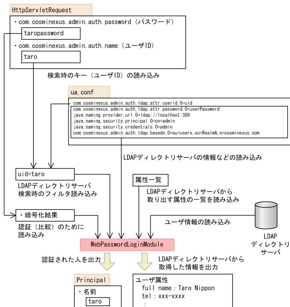
図 5-12 WebPasswordLoginModule の概要
