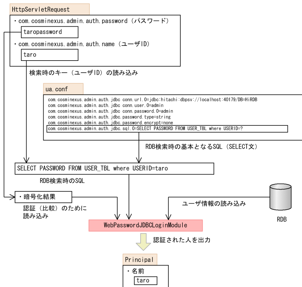
図 5-15 WebPasswordJDBCLoginModule の概要
