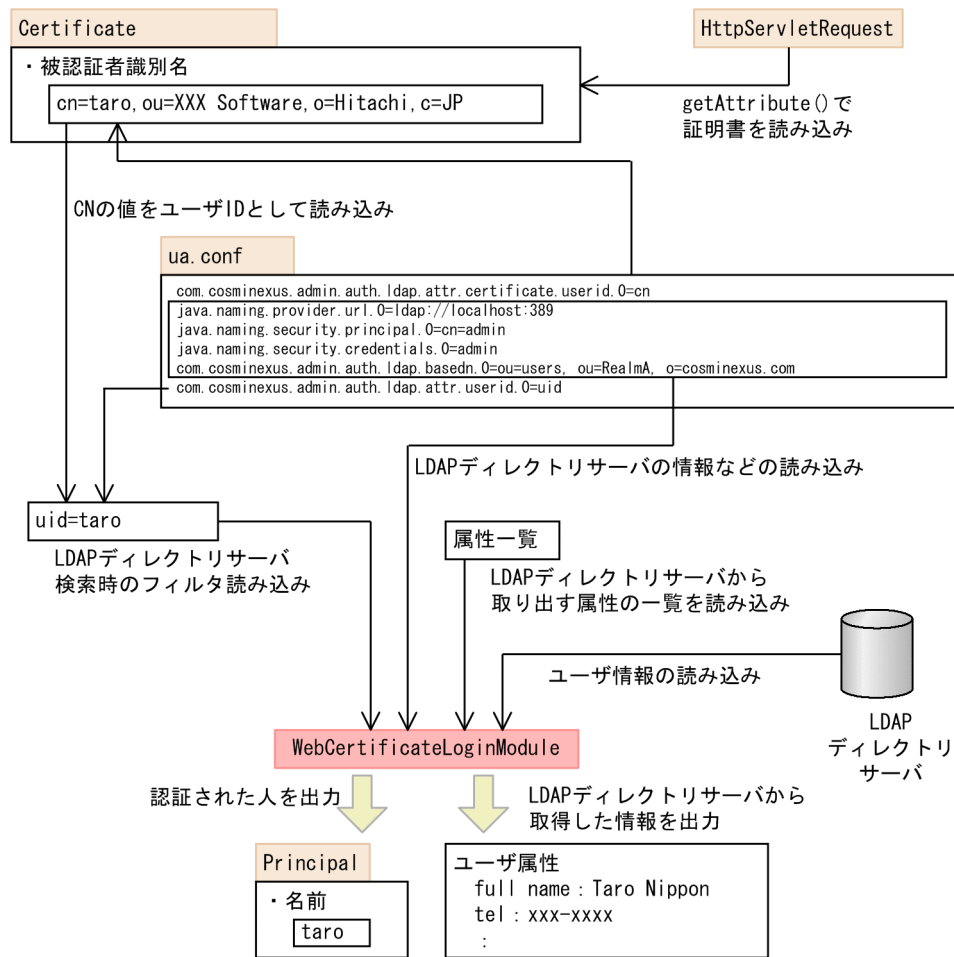
図 5-13 WebCertificateLoginModule の概要
