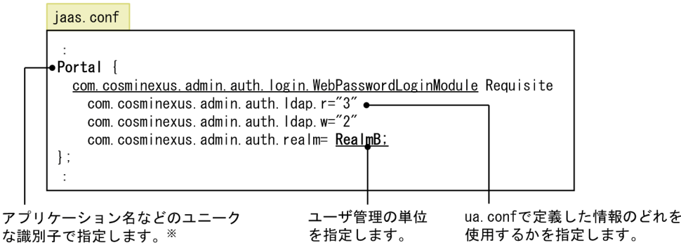
図 5-27 jaas.conf の設定例
