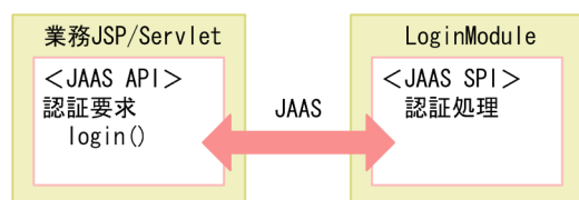
図 5-4 API と SPI の関係
