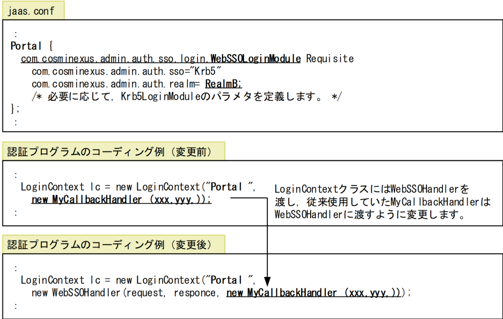
図 5-34 シングルサインオンへの対応例（カスタムログインモジュールの場合）
