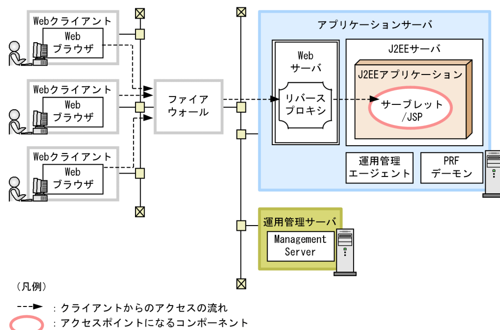
図 3-1 サーブレットと JSP に対するアクセスをファイアウォール経由にする構成
