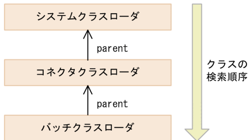
図 2-9 バッチアプリケーションを実行するクラスローダの構成
