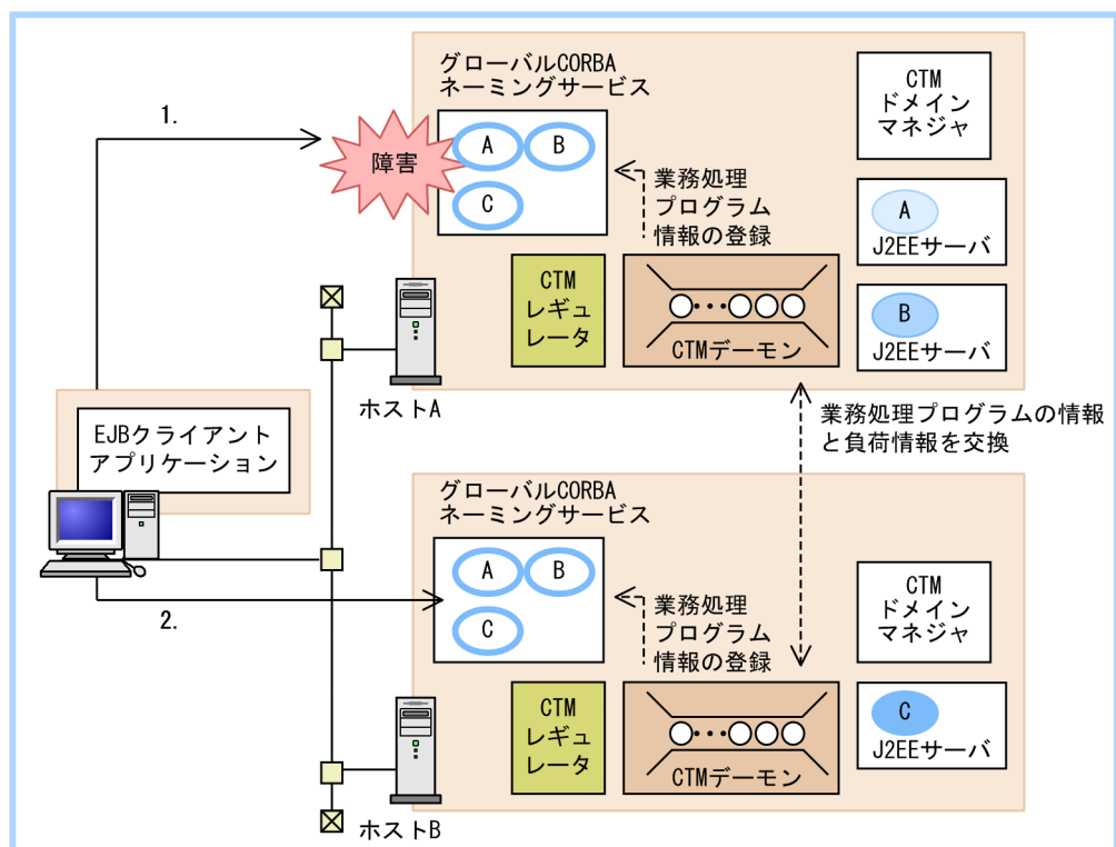
図 3-13 グローバル CORBA ネーミングサービスを使用した処理の流れの例
