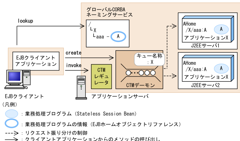
図 3-1 スケジュールキューを共有する例（J2EE アプリケーション単位）
