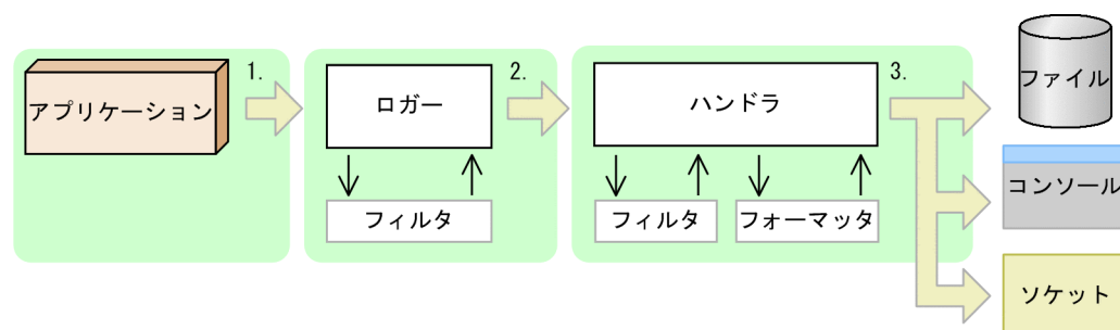
図 8-2 Java ロギングの仕組み
