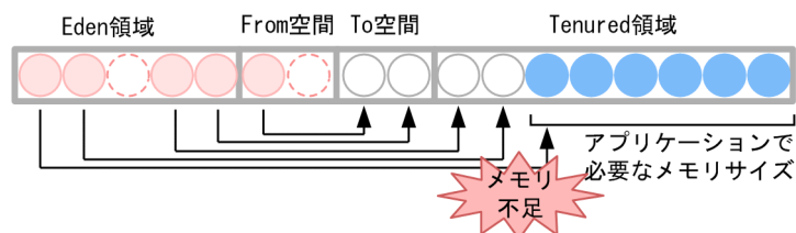
図 7-11 New 領域のメモリサイズを追加する理由の考え方
