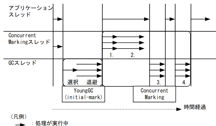
図 7-30 Concurrent Marking の流れ
