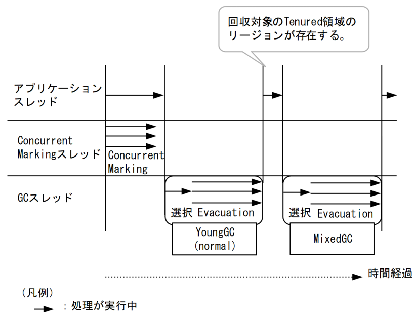
図 7-32 MixedGC の処理の流れ (JDK17 以降の場合)
