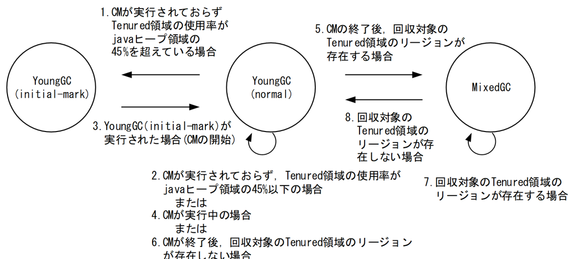
図 7-27 各 GC の状態遷移図 (JDK17 以降の場合)
