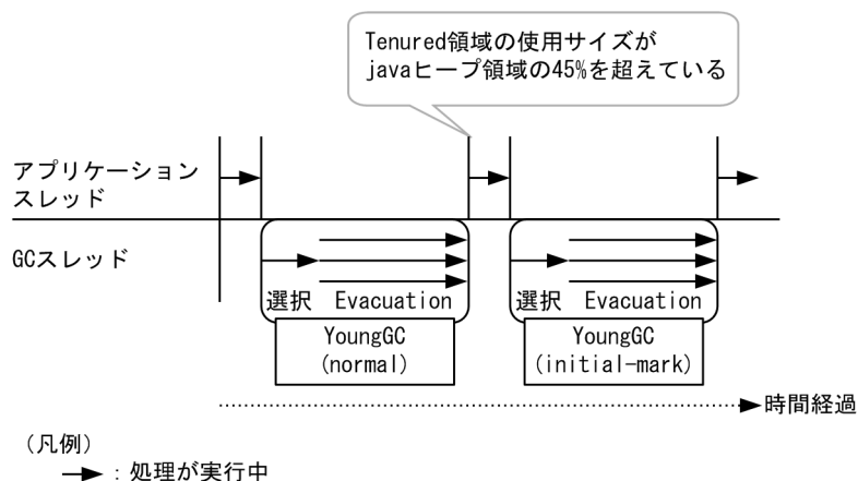
図 7-29 YoungGC の流れ
