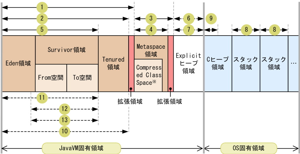
図 7-7 JavaVM で使用するメモリ空間の構成
