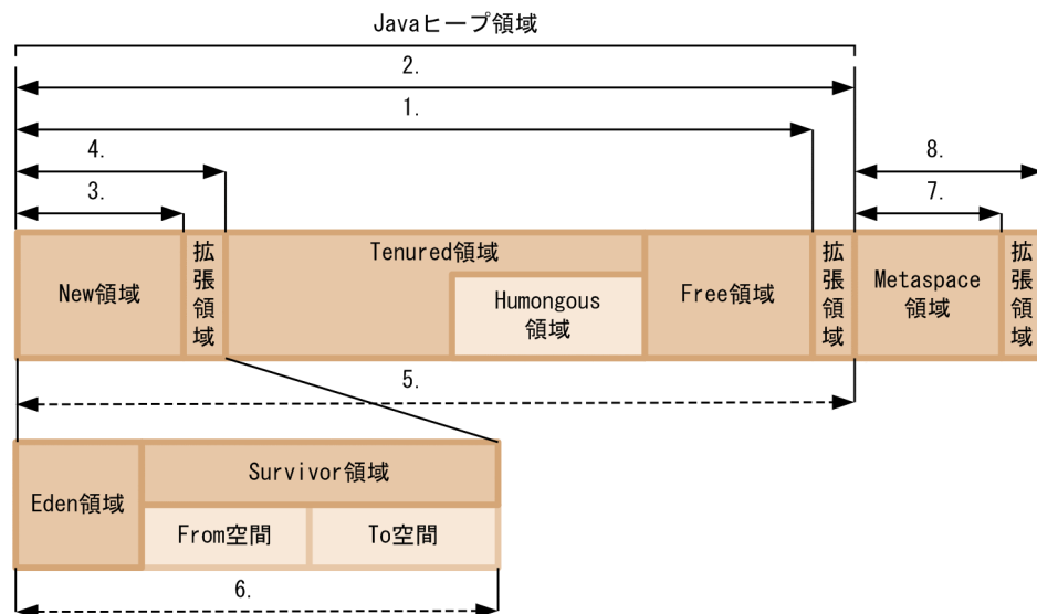
図 7-34 Java ヒープ領域内の各領域と Metaspace 領域のサイズとオプションの対象範囲
