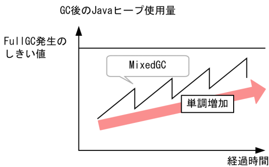
図 7-39 FullGC の発生を抑止するチューニングのイメージ
