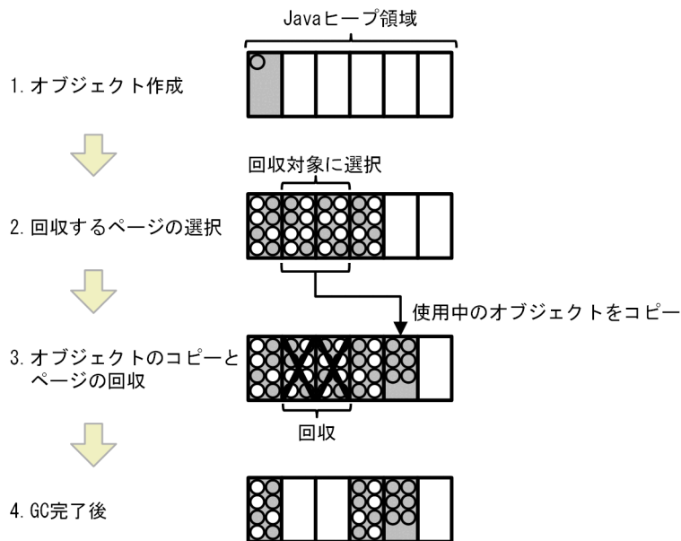
図 7-44 オブジェクト作成から GC 完了までの流れ
