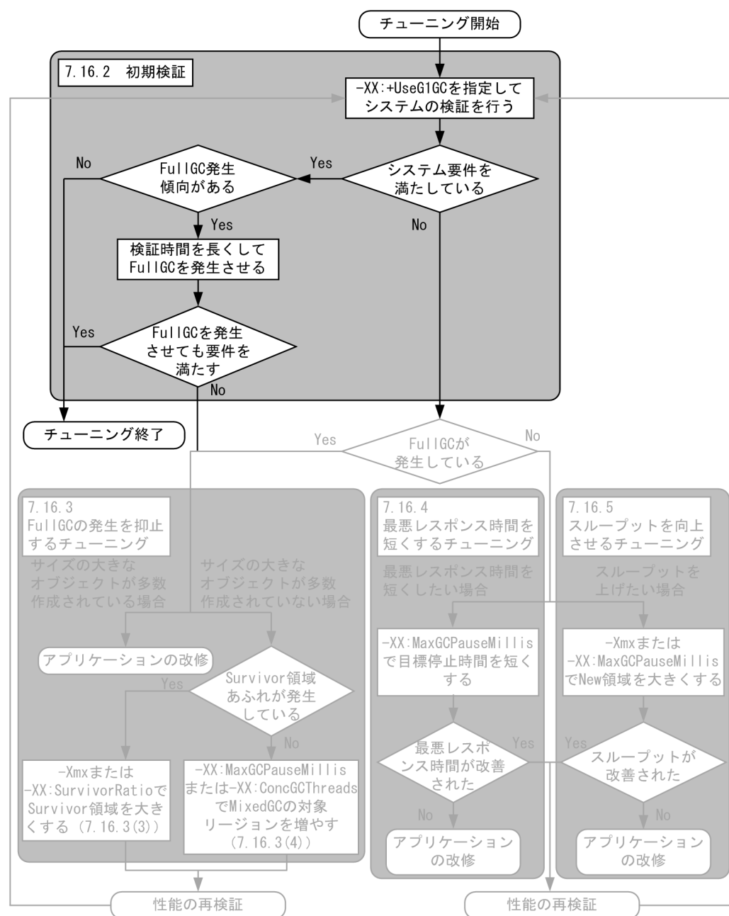
図 7-36 初期検証の流れ
