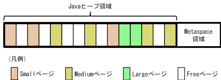
図 7-42 アプリケーション実行中の ZGC で管理するメモリ空間の構成
