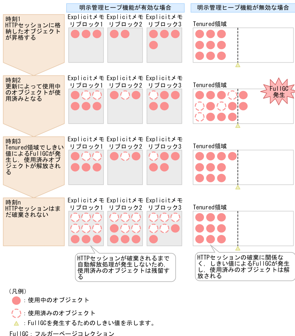
図 A-3 明示管理ヒープ機能が有効な場合と明示管理ヒープ機能が無効な場合のオブジェクトの解放処理の違い
