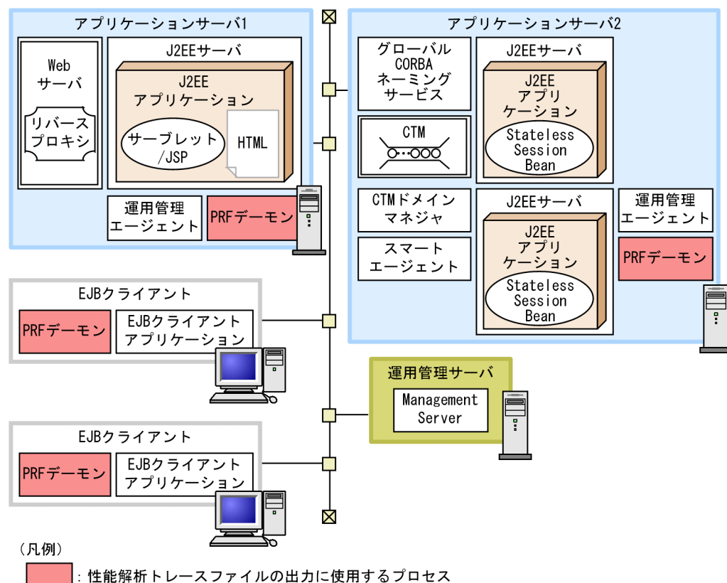
図 3-57 PRF デーモンを配置する例
