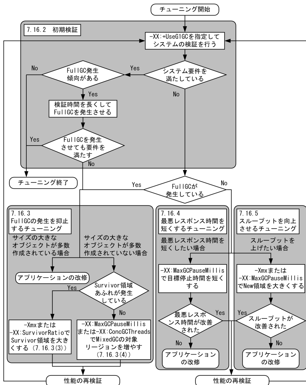
図 7-35 チューニングの全体の流れ
