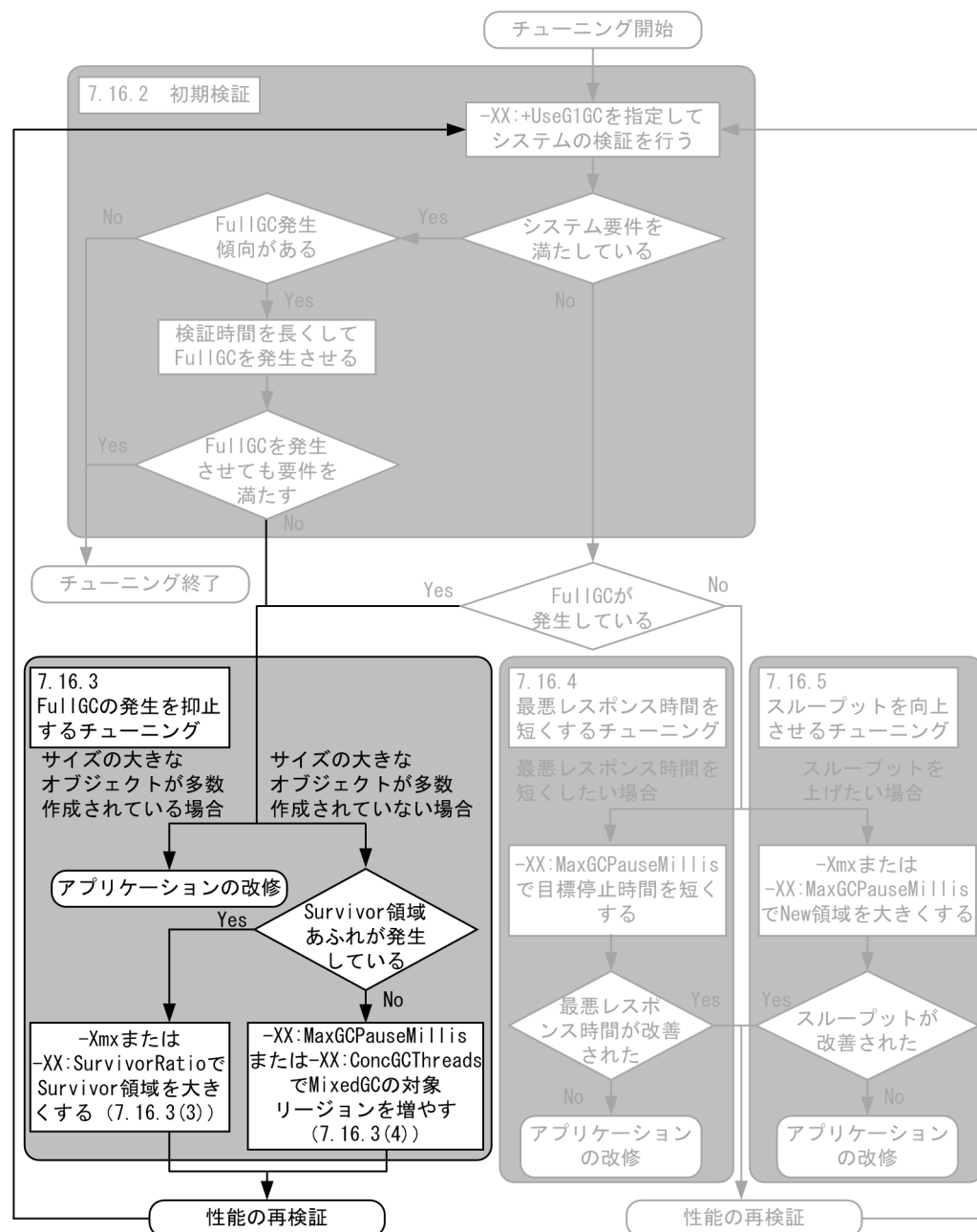
図 7-38 FullGC の発生を抑止するチューニングの流れ
