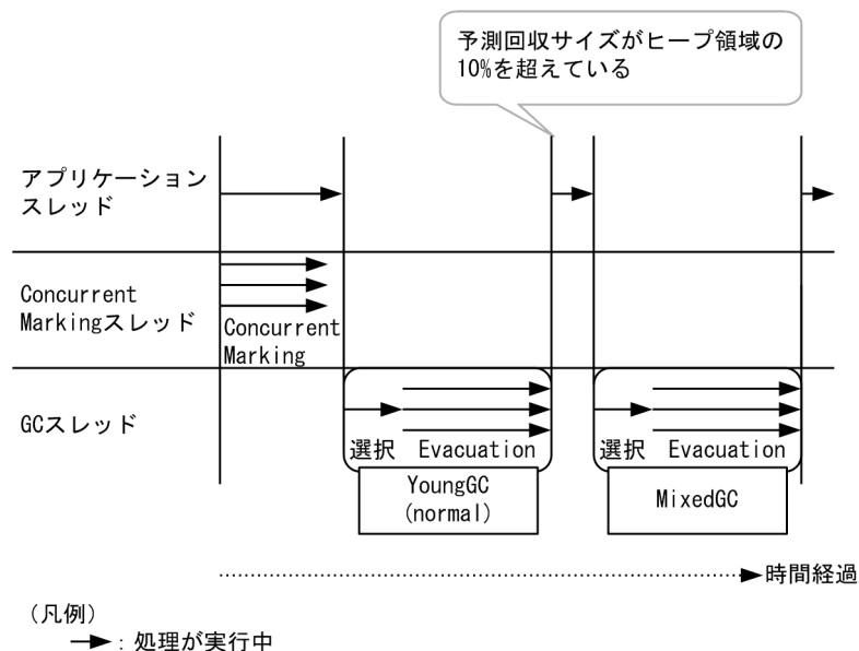
図 7-31 MixedGC の処理の流れ (JDK11 以前の場合)
