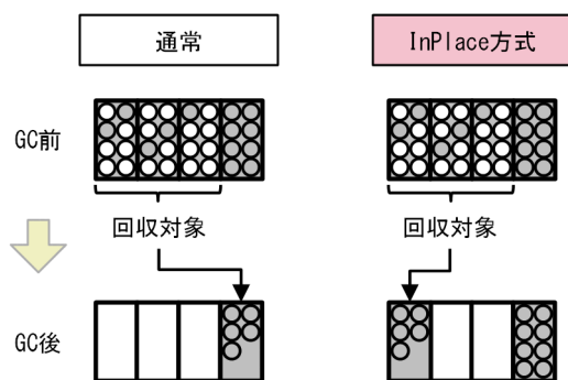
図 7-45 InPlace の概要
