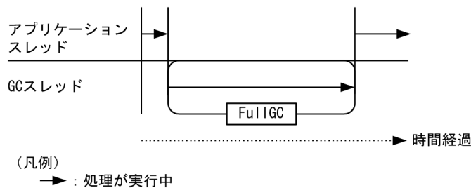
図 7-33 FullGC の流れ
