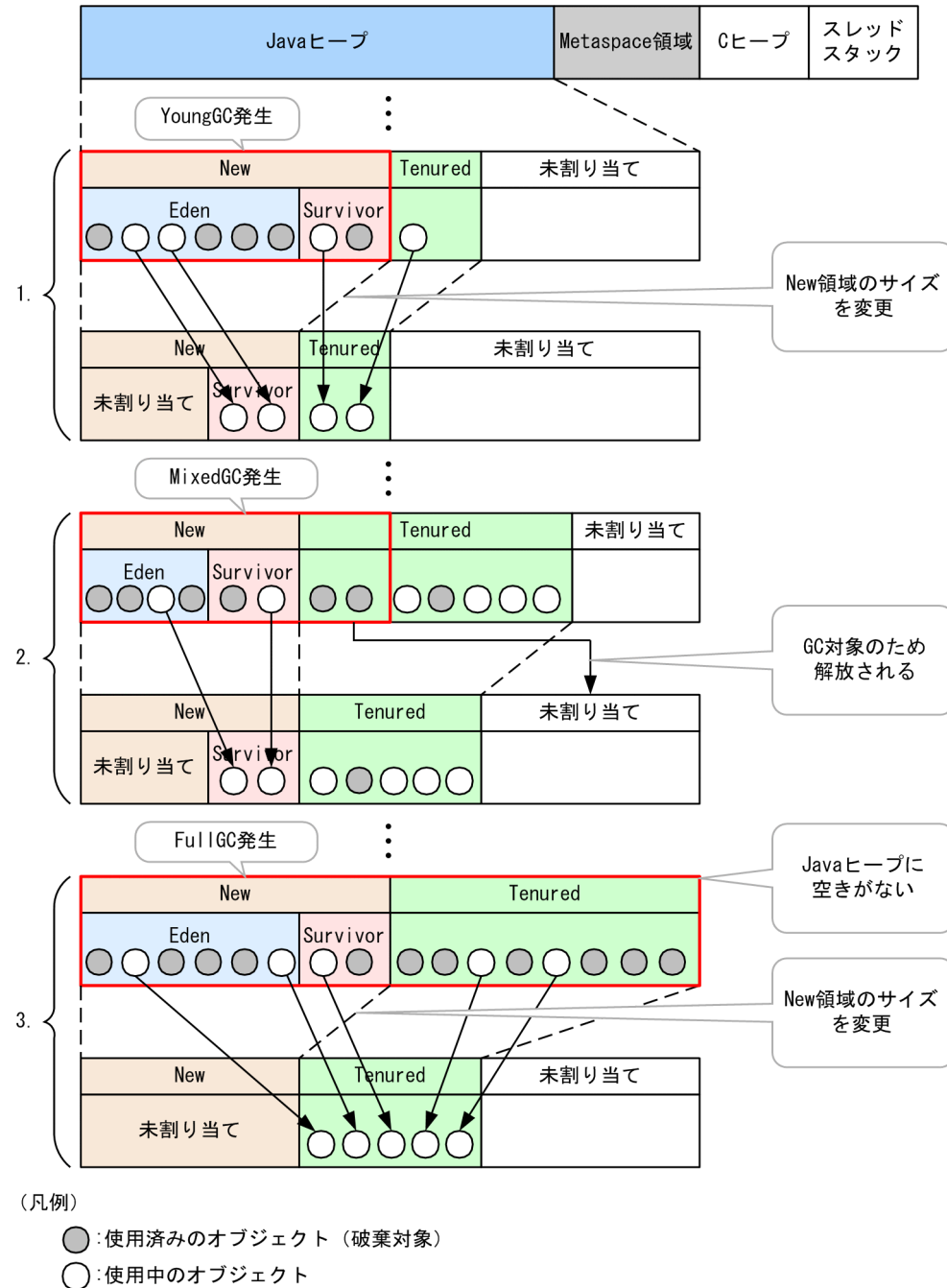
図 7-28 G1GC の流れ
