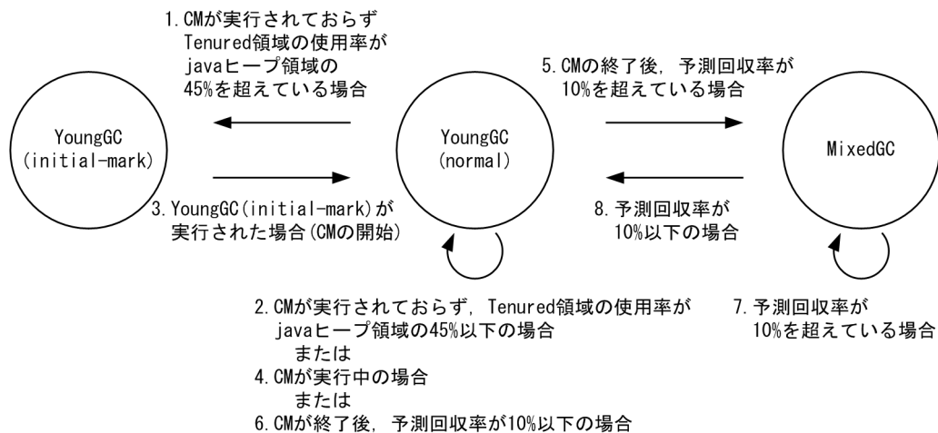
図 7-26 各 GC の状態遷移図 (JDK11 以前の場合)
