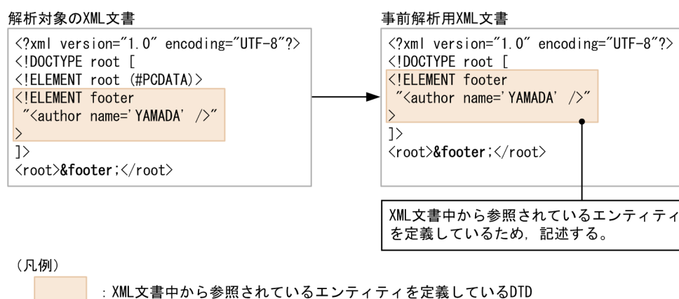
図 3-19 XML 文書中から参照されているエンティティの定義を記述する例（事前解析用 XML 文書の作成指針）
