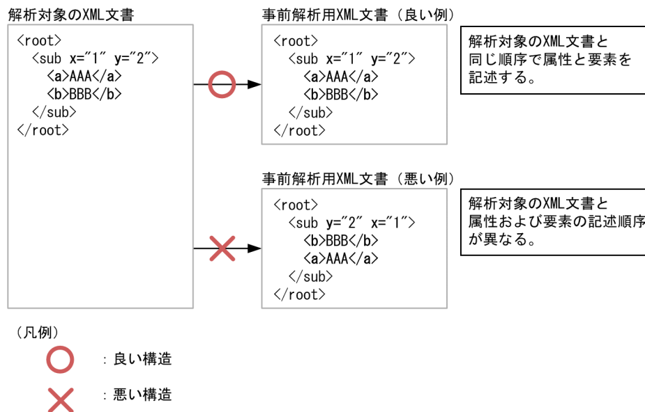
図 3-11 要素と属性を記述する例（事前解析用 XML 文書の作成指針・要素と属性の順序）
