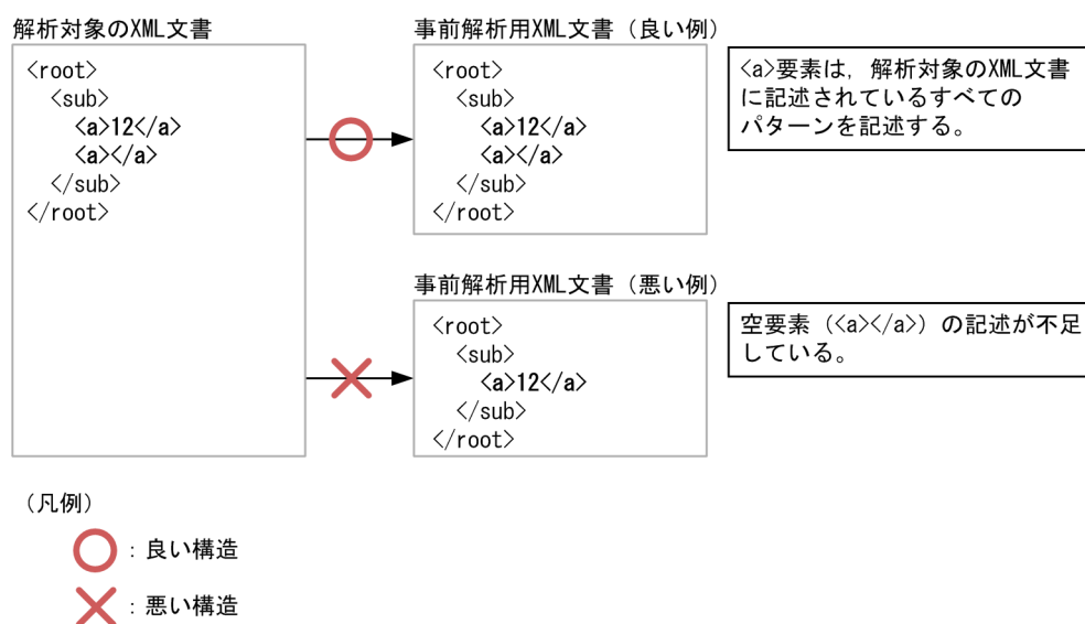
図 3-17 空要素を記述する例（事前解析用 XML 文書の作成指針）
