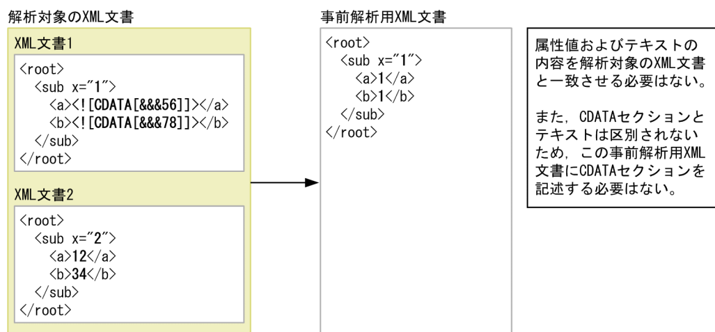
図 3-16 テキスト、CDATA セクション、属性値を記述する例（事前解析用 XML 文書の作成指針）
