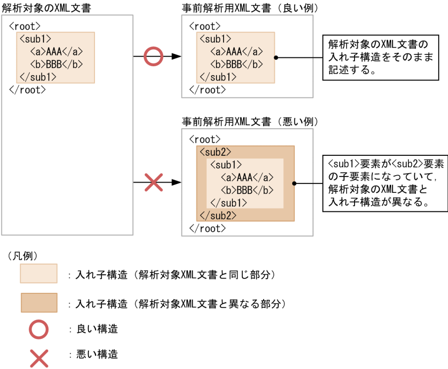
図 3-13 要素の入れ子構造を記述する例（事前解析用 XML 文書の作成指針）
