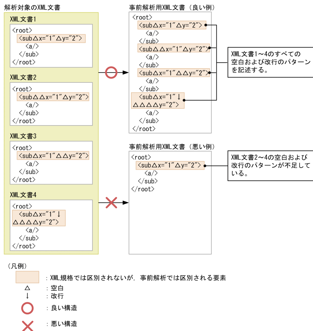
図 3-10 改行文字・空白文字の数や位置が異なる要素を記述する例（事前解析用 XML 文書の作成指針）
