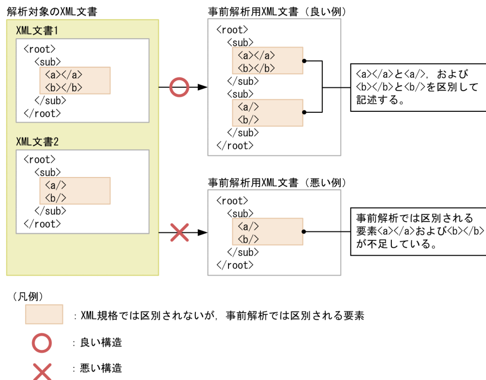
図 3-9 空要素と空要素タグを記述する例（事前解析用 XML 文書の作成指針）
