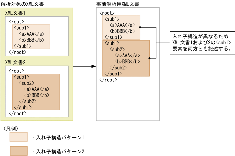
図 3-14 要素の入れ子構造を複数記述する例（事前解析用 XML 文書の作成指針）
