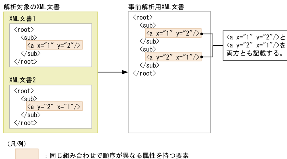
図 3-12 同じ組み合わせで順序が異なる属性を記述する例（事前解析用 XML 文書の作成指針）
