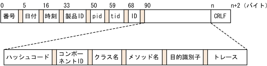
図 9-3 メソッドトレースの出力形式
