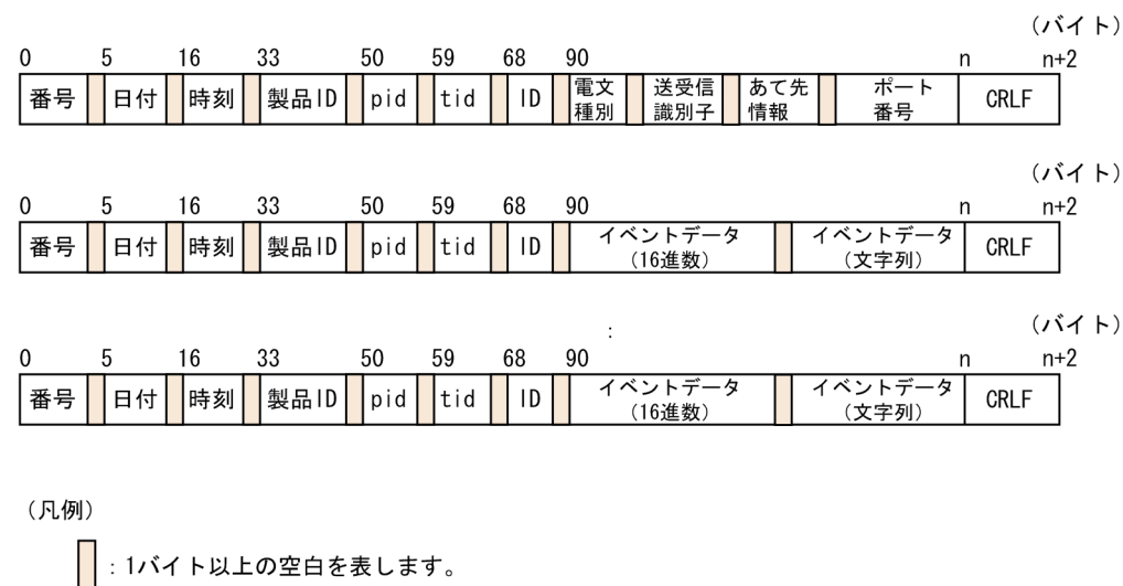
図 9-6 不正イベントトレース出力時の共用キューイベントトレースの出力形式
