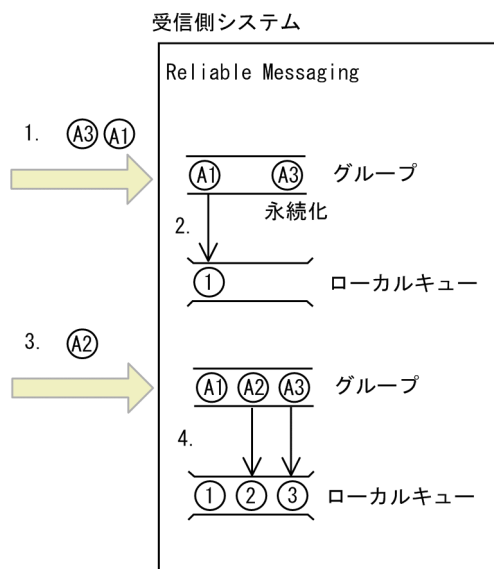
図 2-21 順序保証の仕組み
