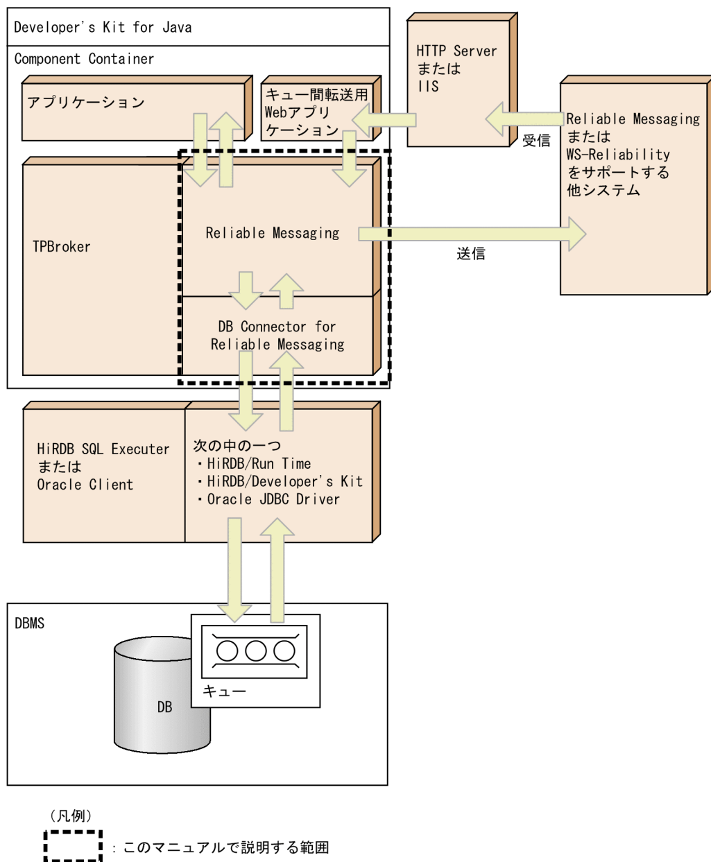
図 1-3 永続版リソースアダプタを使用する場合のシステムのソフトウェア構成
