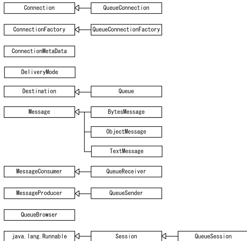
図 7-1 JMS インタフェースの継承
