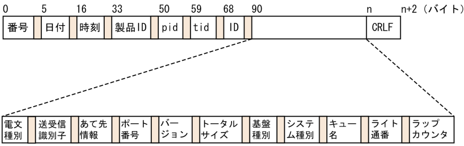
図 9-5 共用キューイベントトレースの出力形式
