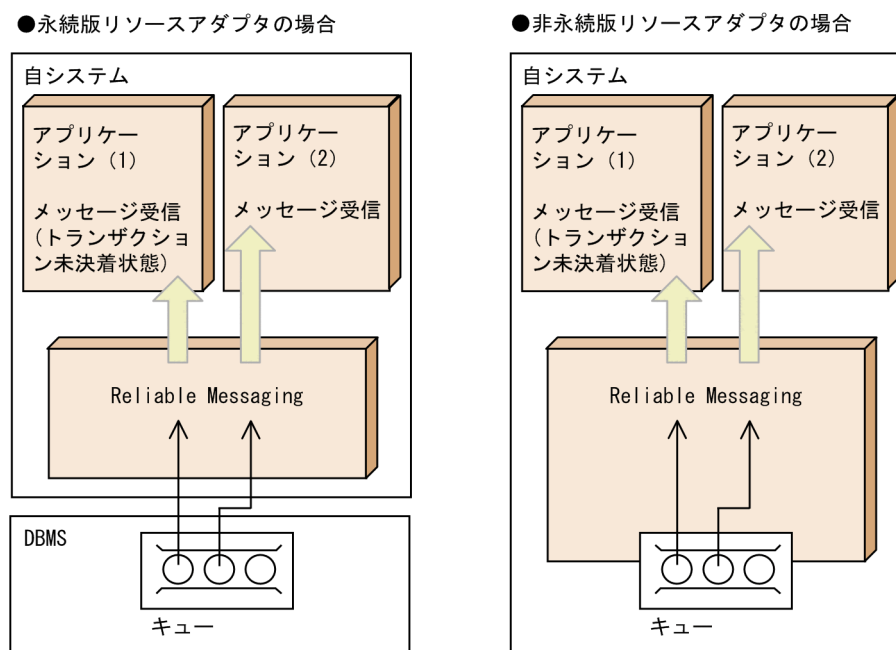
図 2-11 パラレル取り出し属性の概要
