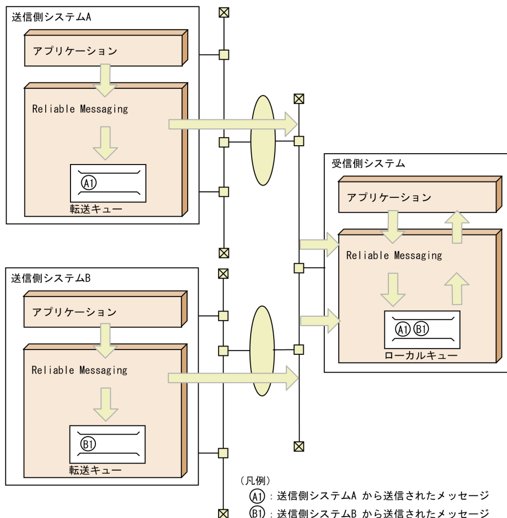
図 2-18 転送キューによるキュー間転送の概要
