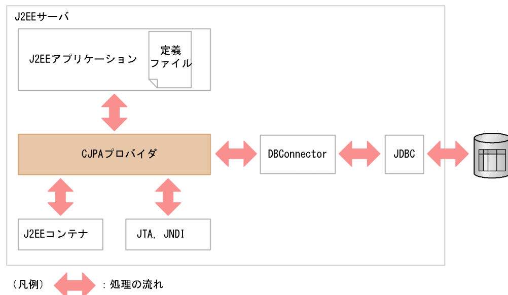
図 8-1 CJPA プロバイダの位置づけ
