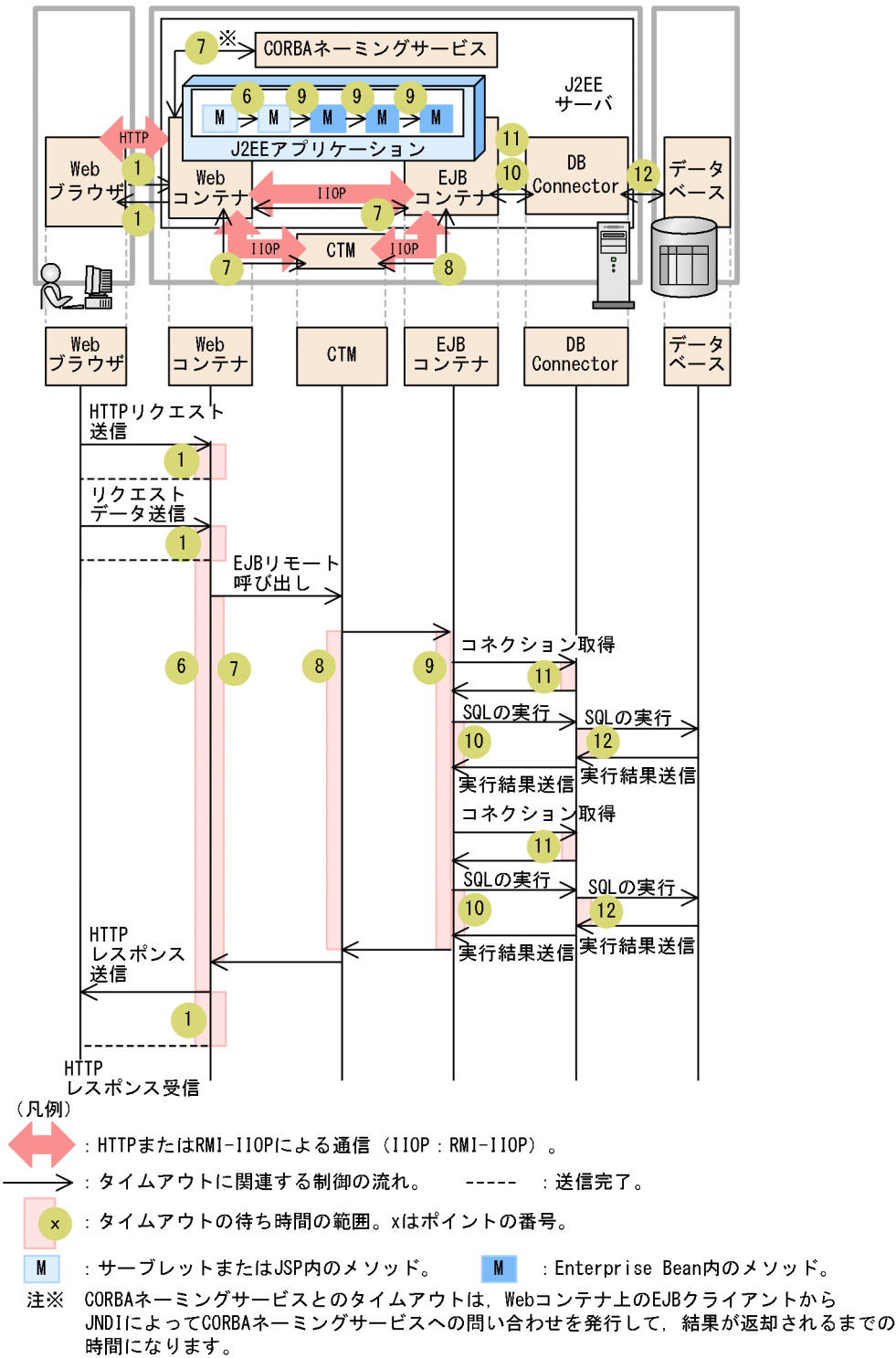
図 16-3 タイムアウトが設定できるポイント（インプロセス HTTP サーバの場合）
