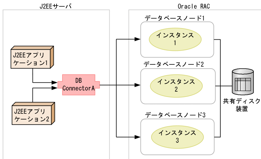
図 19-2 Oracle RAC の機能を使用した接続
