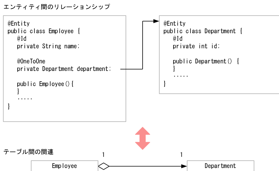
図 8-5 エンティティのリレーションシップとテーブル間の関連
