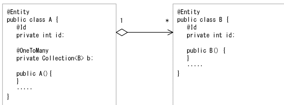
図 8-11 単方向 OneToMany でのデフォルトマッピング
