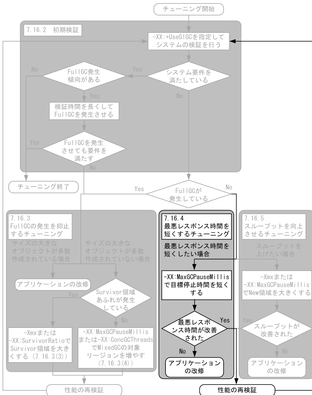
図 7-40 最悪レスポンス時間を短くするチューニングの流れ
