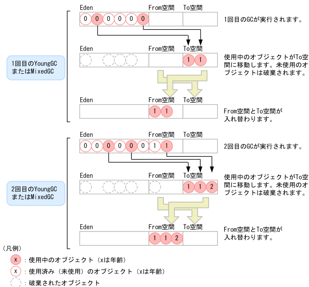
図 7-19 CopyGC 実行時に発生するオブジェクトの移動
