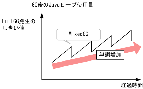
図 7-39 FullGC の発生を抑止するチューニングのイメージ
