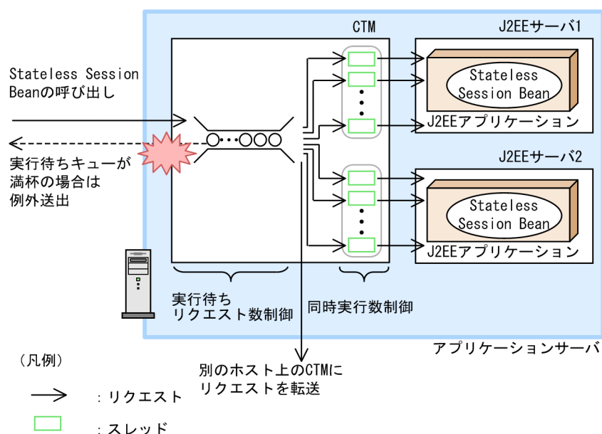
図 8-5 CTM による Stateless Session Bean の同時実行数制御の例
