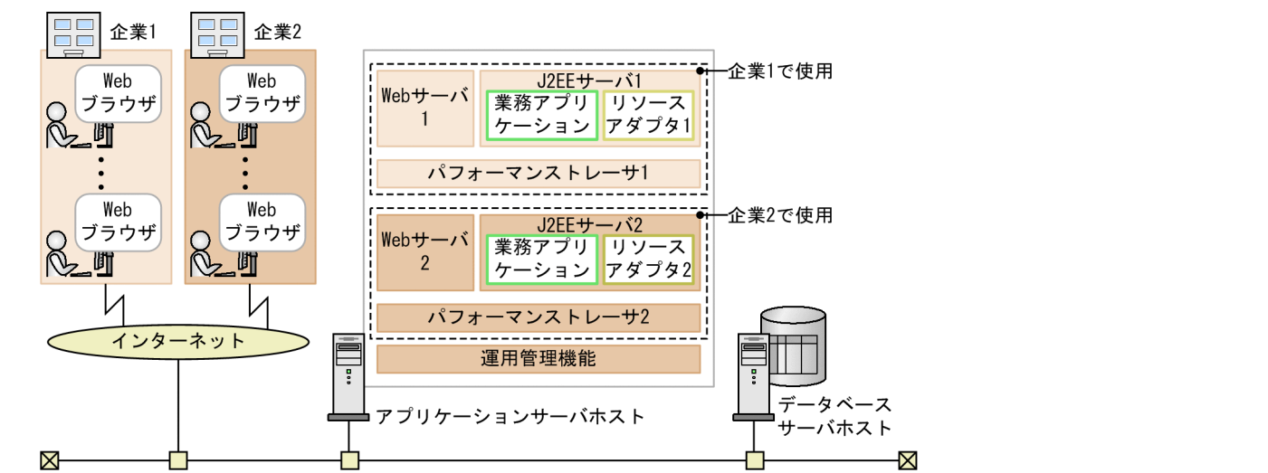
図 1-6 J2EE サーバを複数配置してマルチテナントに対応した Web フロントシステムの構成例
