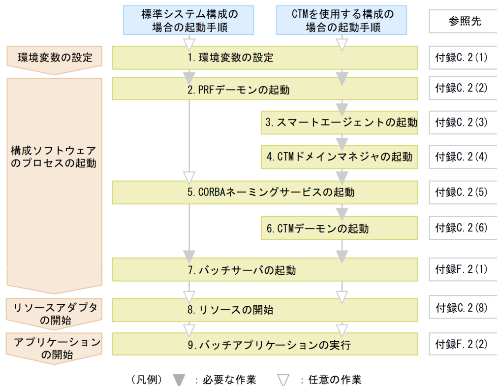
図 F-1 アプリケーションサーバの起動手順の流れ (Windows の場合)
