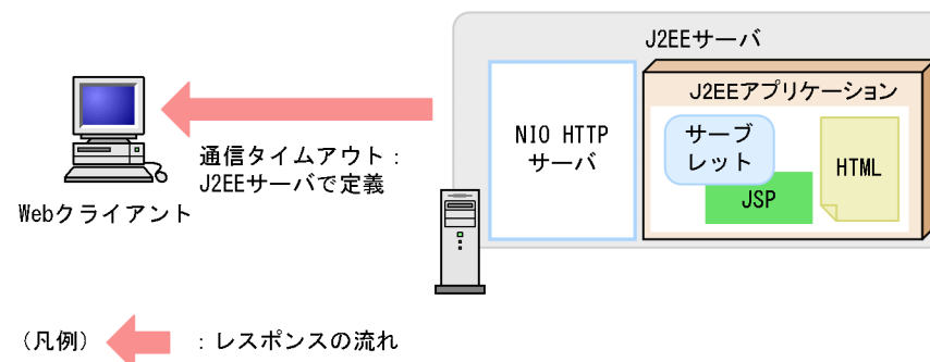
図 7-5 レスポンス送信時の通信タイムアウトの設定場所 (NIO HTTP サーバを使用する場合)
