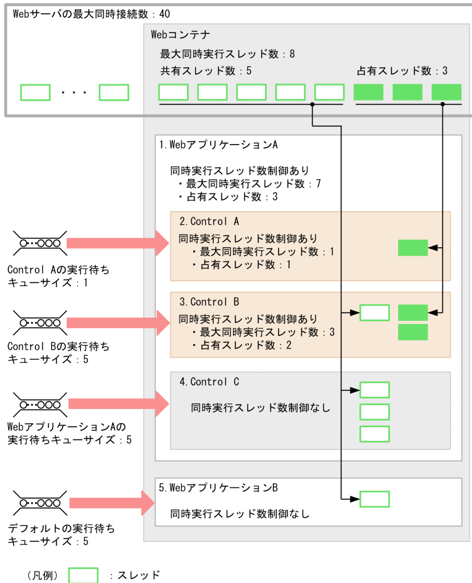
図 2-19 URL グループ単位の設定例
