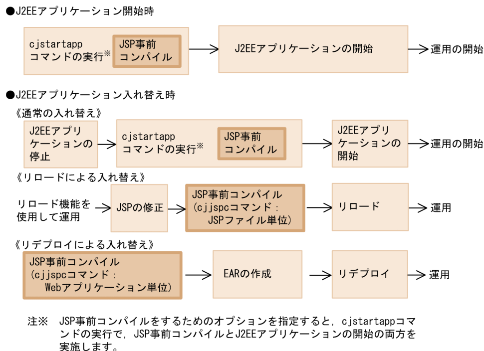
図 2-6 システム運用での JSP 事前コンパイルの適用
