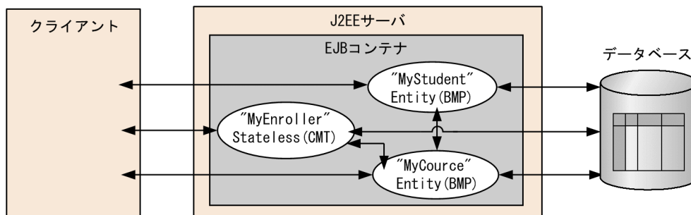
図 L-10 enroller の構成
