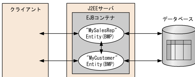
図 L-20 salesrep の構成
