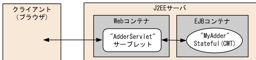
図 L-3 adder の構成
