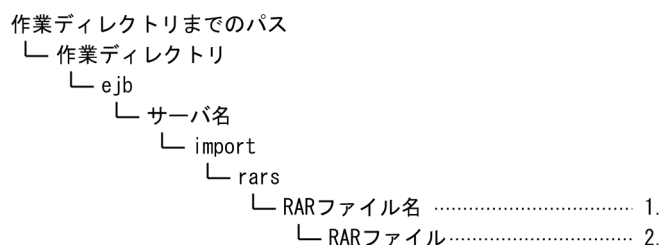
図 C-11 J2EE リソースのディレクトリ構成
