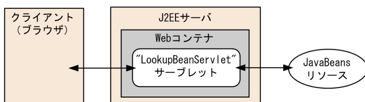
図 L-32 JavaBeans リソースのサンプルプログラムの構成
