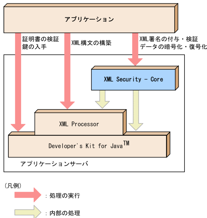
図 1-1 XML Security - Core の仕組み
