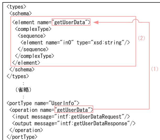
図 3-9 wrapped 形式の WSDL の例
