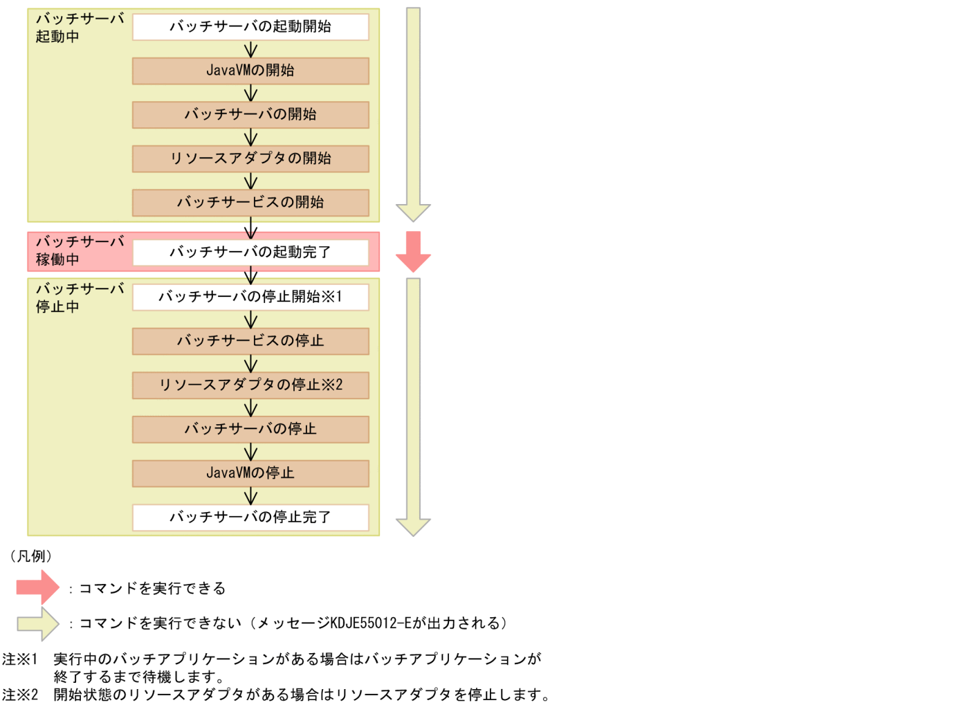
図 2-10 バッチサーバの状態とコマンドの実行可否
