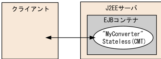
図 L-1 converter の構成
