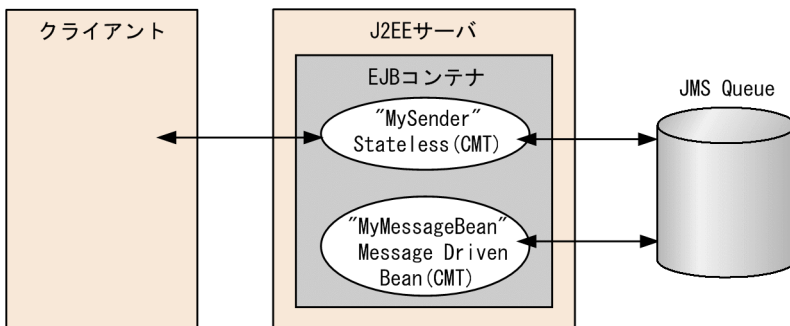
図 L-17 message の構成
