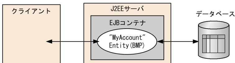
図 L-2 account の構成
