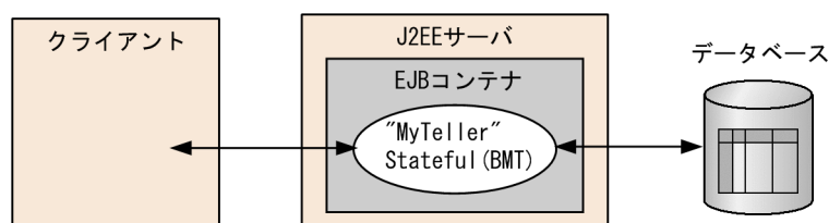
図 L-23 teller の構成
