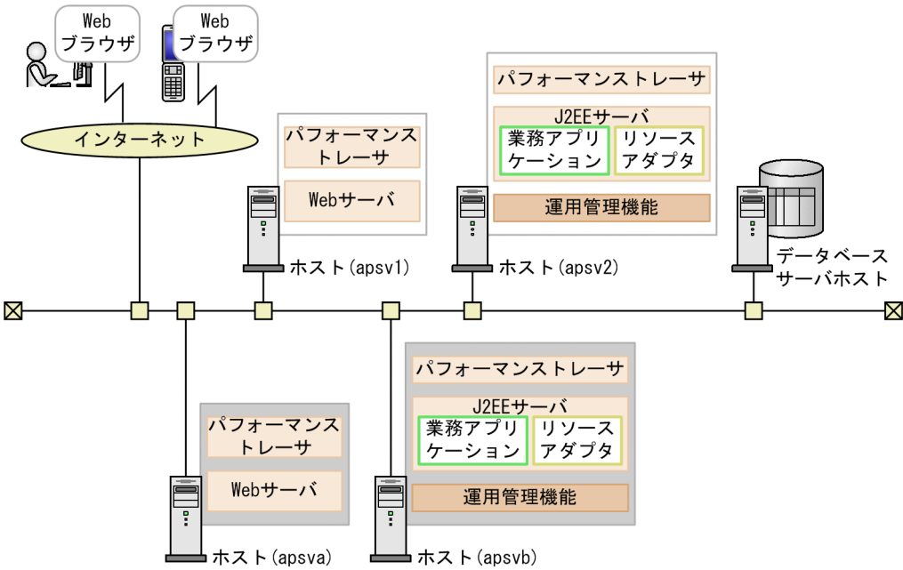
図 4-8 構成・定義情報を入力してほかのホストにシステム環境を移行するシステム運用例
