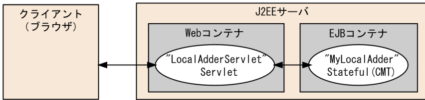
図 L-15 localadder の構成
