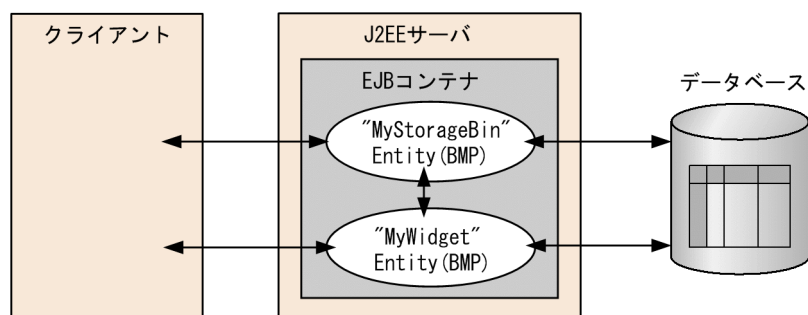
図 L-22 storagebin の構成
