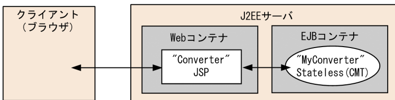
図 L-11 jsptag の構成
