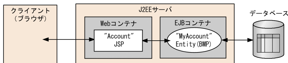
図 L-13 jsptobean の構成
