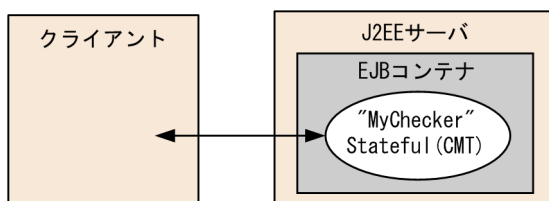
図 L-7 checker の構成
