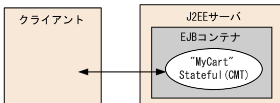
図 L-6 cart の構成
