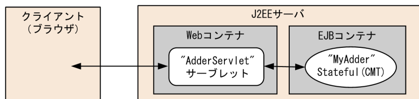
図 L-3 adder の構成
