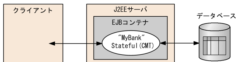
図 L-5 bank の構成
