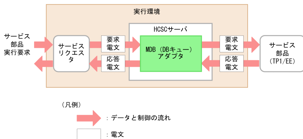
図 9-17 MDB (DB キュー) アダプタからのサービス部品実行
