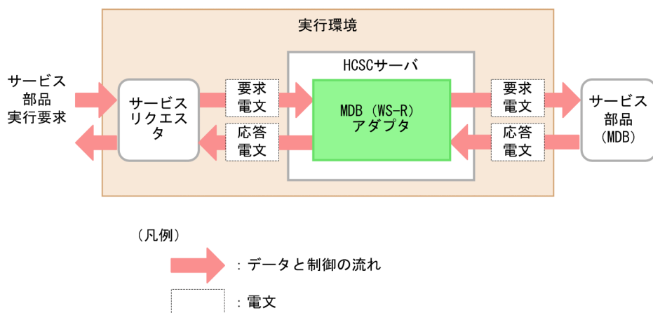
図 9-16 MDB (WS-R) アダプタからのサービス部品実行
