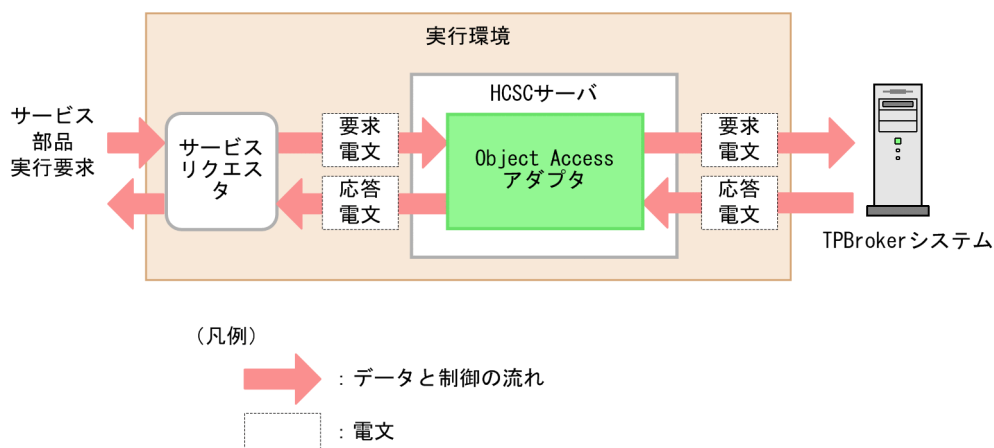
図 9-21 Object Access アダプタからのサービス部品実行
