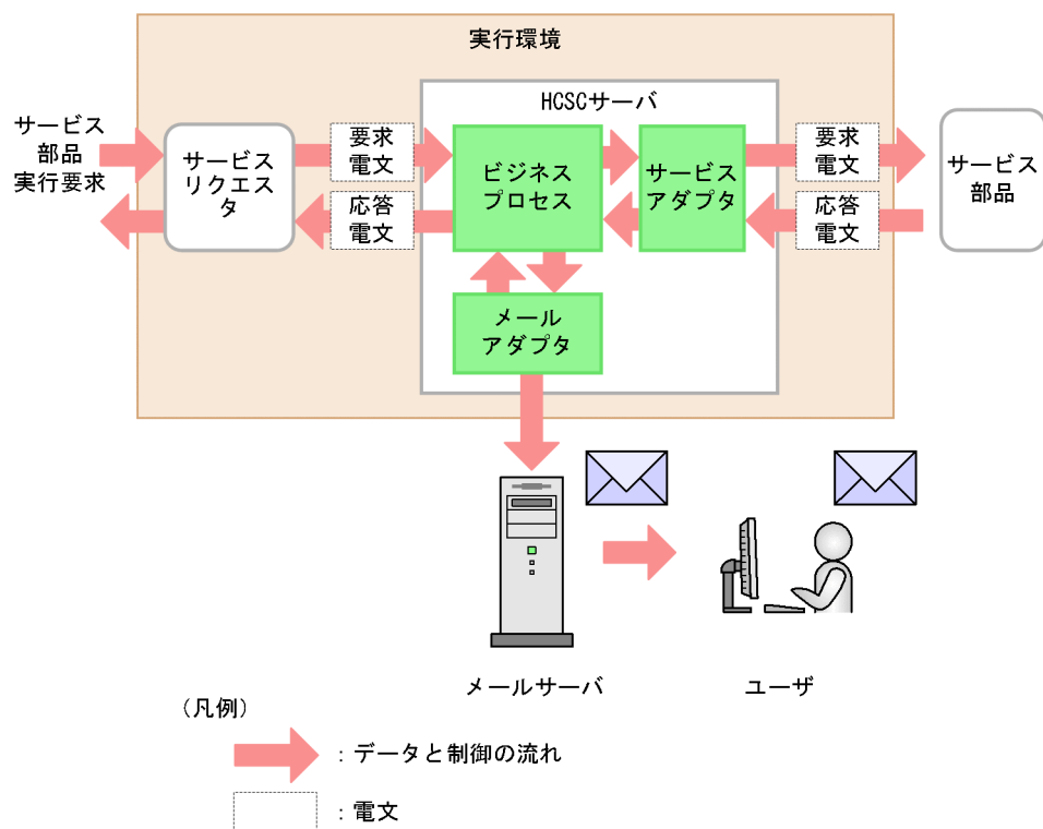
図 9-25 メールアダプタからのメールの送信
