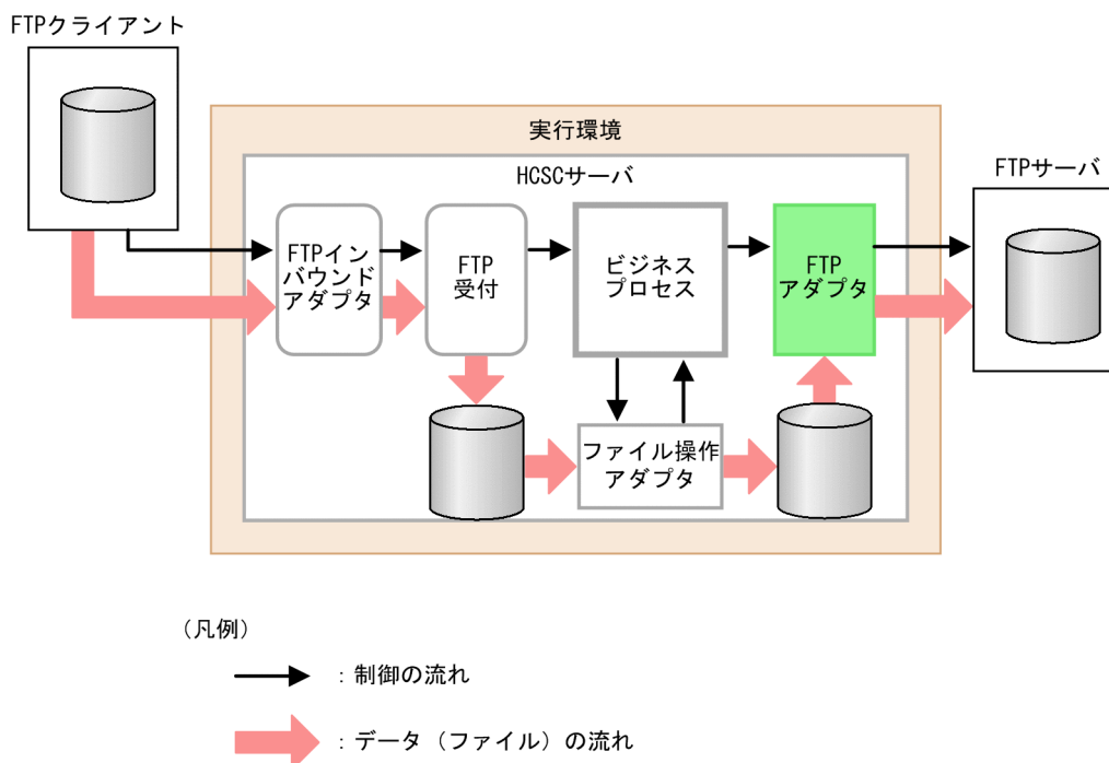
図 9-23 FTP アダプタと FTP サーバとの間のファイルの送受信
