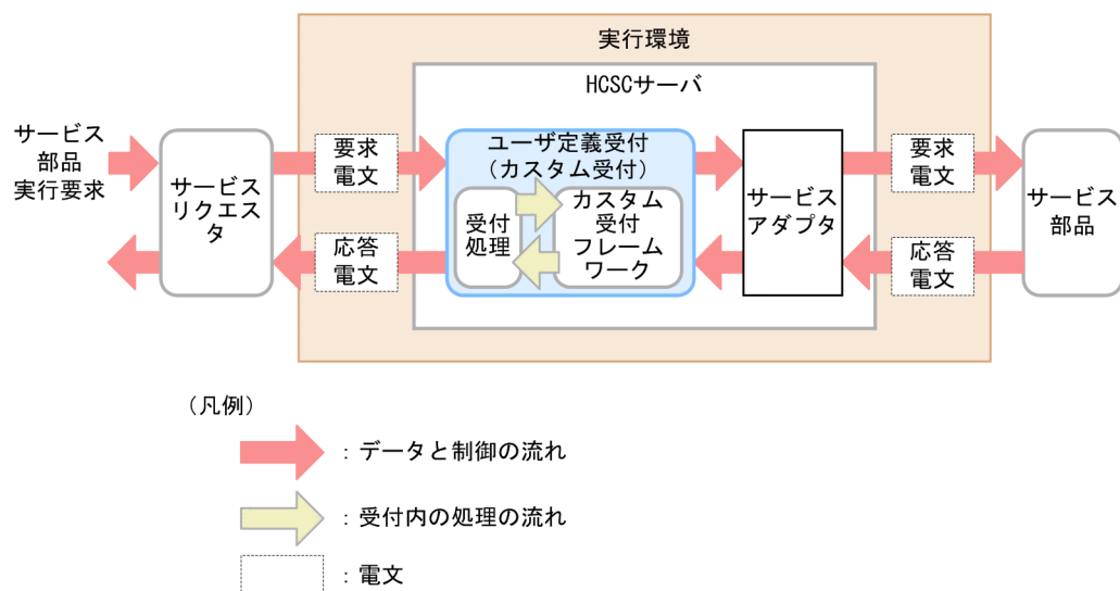
図 9-13 カスタム受付を使用したサービス部品の実行
