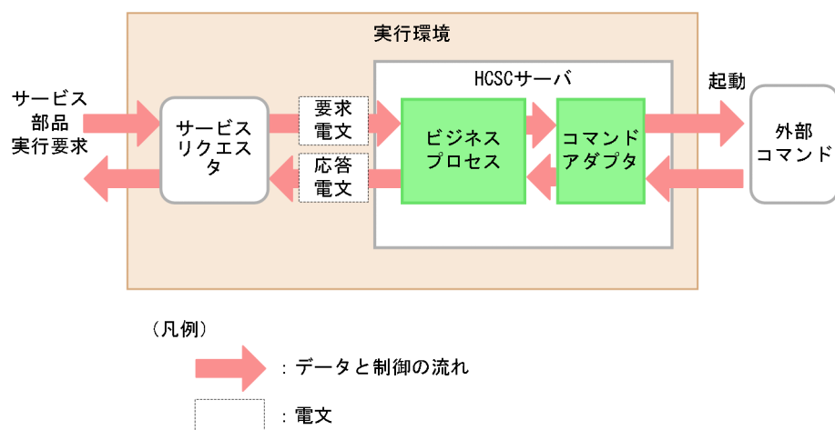
図 9-27 コマンドアダプタからのサービス部品実行
