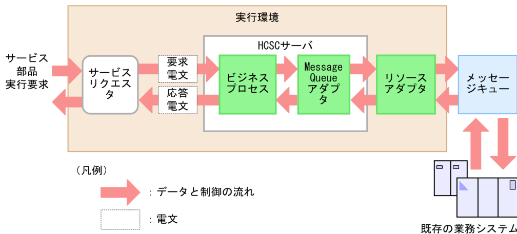
図 9-22 Message Queue アダプタからのメッセージキュー制御
