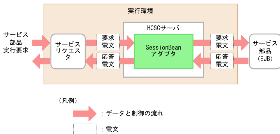
図 9-15 SessionBean アダプタからのサービス部品実行
