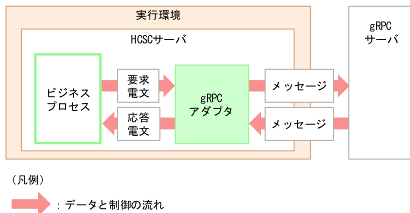
図 9-30 gRPC アダプタと gRPC サーバとのメッセージの送受信
