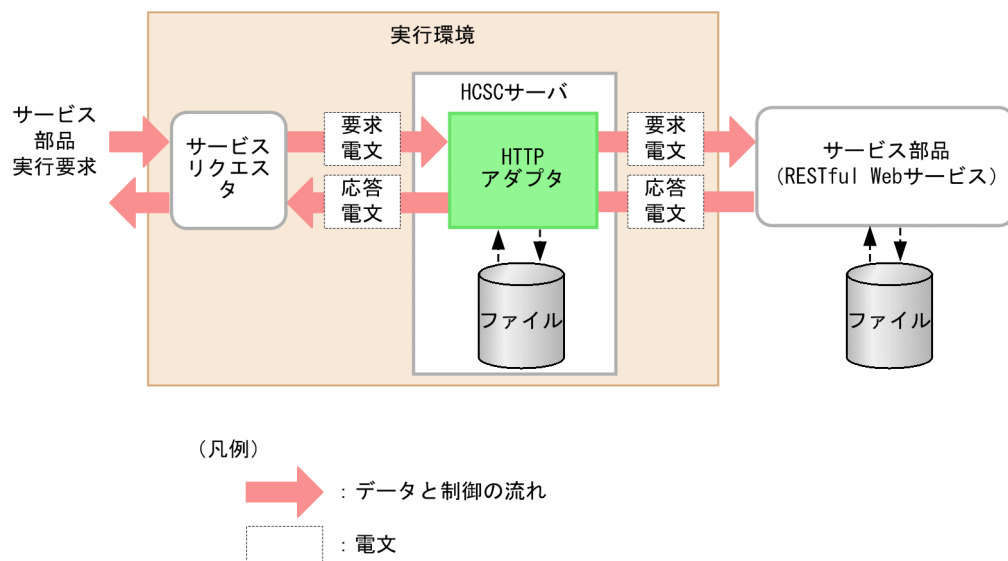
図 9-26 HTTP アダプタからのサービス部品実行
