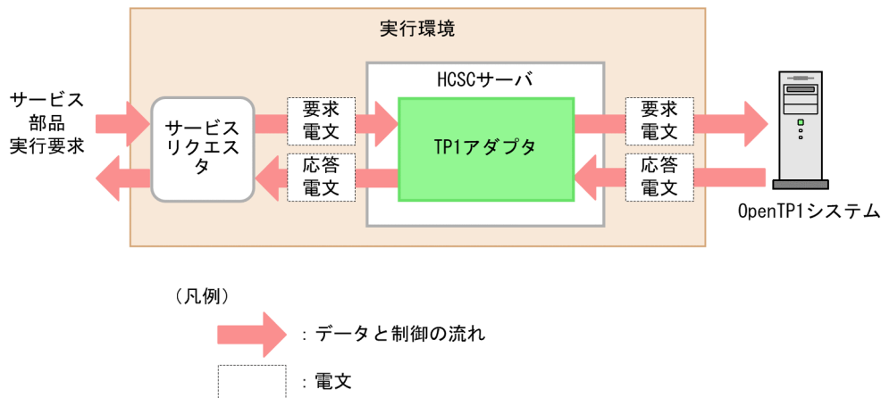
図 9-19 TP1 アダプタからのサービス部品実行
