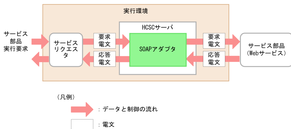
図 9-14 SOAP アダプタからのサービス部品実行
