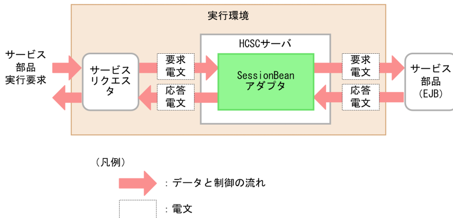
図 9-14 SessionBean アダプタからのサービス部品実行
