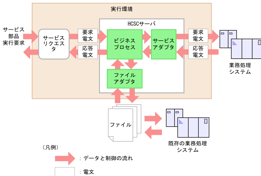
図 9-19 ファイルアダプタからのファイルの入出力
