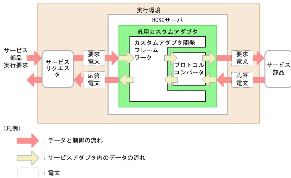
図 9-29 汎用カスタムアダプタからのサービス部品の実行
