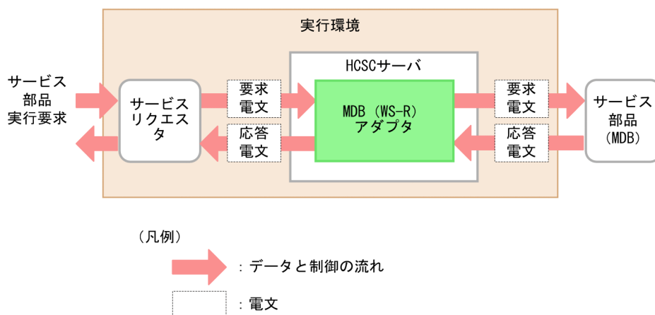
図 9-15 MDB (WS-R) アダプタからのサービス部品実行
