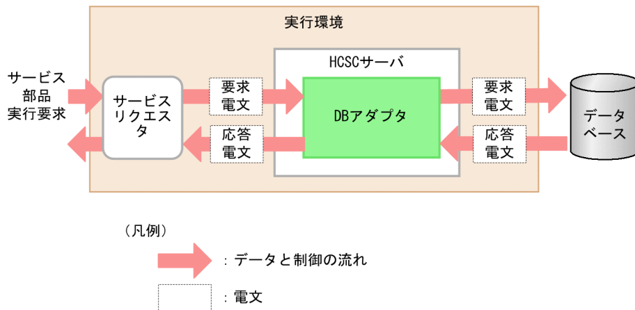
図 9-17 DB アダプタからの SQL 実行
