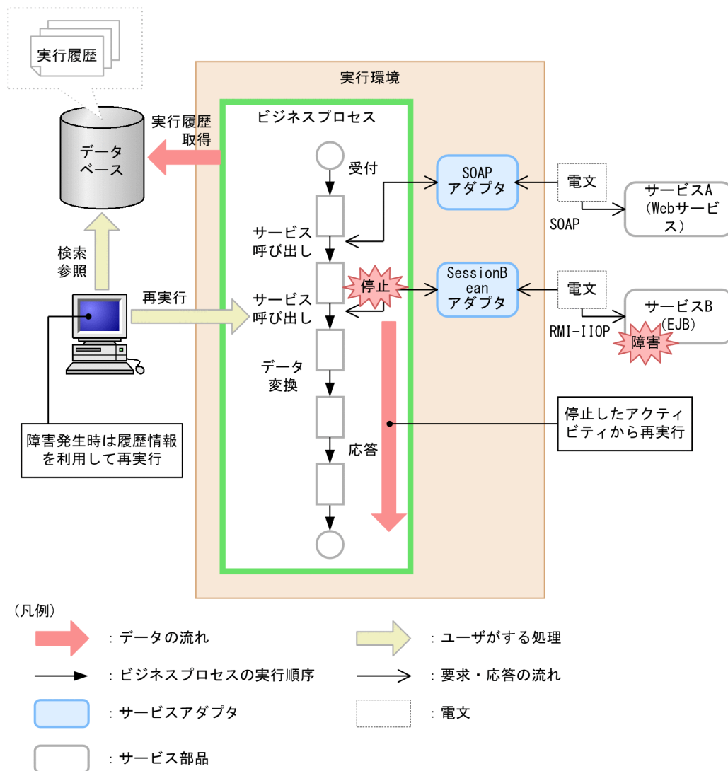
図 9-30 プロセスインスタンスの実行履歴の管理機能
