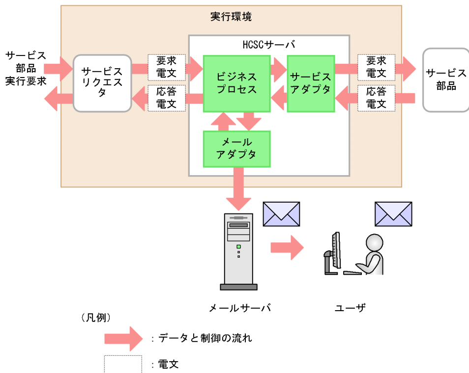
図 9-24 メールアダプタからのメールの送信
