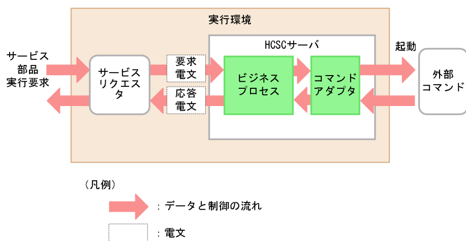
図 9-26 コマンドアダプタからのサービス部品実行
