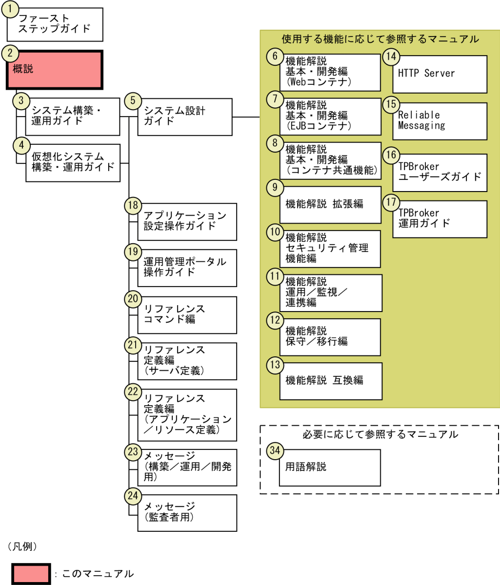
図 3-1 アプリケーションサーバのマニュアル体系（主に実行環境を構築・運用する場合に参照するマニュアル）
