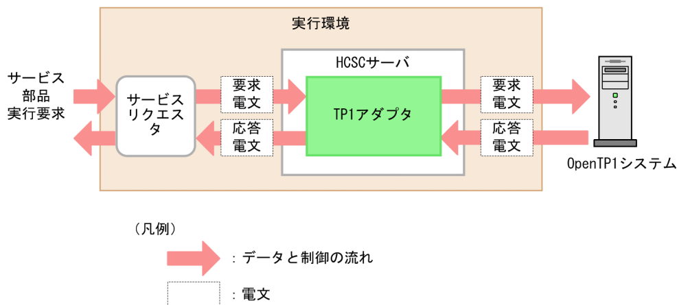
図 9-18 TP1 アダプタからのサービス部品実行
