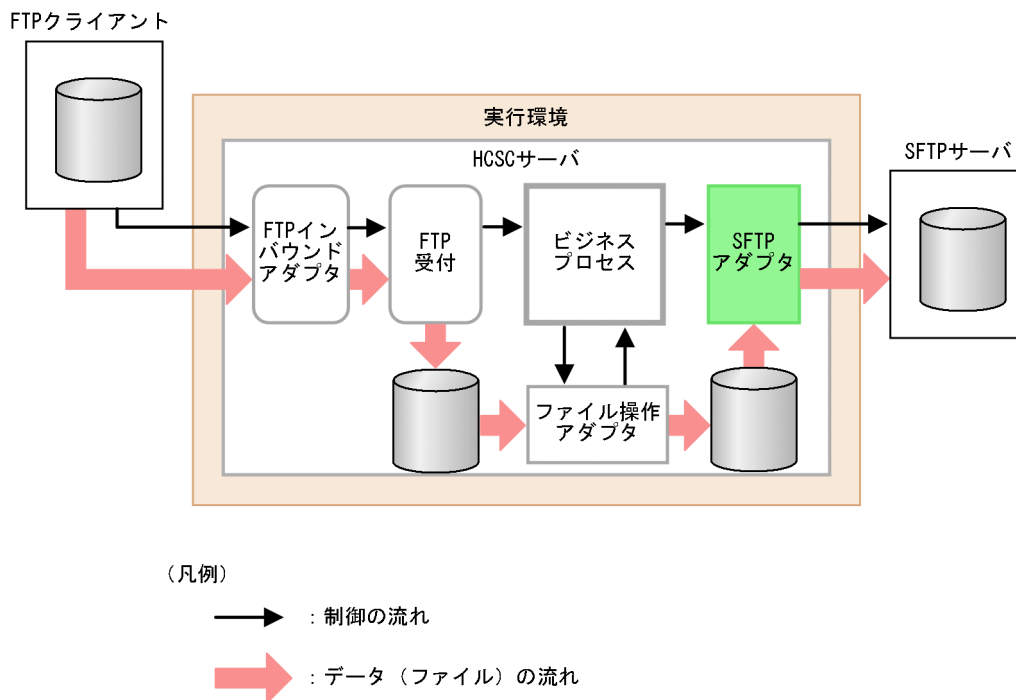
図 9-27 SFTP アダプタから SFTP サーバへのファイル送信
