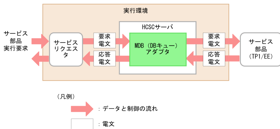
図 9-16 MDB (DB キュー) アダプタからのサービス部品実行
