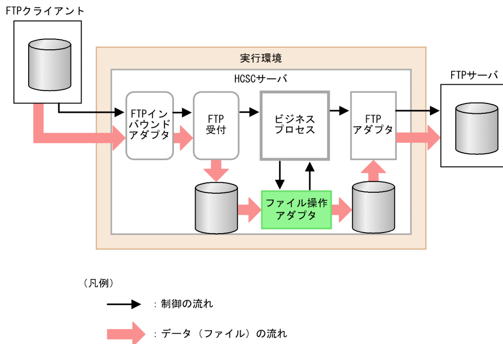
図 9-23 ファイル操作アダプタからのファイルの操作
