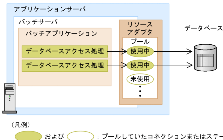
図 4-12 コネクションプールまたはステートメントプールを使用したデータベースアクセスの概要
