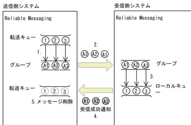
図 2-20 配送保証の仕組み
