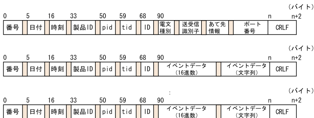
図 9-6 不正イベントトレース出力時の共用キューイベントトレースの出力形式
