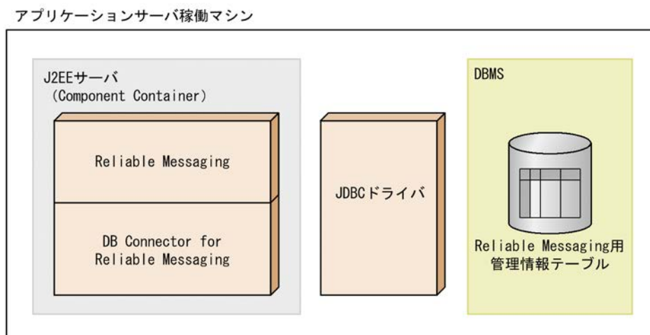
図 C-1 前提となるマシンとソフトウェア構成
