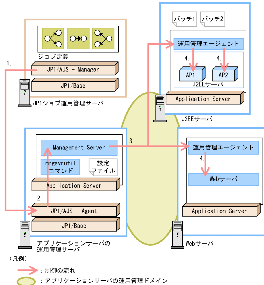
図 14-5 論理サーバおよび J2EE アプリケーションの起動と停止を自動化した場合の処理の流れ
