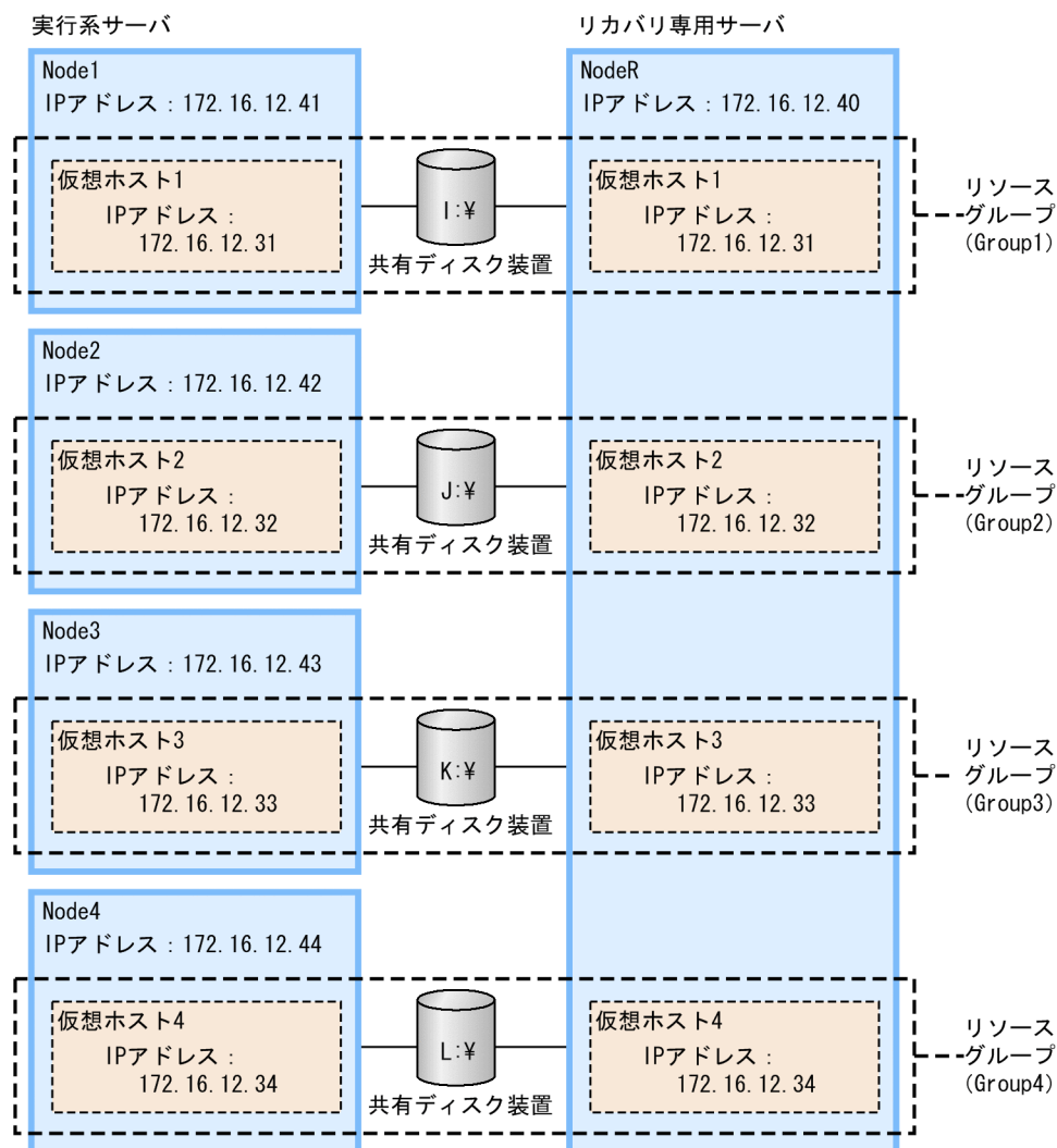
図 19-4 リソースグループの例
