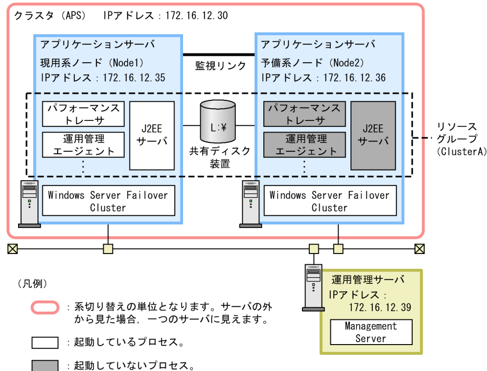
図 17-8 アプリケーションサーバを対象にした 1:1 系切り替えシステムの構成例 (Windows の場合)
