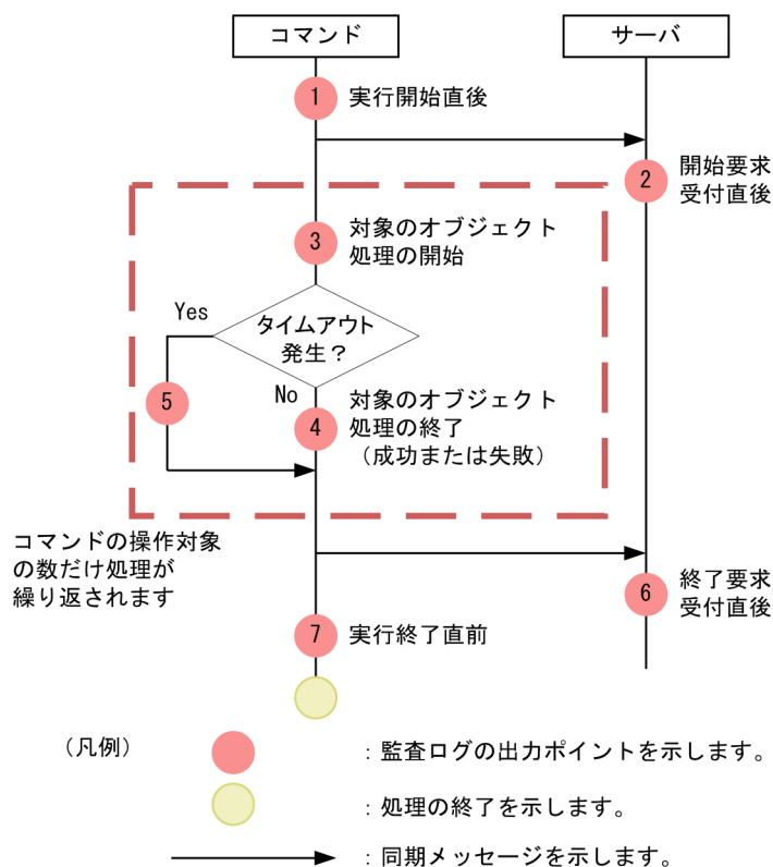
図 6-6 監査ログの出力ポイント（cjresetv 以外のサーバ管理コマンド）
