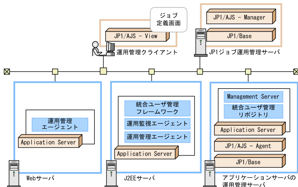
図 14-3 JP1/AJS と連携してシステムの自動運転をする場合のシステム構築例 (J2EE サーバの場合)
