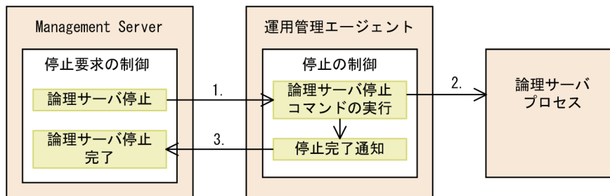
図 2-2 論理サーバの停止
