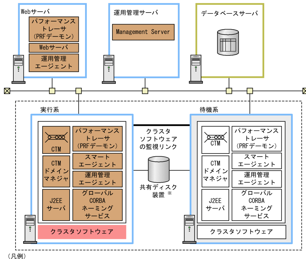
図 17-1 アプリケーションサーバを 1:1 系切り替えシステムで運用する場合のシステム構成例
