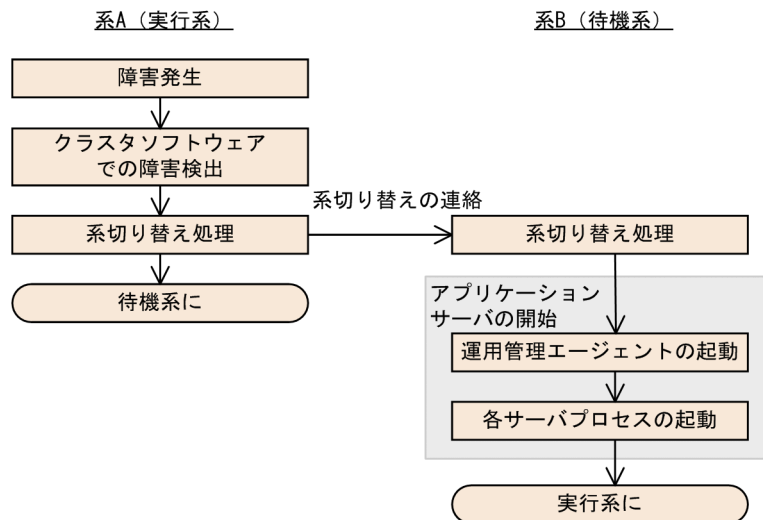
図 17-4 アプリケーションサーバの 1:1 系切り替えシステムでの自動系切り替えの処理の流れ
