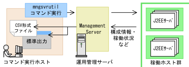
図 8-1 稼働情報のファイルへの出力の流れ
