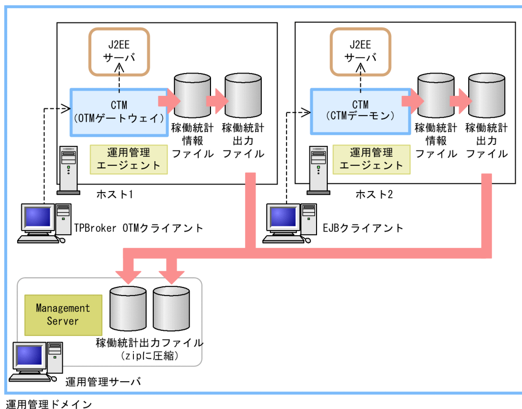
図 10-1 CTM の稼働統計情報の収集の概要
