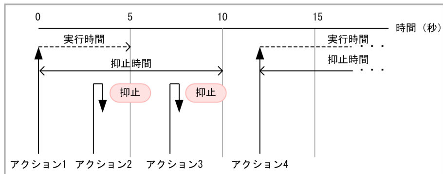
図 9-2 Management アクションの制御例 1
