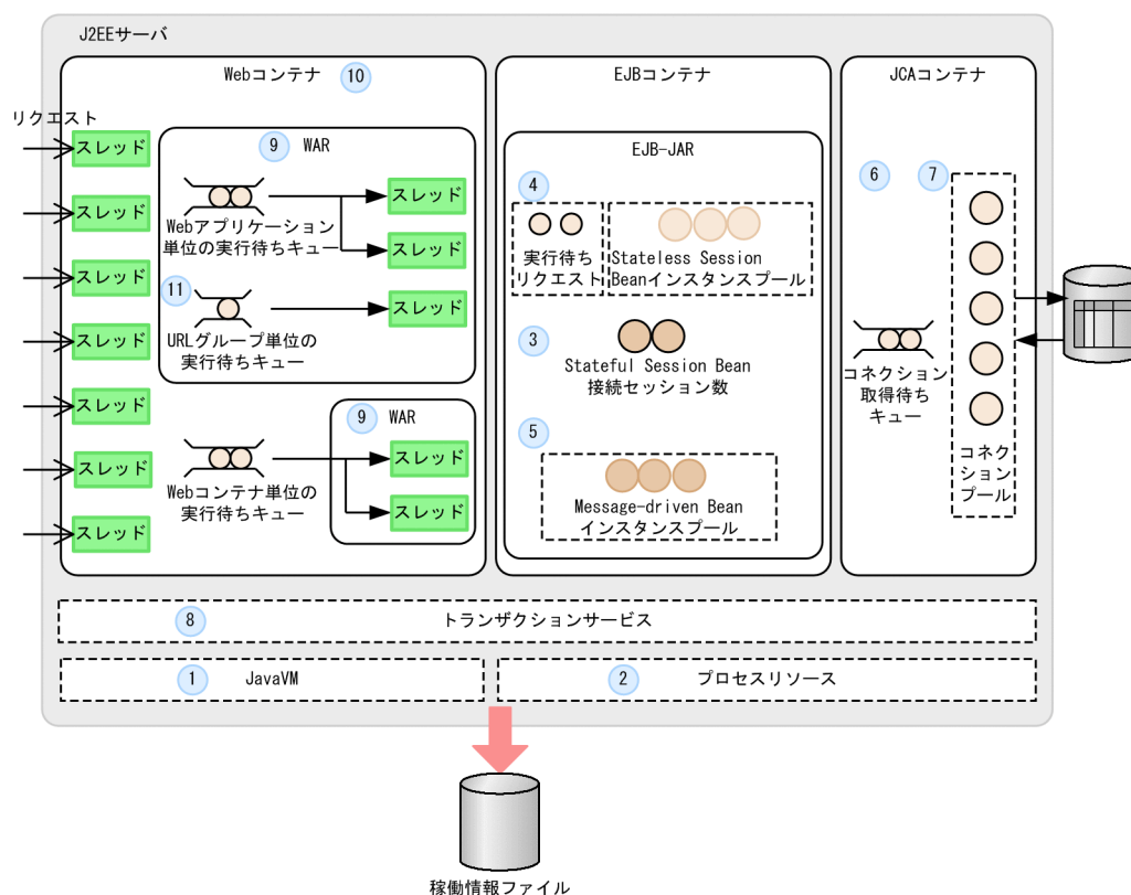
図 3-1 稼働情報の種類と稼働情報を出力する J2EE サーバの機能
