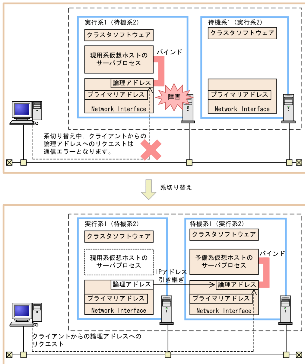
図 18-2 相互系切り替えシステムでの系切り替えの動作
