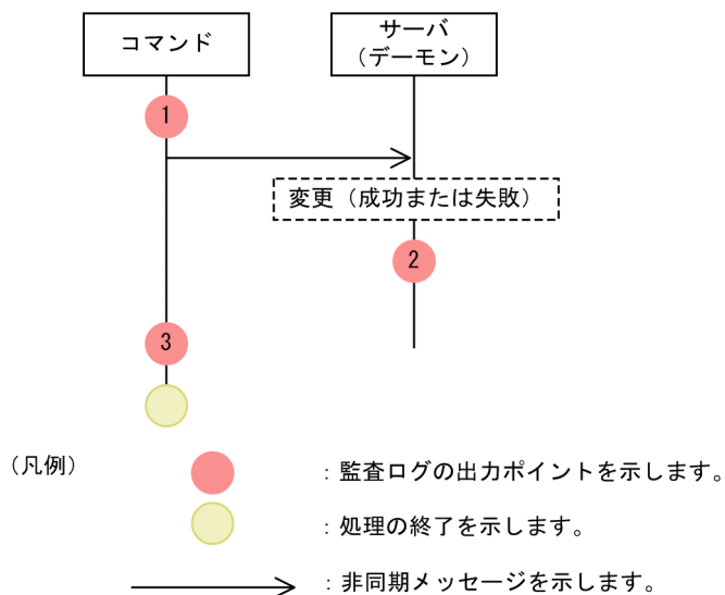
図 6-13 監査ログの出力ポイント（プロセスへの通信・共有メモリへのアクセスを実行するコマンド）
