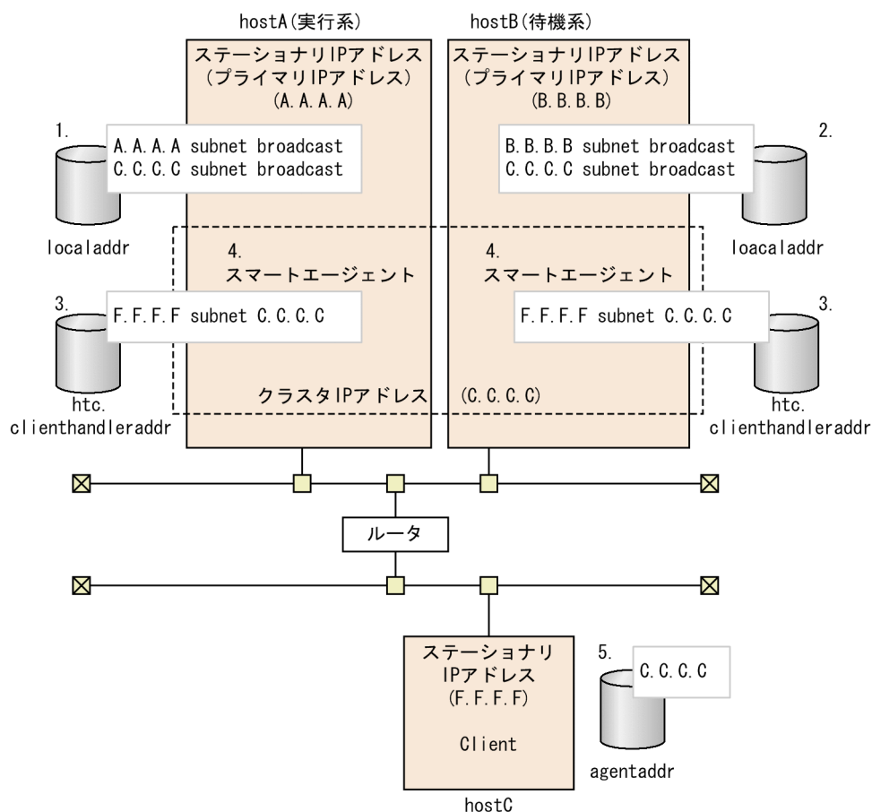
図 A-1 スマートエージェントをフェイルオーバーの対象にする場合の IP アドレスの設定例
