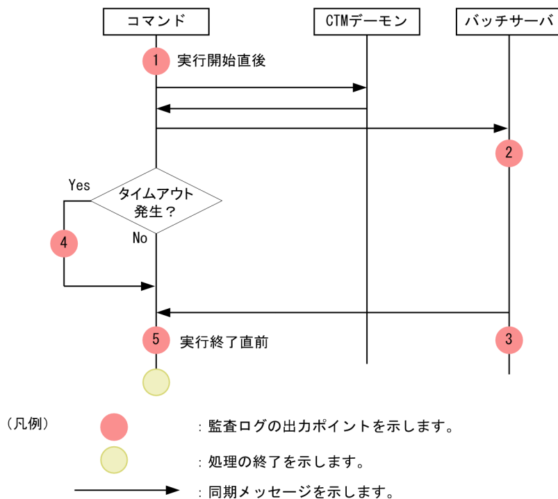
図 6-10 監査ログの出力ポイント (cjkiljob コマンド)
