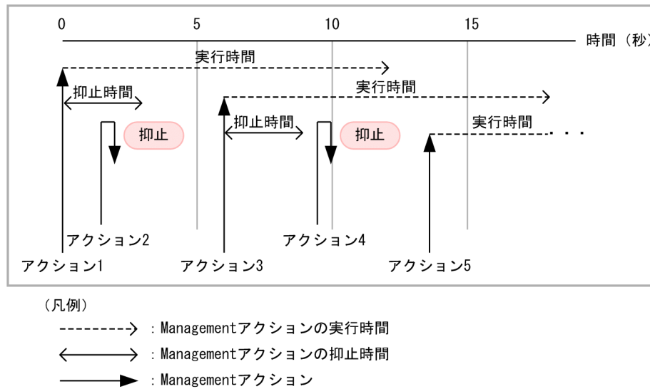
図 9-4 Management アクションの制御例 3
