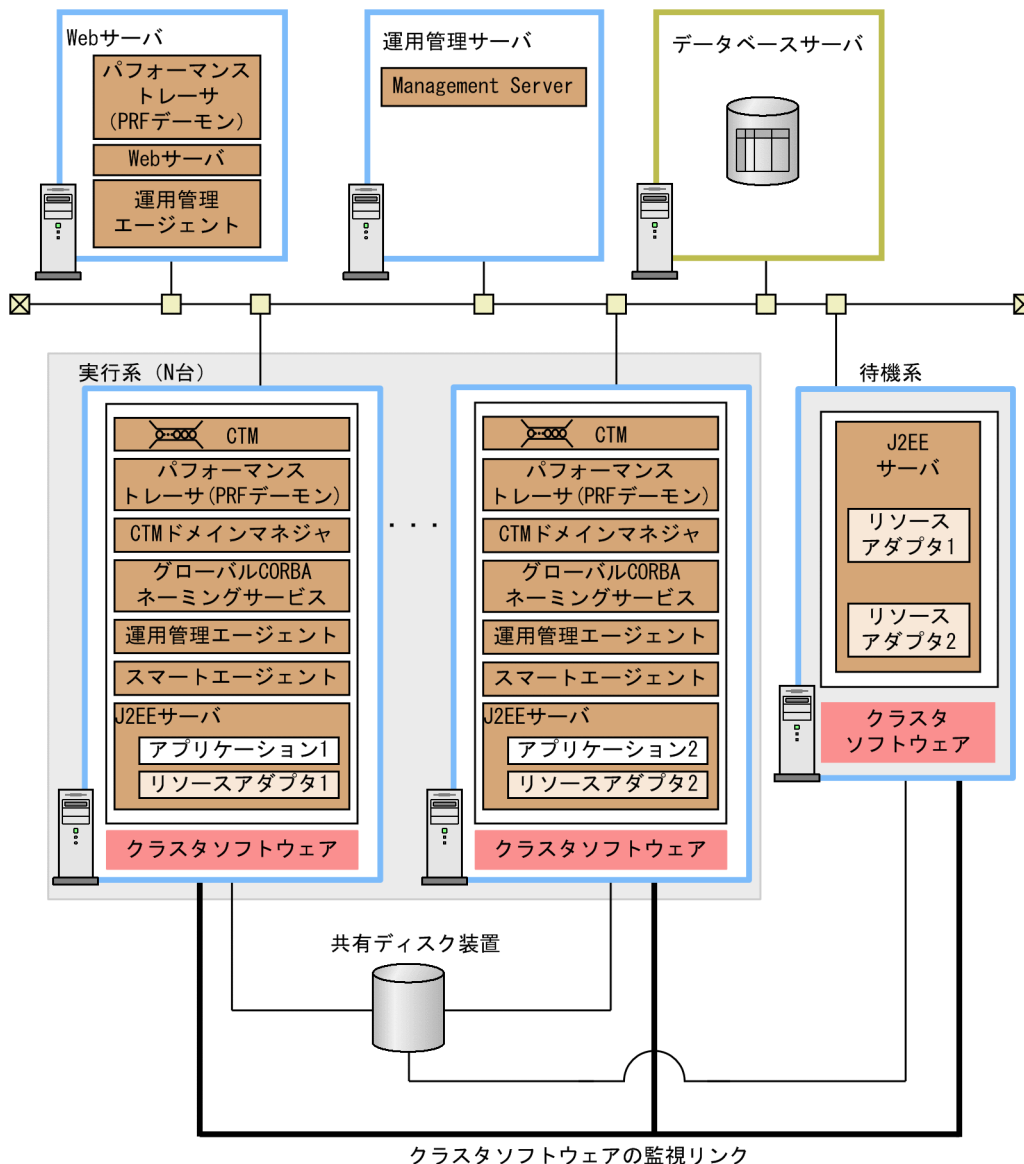
図 19-1 N:1 リカバリシステムのシステム構成例
