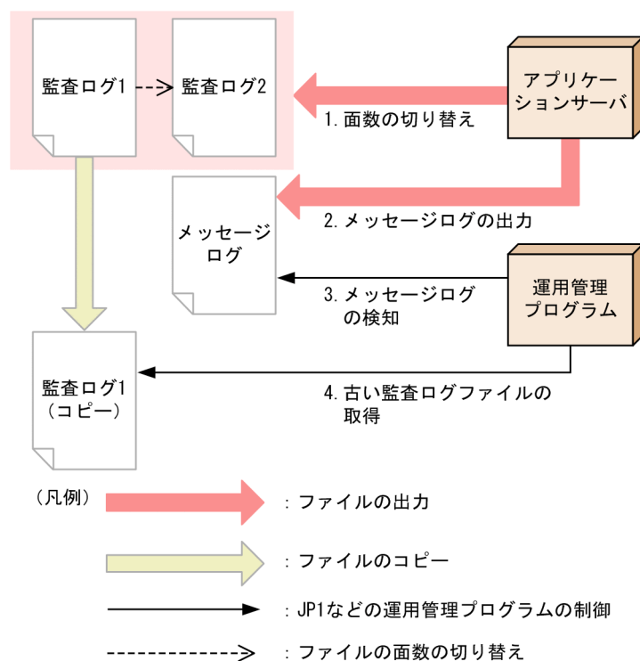
図 6-3 JP1 などの運用管理プログラムを使用して監査ログを自動でアーカイブする流れ
