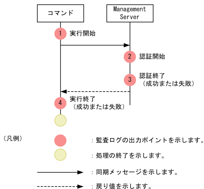
図 6-18 監査ログの出力ポイント（Management Server による承認処理を実行するコマンド）
