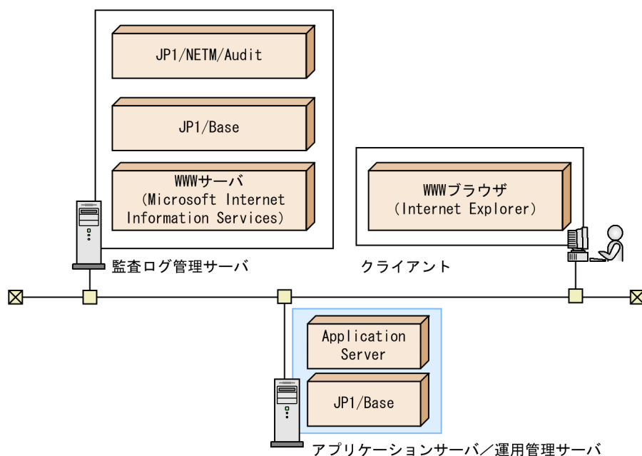
図 15-2 JP1/Audit Management - Manager と連携して監査ログの収集および一元管理をする場合のシステム構成例
