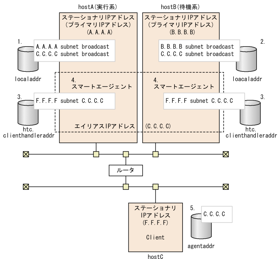
図 B-1 スマートエージェントを系切り替えの対象にする場合の IP アドレスの設定例
