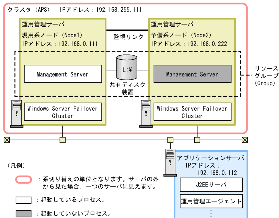
図 17-10 運用管理サーバを対象にした 1:1 系切り替えシステムの構成例（Windows の場合）
