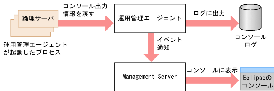
図 11-1 コンソール出力情報の取得
