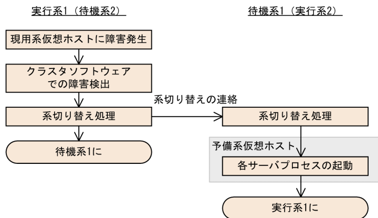
図 18-3 相互系切り替えシステムでの自動系切り替えの処理の流れ
