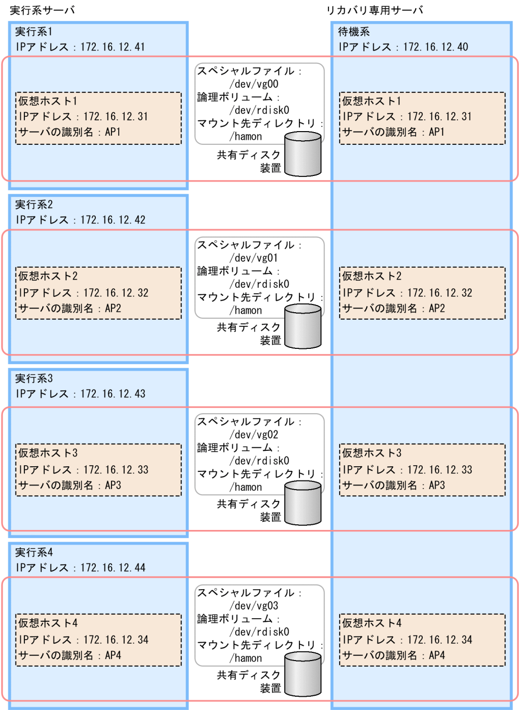
図 19-7 N:1 リカバリ構成での仮想ホストの構成例
