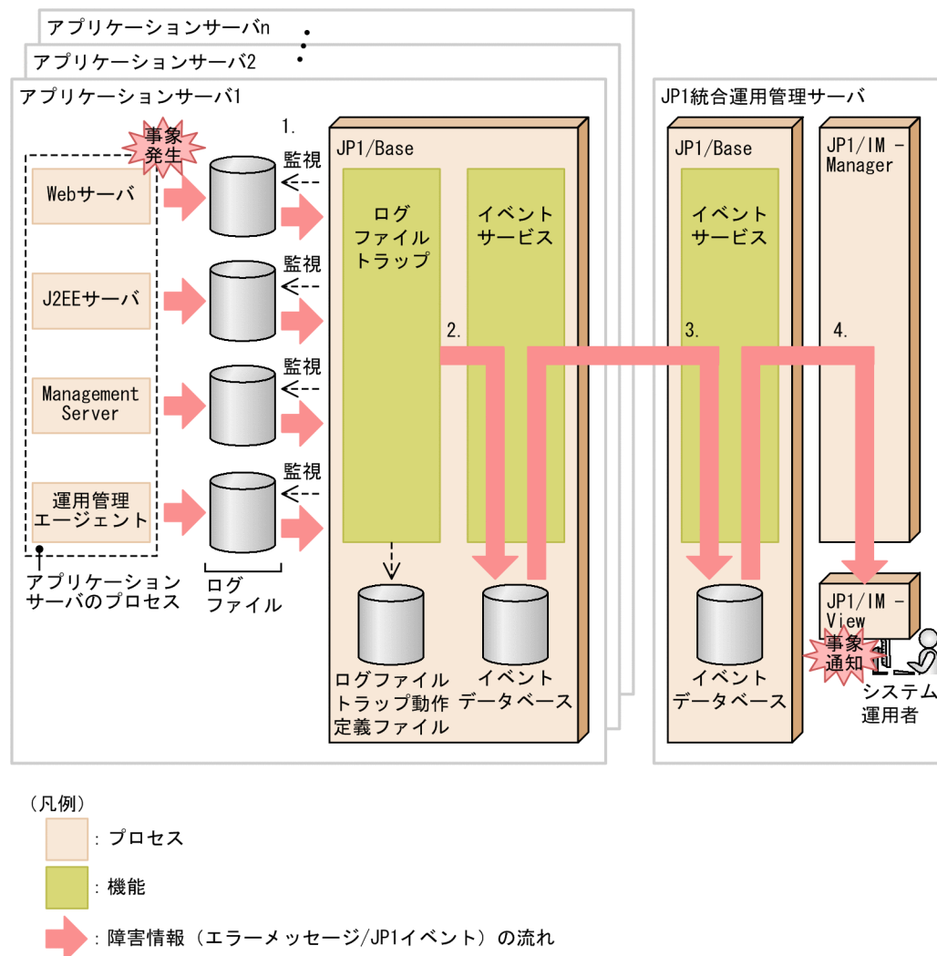
図 13-7 Web フロントシステムでのシステム構成と運用例（JP1/IM を使用したシステムの集中監視）
