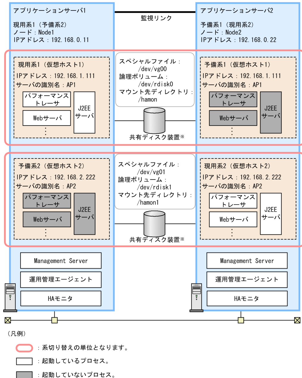
図 18-7 相互系切り替えシステムの構成例（UNIX の場合）
