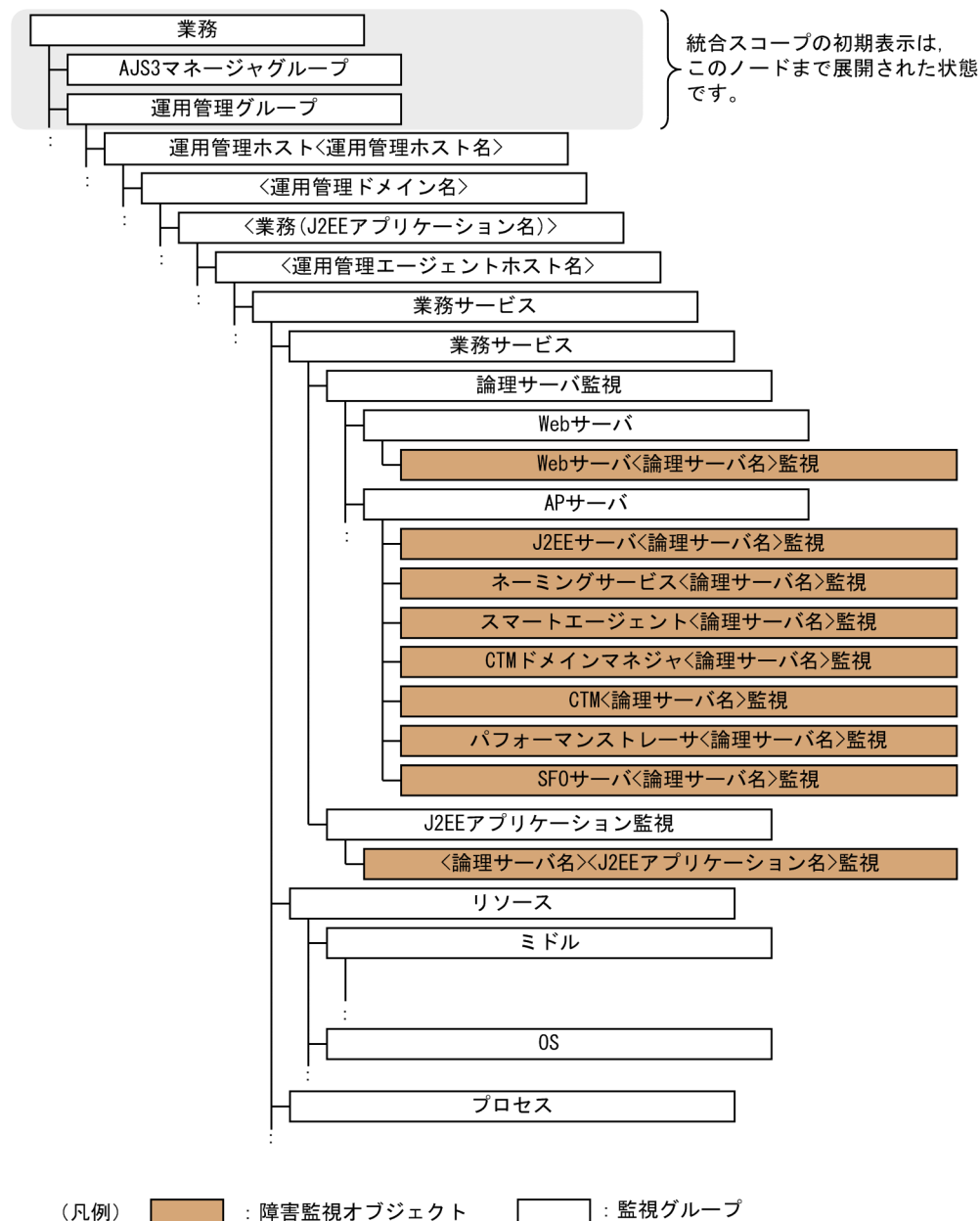
図 13-3 業務指向ツリーの構成
