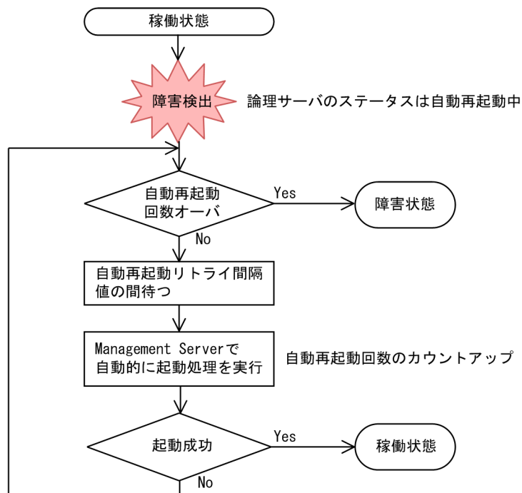
図 2-3 障害発生時の自動再起動
