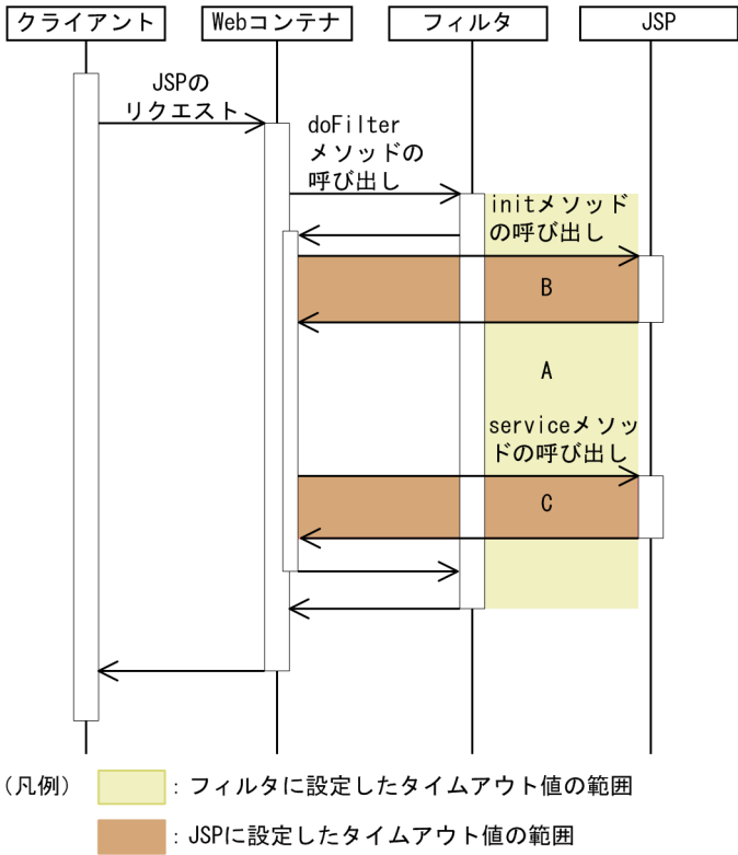
図 5-6 フィルタを経由した JSP の初回リクエストのタイムアウト設定
