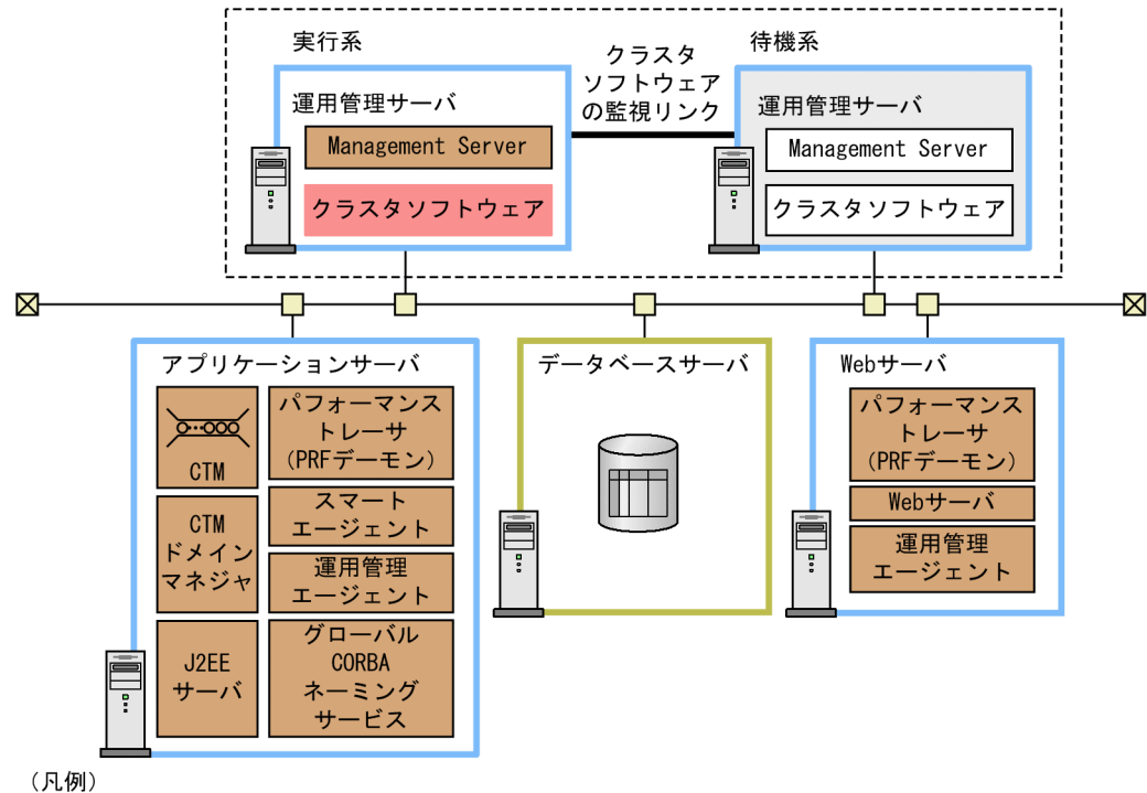
図 17-2 運用管理サーバを 1:1 系切り替えシステムで運用する場合のシステム構成例
