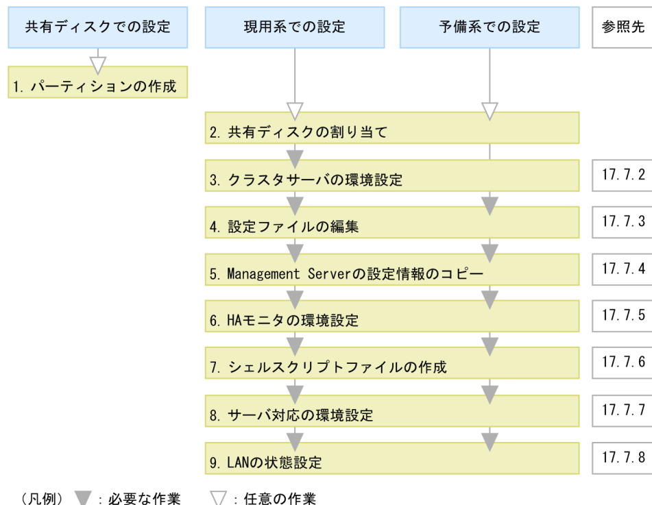
図 17-15 運用管理サーバを対象にした 1:1 系切り替えシステムの設定手順（UNIX の場合）
