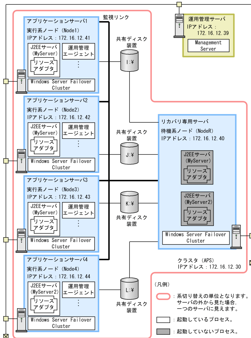
図 19-3 システムの構成例 (N:1 リカバリシステムの場合)
