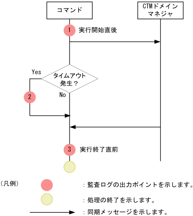
図 6-11 監査ログの出力ポイント（cjlistjob コマンド）
