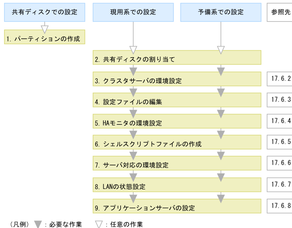
図 17-13 アプリケーションサーバを対象にした 1:1 系切り替えシステムの設定手順（UNIX の場合）
