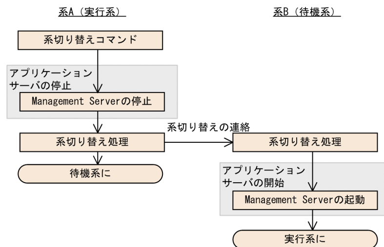
図 17-7 運用管理サーバの 1:1 系切り替えシステムでの計画系切り替えの処理の流れ
