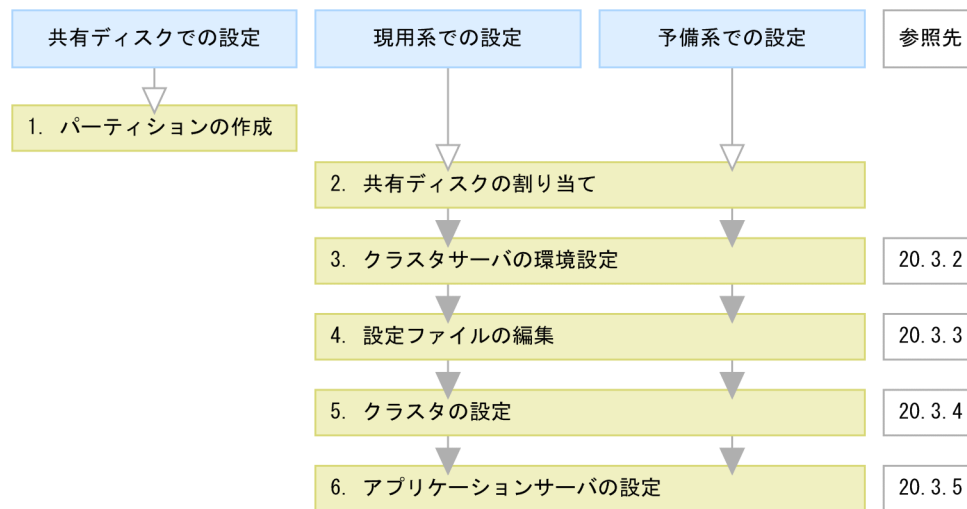
図 20-3 ホスト単位管理モデルを対象にした系切り替えシステムの設定手順
