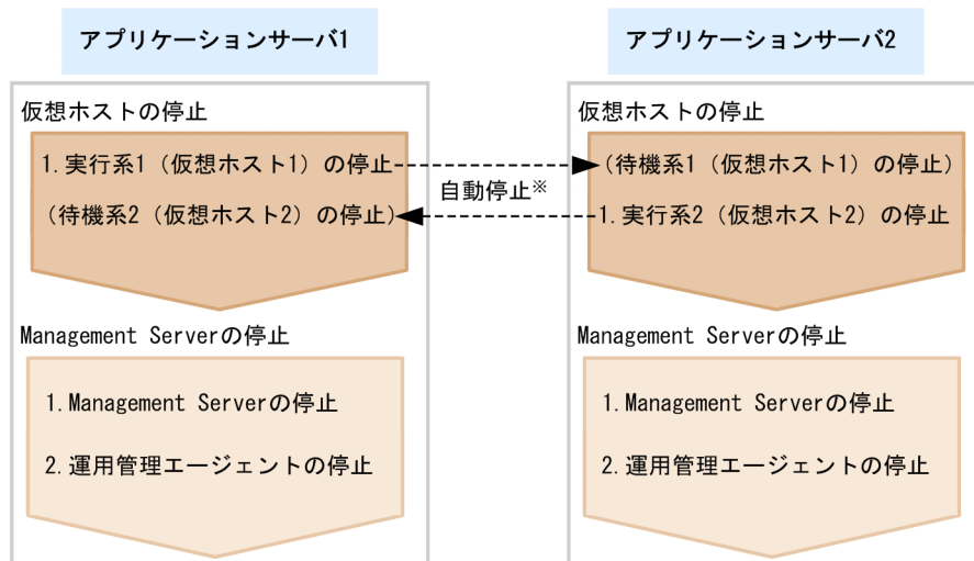
図 18-12 相互系切り替えシステムの停止の流れ
