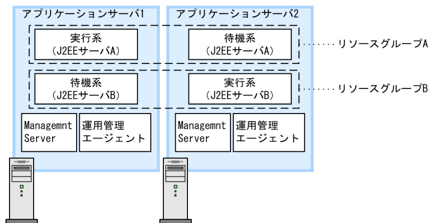
図 18-9 相互スタンバイシステムの構成例
