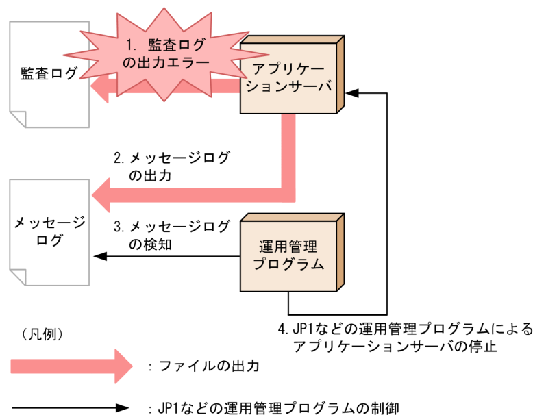
図 6-2 JP1 などの運用管理プログラムを使用して監査ログの出力に失敗した場合にシステムを自動で停止する流れ
