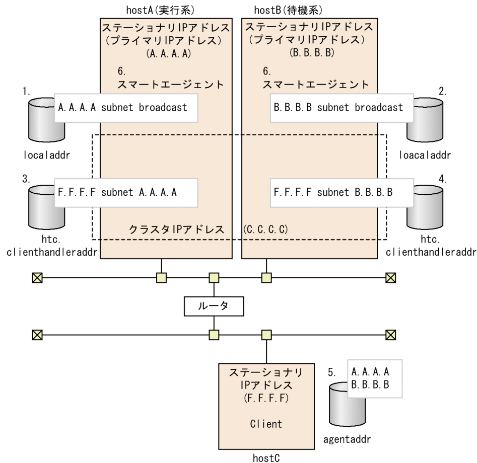
図 A-2 スマートエージェントをフェイルオーバーの対象にしない場合の IP アドレスの設定例
