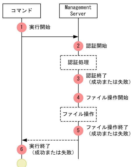
図 6-19 監査ログの出力ポイント（Management Server によるファイル操作を実行するコマンド）
