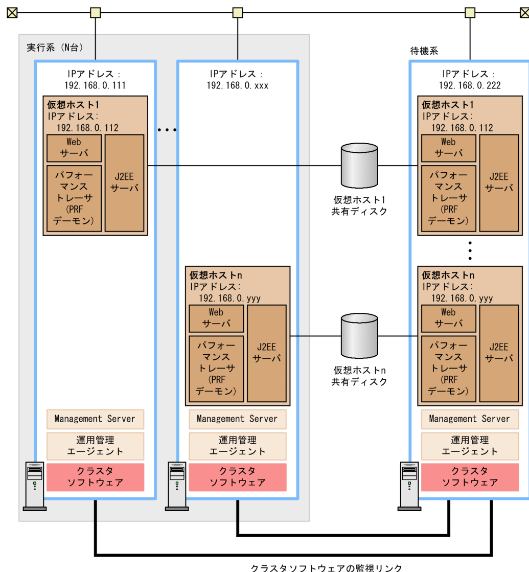
図 20-1 ホスト単位管理モデルを対象にした系切り替えシステムのシステム構成例
