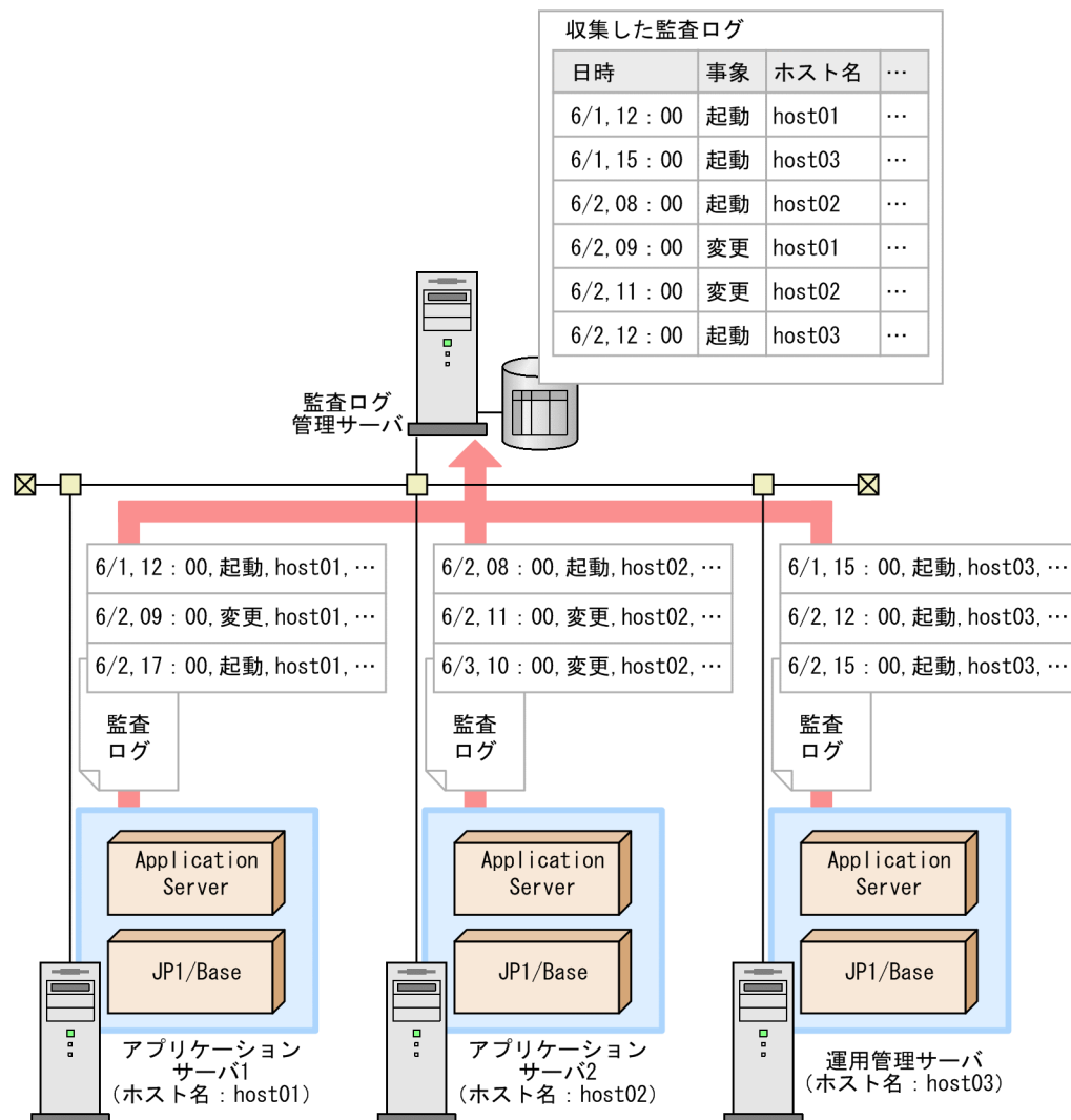
図 15-1 JP1/Audit Management - Manager を使用した監査ログの収集・一元管理の例
