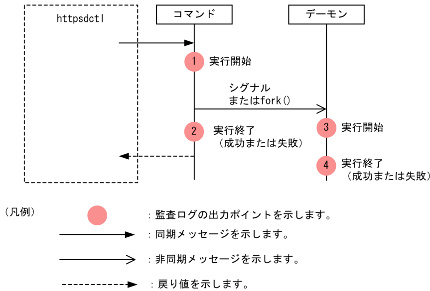
図 6-25 監査ログの出力ポイント (httpsdctl ユティリティから HTTP Server の起動・停止を実行するコマンド)
