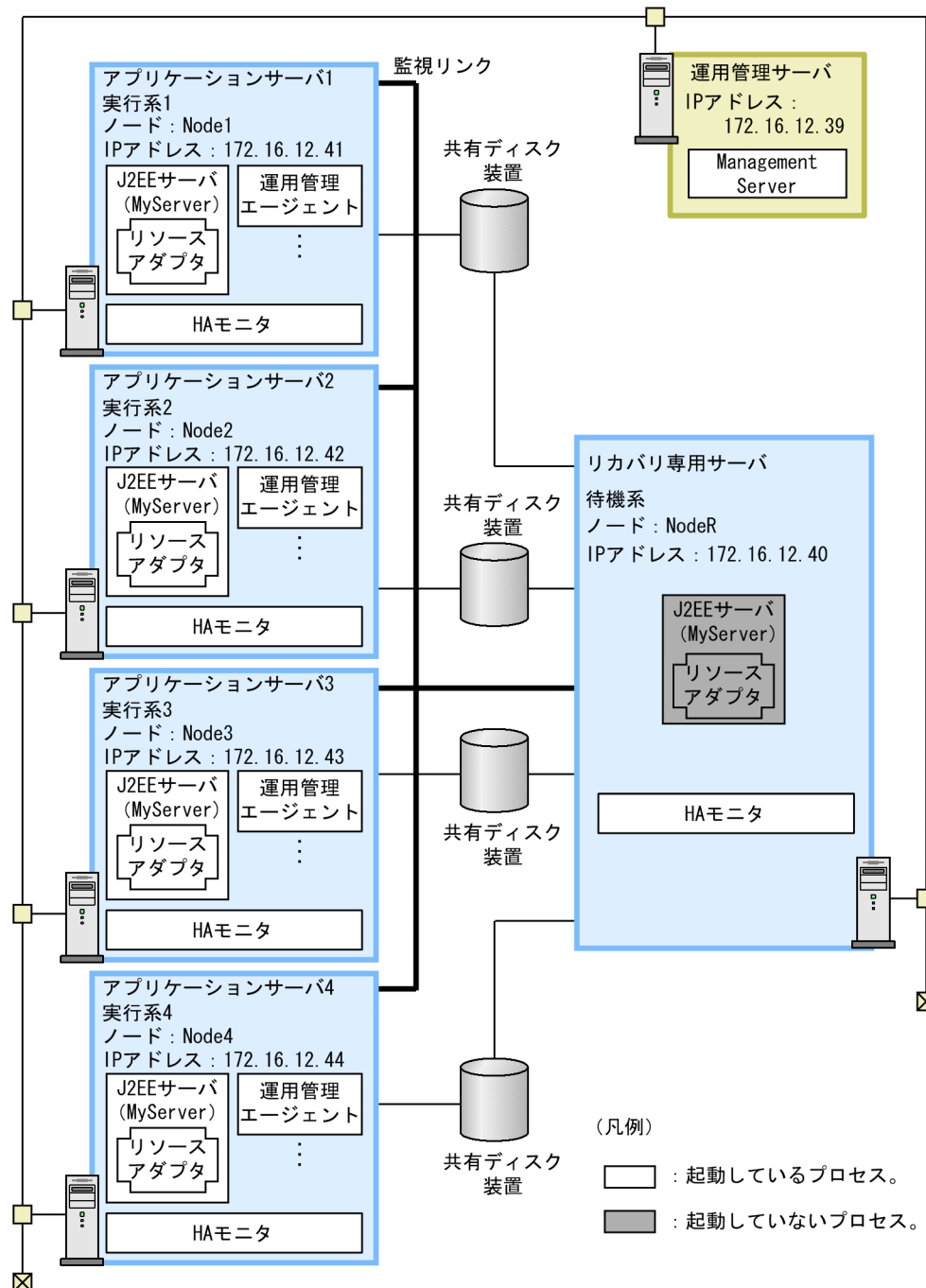
図 19-6 N:1 リカバリシステムの構成例 (UNIX の場合)
