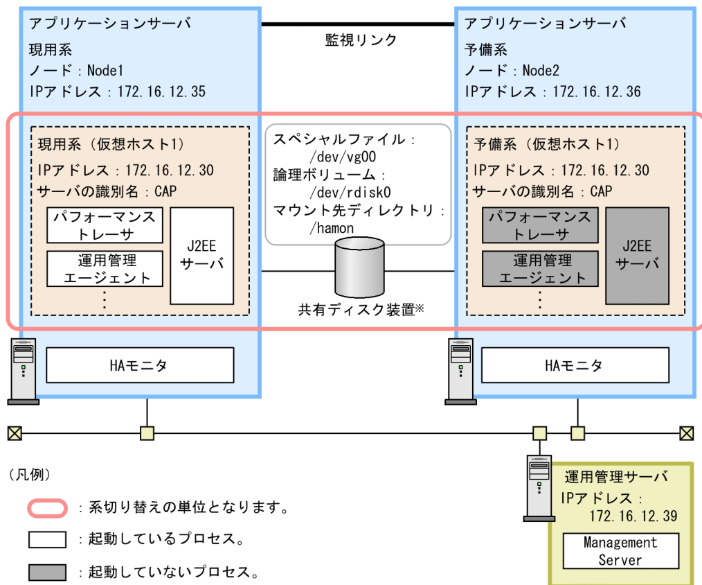
図 17-12 アプリケーションサーバを対象にした 1:1 系切り替えシステムの構成例（UNIX の場合）
