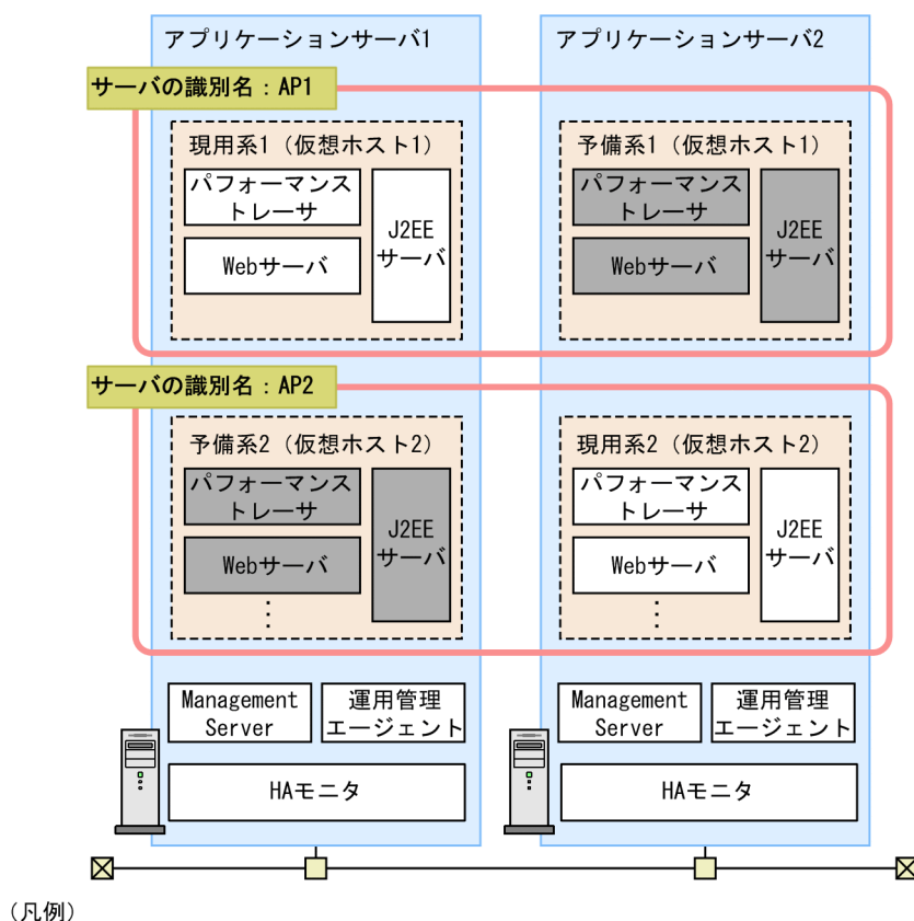
図 18-10 相互系切り替えシステムのシステム構成例
