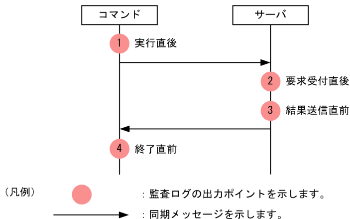
図 6-8 監査ログの出力ポイント（cjexecjob コマンド、cjkilljob コマンド、および cjlistjob コマンド）
