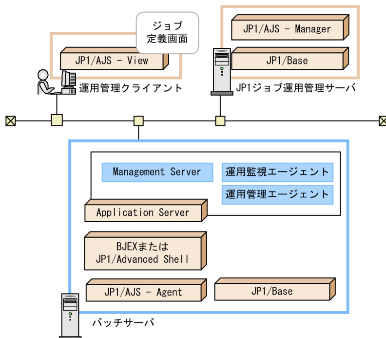
図 14-4 JP1/AJS と連携してシステムの自動運転をする場合のシステム構築例（バッチサーバの場合）
