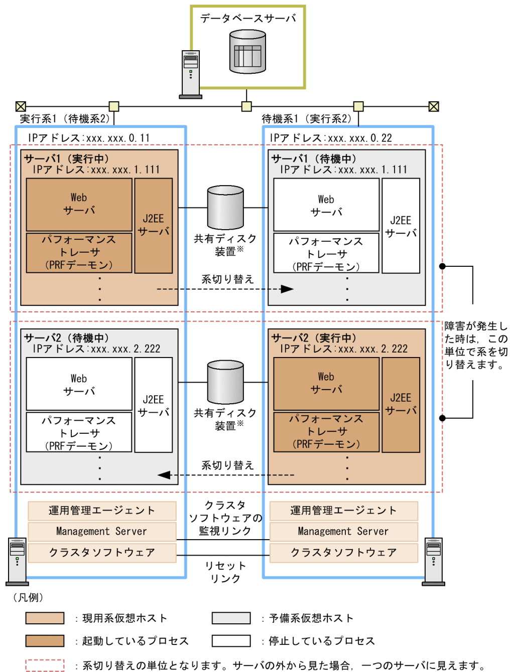
図 18-1 相互系切り替えシステムの構成例
