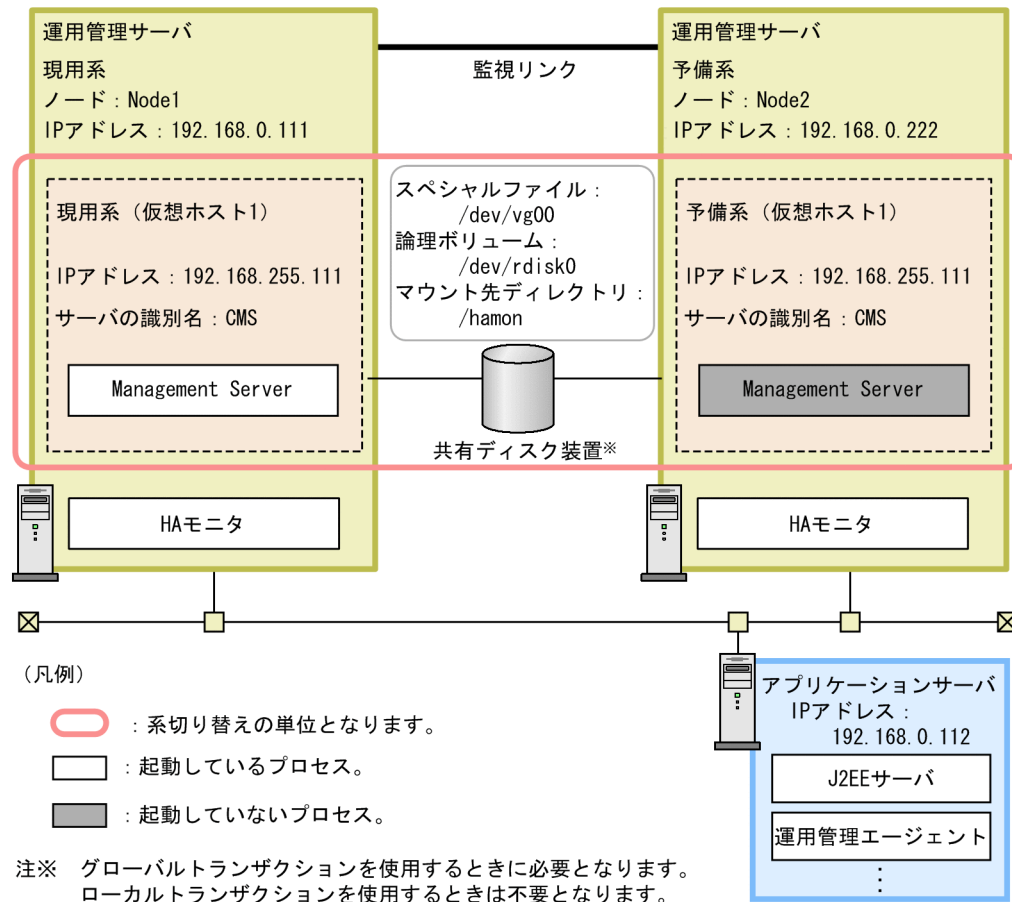
図 17-14 運用管理サーバを対象にした 1:1 系切り替えシステムの構成例 (UNIX の場合)
