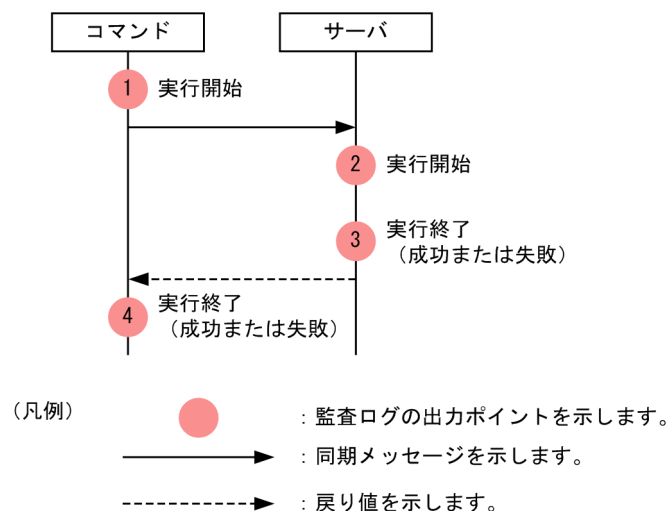
図 6-23 監査ログの出力ポイント（HTTP Server の起動・停止を実行するコマンド）
