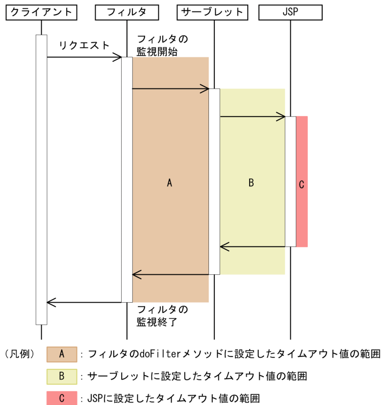
図 5-3 フィルタ/サーブレット/JSP 呼び出しのタイムアウト設定
