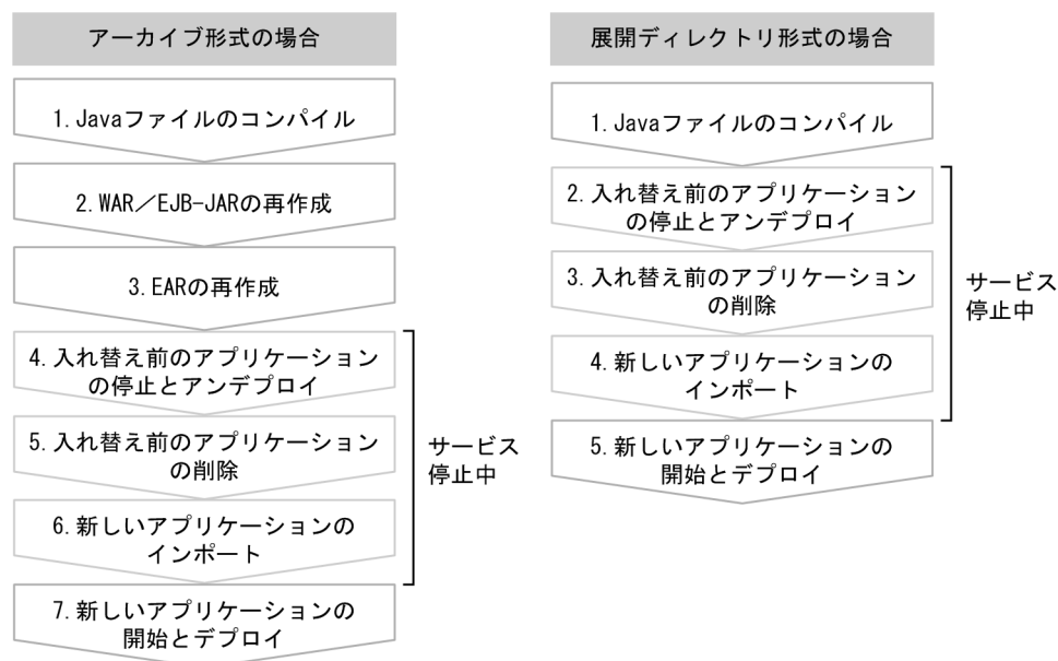
図 5-14 通常の J2EE アプリケーションの入れ替えの手順
