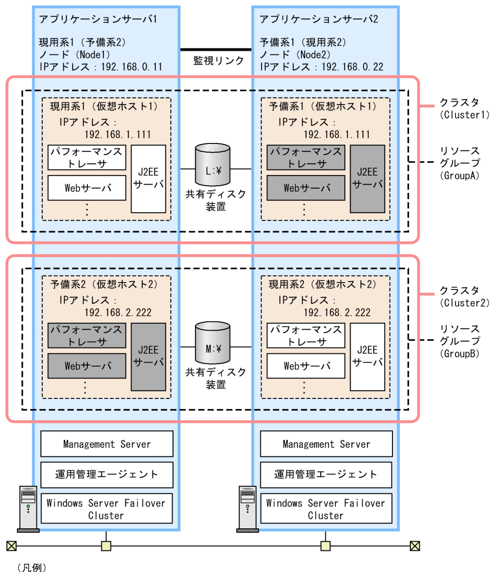
図 18-5 相互系切り替えシステムの構成例（Windows の場合）
