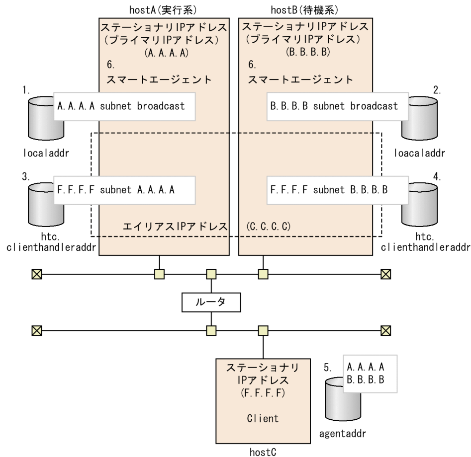
図 B-2 スマートエージェントを系切り替えの対象にしない場合の IP アドレスの設定例
