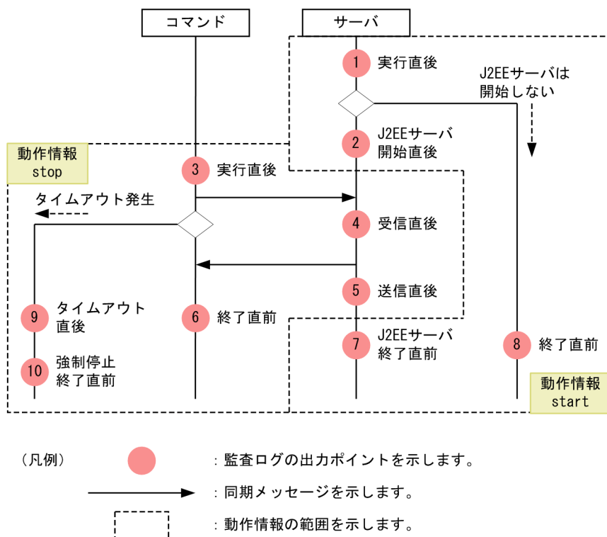
図 6-4 監査ログの出力ポイント（サーバプロセスを起動・停止する、サーバ管理コマンド以外のコマンド）
