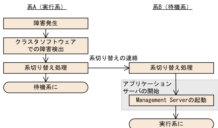
図 17-5 運用管理サーバの 1:1 系切り替えシステムでの自動系切り替えの処理の流れ
