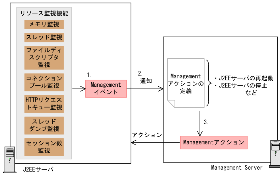
図 9-1 Management イベントと Management アクション
