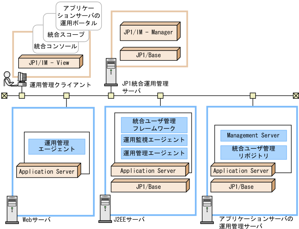
図 13-2 JP1/IM と連携してシステムの集中監視をする場合のシステム構成例
