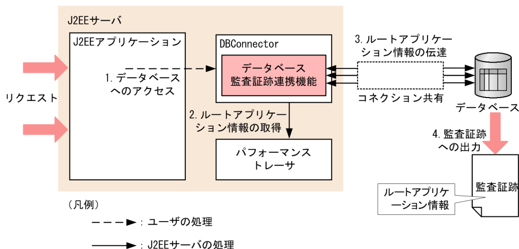
図 7-1 データベース監査証跡への情報の出力の流れ
