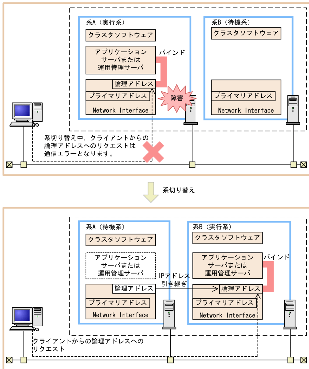
図 17-3 1:1 系切り替えシステムでの系切り替えの動作
