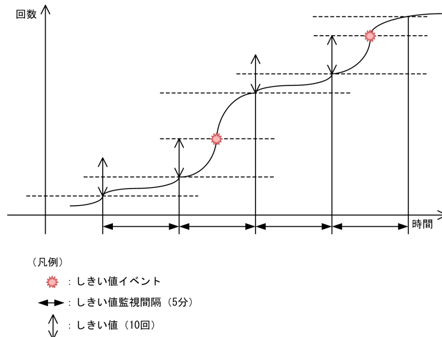
図 3-3 しきい値のイベント発行（FullGC 回数の場合）
