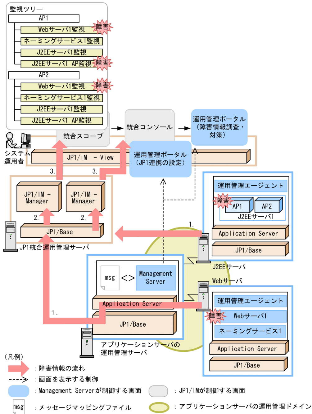
図 13-5 JP1/IM と連携した障害監視処理の流れ
