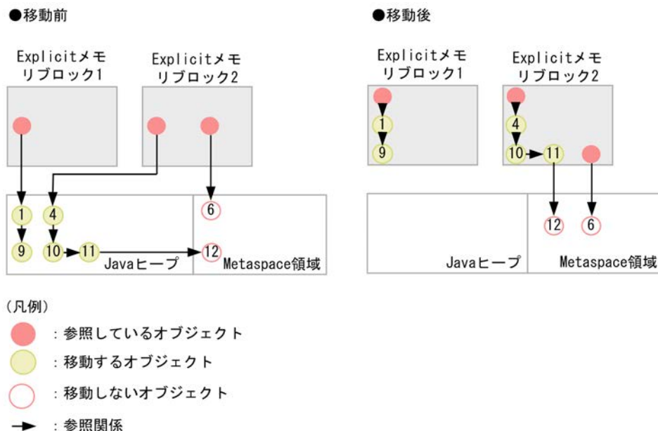
図 8-11 参照関係に基づいて移動するオブジェクト (例 1)
