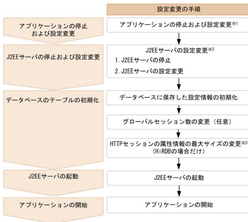
図 6-13 データベースセッションフェイルオーバー機能に関する設定の変更の流れ
