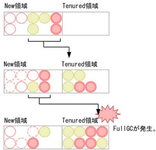
図 8-2 明示管理ヒープ機能を使用していない場合の昇格と明示管理ヒープ機能を使用している場合の昇格の違い
