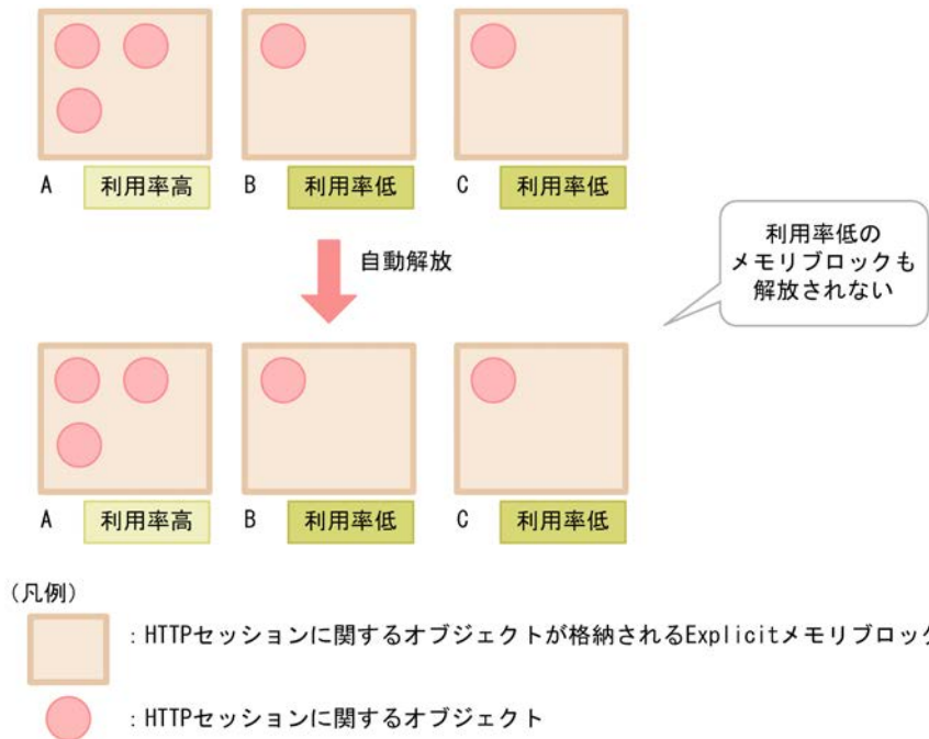
図 8-21 HTTP セッションで利用する Explicit ヒープの省メモリ化機能を利用していない場合
