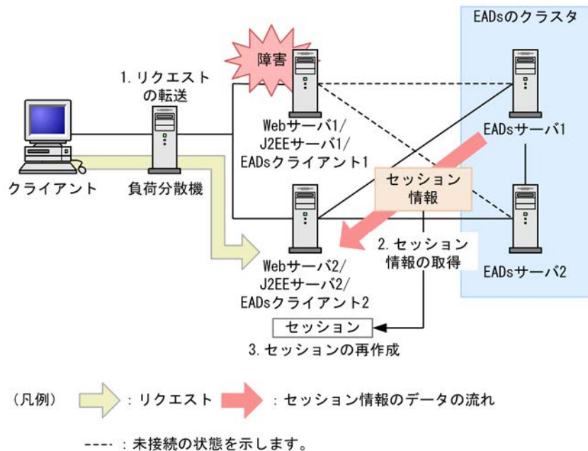
図 5-10 J2EE サーバで障害が発生した場合の処理（EADs セッションフェイルオーバー機能）
