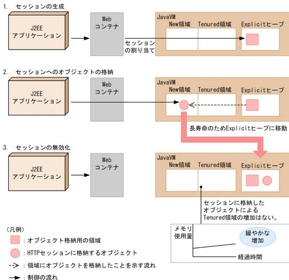
図 8-8 明示管理ヒープ機能を利用した例
