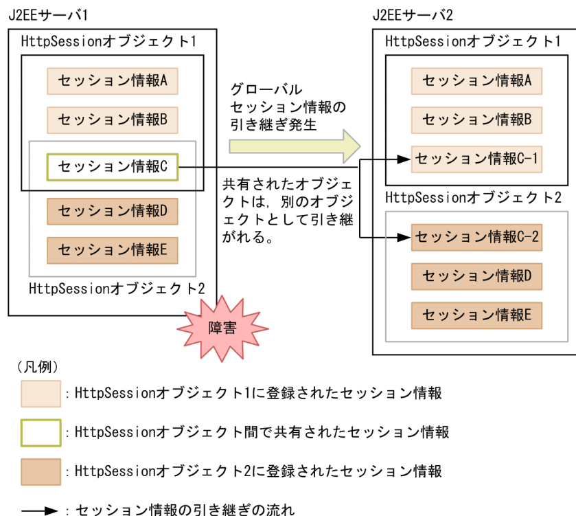
図 5-15 異なる HttpSession オブジェクトに同一のオブジェクトが登録されている場合の引き継ぎの例
