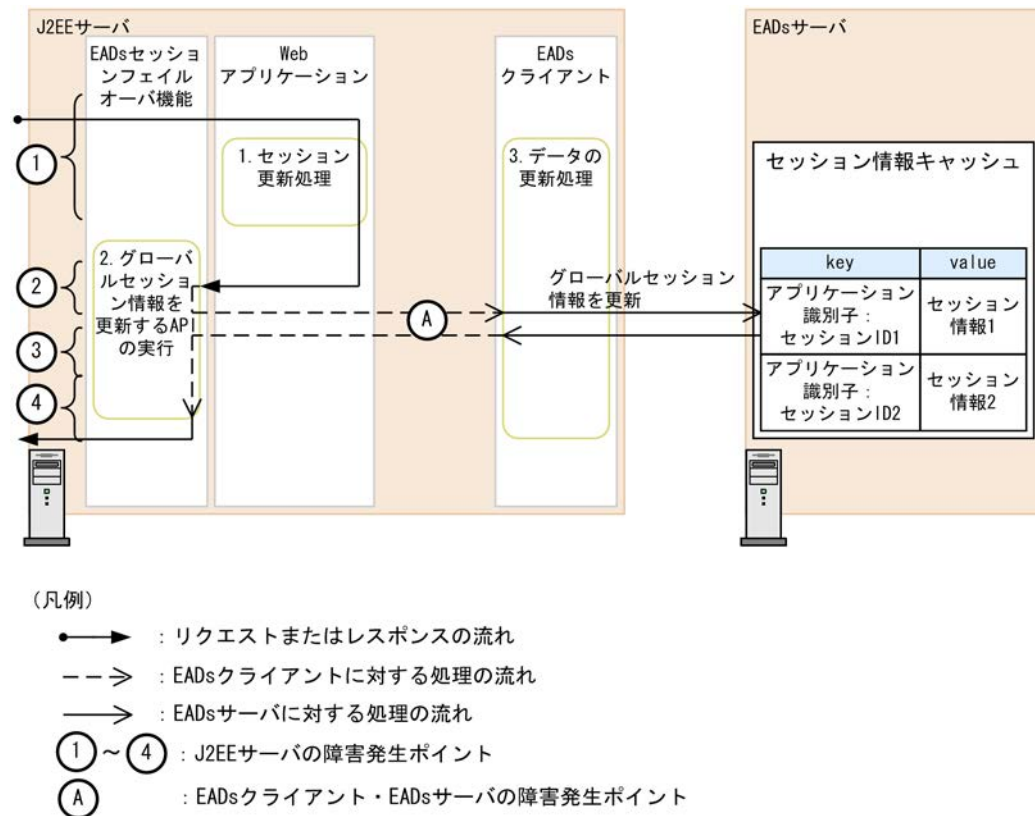
図 7-10 グローバルセッション情報の更新処理の流れと障害発生ポイント (EADs セッションフェイルオーバー機能)
