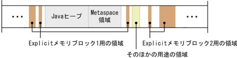
図 8-6 仮想メモリ空間の利用イメージ (32 ビット版の場合)
