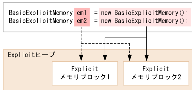
図 8-23 ExplicitMemory インスタンスと Explicit メモリブロックの関係
