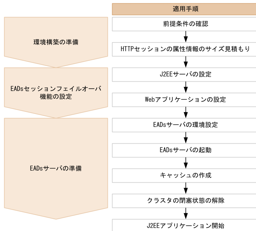
図 7-1 適用手順（EADs セッションフェイルオーバー機能）
