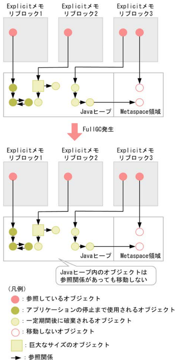
図 8-16 Explicit メモリブロックへのオブジェクト移動制御機能を利用している場合
