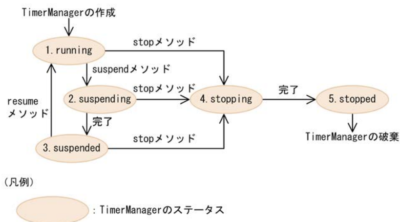
図 10-6 TimerManager のステータス遷移
