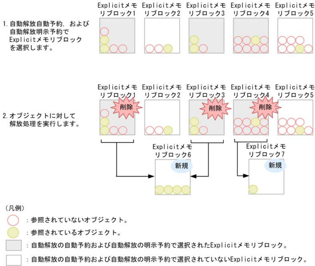
図 8-13 Explicit メモリブロックの自動解放
