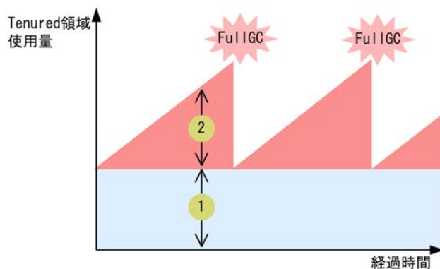
図 8-1 FullGC で回収されるオブジェクト、および FullGC で回収されないオブジェクト
