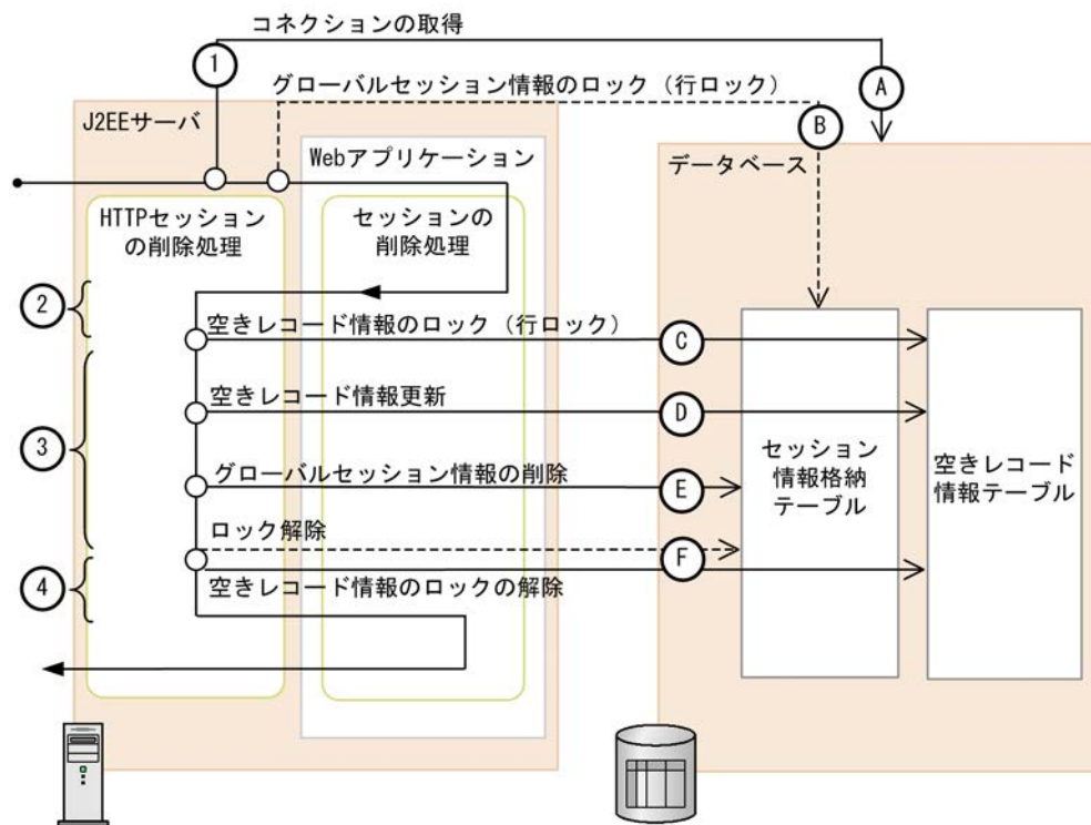
図 6-10 グローバルセッション情報の削除処理の流れと障害発生ポイント
