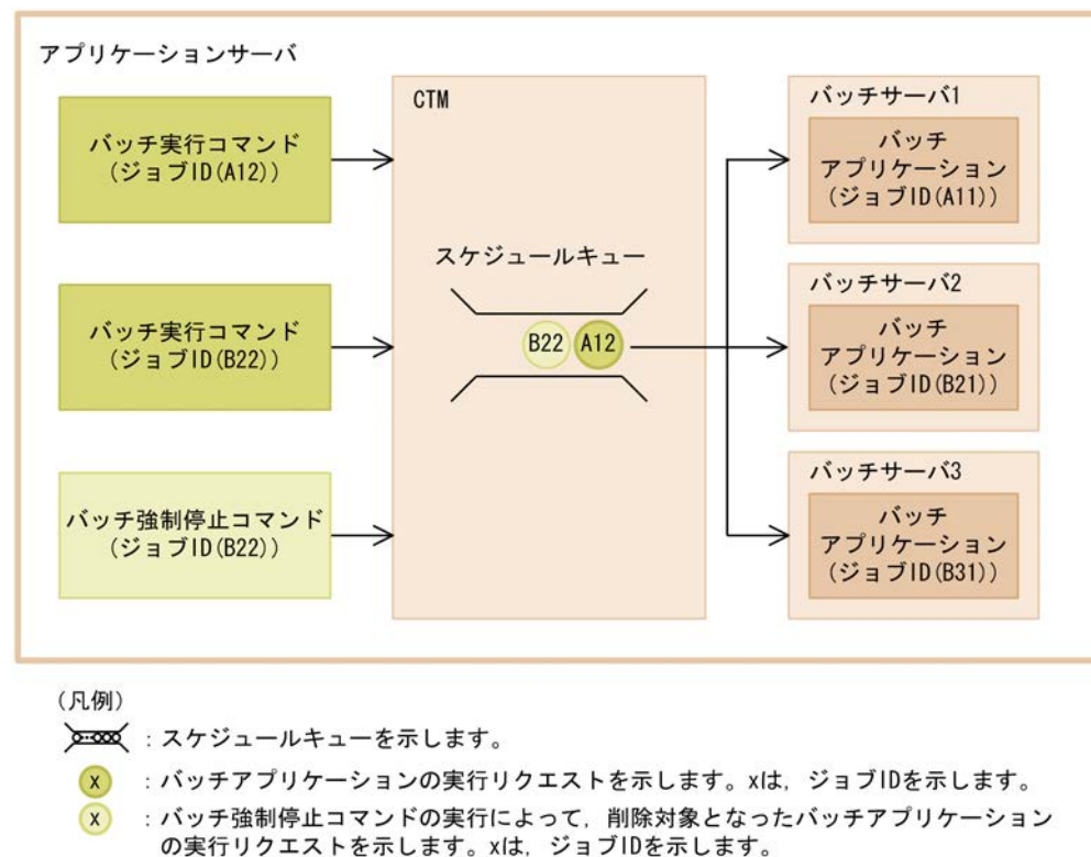
図 4-2 スケジューリング機能を使用したバッチアプリケーション実行の流れ
