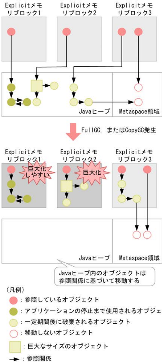
図 8-15 Explicit メモリブロックへのオブジェクト移動制御機能と、明示管理ヒープ機能適用除外クラス指定機能を利用していない場合
