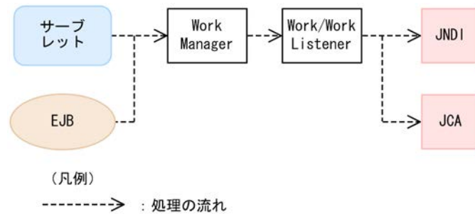
図 10-2 WorkManager を使用した非同期スレッド処理の流れ
