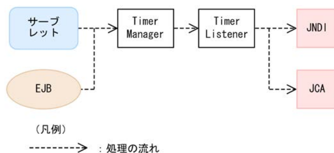
図 10-1 TimerManager を使用した非同期タイマ処理の流れ
