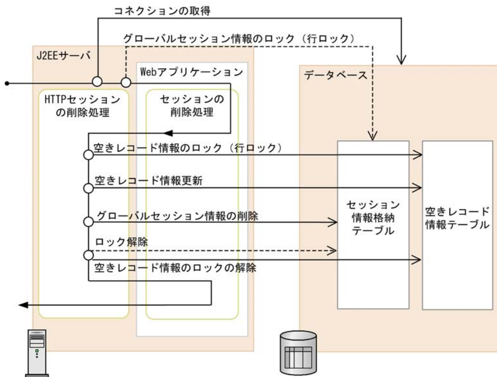
図 6-4 グローバルセッション情報の削除（データベースセッションフェイルオーバー機能）
