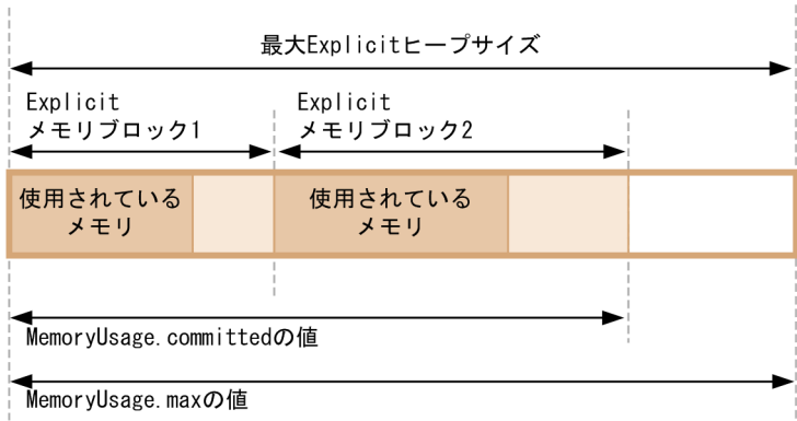
図 8-25 各フィールドが示す値（MemoryUsage クラスのインスタンス）
