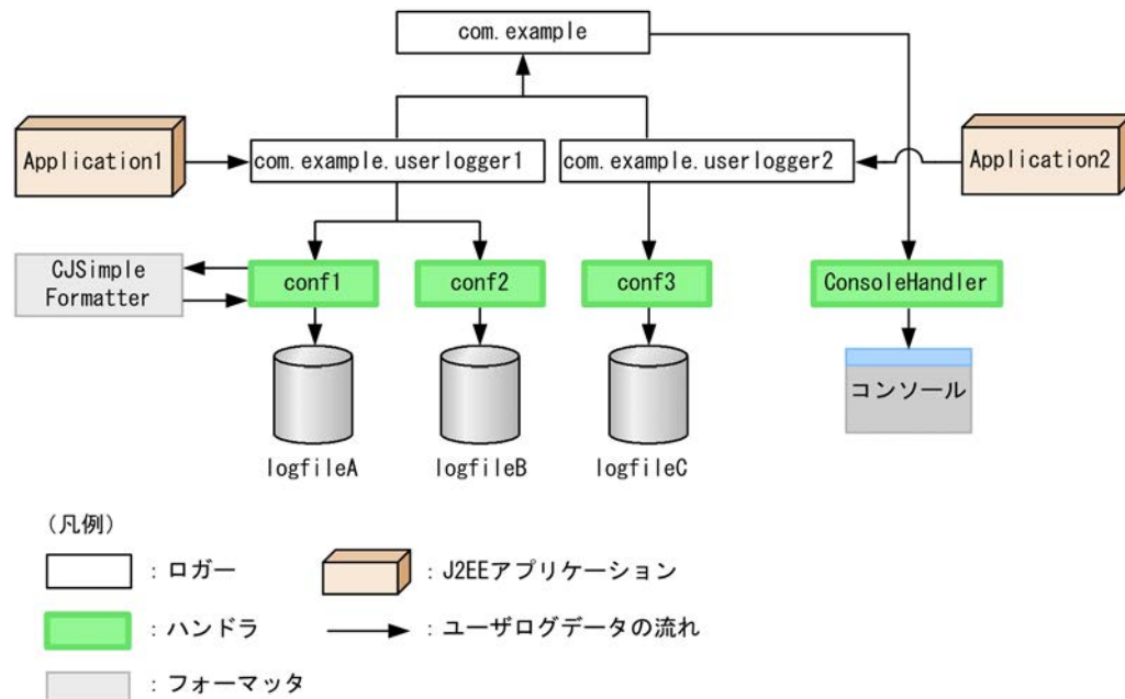
図 9-4 J2EE アプリケーションのユーザログ出力例
