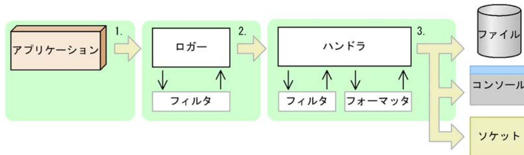
図 9-2 Java ロギングの仕組み
