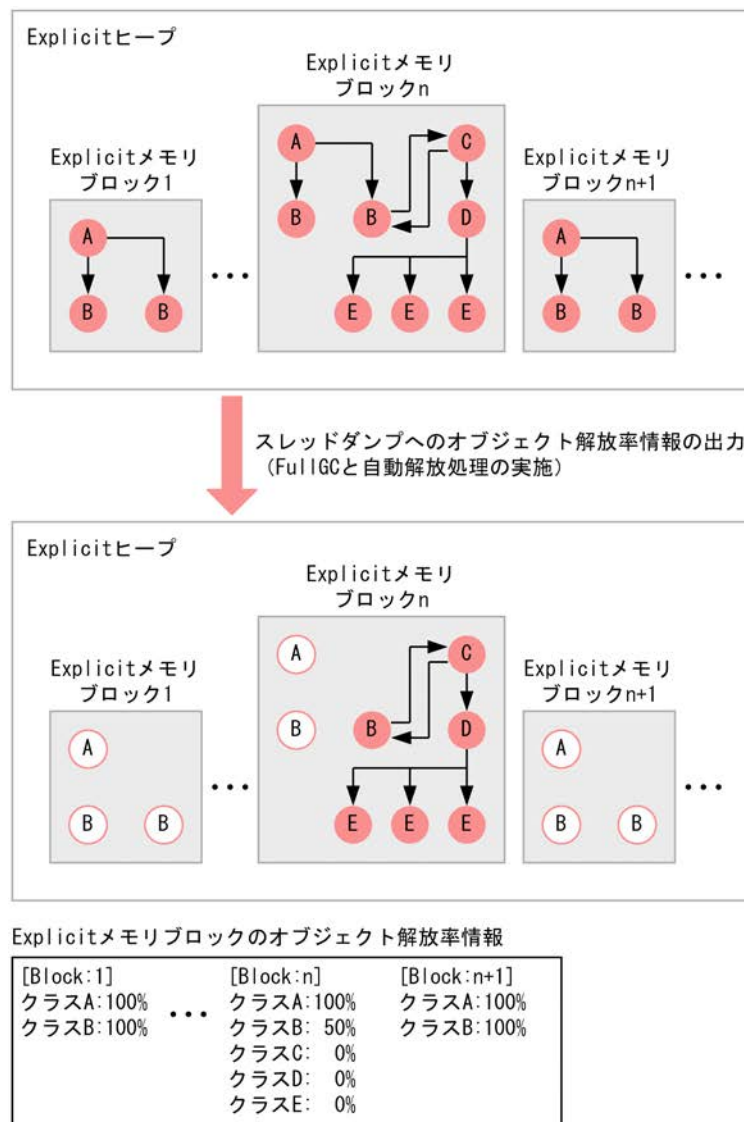
図 8-19 オブジェクト解放率情報の出力例
