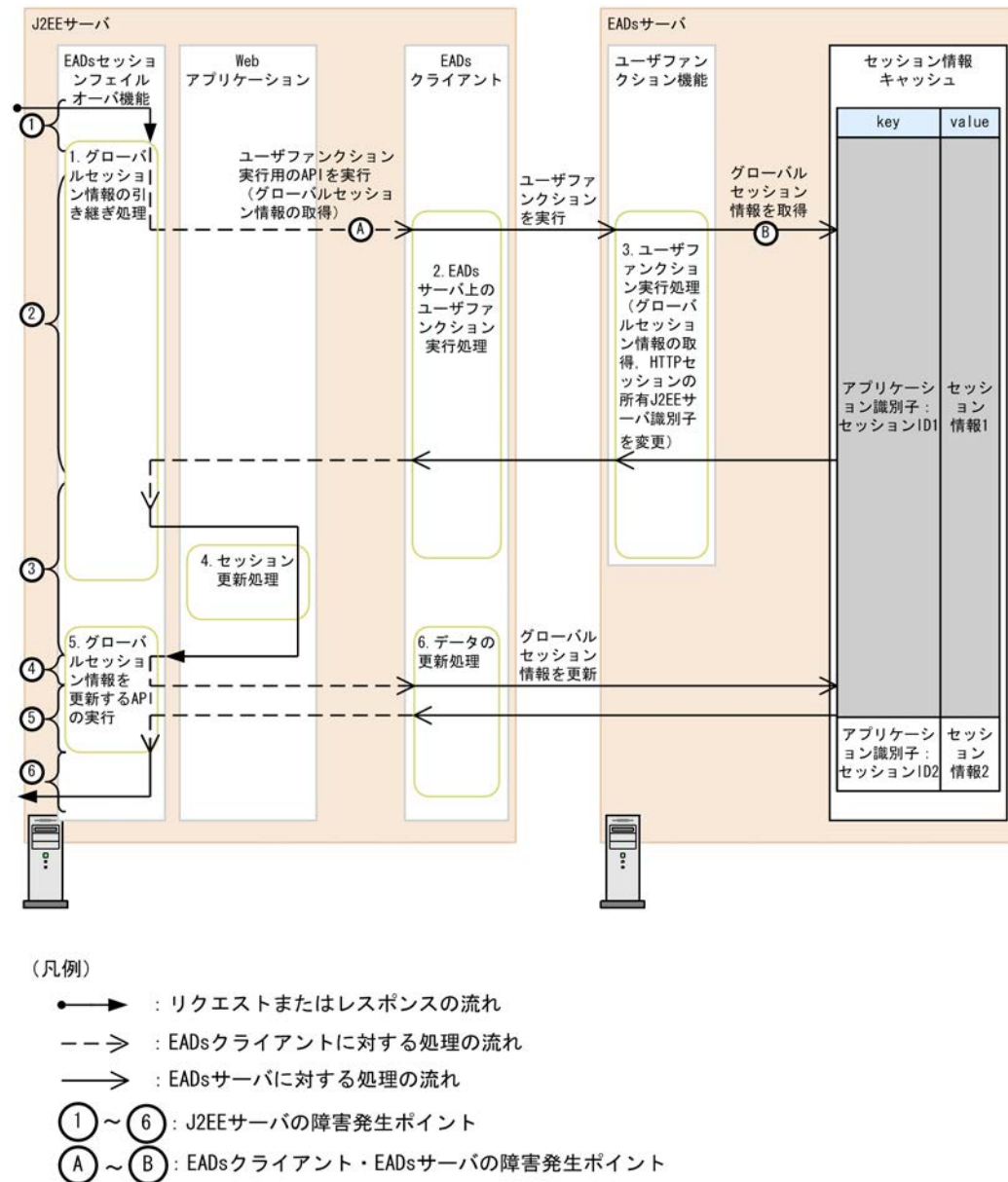
図 7-13 グローバルセッション情報を使用したグローバルセッション引き継ぎ処理の流れと障害発生ポイント (EADs セッションフェイルオーバー機能)
