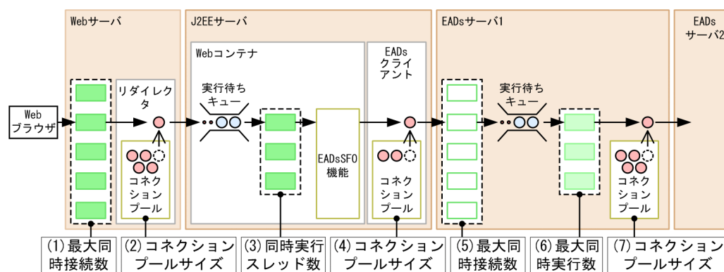
図 7-3 同時接続数，同時実行数，およびコネクションプールサイズが設定できるポイント
