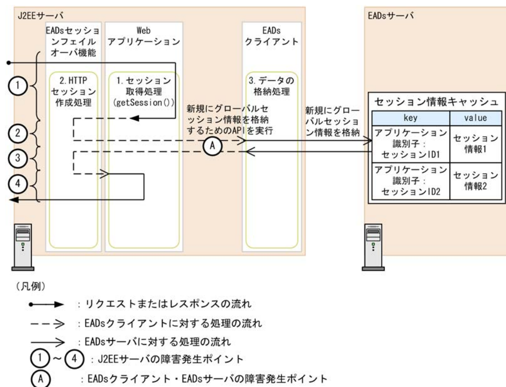
図 7-9 グローバルセッション情報の作成処理の流れと障害発生ポイント（EADs セッションフェイルオーバー機能）
