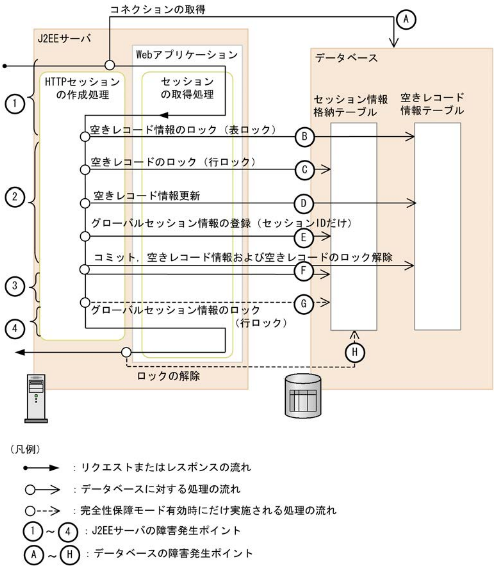
図 6-8 グローバルセッション情報の作成処理の流れと障害発生ポイント
