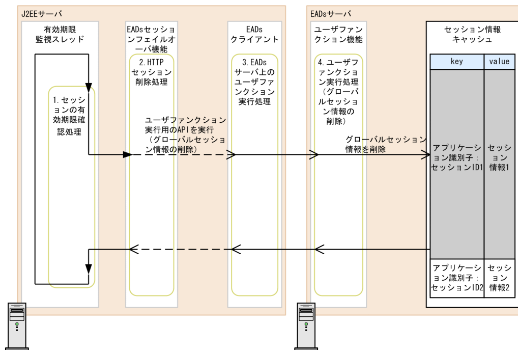
図 7-8 グローバルセッション情報の有効期限が切れた場合の処理（EADs セッションフェイルオーバー機能）
