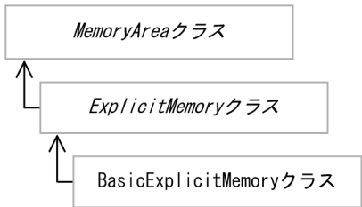
図 8-24 明示管理ヒープ機能 API のクラス階層
