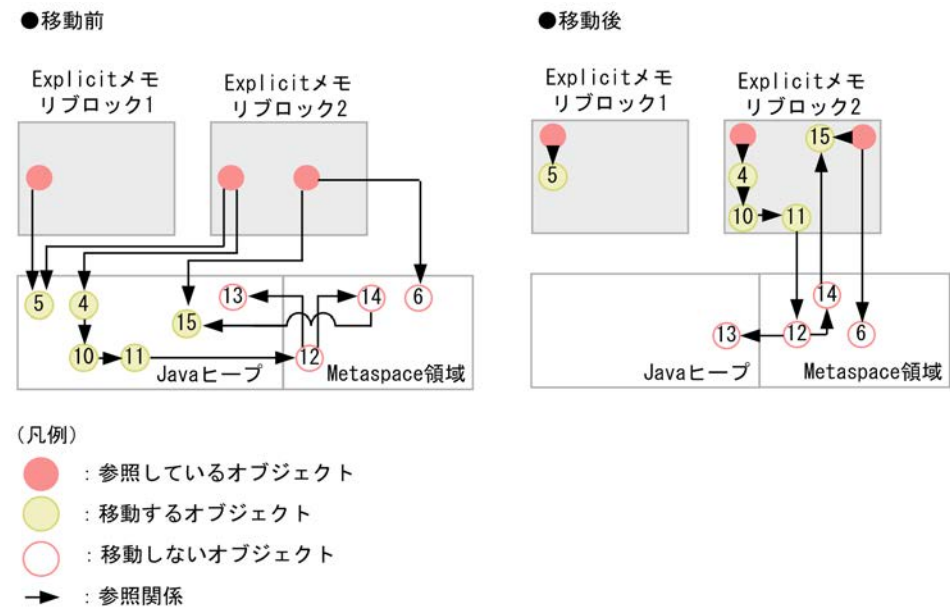
図 8-12 参照関係に基づいて移動するオブジェクト（例 2）
