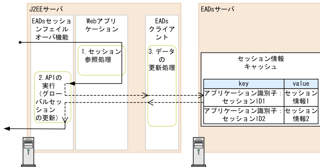
図 5-14 参照専用リクエストの処理 (EADs セッションフェイルオーバー機能)
