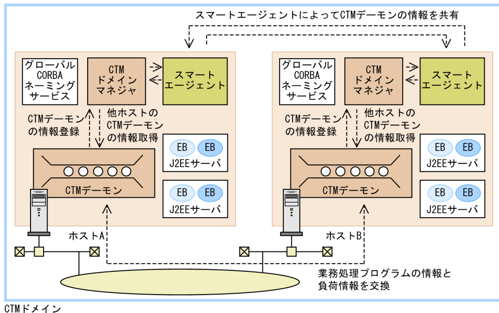
図 3-11 異なるネットワークセグメントでの CTM ドメインマネージャによる情報共有
