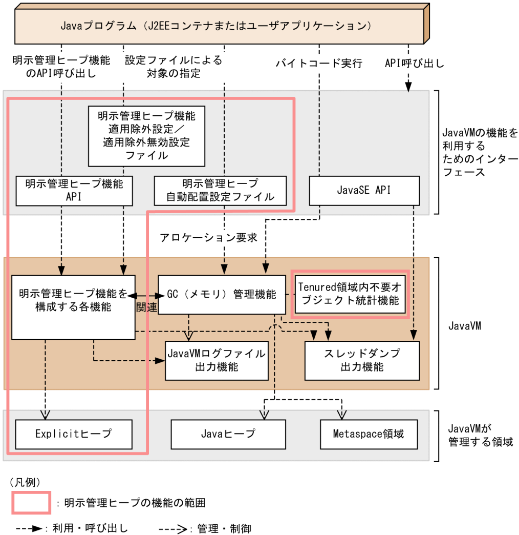
図 8-3 明示管理ヒープ機能の位置づけ
