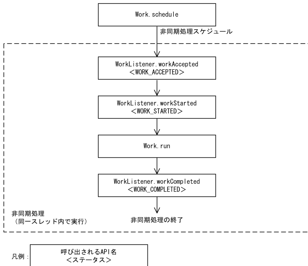
図 10-10 WorkListener インタフェースの API が呼び出される流れとステータスの遷移
