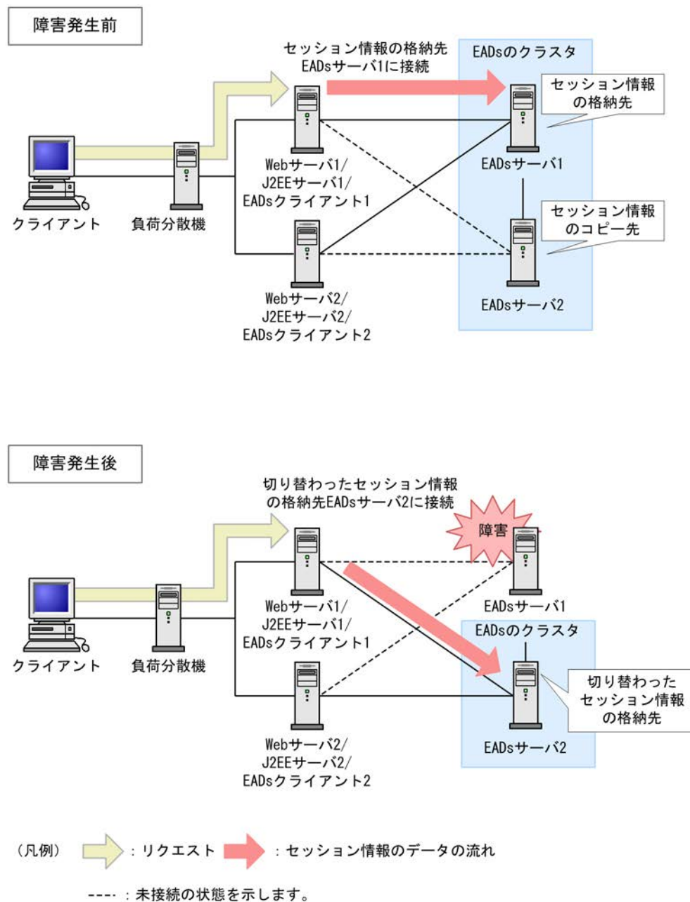
図 5-11 EADs サーバで障害が発生した場合の処理の流れ
