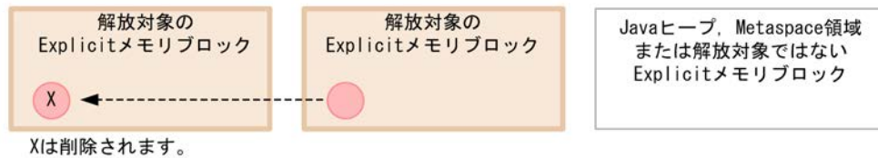
図 8-14 Explicit メモリブロック解放時に外部から参照されている場合の動作
