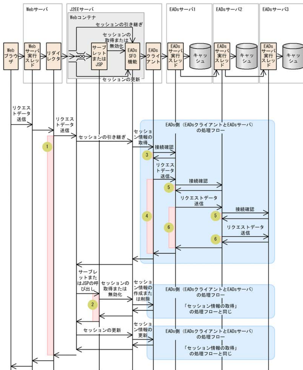
図 7-2 タイムアウトが設定できるポイント (セッションの引き継ぎ)
