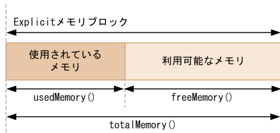
図 8-26 各 API で取得できる値
