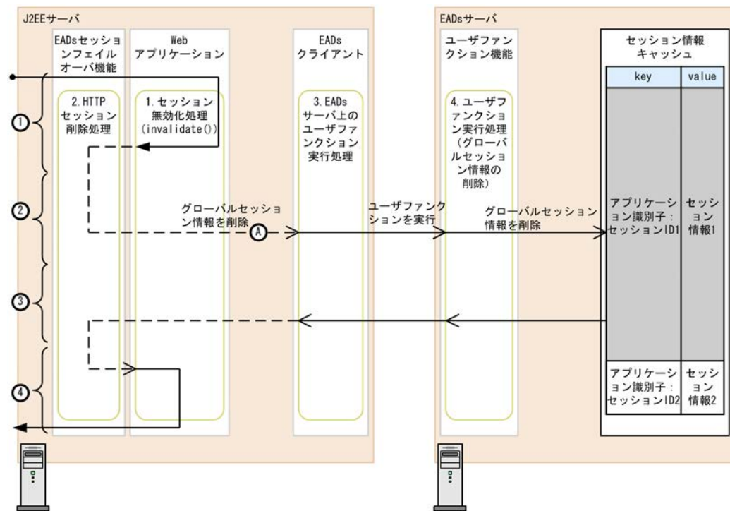
図 7-11 グローバルセッション情報の削除処理の流れと障害発生ポイント (EADs セッションフェイルオーバー機能)
