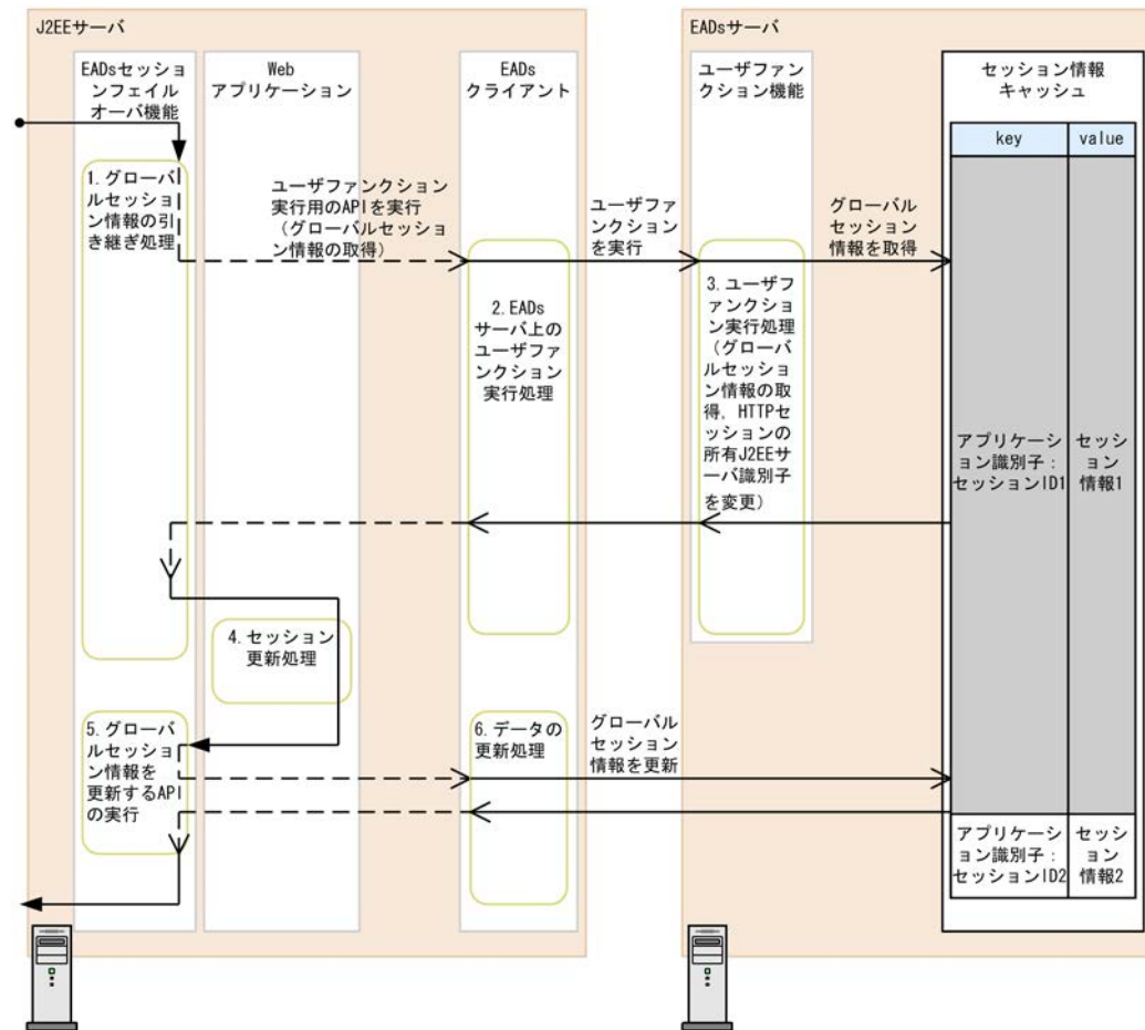
図 7-7 グローバルセッション情報を使用したセッション情報の引き継ぎ (EADs セッションフェイルオーバー機能)
