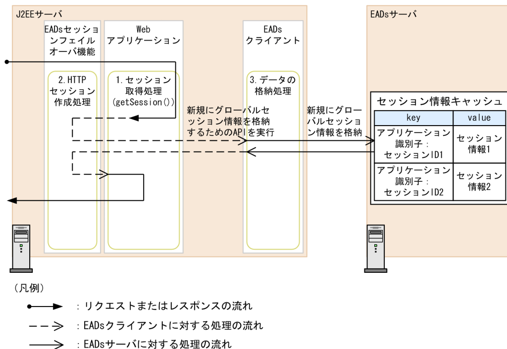
図 7-4 グローバルセッション情報の作成 (EADs セッションフェイルオーバー機能)
