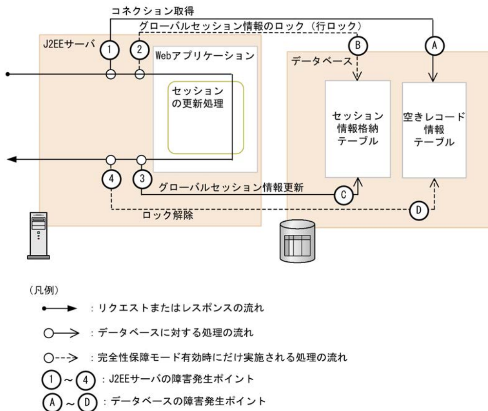
図 6-9 グローバルセッション情報の更新処理の流れと障害発生ポイント
