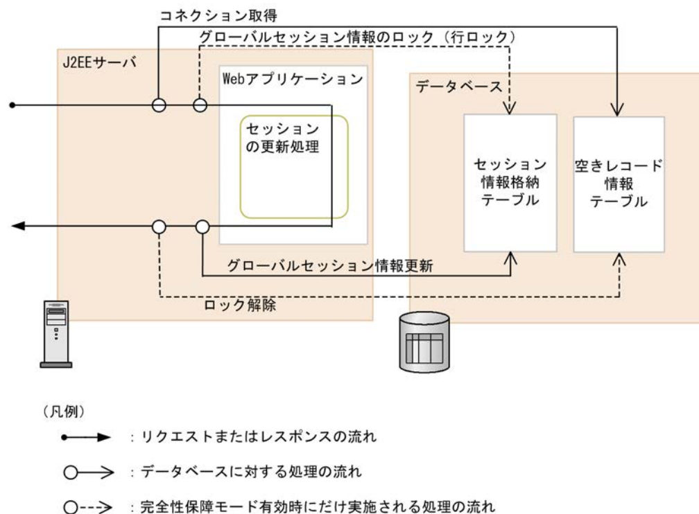
図 6-3 グローバルセッション情報の更新 (データベースセッションフェイルオーバー機能)
