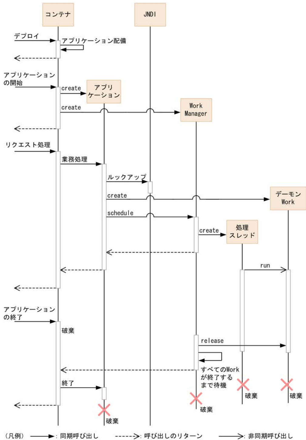
図 10-8 デーモン Work のライフサイクル
