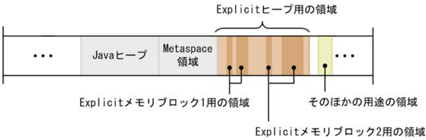
図 8-5 仮想メモリ空間の利用イメージ (64 ビット版の場合)
