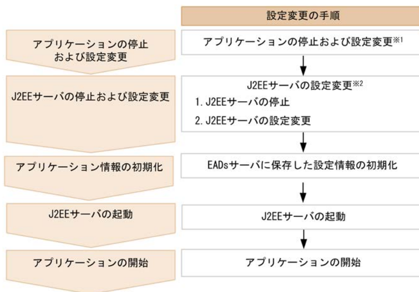
図 7-14 EADs セッションフェイルオーバー機能に関する設定の変更の流れ
