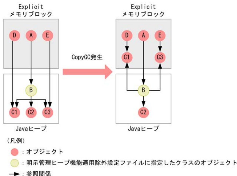
図 8-18 明示管理ヒープ機能適用除外対象のオブジェクトからの参照経路が複数ある場合の例
