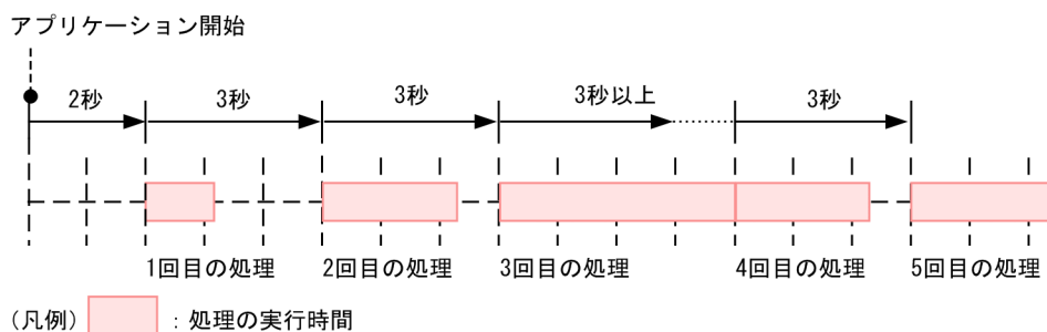
図 10-3 fixed-rate の処理のイメージ
