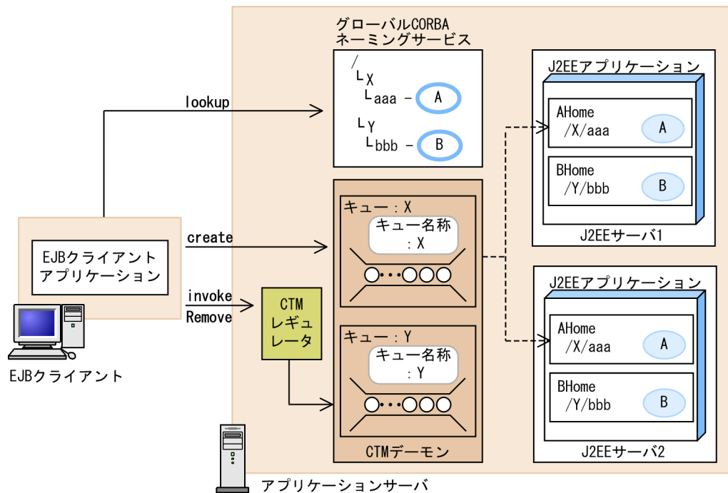
図 3-2 スケジュールキューを共有する例 (Bean 単位)
