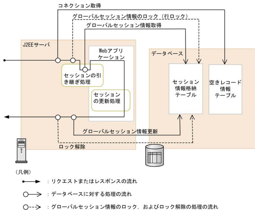
図 6-5 グローバルセッション情報を使用したセッション情報の引き継ぎ（データベースセッションファイルオーバー機能）
