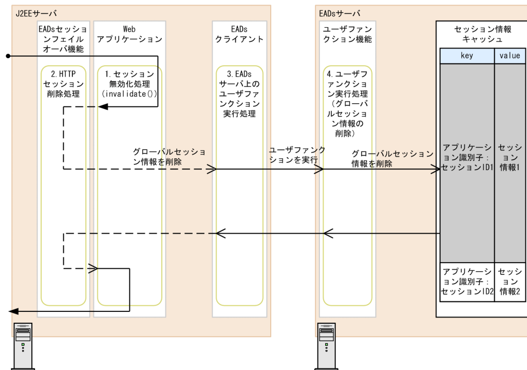
図 7-6 グローバルセッション情報の削除 (EADs セッションフェイルオーバー機能)
