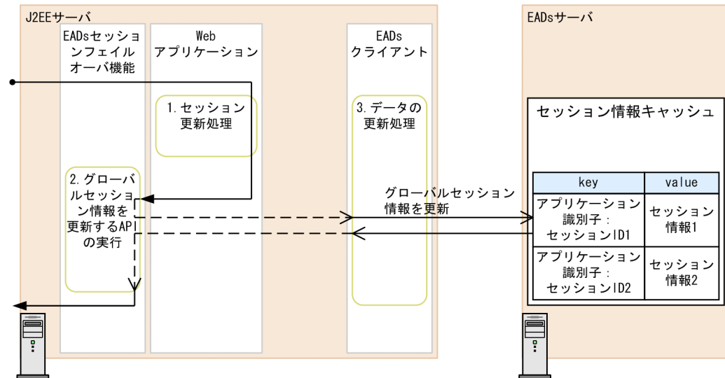
図 7-5 グローバルセッション情報の更新 (EADs セッションフェイルオーバー機能)
