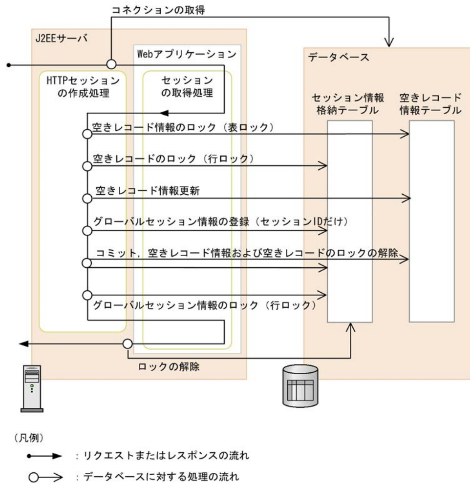
図 5-8 完全性保障モードを有効にした場合のリクエスト処理の流れ
