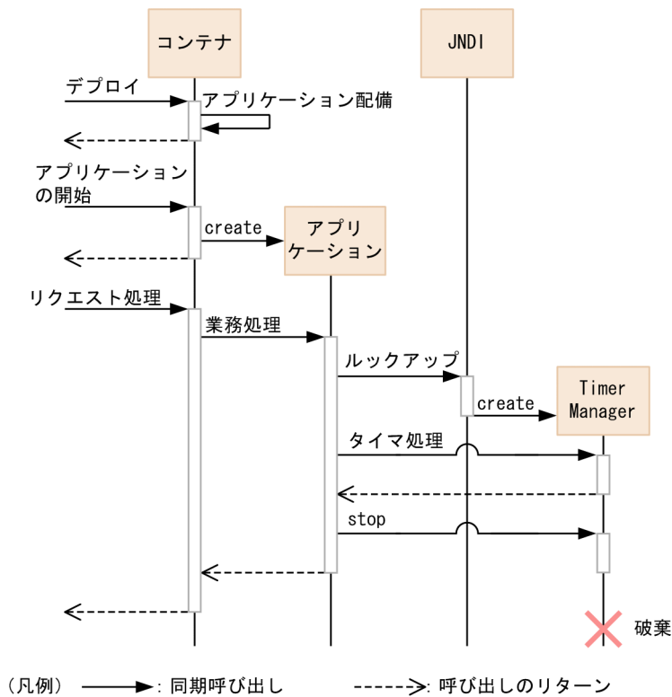
図 10-5 TimerManager のライフサイクル
