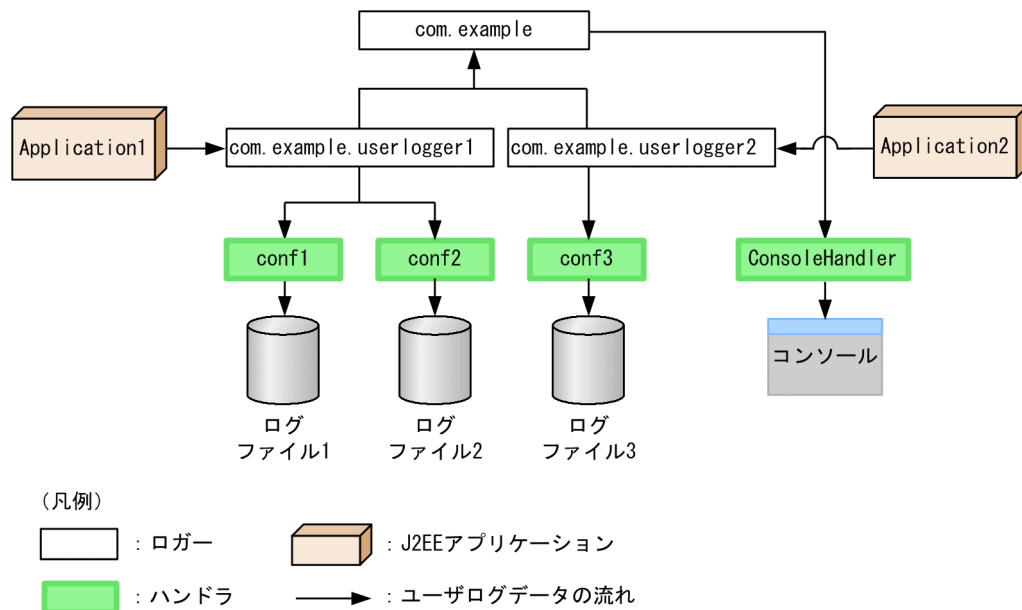
図 9-3 ロガーとハンドラの作成例
