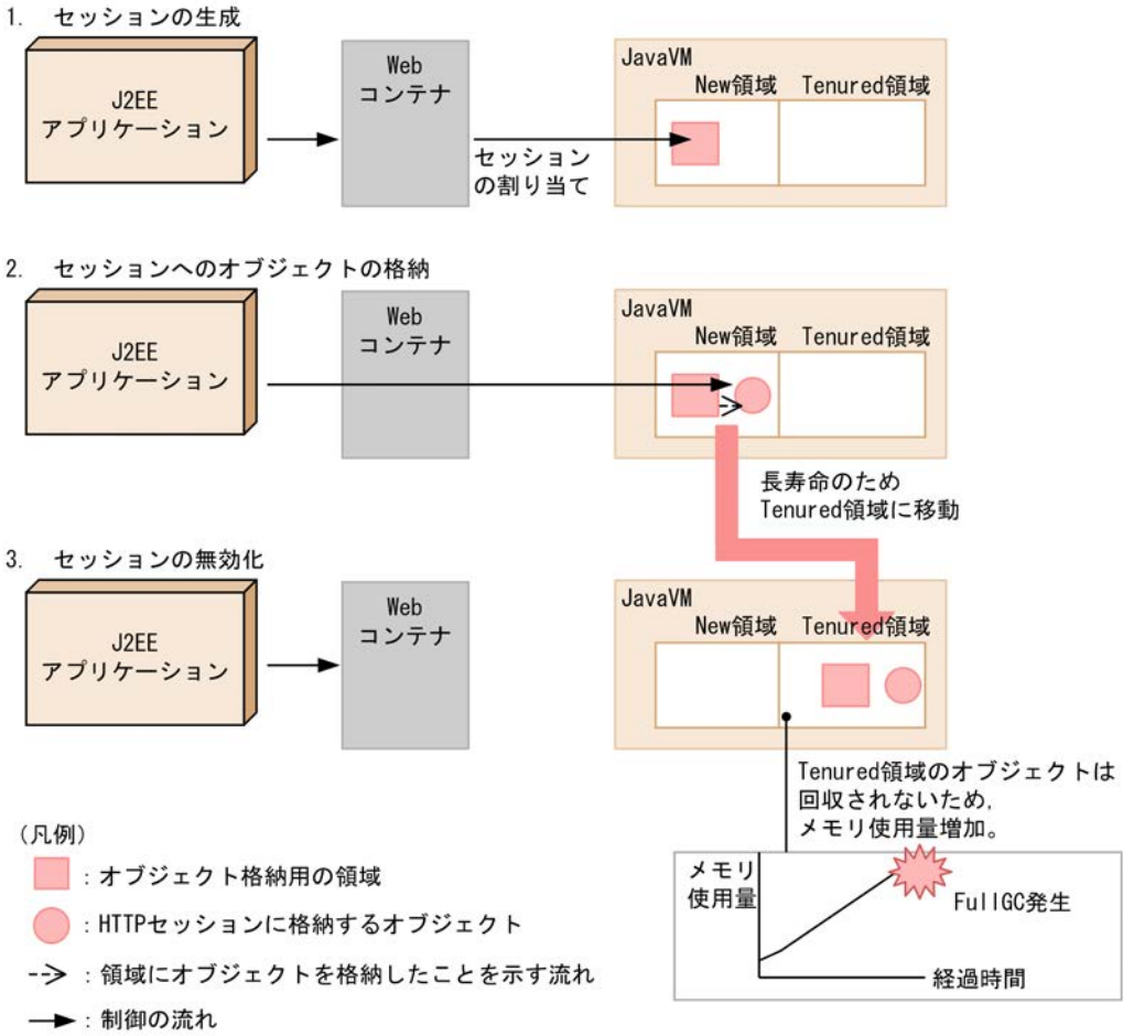
図 8-7 明示管理ヒープ機能を利用していない場合の例
