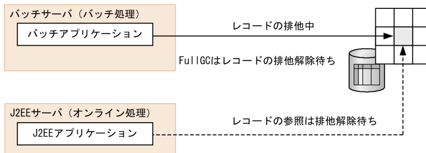
図 2-14 GC 制御機能を使用している場合
