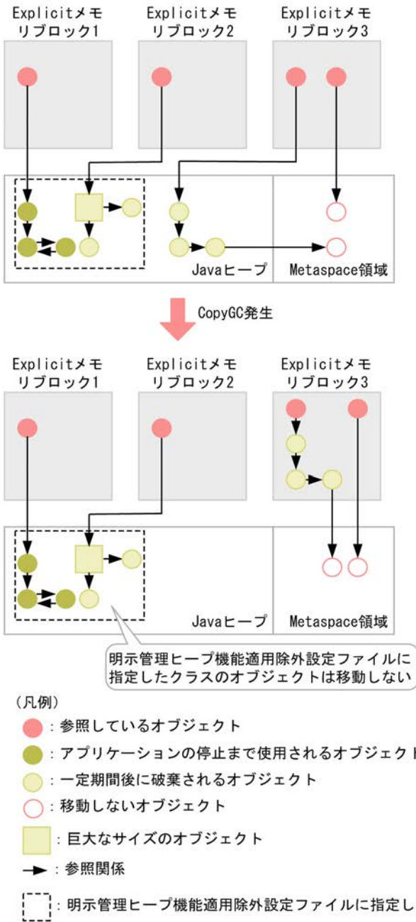
図 8-17 Explicit メモリブロックへのオブジェクト移動制御機能に加えて明示管理ヒープ機能適用除外クラス指定機能を利用している場合
