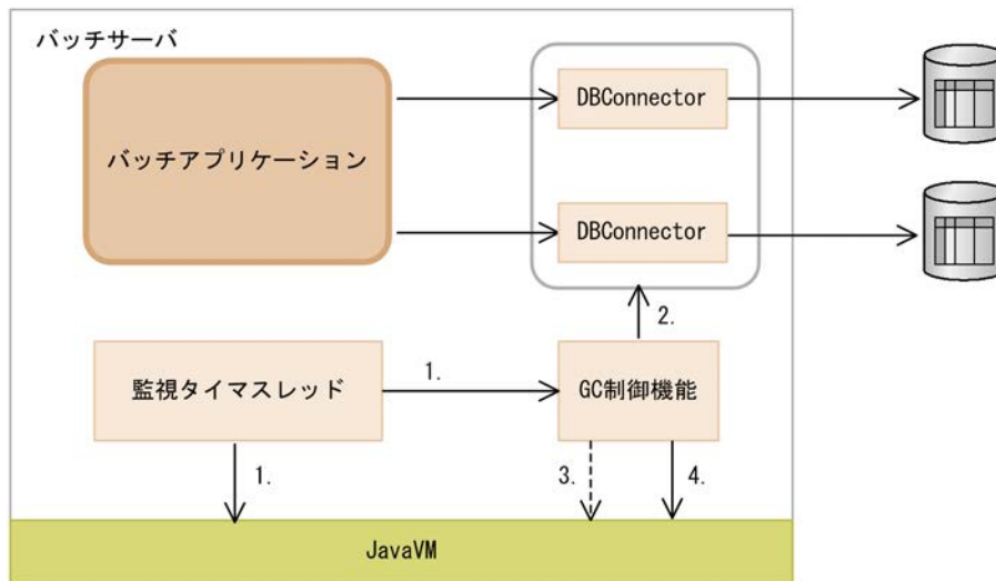
図 2-15 GC 制御の処理の流れ
