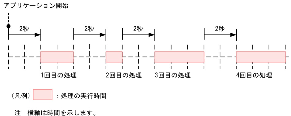
図 10-4 fixed-delay の処理のイメージ
