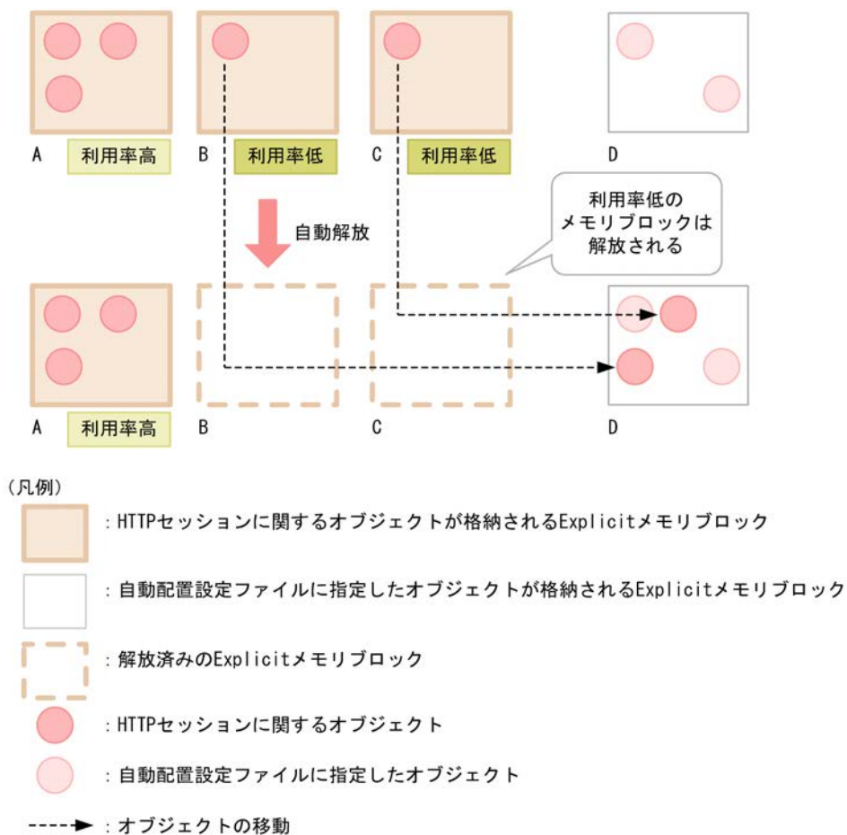
図 8-22 HTTP セッションで利用する Explicit ヒープの省メモリ化機能を利用している場合
