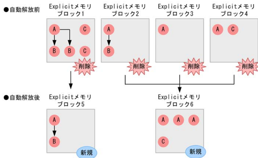
図 8-20 オブジェクト解放率情報の算出例
