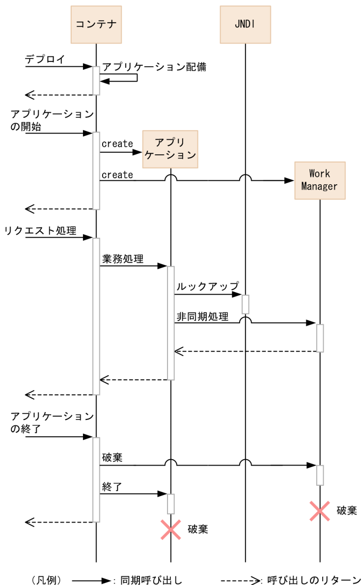
図 10-7 WorkManager のライフサイクル
