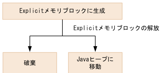
図 8-9 Explicit メモリブロックに配置するオブジェクトのライフサイクル
