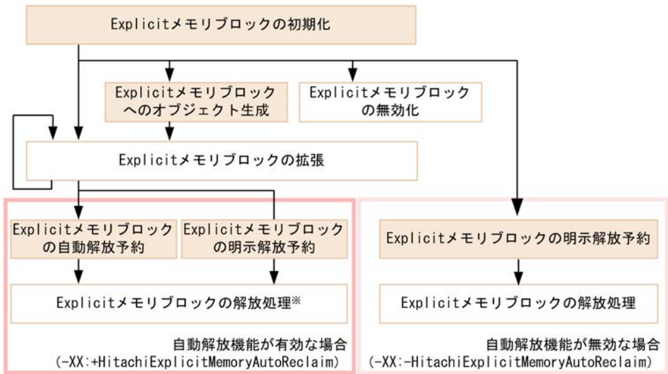
図 8-10 Explicit メモリブロックのライフサイクル
