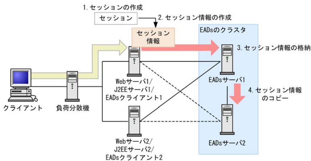
図 5-9 セッション情報の格納の流れ (EADs セッションフェイルオーバー機能)
