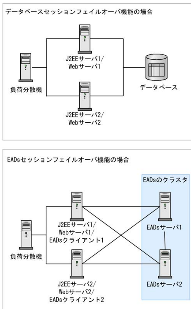
図 5-3 セッションフェイルオーバー機能の前提となる構成
