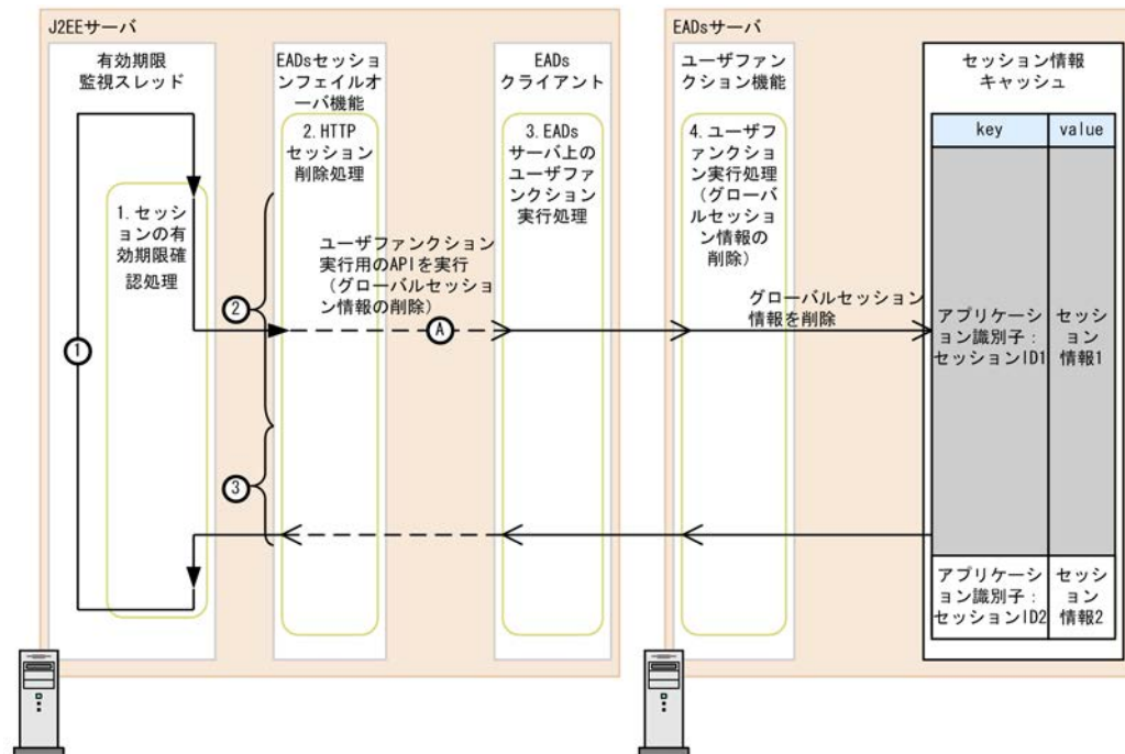
図 7-12 有効期限切れによるグローバルセッション情報削除処理の流れと障害発生ポイント（EADs セッションフェイルオーバー機能）
