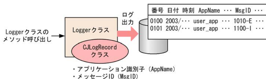
図 9-1 ユーザログ機能の処理の流れ
