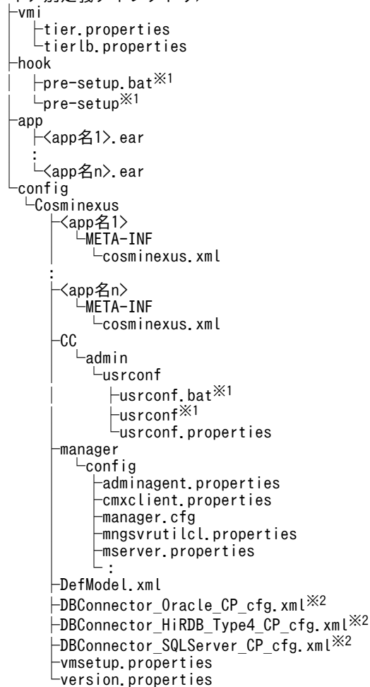
図 5-2 ティア別定義ディレクトリの構成
