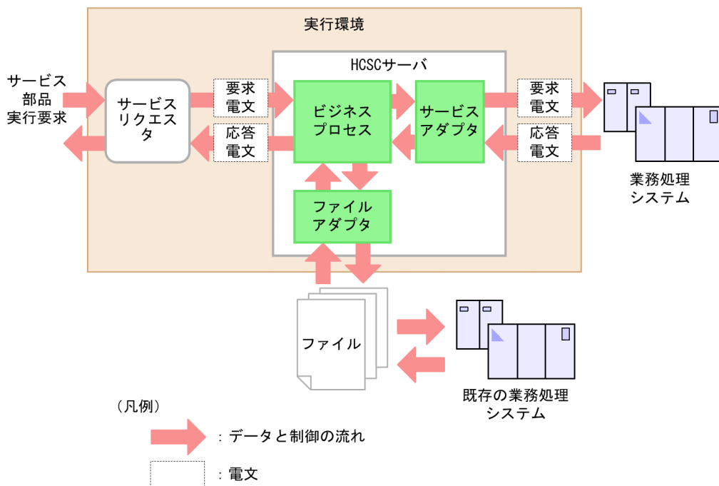
図 9-17 ファイルアダプタからのファイルの入出力
