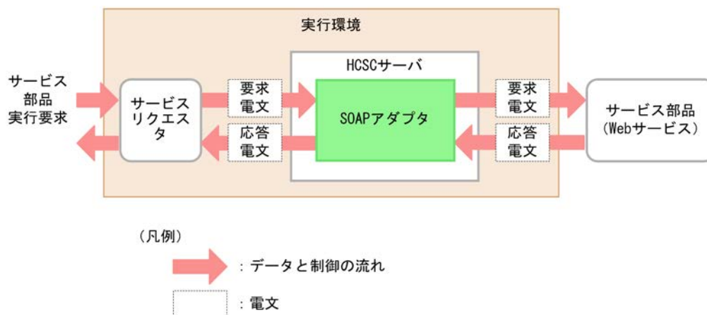
図 9-11 SOAP アダプタからのサービス部品実行
