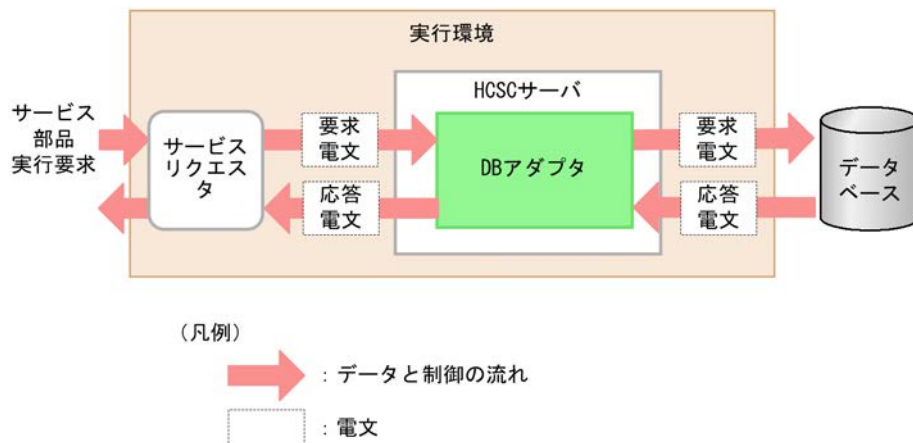
図 9-15 DB アダプタからの SQL 実行
