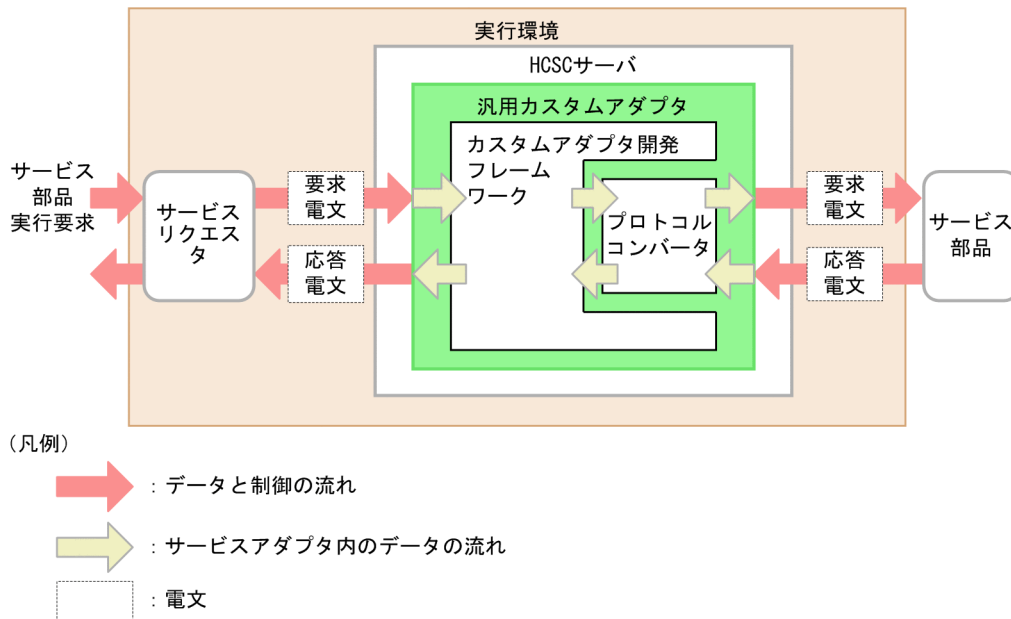
図 9-24 汎用カスタムアダプタからのサービス部品の実行
