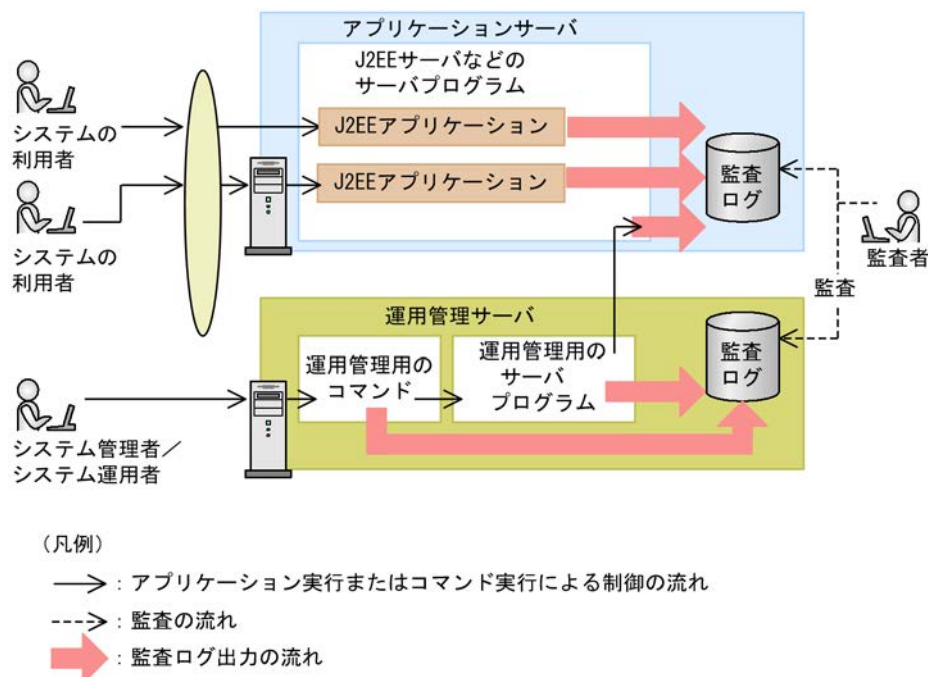
図 4-7 アプリケーションサーバでの監査ログ出力の概要
