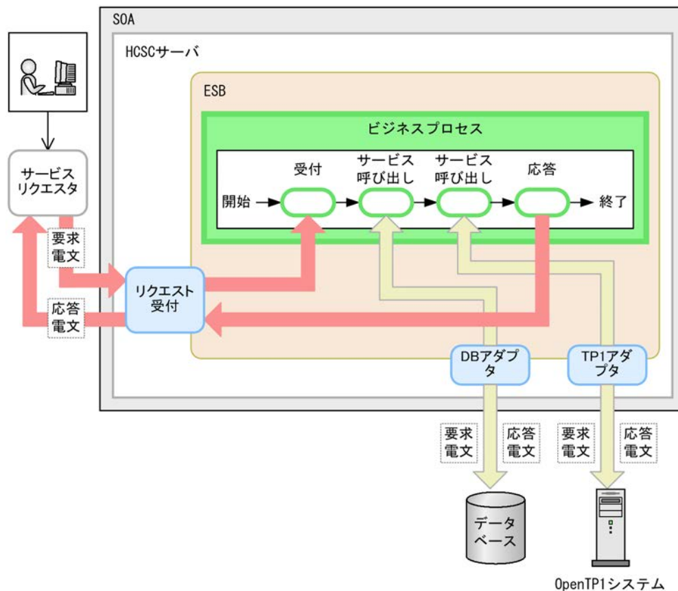
図 9-2 ビジネスプロセスからのサービス部品実行
