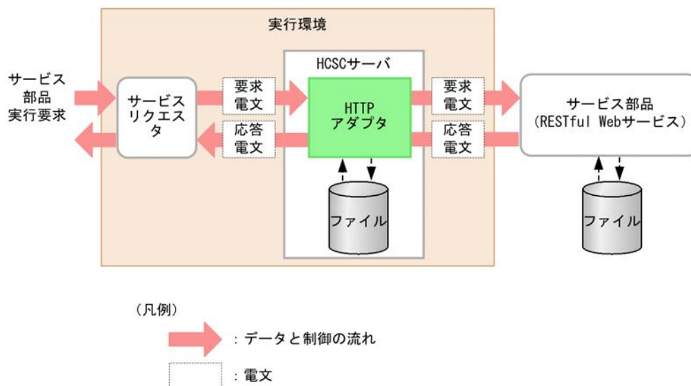
図 9-23 HTTP アダプタからのサービス部品実行
