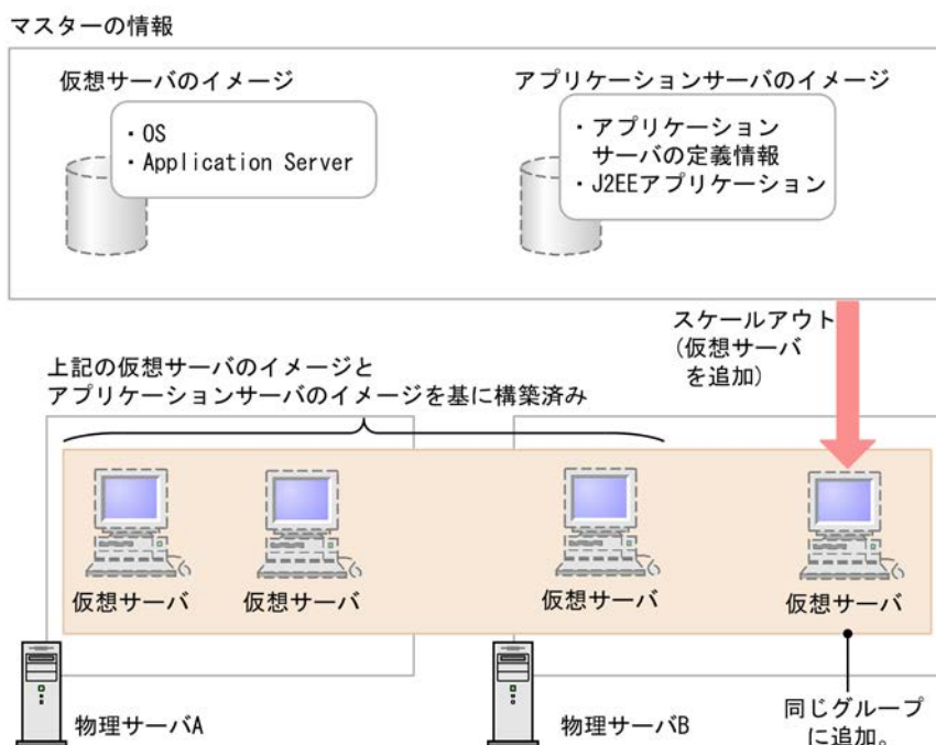
図 4-12 仮想サーバを追加する例
