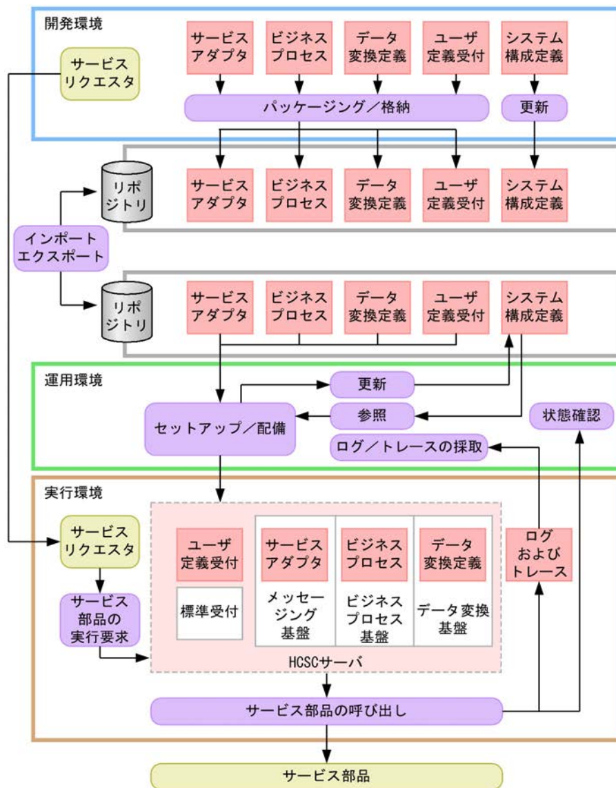
図 10-8 システムの運用と開発環境、運用環境および実行環境の関係
