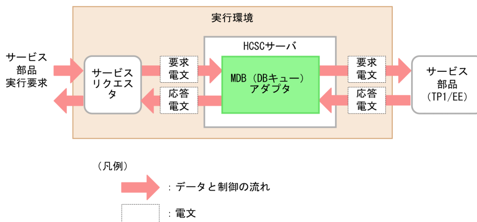
図 9-14 MDB (DB キュー) アダプタからのサービス部品実行
