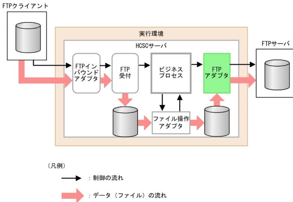
図 9-20 FTP アダプタと FTP サーバとの間のファイルの送受信
