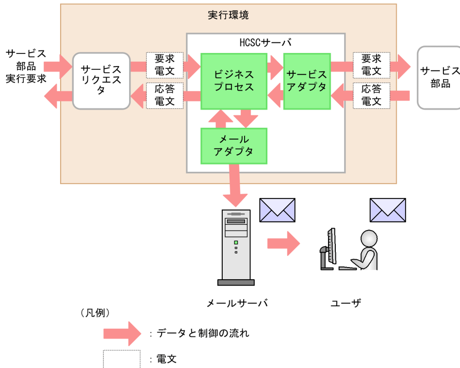
図 9-22 メールアダプタからのメールの送信
