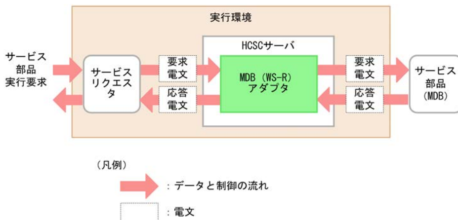
図 9-13 MDB (WS-R) アダプタからのサービス部品実行
