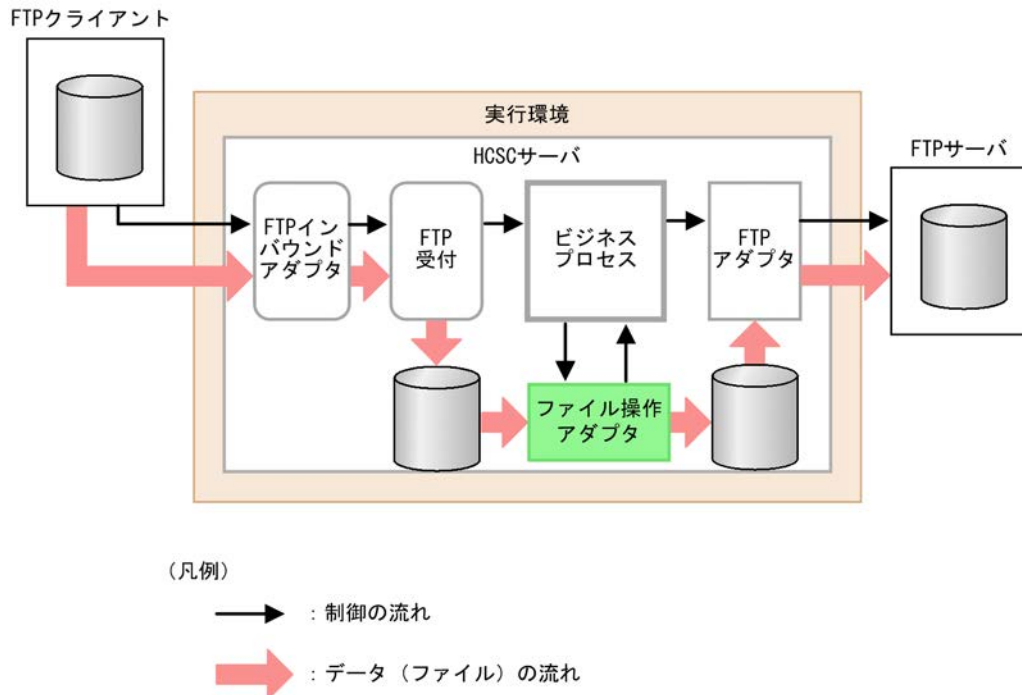
図 9-21 ファイル操作アダプタからのファイルの操作
