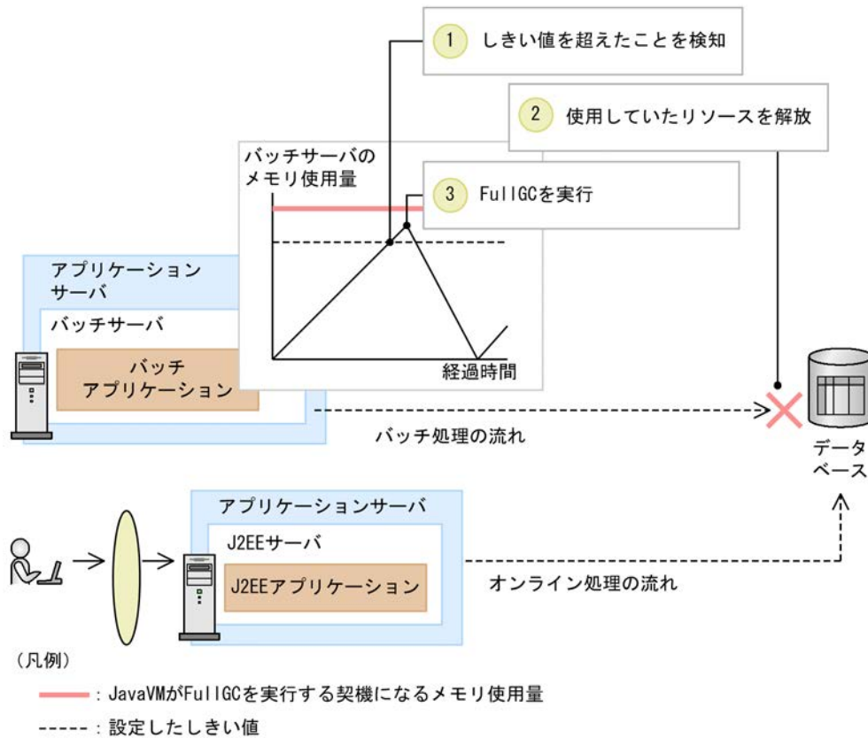
図 4-15 バッチサーバでの FullGC 制御の概要
