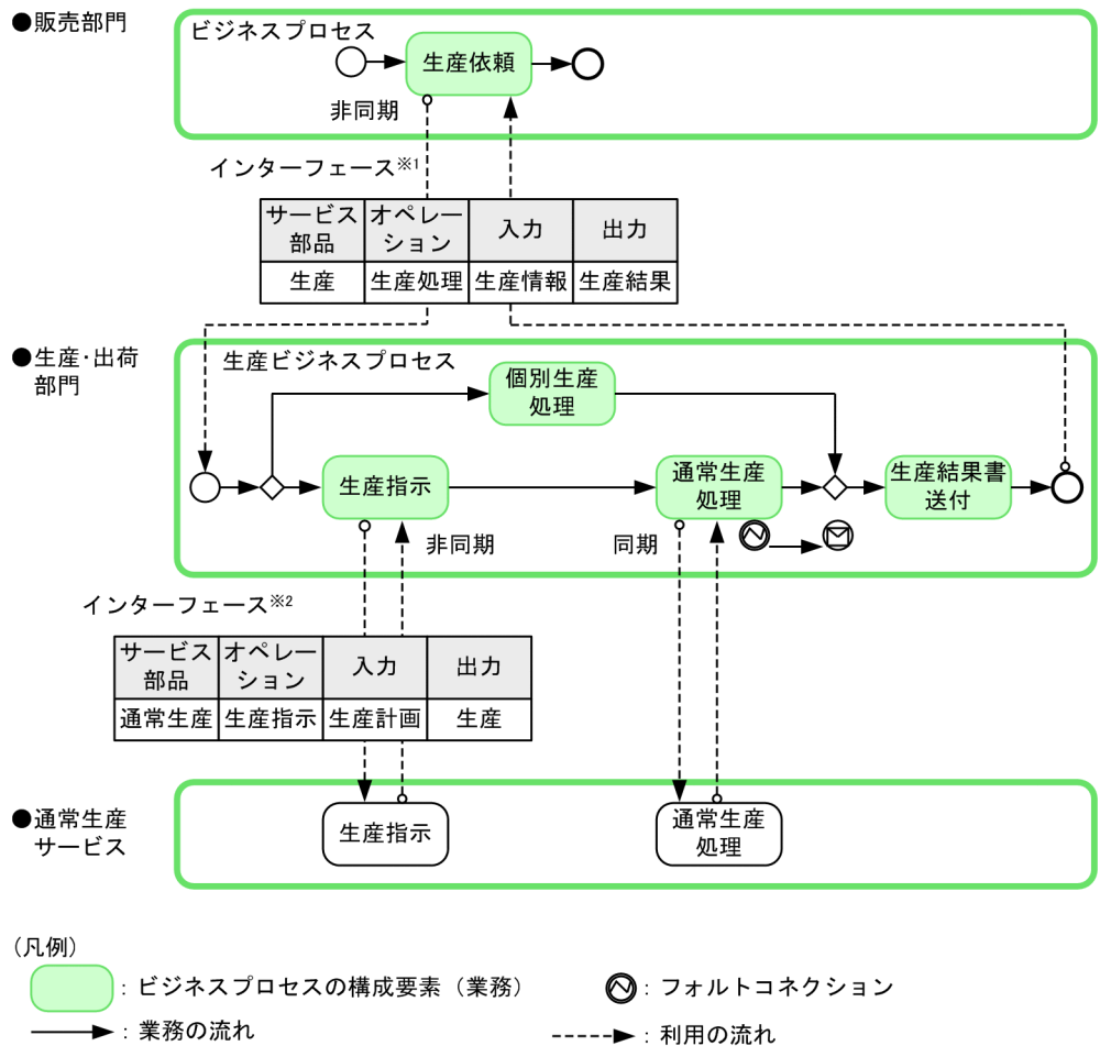
図 10-4 サービスおよびビジネスプロセスのインターフェースの設計例
