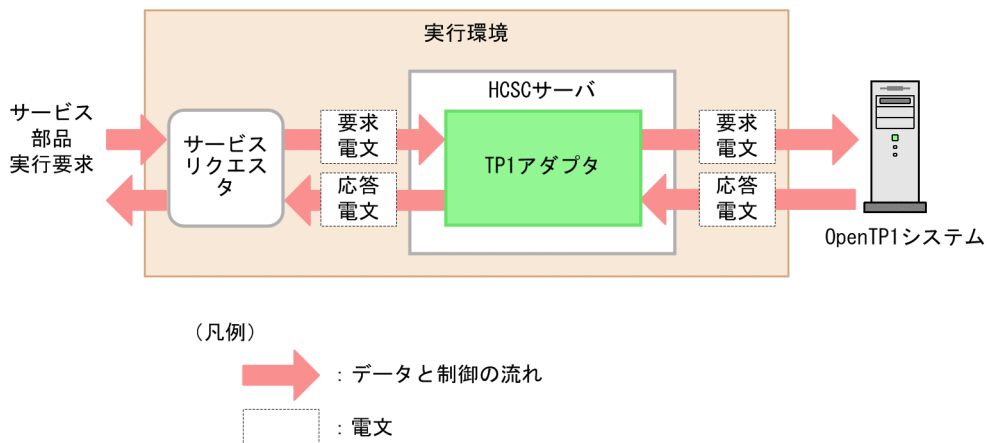
図 9-16 TP1 アダプタからのサービス部品実行
