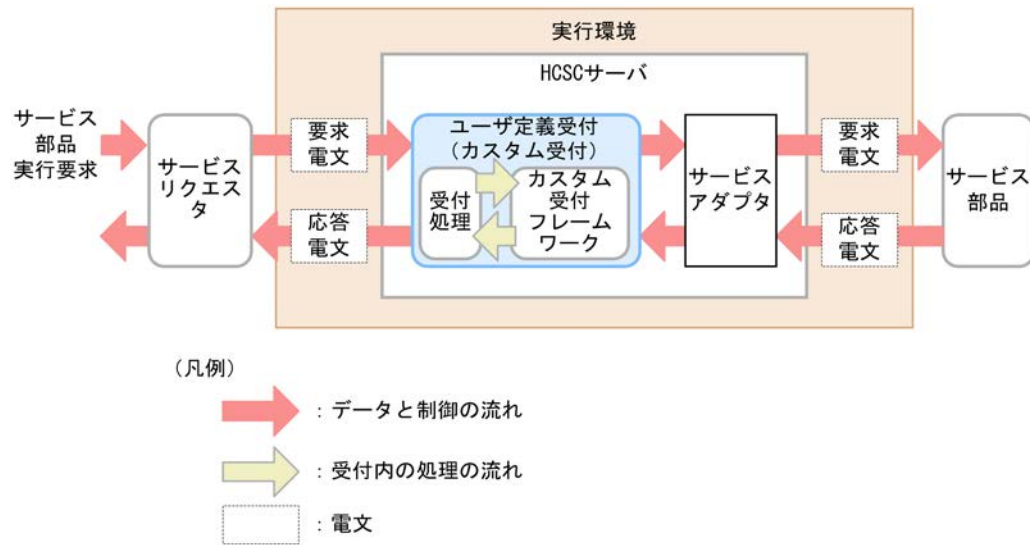
図 9-10 カスタム受付を使用したサービス部品の実行
