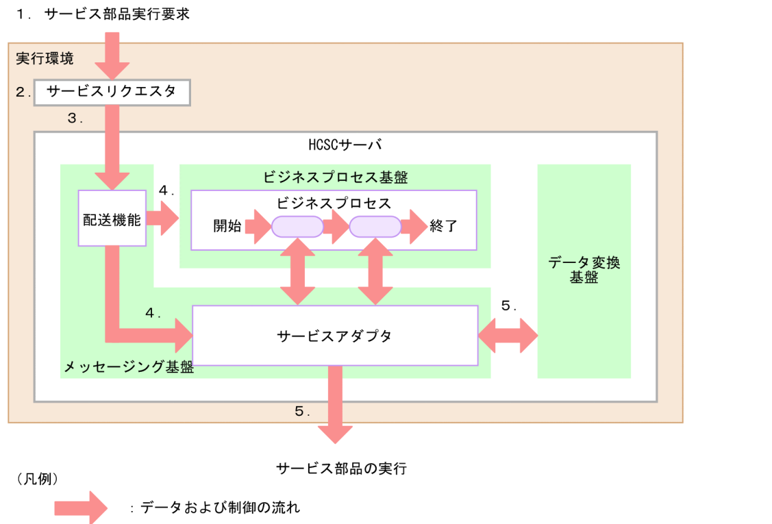
図 10-9 実行環境での制御の流れ
