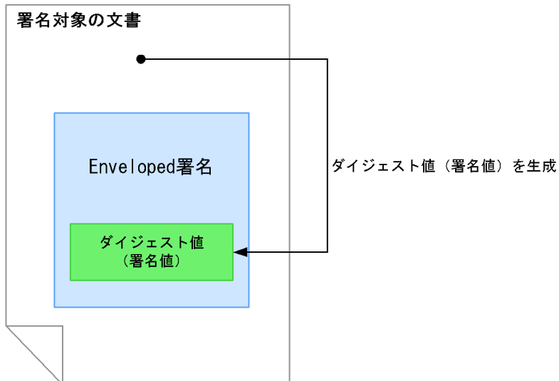
図 3-1 Enveloped 署名と署名対象の文書の間
