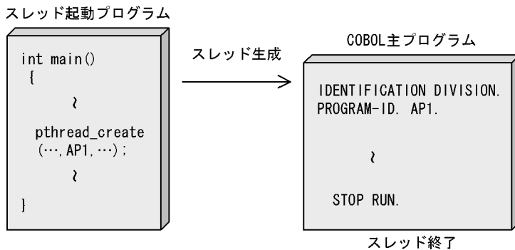
図 25-2 COBOL プログラムがスレッド開始関数となる例
