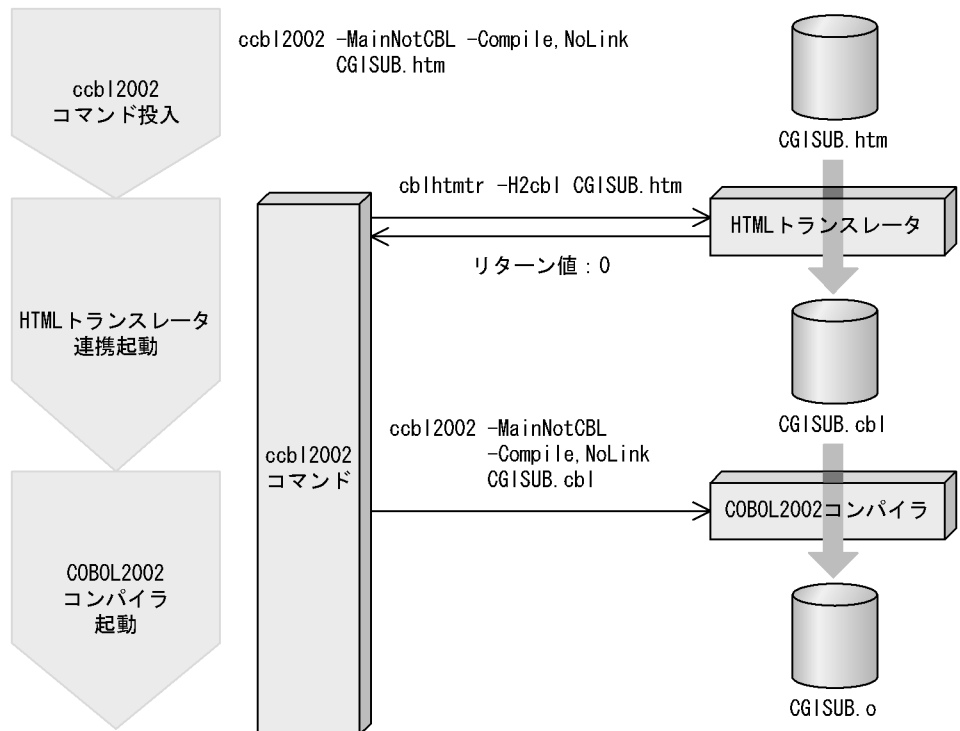
図 24-5 ccb12002 コマンドで HTML ファイルをコンパイルするときの流れ
