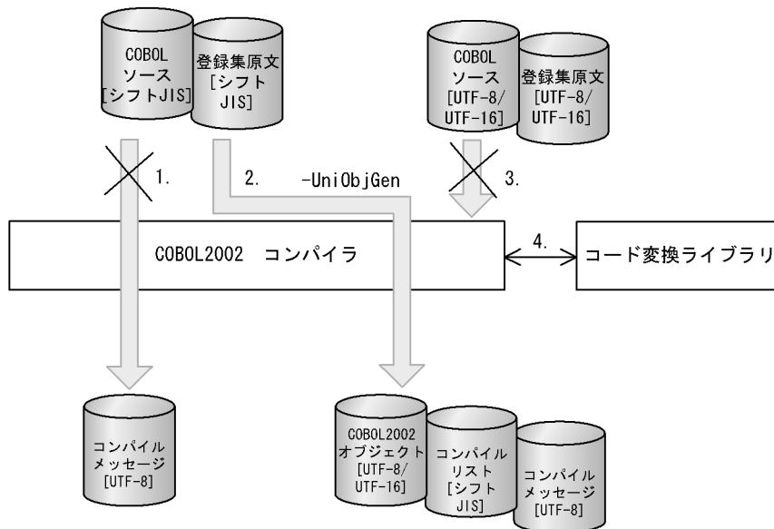
図 26-2 コンパイルでの Unicode 機能 ( UTF-8 環境下 )
