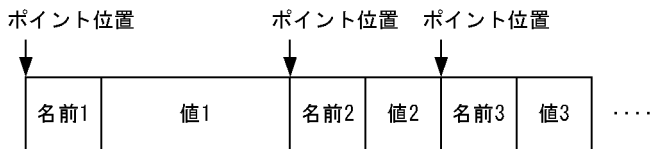
図 24-4 CGI リストの構造
