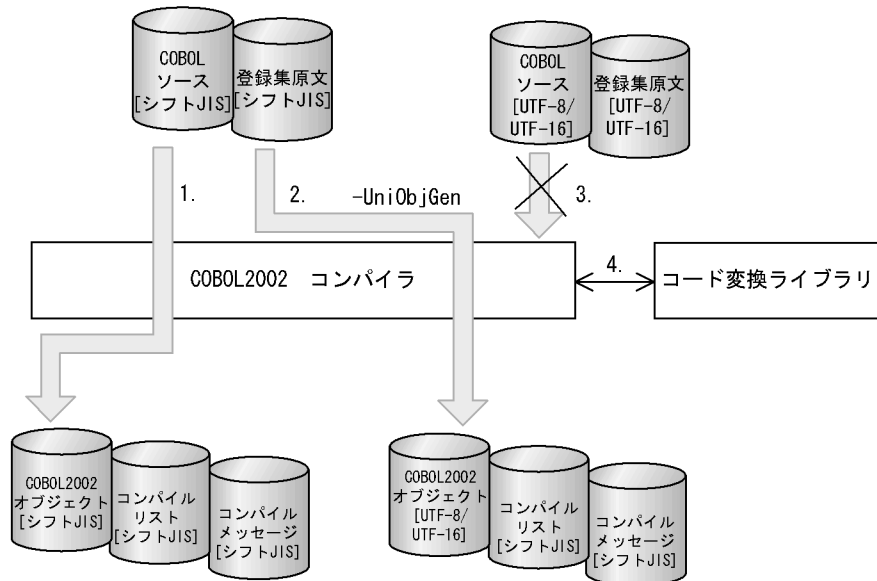
図 26-1 コンパイルでの Unicode 機能 ( シフト JIS 環境下 )
