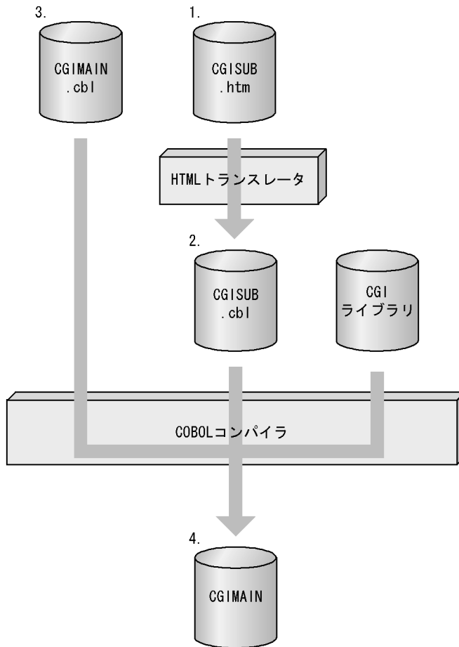
図 24-1 スタティック型 CGI プログラムの作成手順
