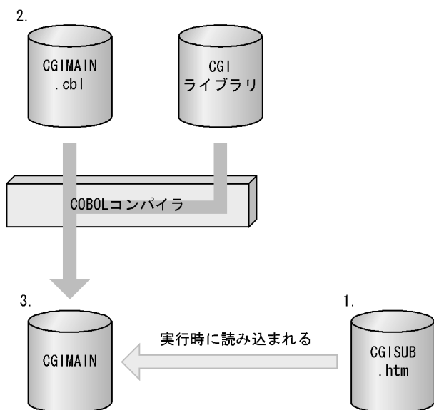
図 24-2 インタプリット型 CGI プログラムの作成手順
