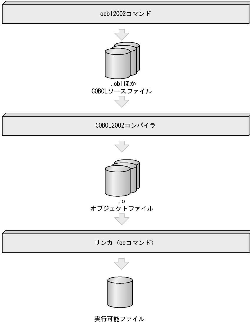
図 31-1 コンパイル時の入出力の流れ
