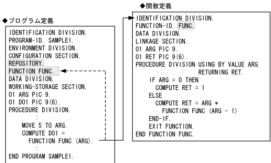
図 2-1 関数定義
