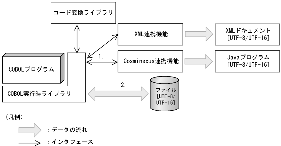
図 26-3 プログラム実行時の Unicode 機能
