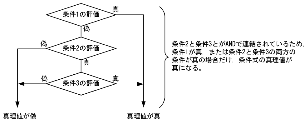
図 5-3 条件 1 OR 条件 2 AND 条件 3 の評価
