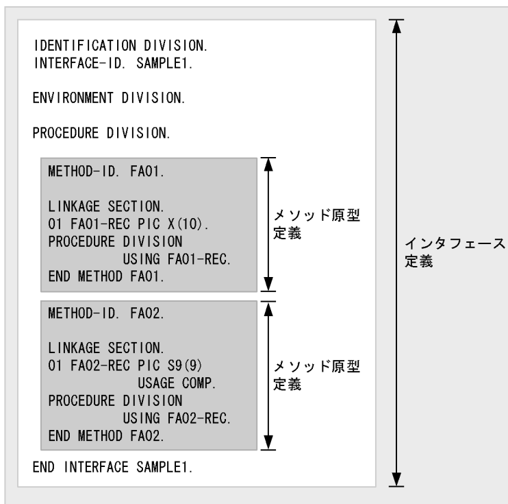
図 3-5 インタフェース定義
