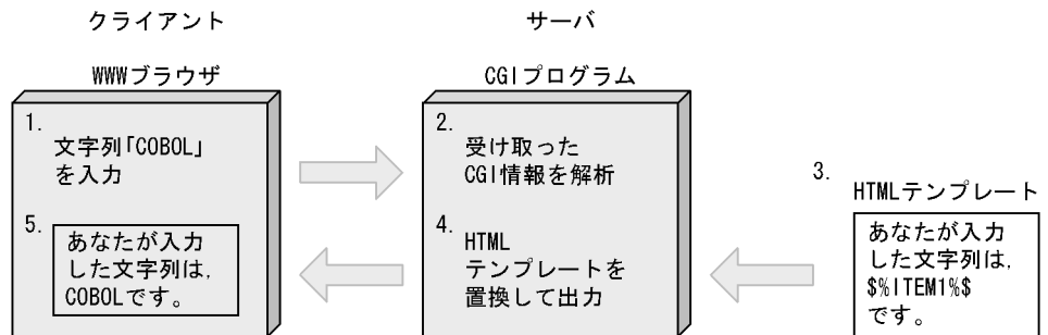
図 24-6 HTML テンプレート機能で動的な Web ページが出力される例
