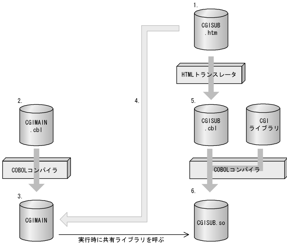
図 24-3 ダイナミック型 CGI プログラムの作成手順
