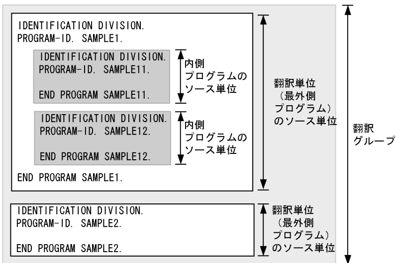
図 3-1 翻訳グループの構成
