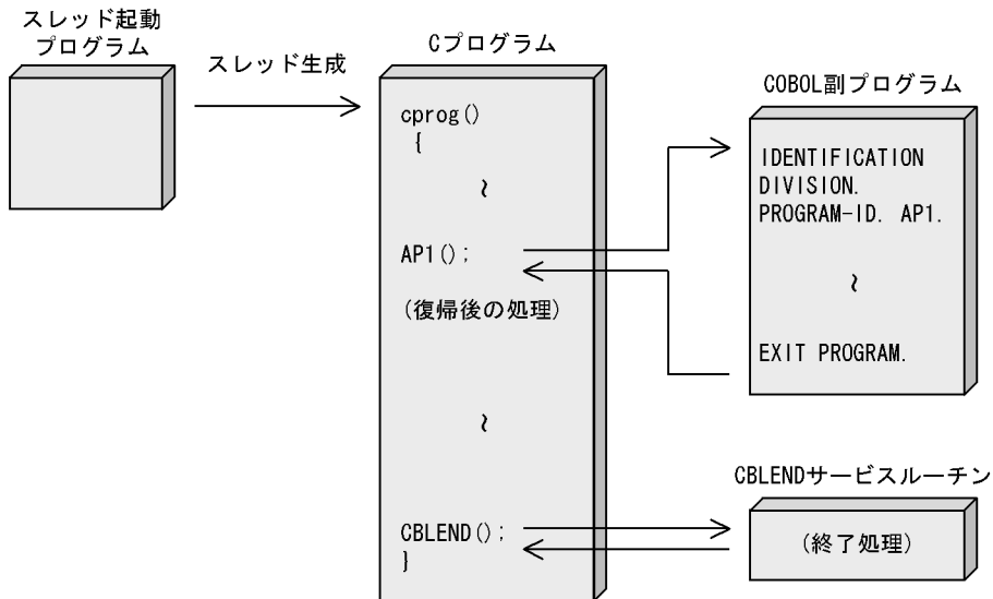
図 25-1 COBOL 以外のプログラムからの呼び出しの例
