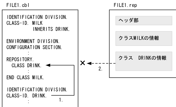
図 32-3 同じソースファイル中の翻訳単位名の検索の例
