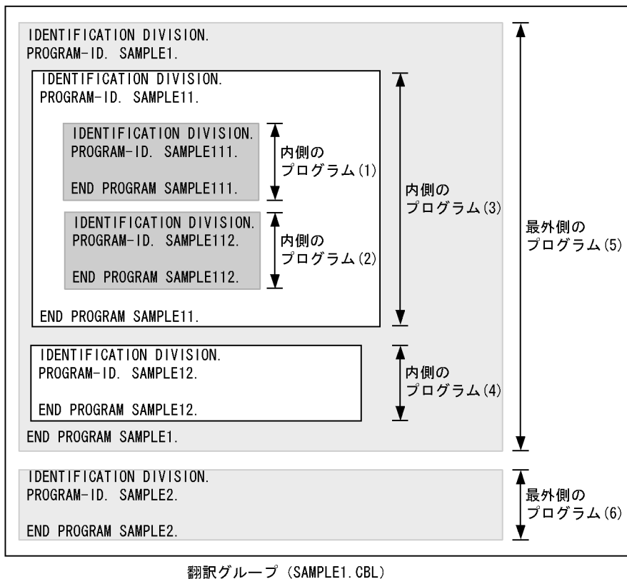
図 3-2 翻訳単位の考え方
