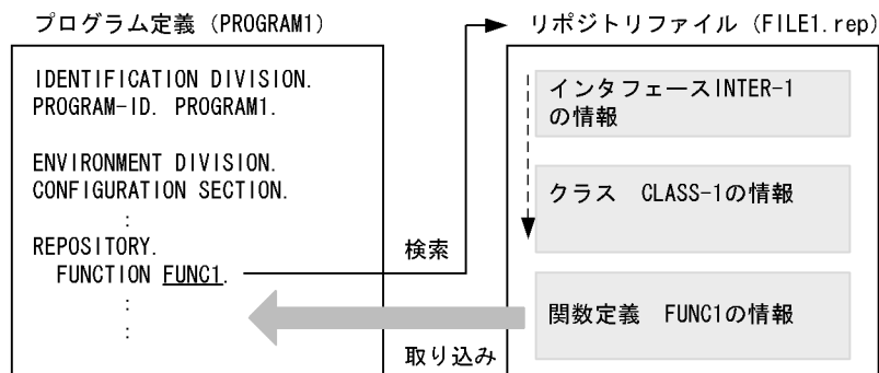
図 32-2 リポジトリファイルとリポジトリ段落の関係
