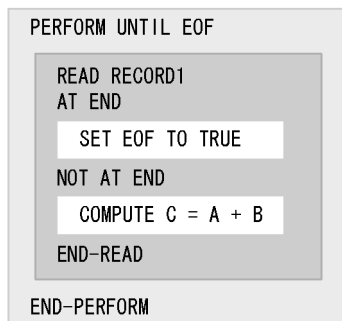
図 21-4 文の範囲
