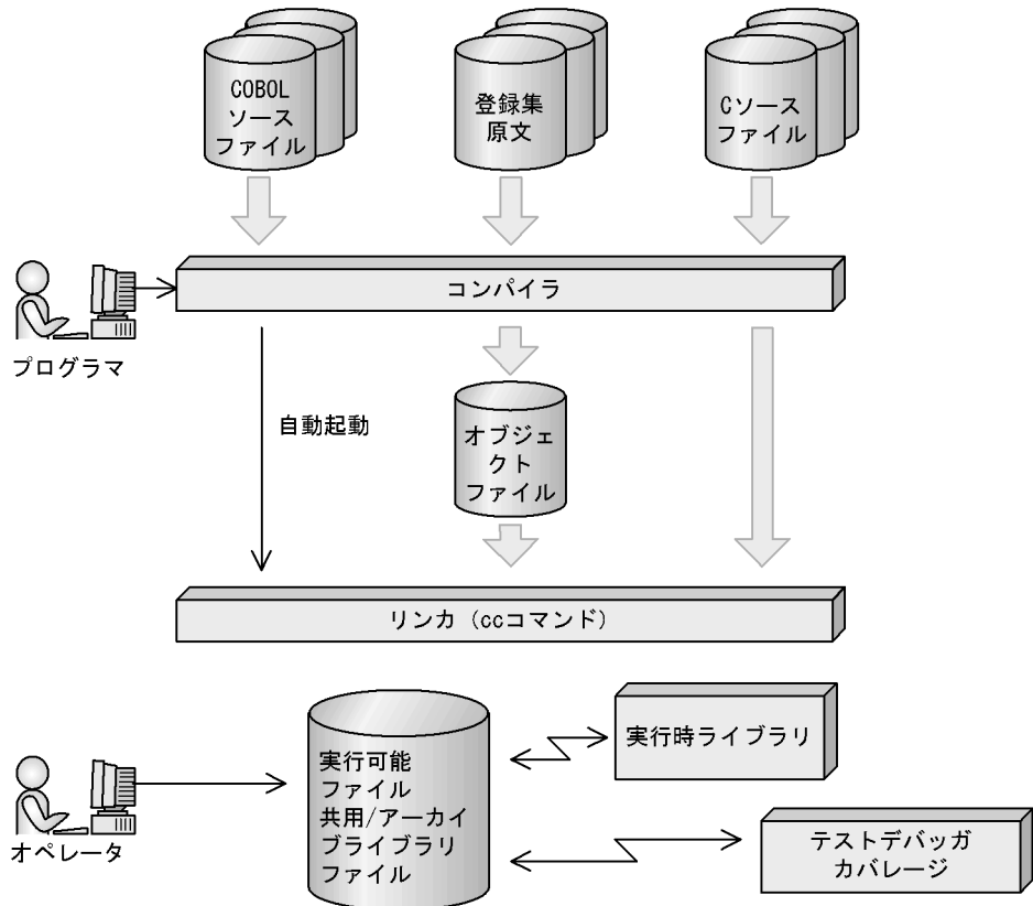
図 1-1 COBOL2002 の構成
