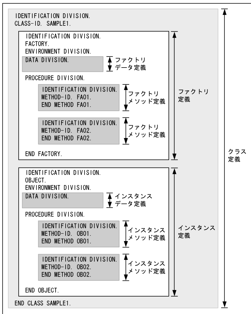
図 3-4 クラス定義
