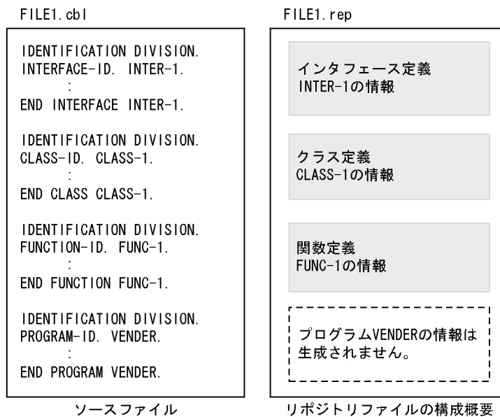
図 32-1 ソースファイルとリポジトリファイルの関係
