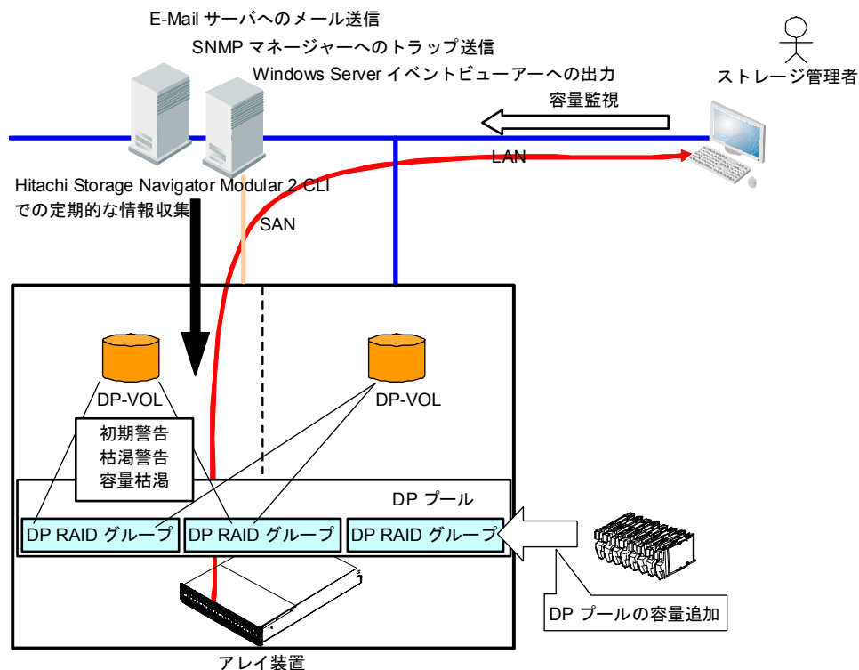
図 2-7 DP プールの使用容量警告監視の概念図
