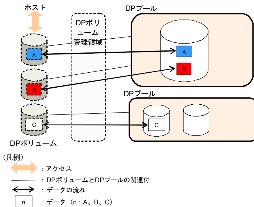
図 2-1 DP プールと DP ボリュームの関係
