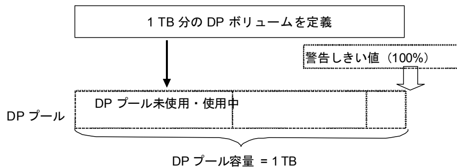
図 2-10 警告しきい値が 100%の場合の DP プール容量
