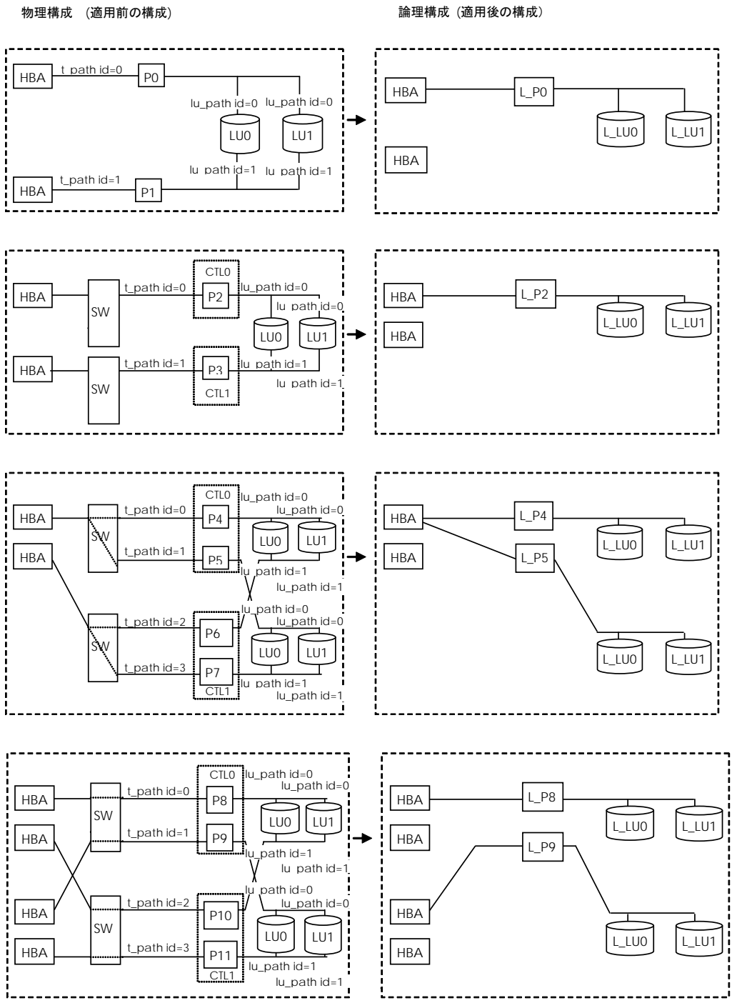
図 2-1 構成図
