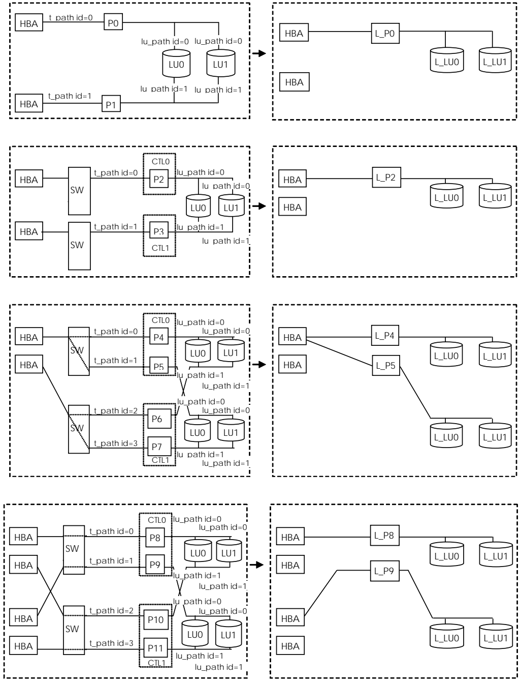
図 2-1 構成図
