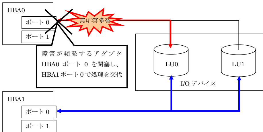
図 12 障害による HBA ポート閉塞
