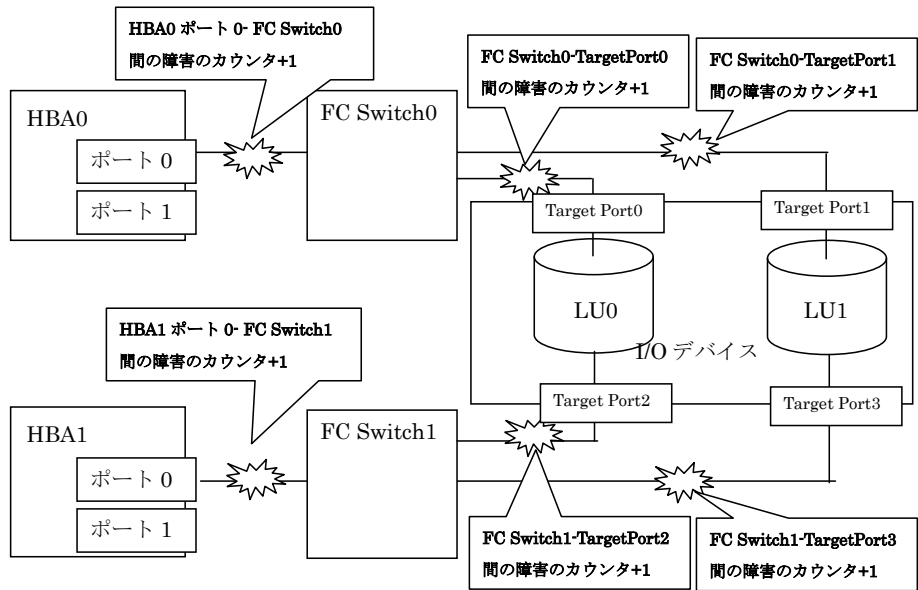
図 10 LinkDown 障害カウンタの管理単位(VMware FC Switch-HBA 間、FC Switch-I/O 間の LinkDown 発生時)
