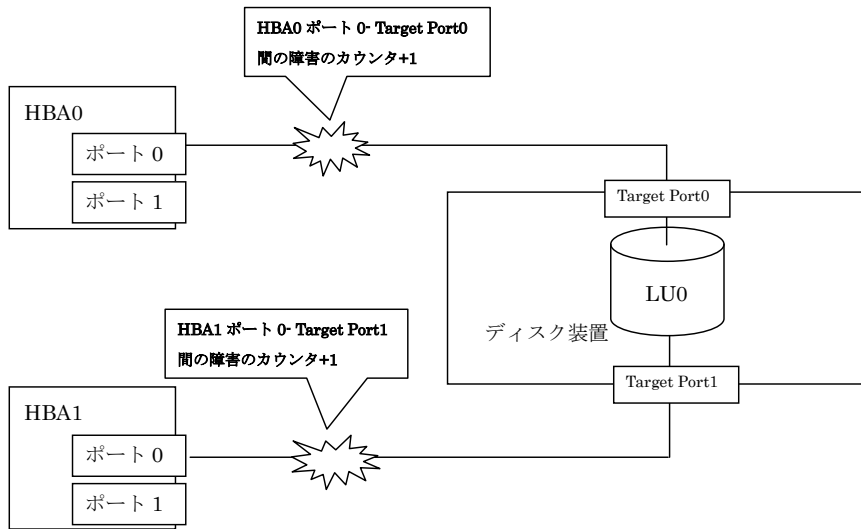
図 9 LinkDown 障害カウンタの管理単位(VMware HBA-I/O 間の LinkDown 発生時)
