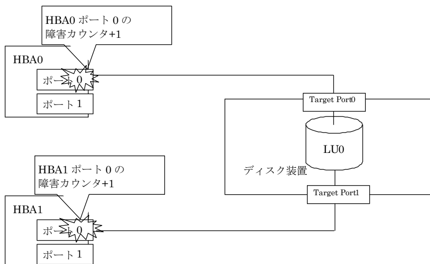
図 8 監視対象の HBA 障害
