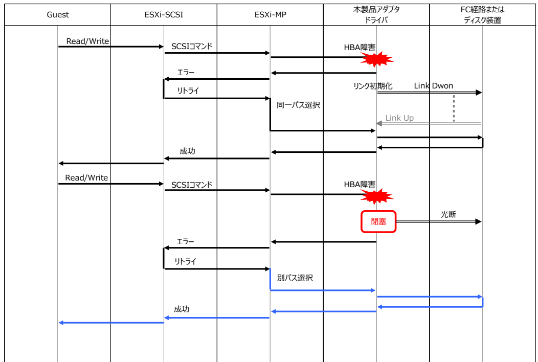
図 13 HBA 障害の閾値設定
