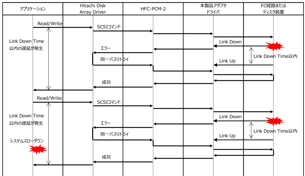
図 1 瞬断が繰り返し発生したケース
