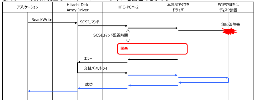
図 16 タイムアウト障害の閾値設定
