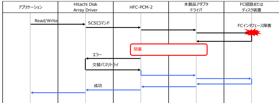
図 15 FC インタフェース障害の閾値設定
