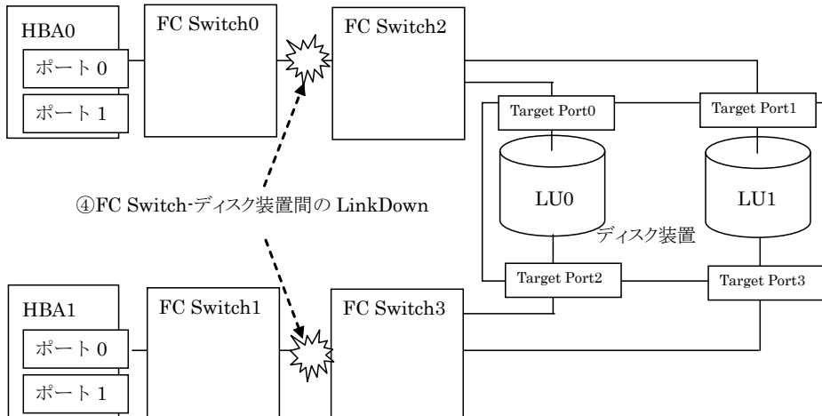
図 7 監視対象の LinkDown(FC Switch 構成(カスケード接続))
