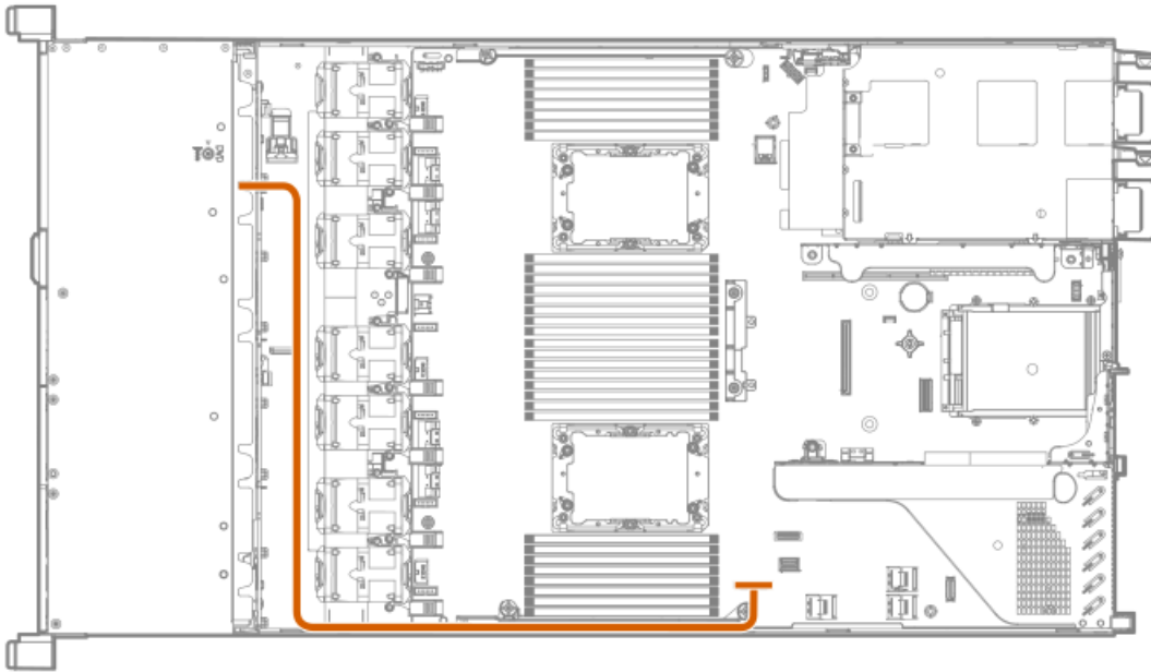
SFF (2.5型) オプティカルディスクドライブのケーブル接続
