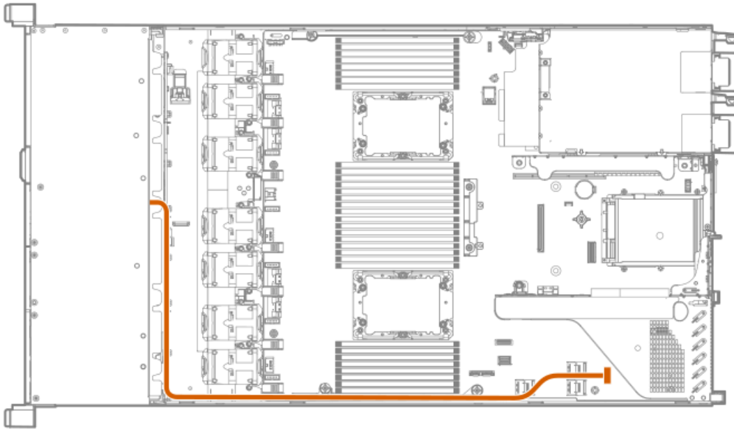
フロント電源/SID/USBケーブル接続
