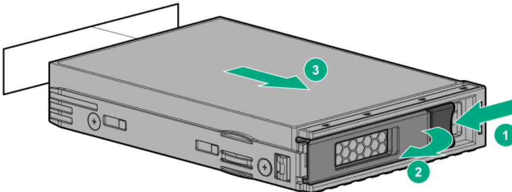
図 2. LFF (3.5型) ドライブ
