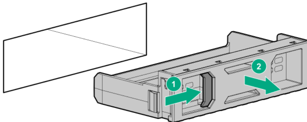
図 2. LFF (3.5型) ドライブblankを取り外す
