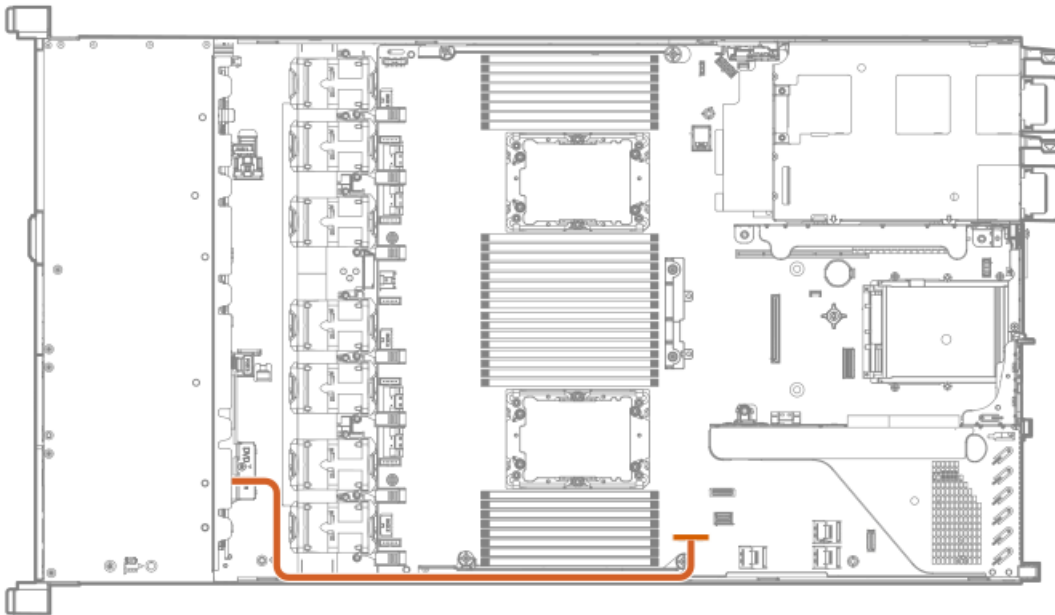
LFF (3.5型) フロントディスプレイポート/USBケーブル接続
