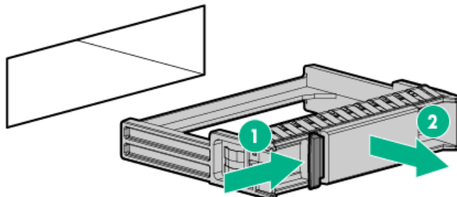
図 1. SFF (2.5型) ドライブblankを取り外す
