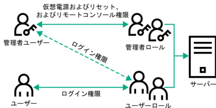
図6: 複数の（重複する）ロール
