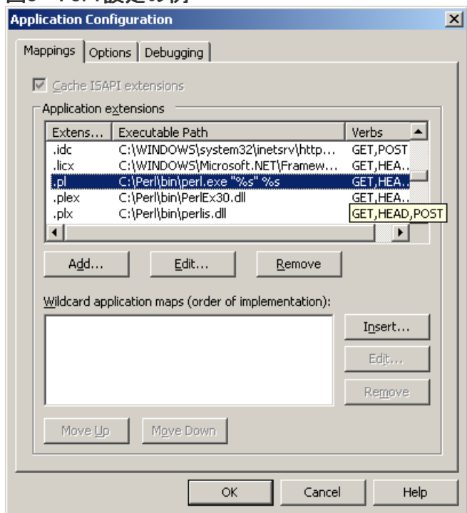
図3: Perl設定の例
