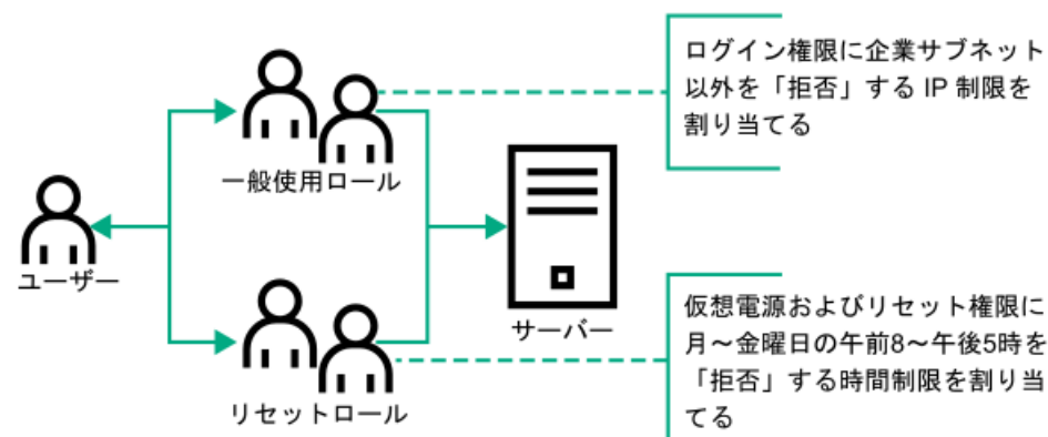
図10: 制限およびロールの作成
