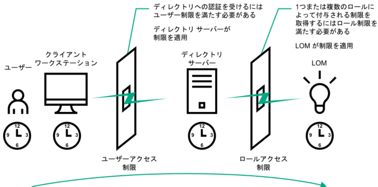
図8: ディレクトリのログイン制限
